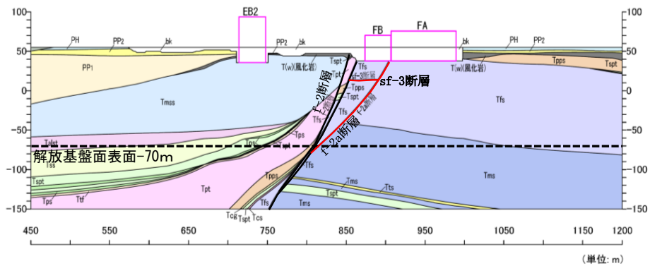
第3-2図 岩盤分類図 (EW4断面) (21/35)
