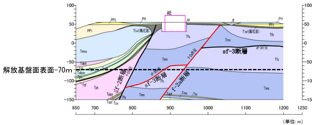
第 3-2 図 岩盤分類図 (NS17 断面) (17/35)
