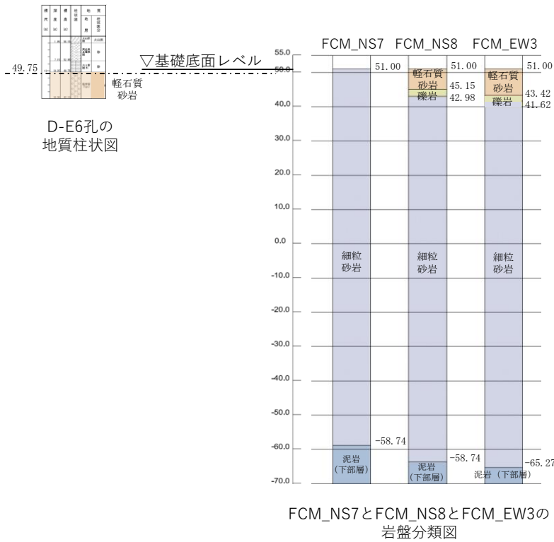
第 4-2 図 D-E6 及び FCM 直下の岩盤分類図の対応
