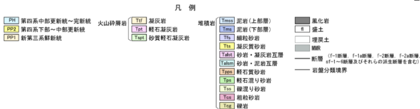
第3-2図 岩盤分類図 (EW5断面) (22/35)
