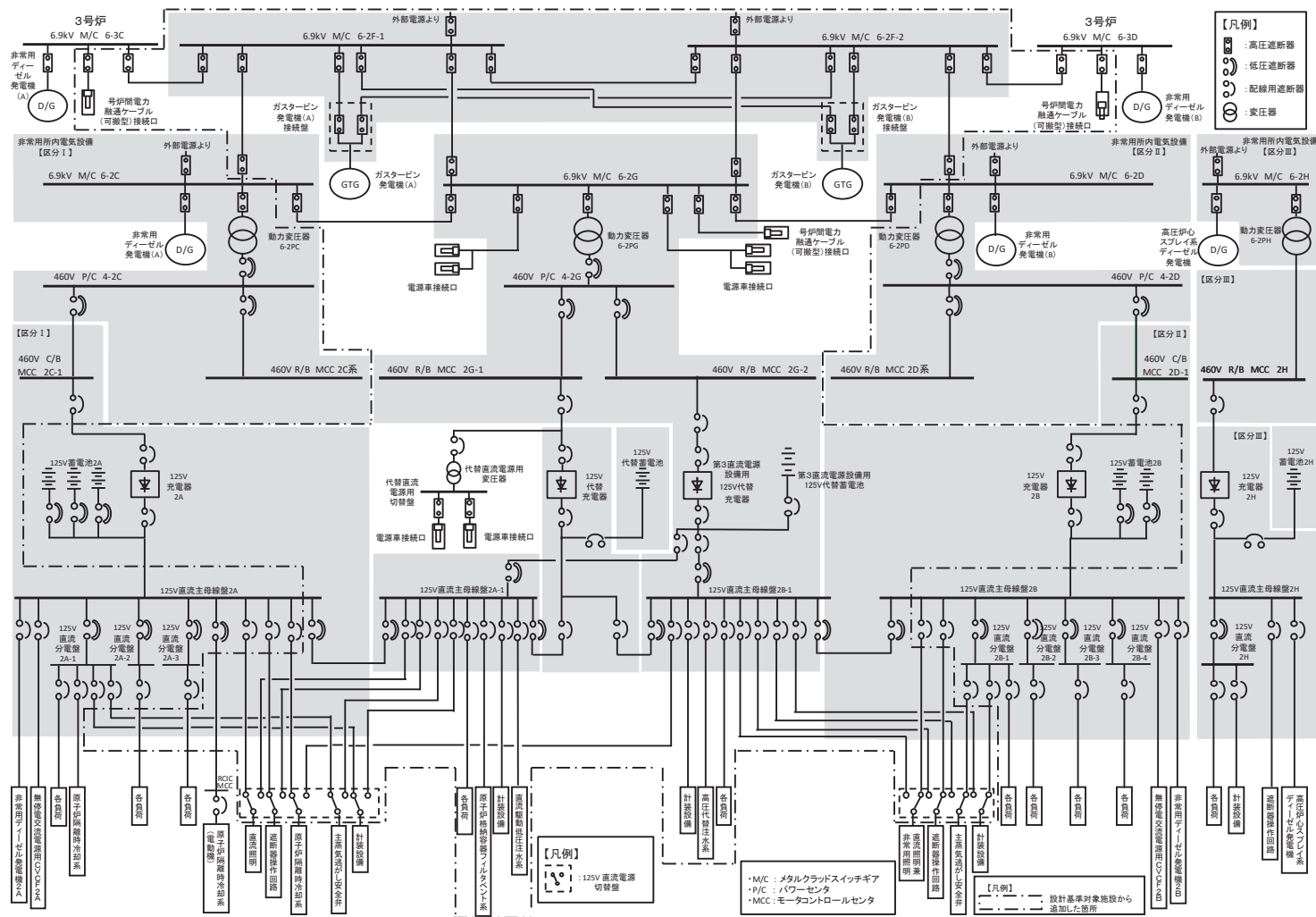
第 1. 14-3 図 直流通源単線結線図 (125V 系統)
