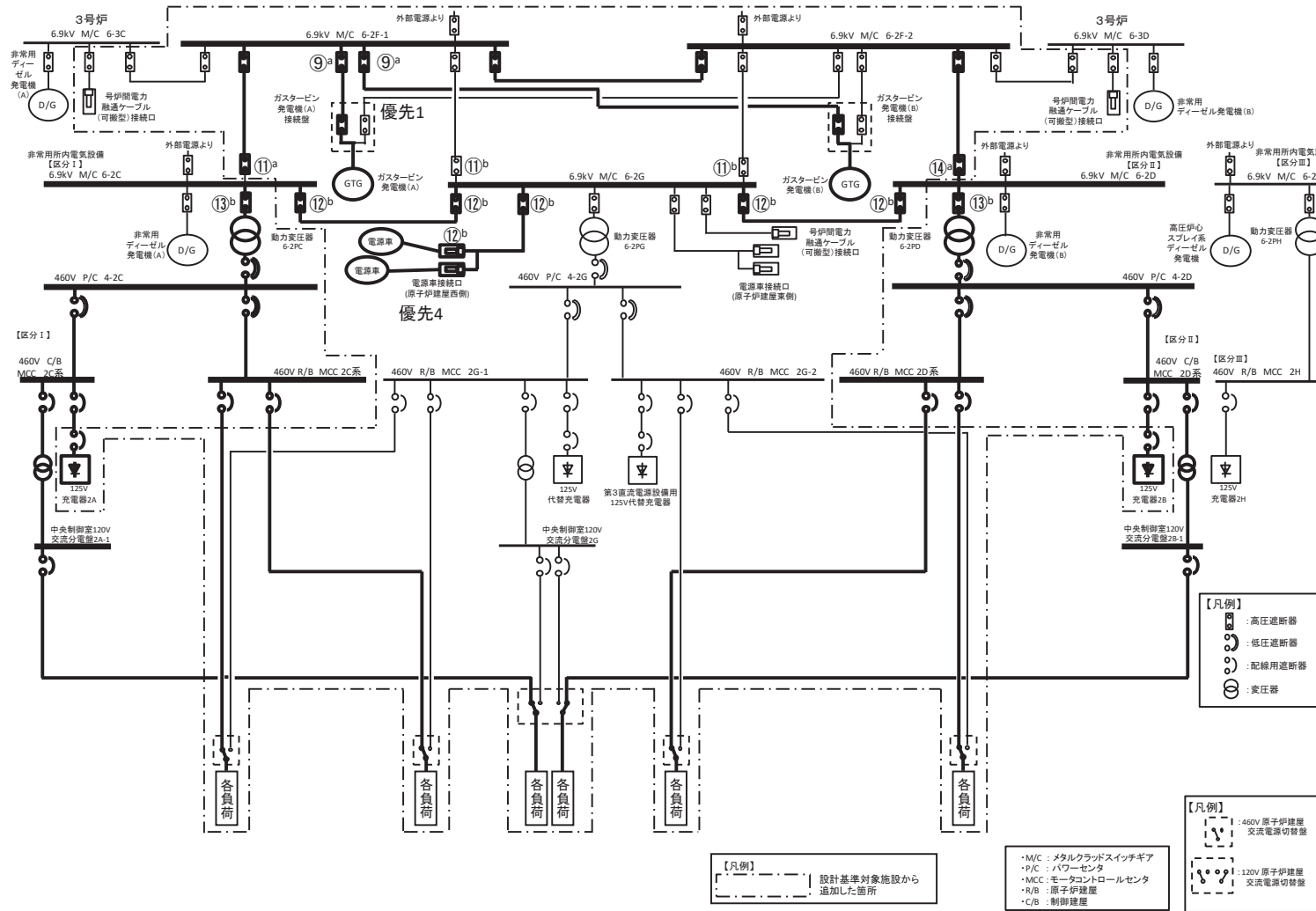
第 1. 14-6 図 ガスタービン発電機又は電源車によるメタクラ 2C 系及びメタクラ 2D 系受電 概要図
