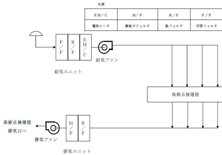
第20図 保守点検建屋換気系統概要図
