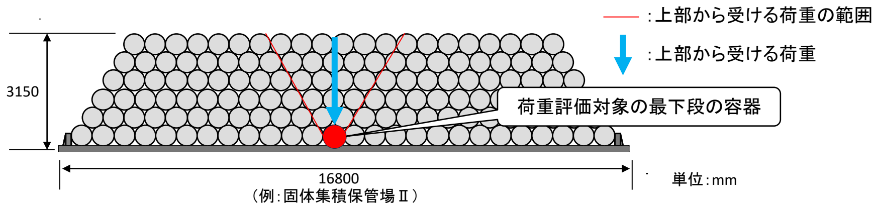
ドラム缶型廃棄物パッケージ(横積み)の荷重評価モデル
