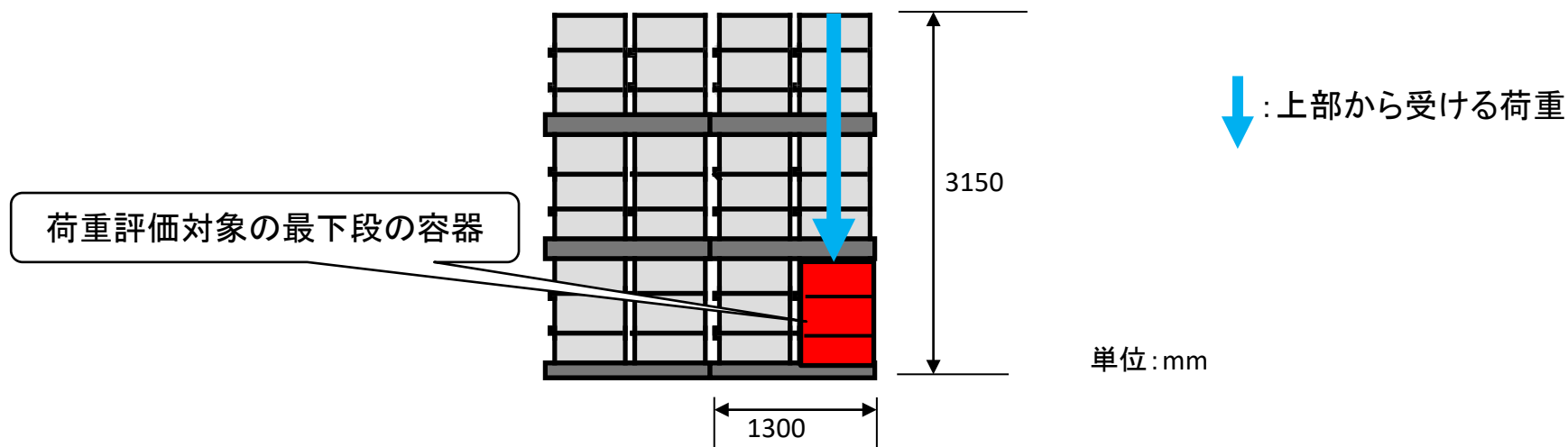
ドラム缶型廃棄物パッケージ(縦積み)の荷重評価モデル
