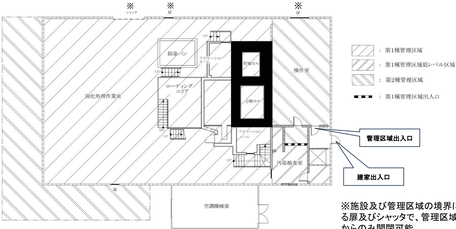
β・γ 固体処理棟Ⅳ 1階平面図
