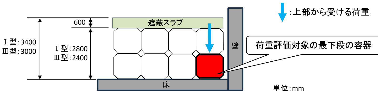
ブロック型廃棄物パッケージの荷重評価モデル
