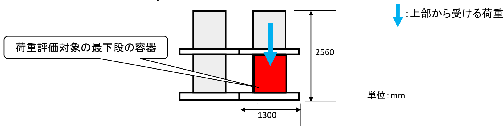
角型鋼製廃棄物パッケージの荷重評価モデル
