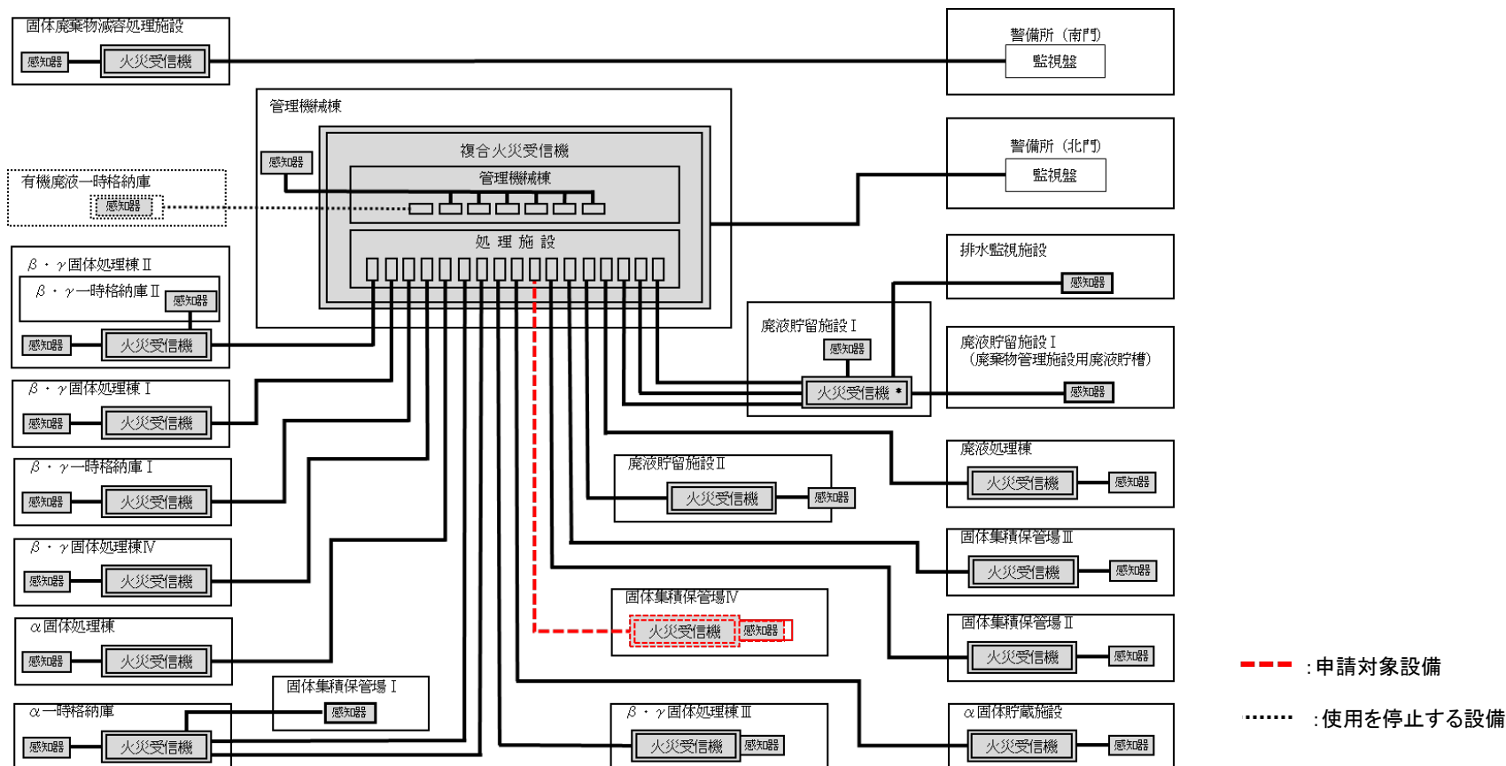
廃棄物管理施設の自動火災報知設備系統図
