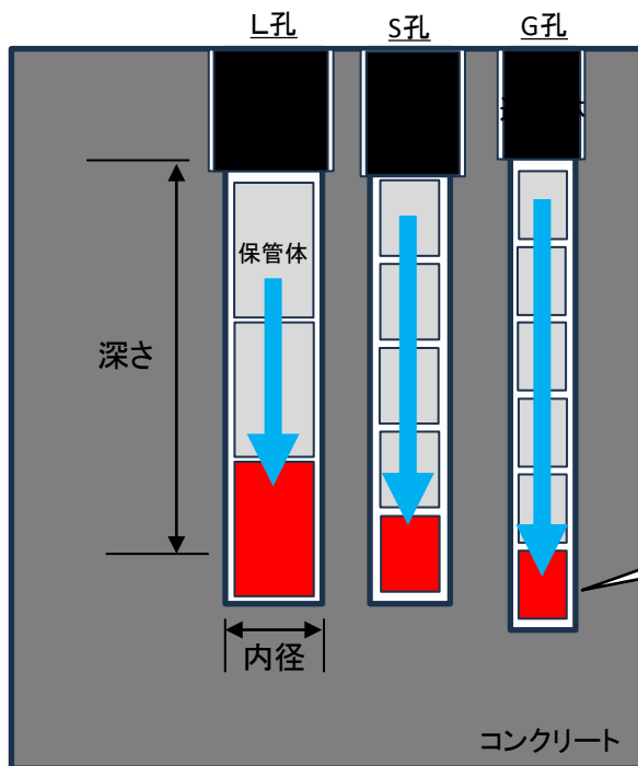
保管体の荷重評価モデル
