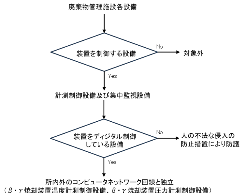
不正アクセス行為対象設備選定フロー図
