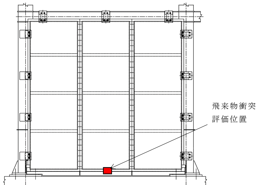
第 2-10 図 相対する 2 辺以上で支持する防護板 飛来物衝突評価位置
