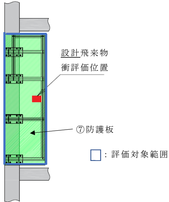
第2-30図 1辺で支持する防護板 設計飛来物衝突評価(水平)位置
