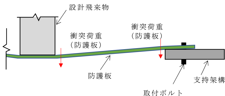
第2-29図 防護板に作用する荷重
