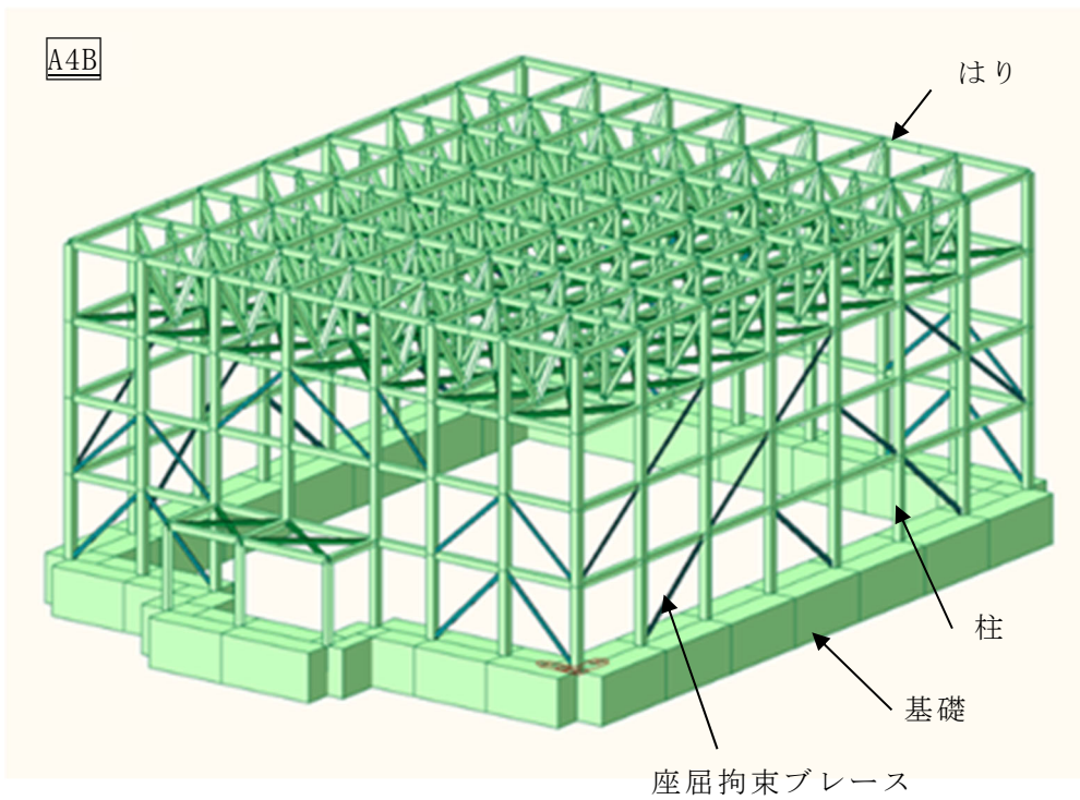
第2-34図 支持架構の構造概要(2/2)
