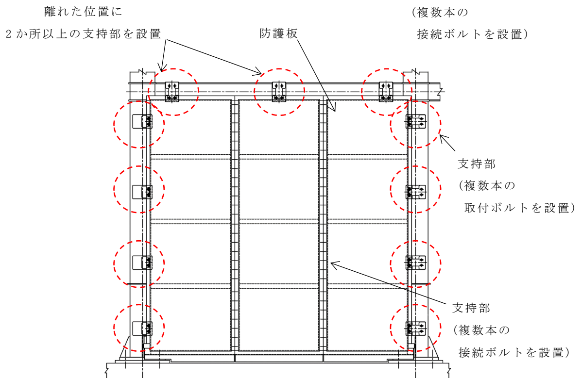
第2-8図 支持部の配置(2/2)
