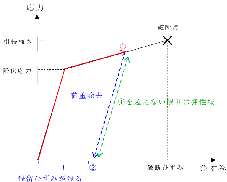
第 2 -33図 取付ボルトの応力-ひずみ線図
