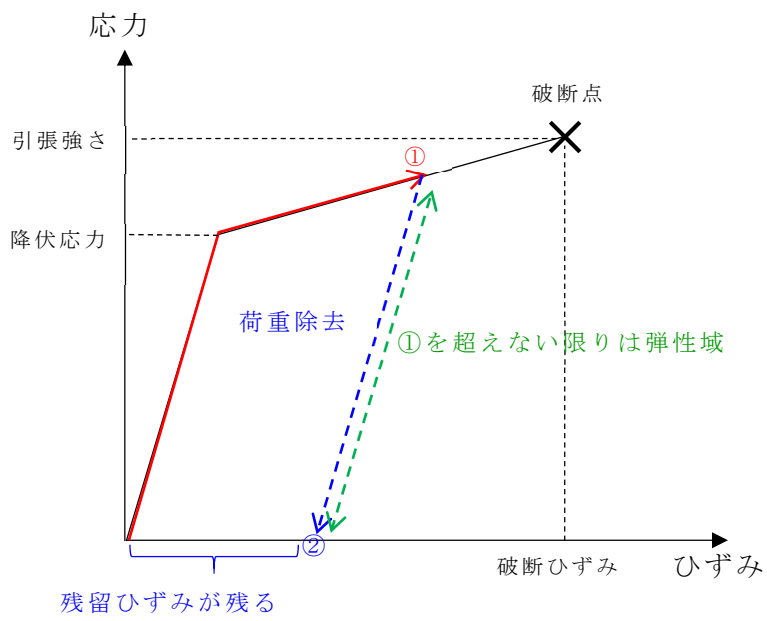
第 2-11 図 取付ボルトの応力-ひずみ線図
