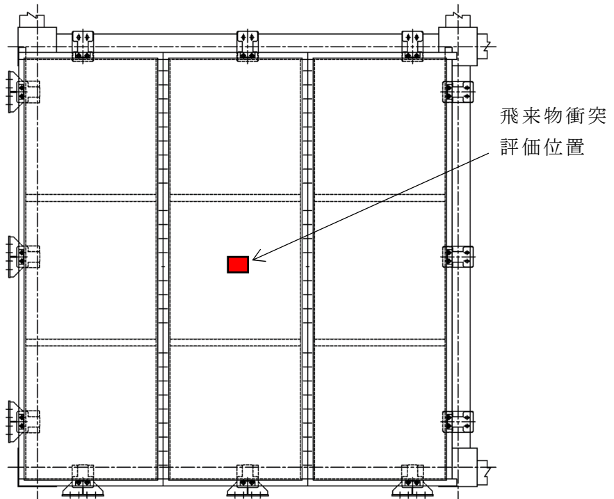
第 2 - 9 図 4 辺で支持する防護板 飛来物衝突評価位置
