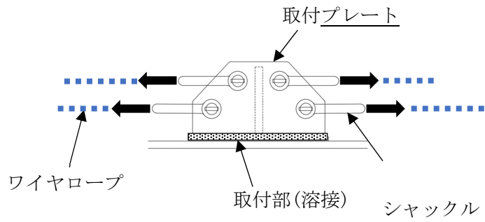
第3-2図 取付プレートへの荷重作用状況
