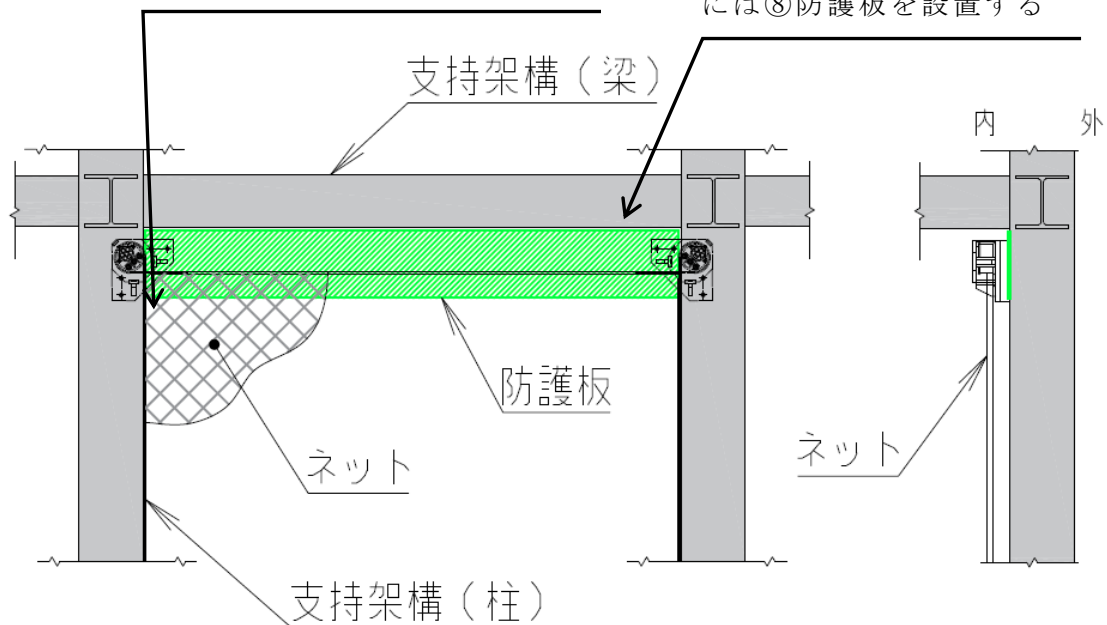
第2-19図 ⑥防護板及び⑧防護板の設置状況
