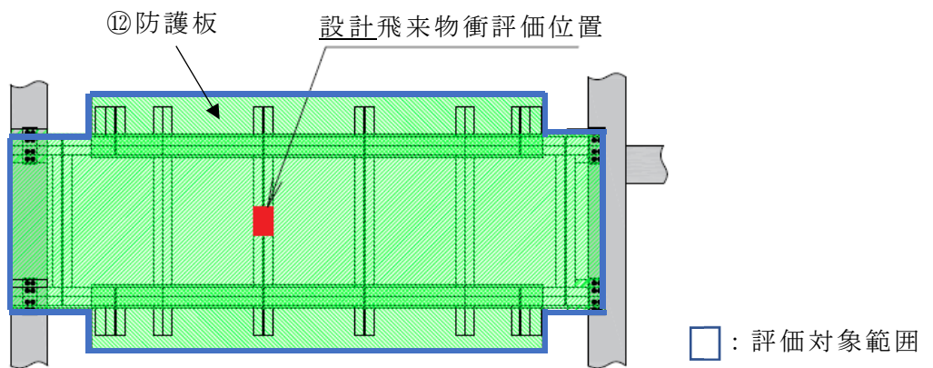
第2-31図 相対する2辺以上で支持する防護板 設計飛来物衝突評価(鉛直)位置
