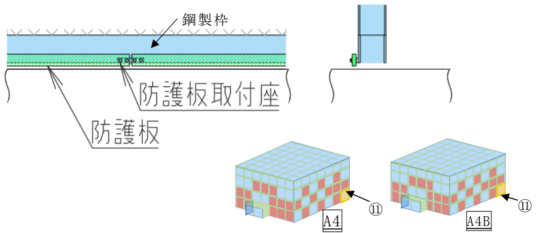
第 2 -11 図 ⑪防護板 (③用, 外取付)
