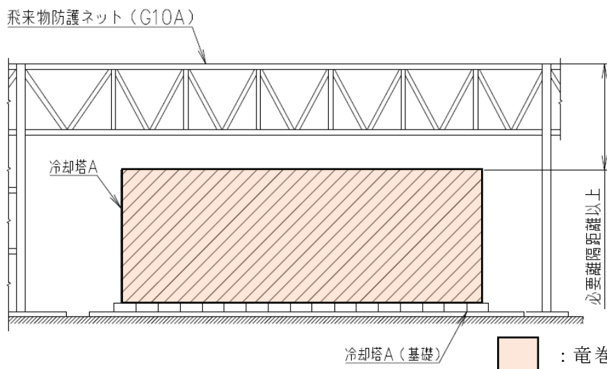
第 2-2 図 冷却塔 A と飛来物防護ネット (G10A) の配置図
