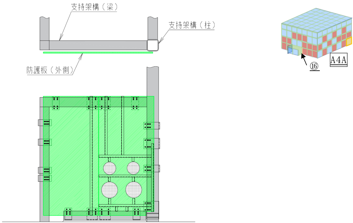
第 2 - 15 図 ⑬防護板 (張出部南側面, 配管貫通部, 外取付)
