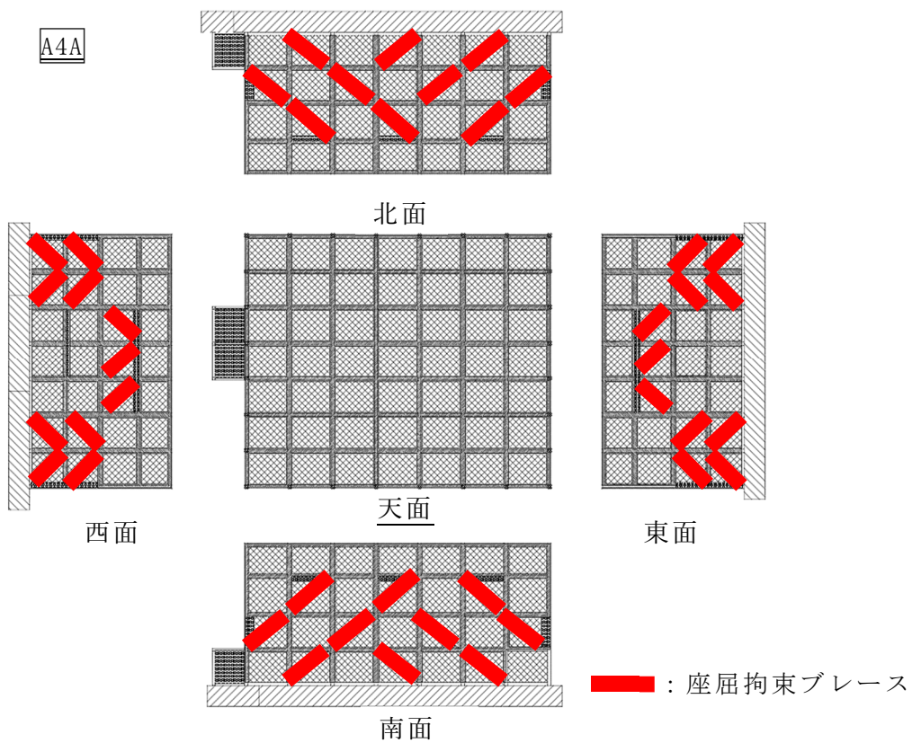
第 2 -36図 座屈拘束ブレースの配置概要(1/2)
