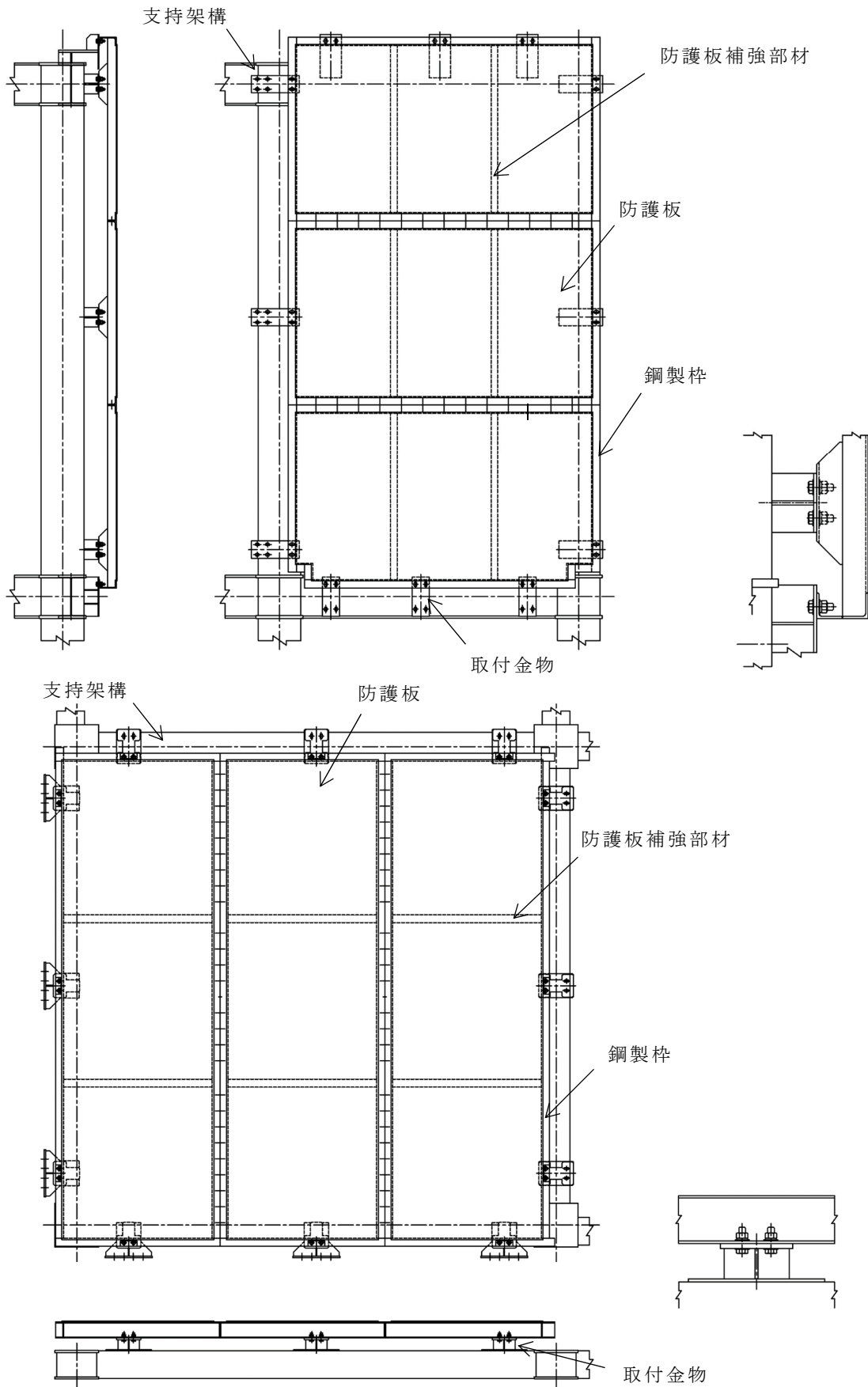
第 2 - 5 図 防護板 (4 辺で支持)
