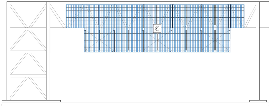
第 2 - 3 図 防護ネット及び防護板割付図 (5/5)
