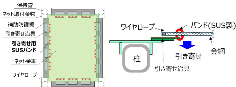
第3-1図 防護ネットの引き寄せ装置
