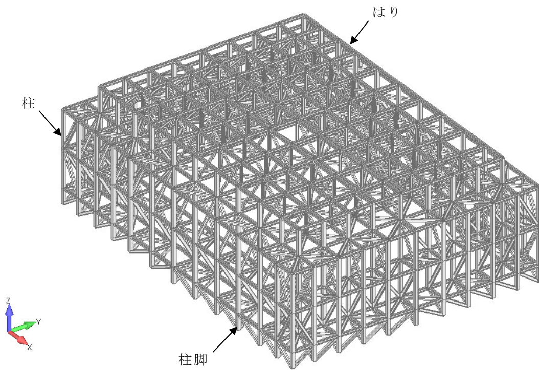
飛来物防護ネット (F1A)
