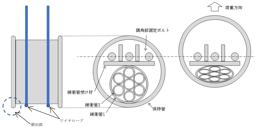
第3-3図 保持管の構造 (左：変形前, 右：変形後)
