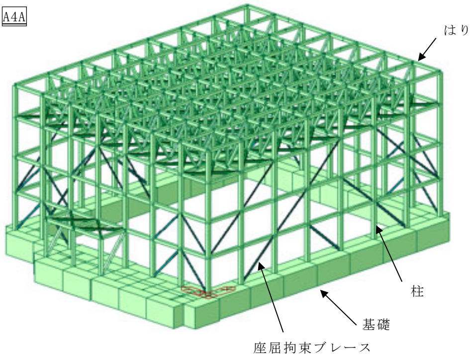
第2-34図 支持架構の構造概要(1/2)
