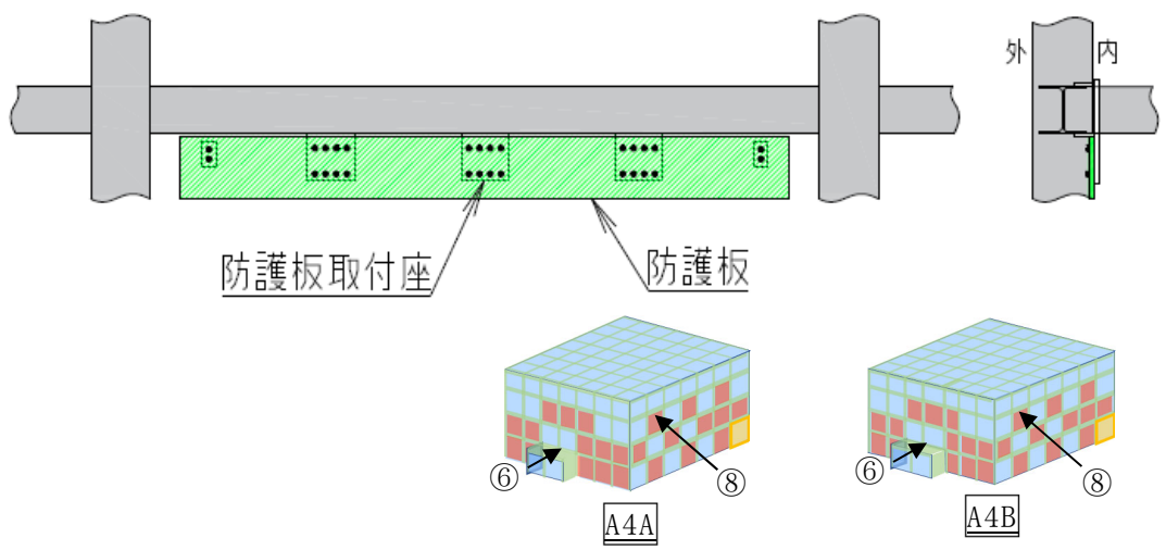
※⑥防護板(①用, 内取付)についても同一の構造である。 第 2-17 図 ⑧防護板(②用, 防護板補強無し, 内取付)
