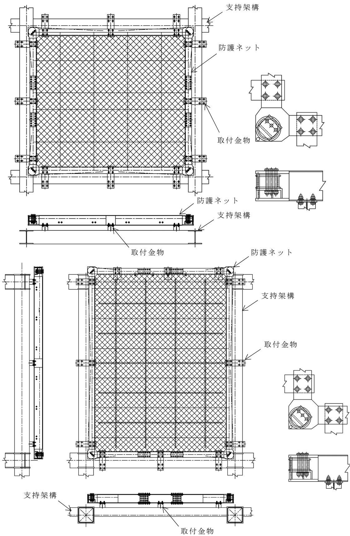
飛来物防護ネット (F1A) 第 2-4 図 防護ネットの構造概要 (1/2)
