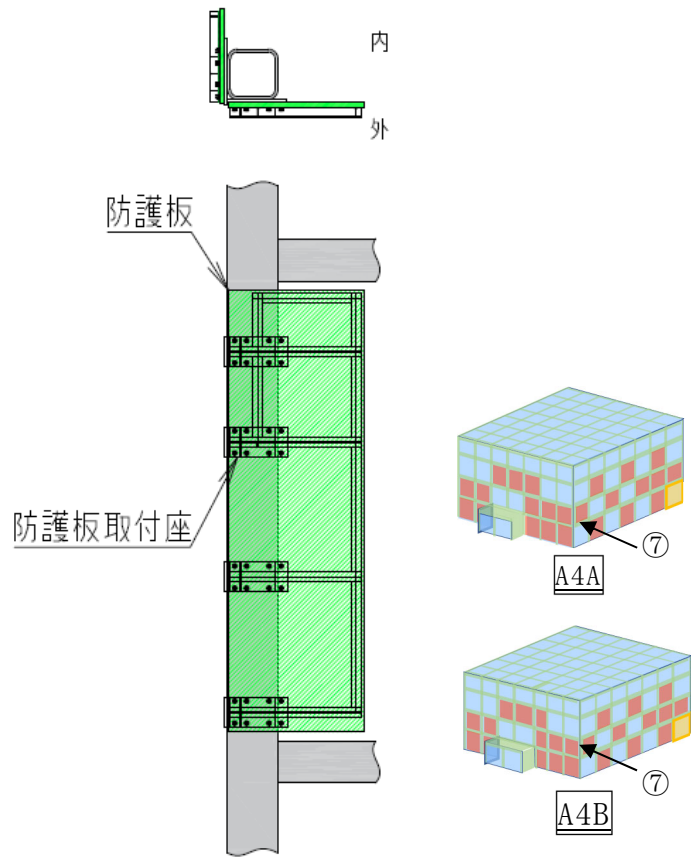
第 2-16 図 ⑦防護板(②用, 防護板補強有り, 外取付)
