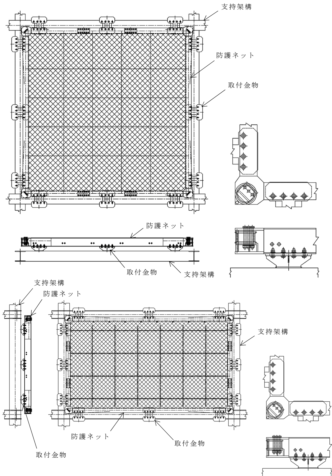
飛来物防護ネット (F1B) 第 2-4 図 防護ネットの構造概要 (2/2)
