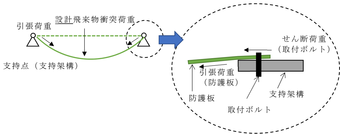
第 2 -25 図 防護板に大変形が生じた時点の支持部への作用荷重
