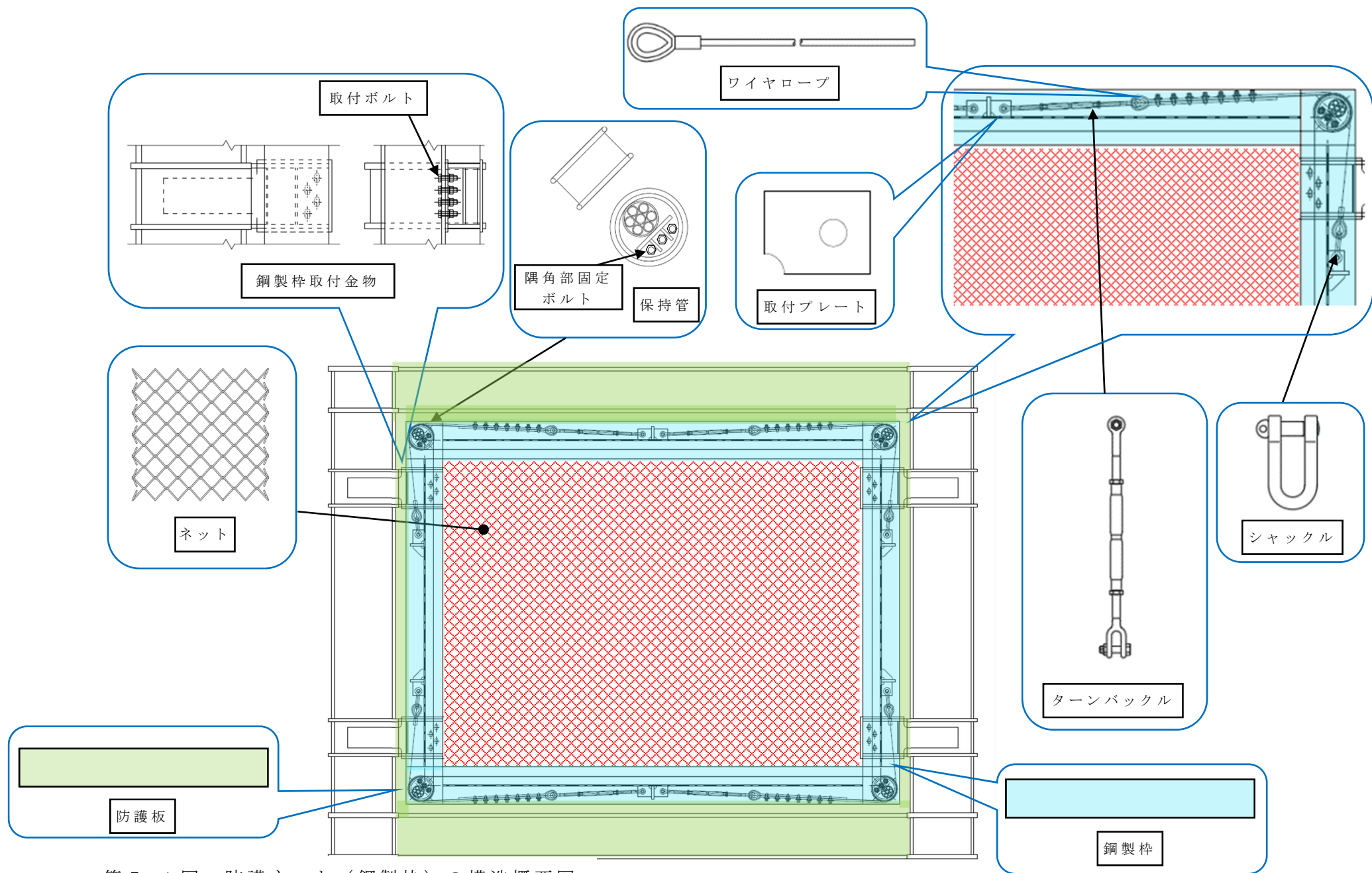
第5-1図 防護ネット（鋼製枠）の構造概要図
