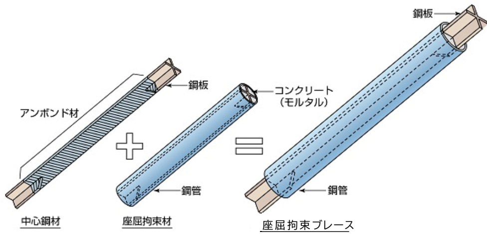
第 2 -35図 座屈拘束ブレースの構造概要
