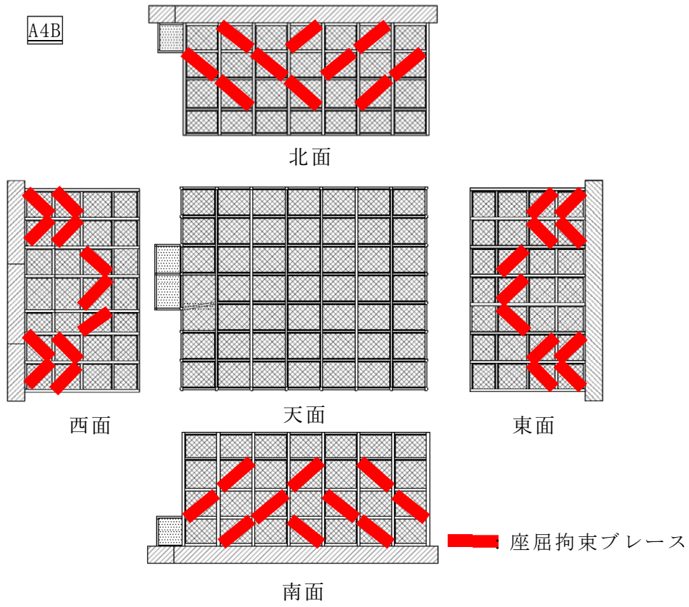
第 2 -36 図 座屈拘束ブレースの配置概要 (2/2)
