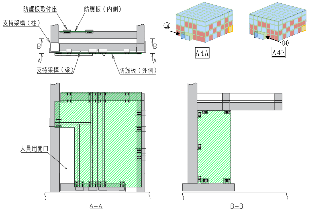
第 2-14 図 ⑭防護板(張出部, 人員用開口, 外取付)
