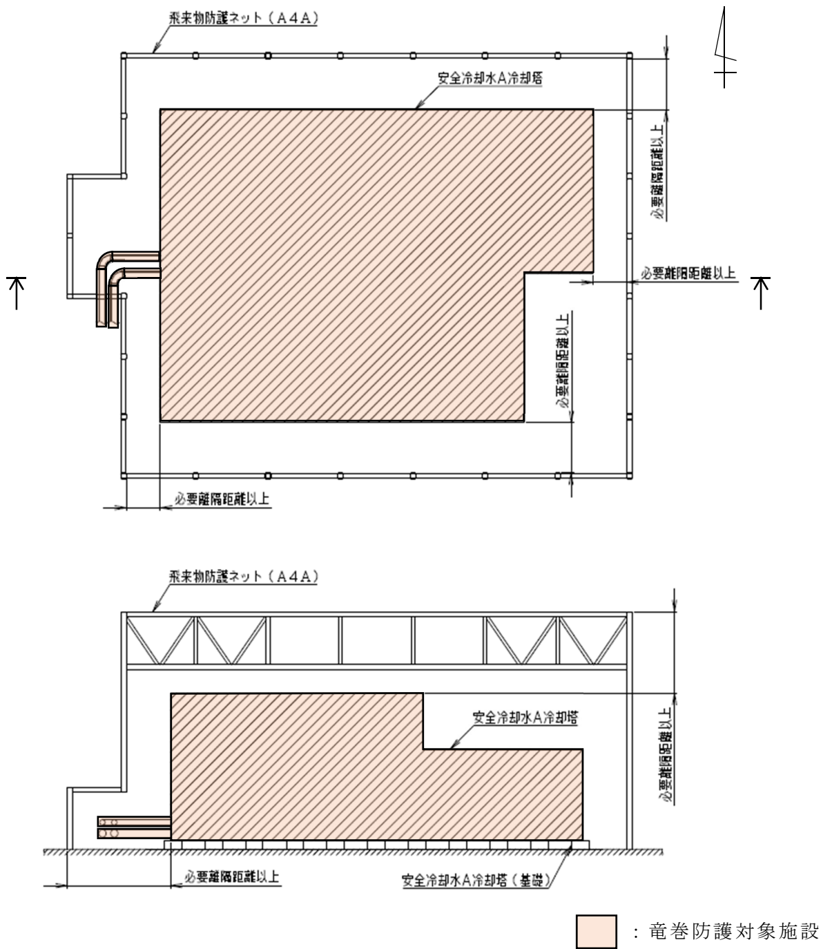
第2-2図 安全冷却水A,B冷却塔と飛来物防護ネット(A4A,B)の配置図(1/2)
