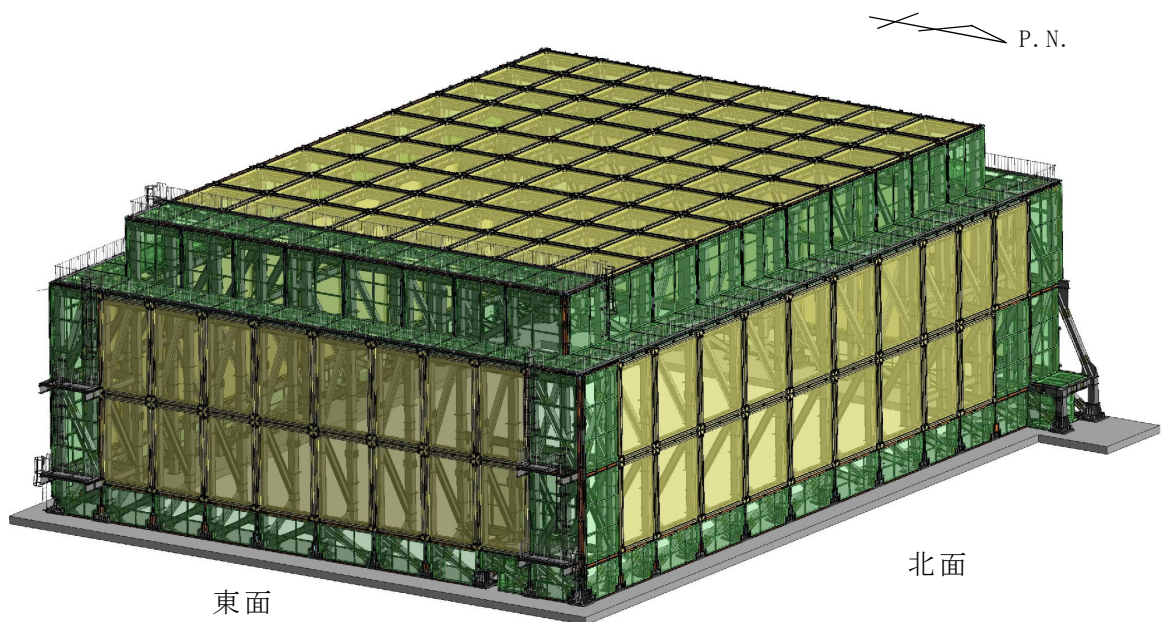
飛来物防護ネット (F1A) 全景
