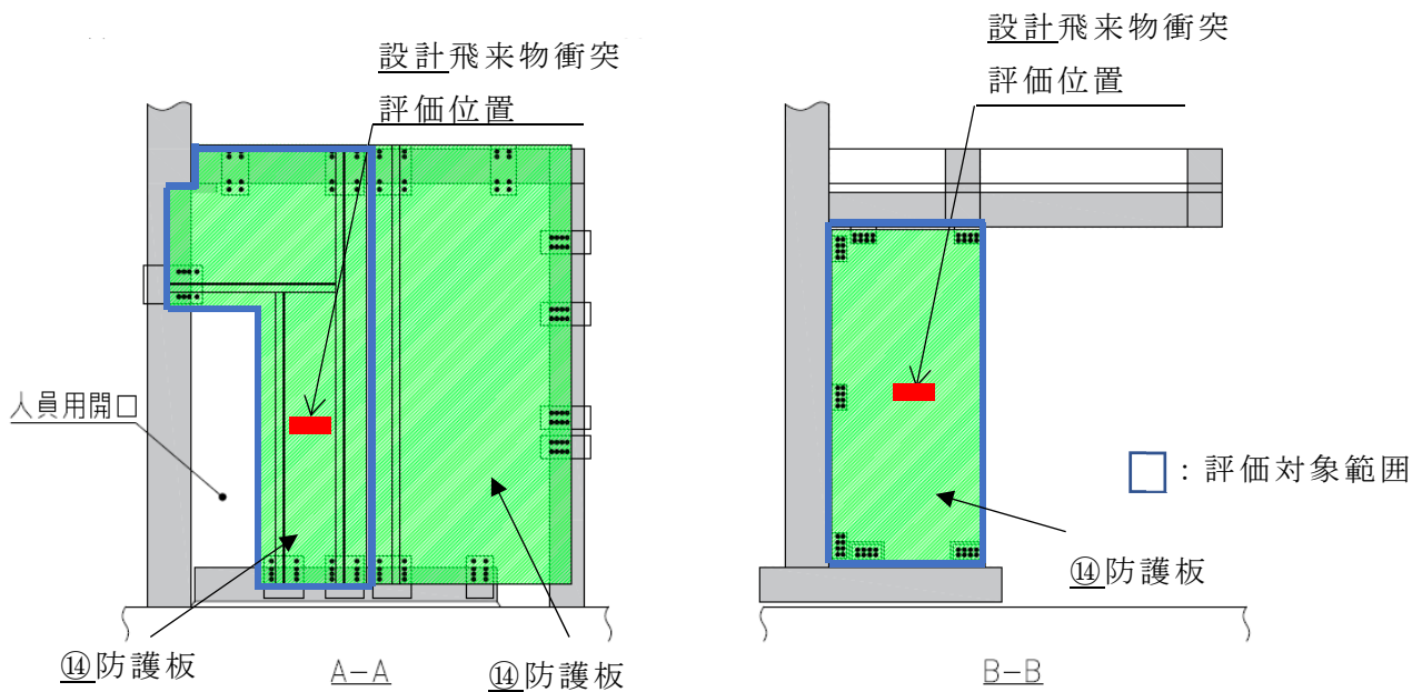
第 2 -32図 相対する 2 辺以上で支持する防護板 設計飛来物衝突評価(水平)位置
