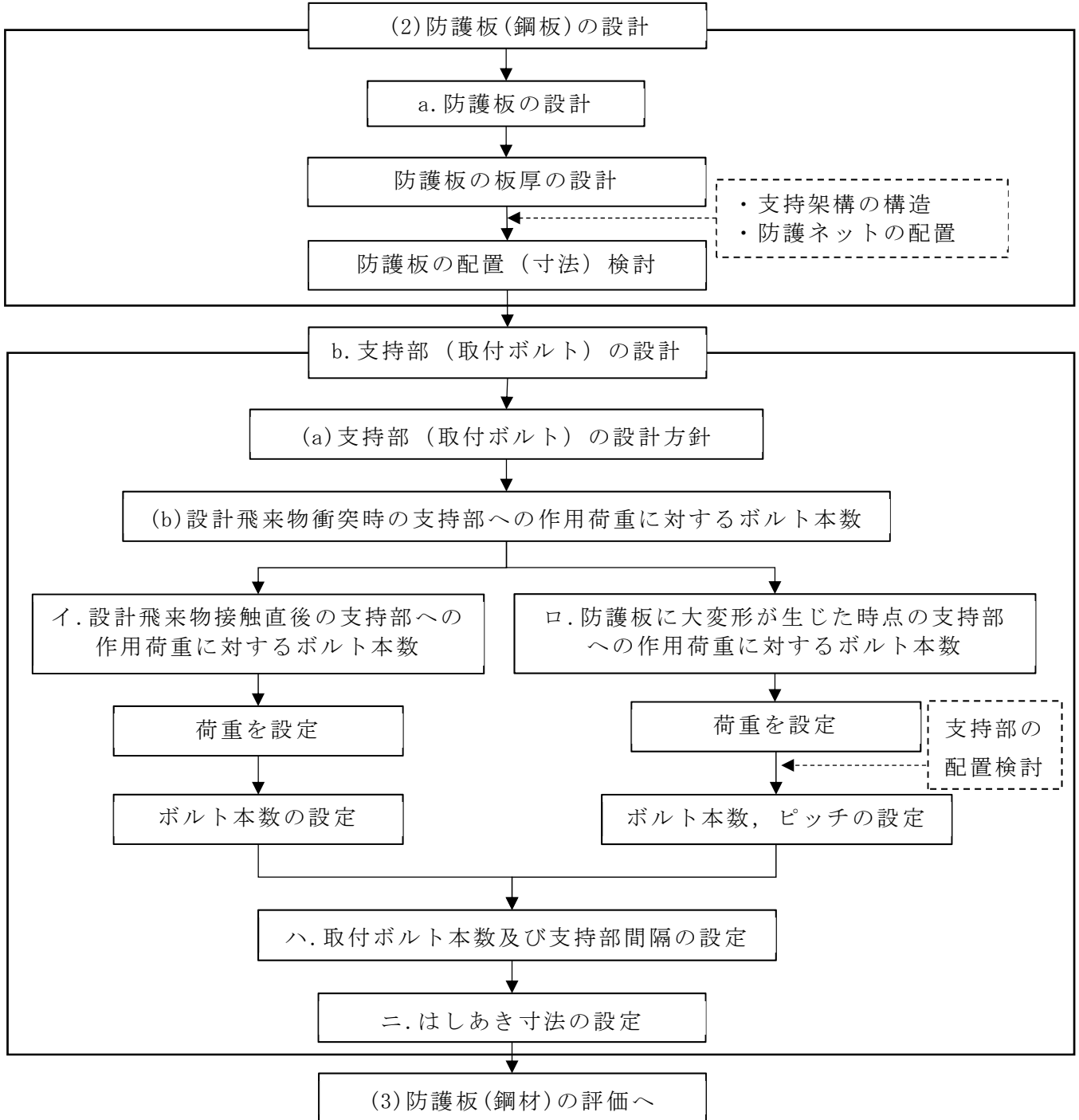
第2-20図 防護板(鋼材)の設計フロー
