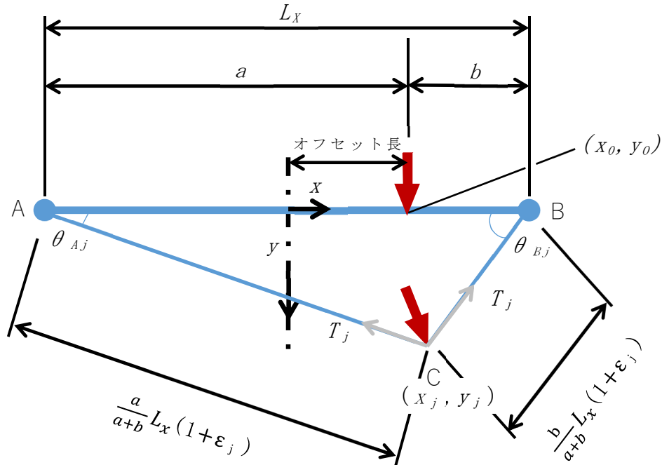
第2-3図 展開方向オフセット衝突の交点列1列の変形状態の模式図
