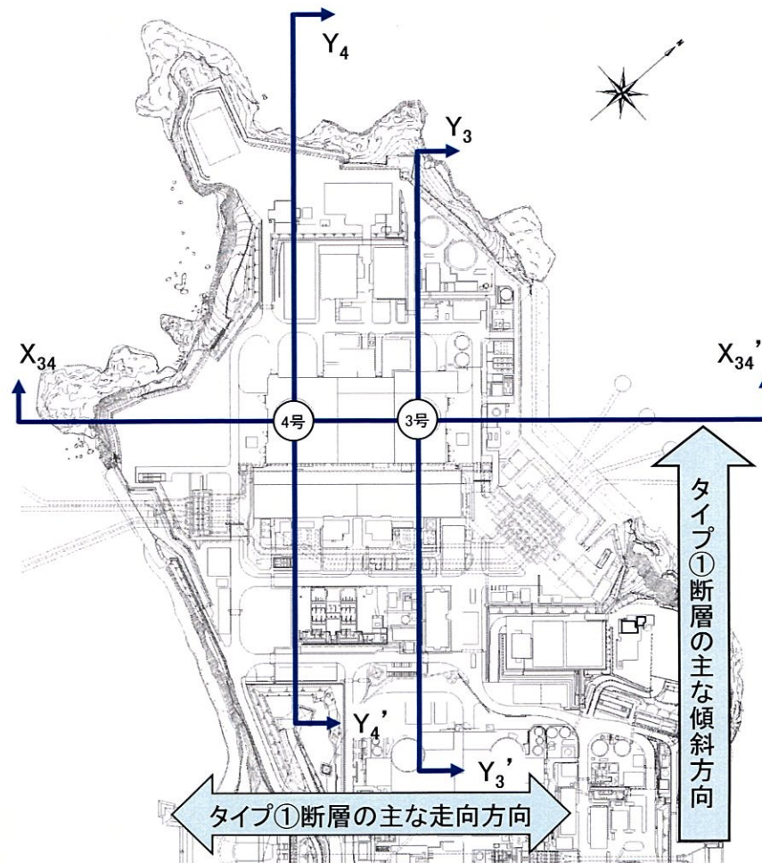
評価対象断面位置図
