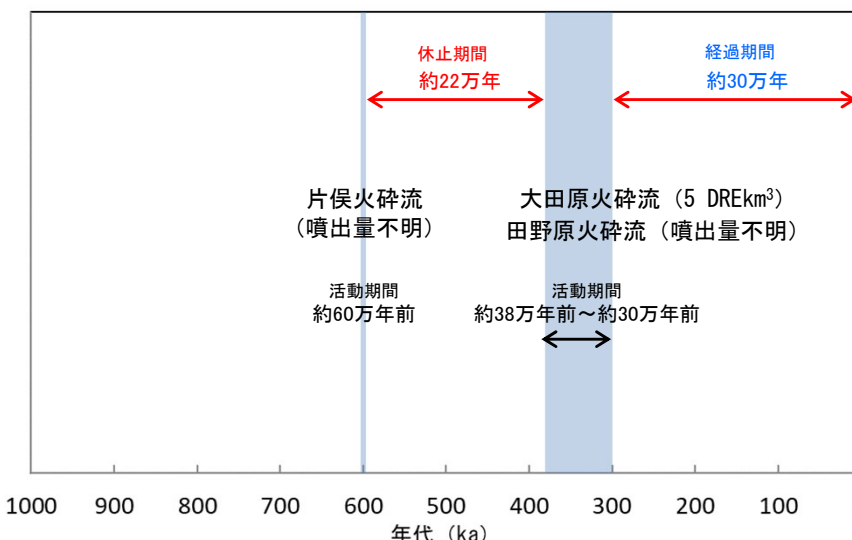
塩原カルデラの階段ダイヤグラム
