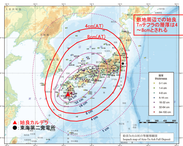
始良Tnテフラの分布(宝田他(2022)に加筆)
