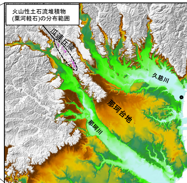
栗河軽石の分布は, 坂本・宇野沢(1976)に基づき作成
