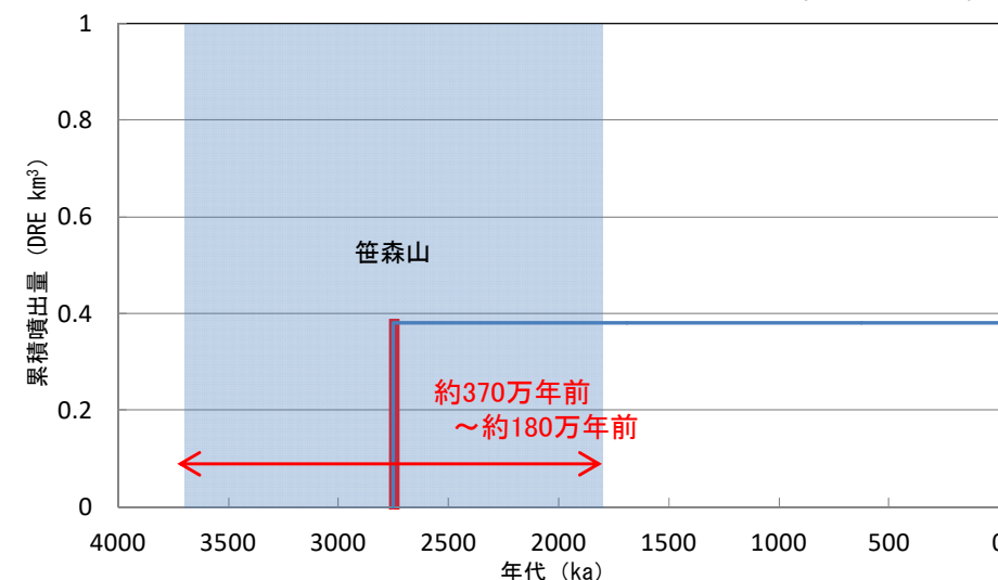
笹森山の階段ダイヤグラム
