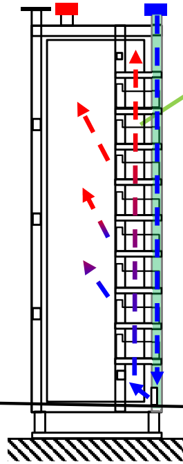
側面図
