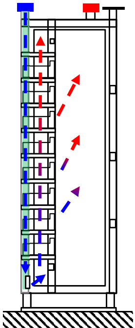
側面図
