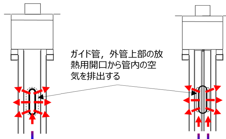
PWR燃料用ガイド管
