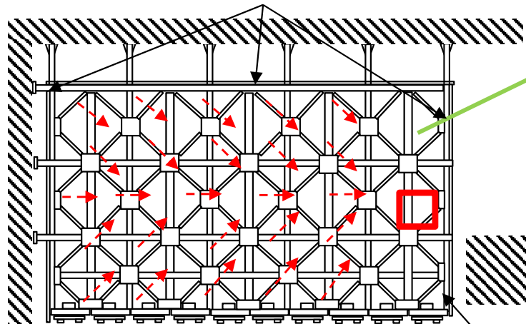
燃料棒貯蔵棚-1 上面図
