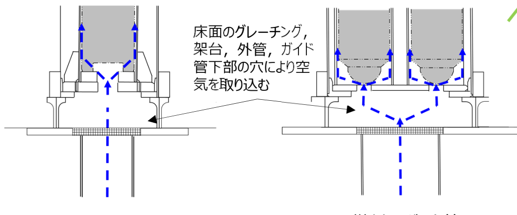
PWR燃料用ガイド管
