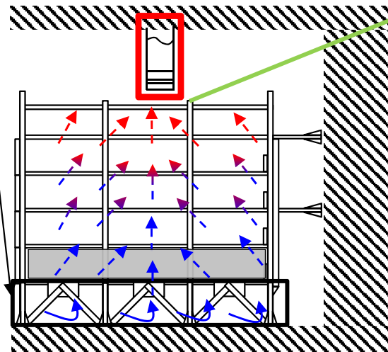
燃料棒貯蔵棚-1 断面図
