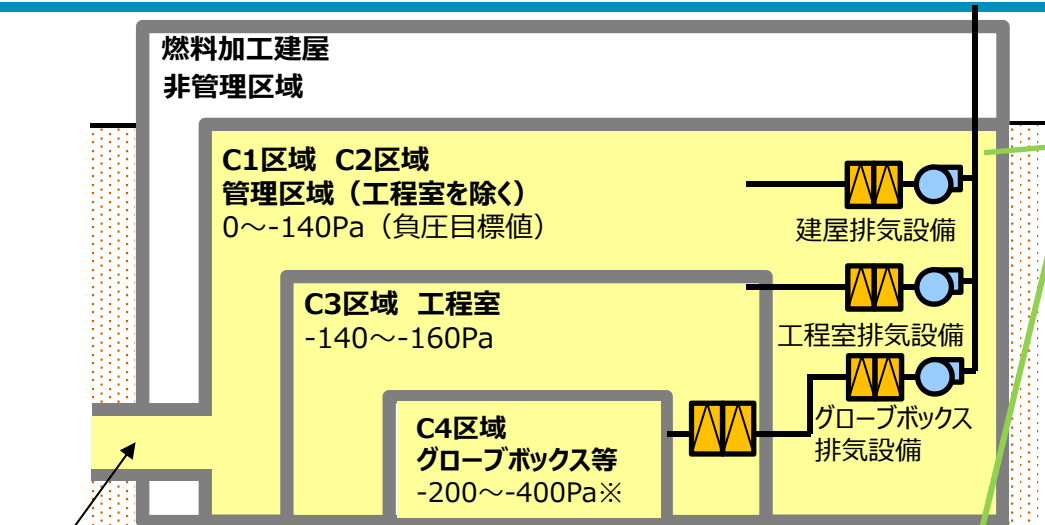
第3.12.1-2表 MOX燃料加工施設における負圧目標値 (1/2)
