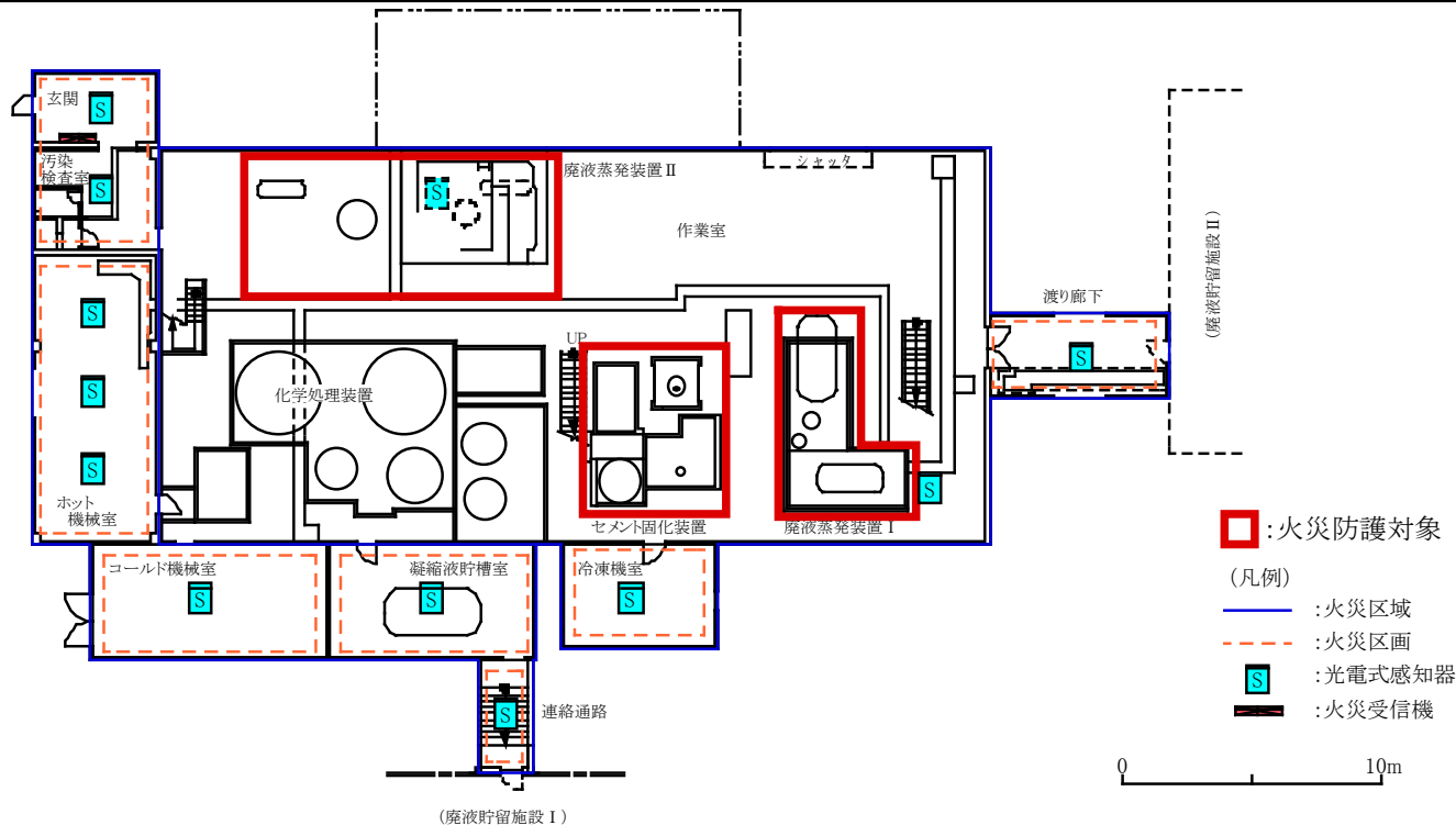
(例) 施設ごとの火災区域、火災区画(廃液処理棟)
