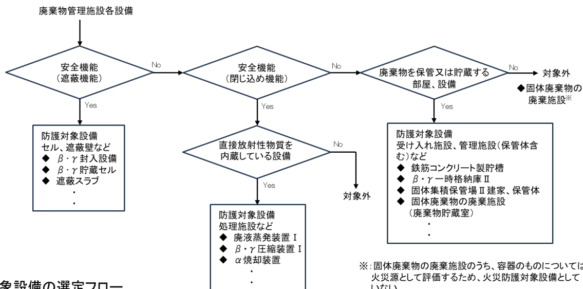
火災防護対象設備の選定フロー
