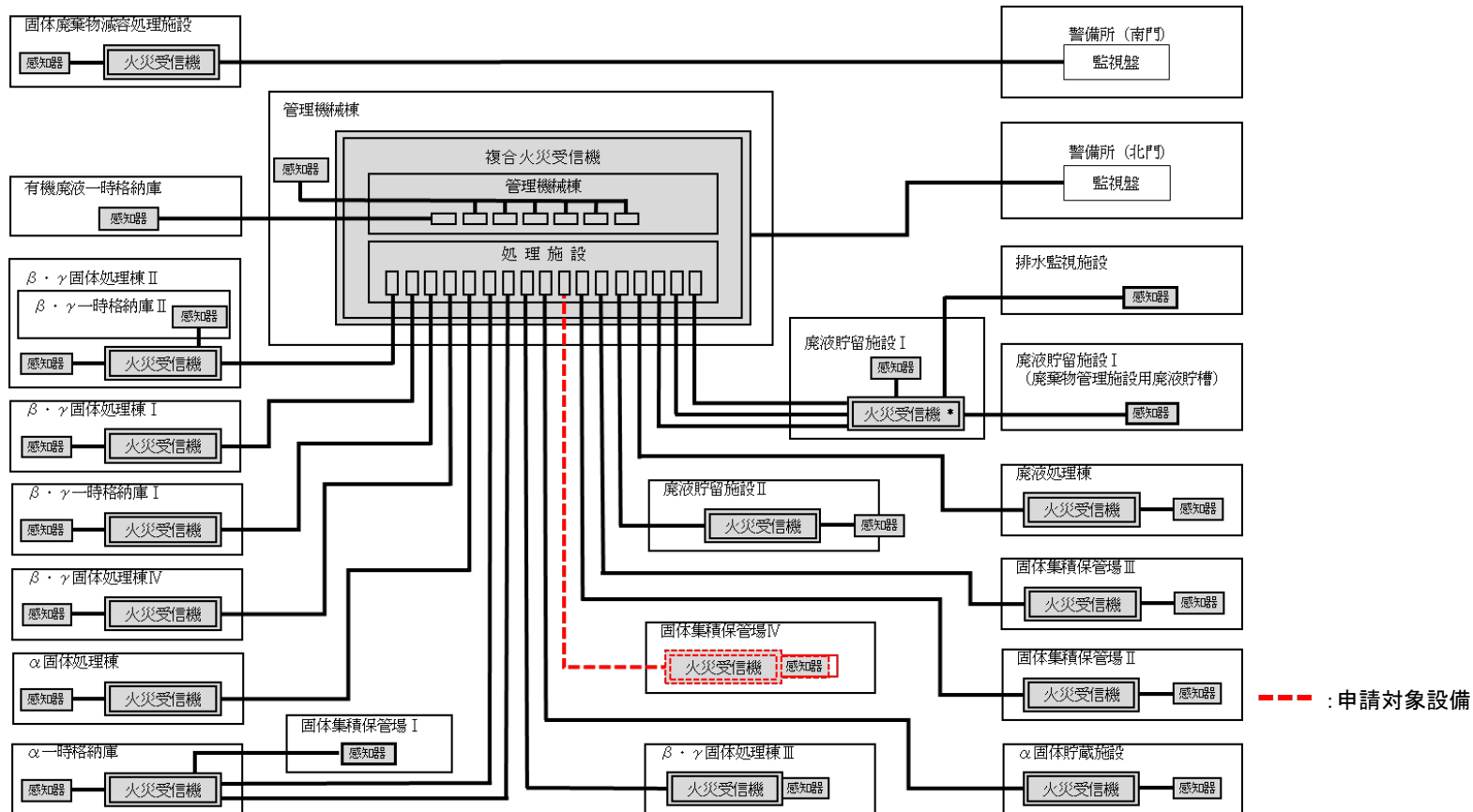
廃棄物管理施設の自動火災報知設備系統図
