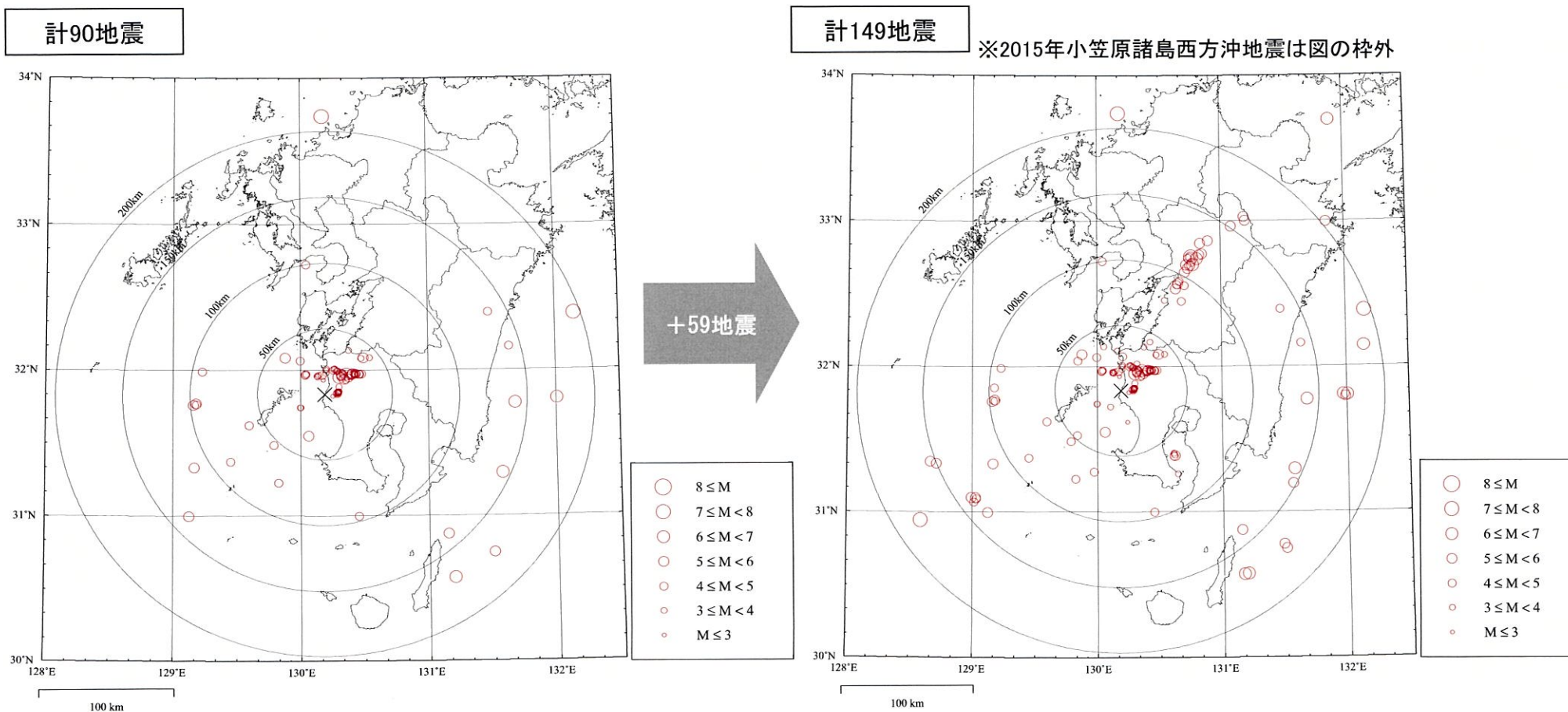
敷地地盤における観測地震の震央分布 (観測開始～2019年度)
