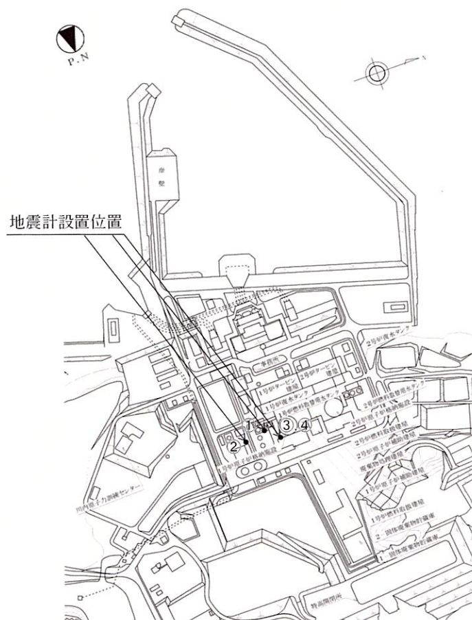
敷地の鉛直アレイ地震計平面配置図
