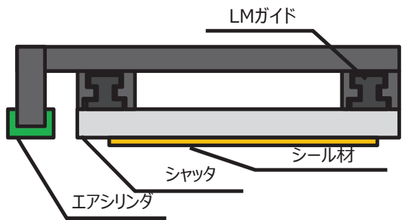
シャッタ上面図
