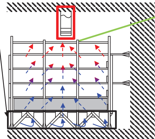
燃料棒貯蔵棚-1 断面図
