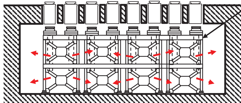
一時保管ピット 正面図
