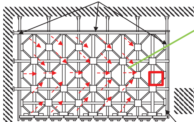
燃料棒貯蔵棚-1 上面図
