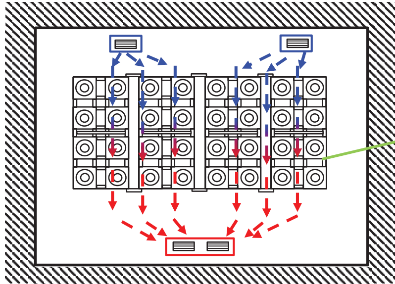
一時保管ピット 上面図
