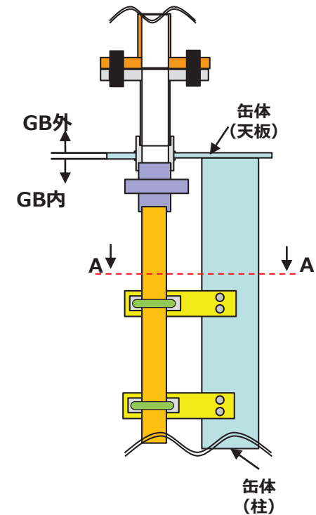
消火配管管台詳細
