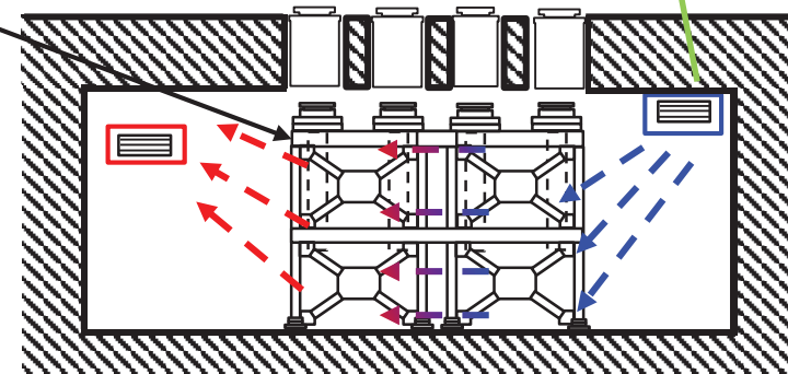
一時保管ピット 側面図
