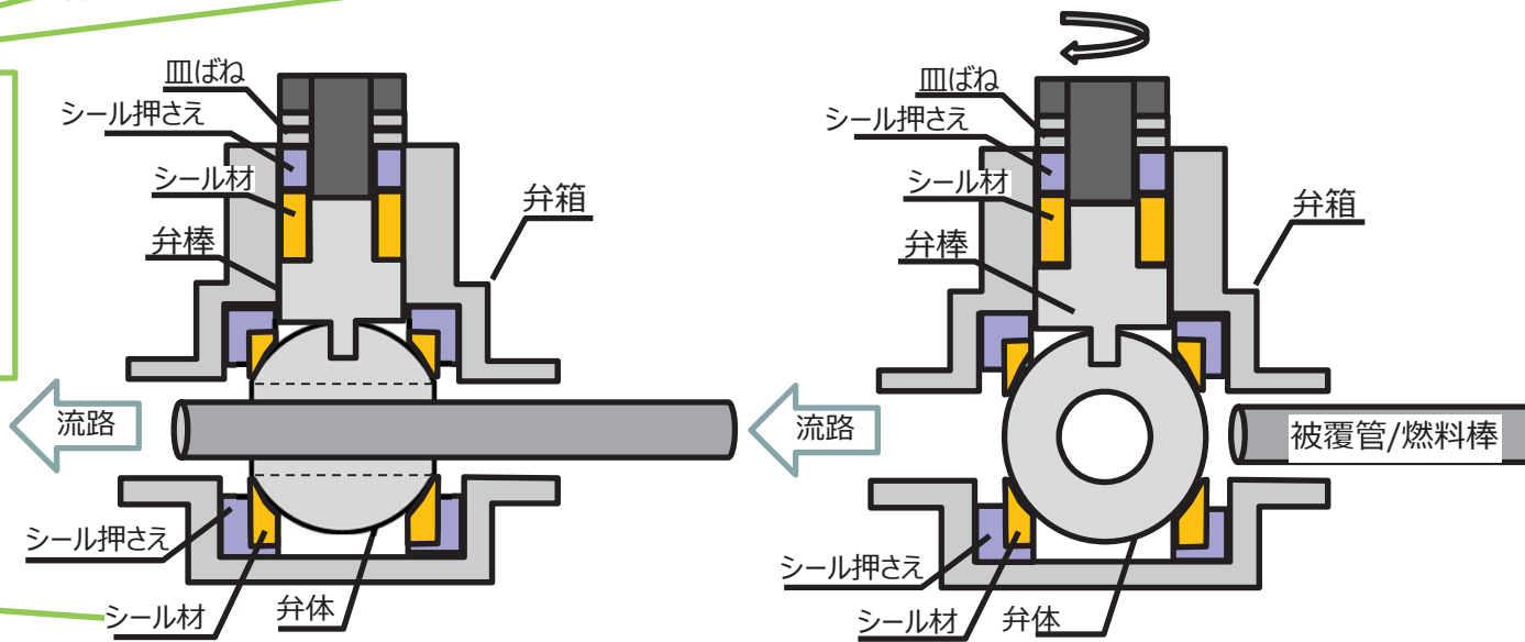
断面図 弁開放時
