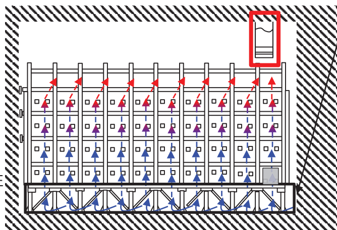
燃料棒貯蔵棚-1 正面図
