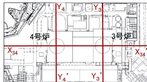
断面位置図
