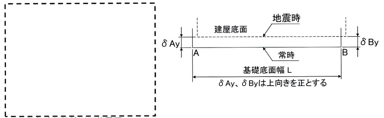
緊急時対策棟断面位置図
