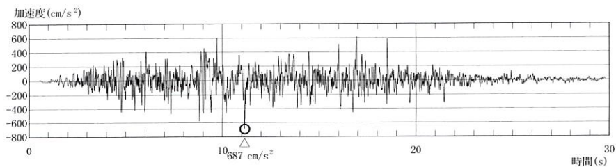
加速度(水平動)
