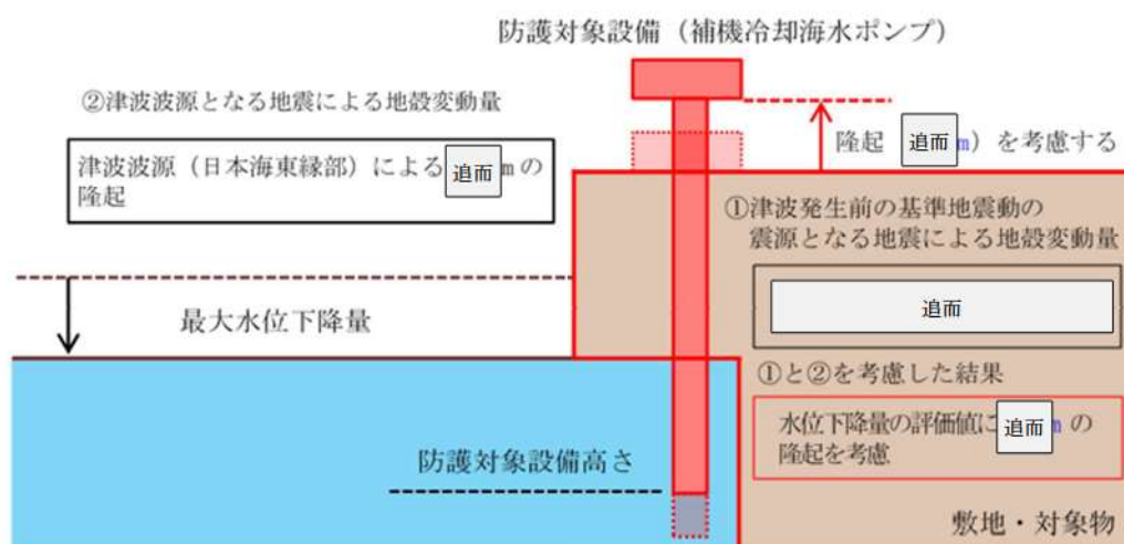
【水位下降側】
