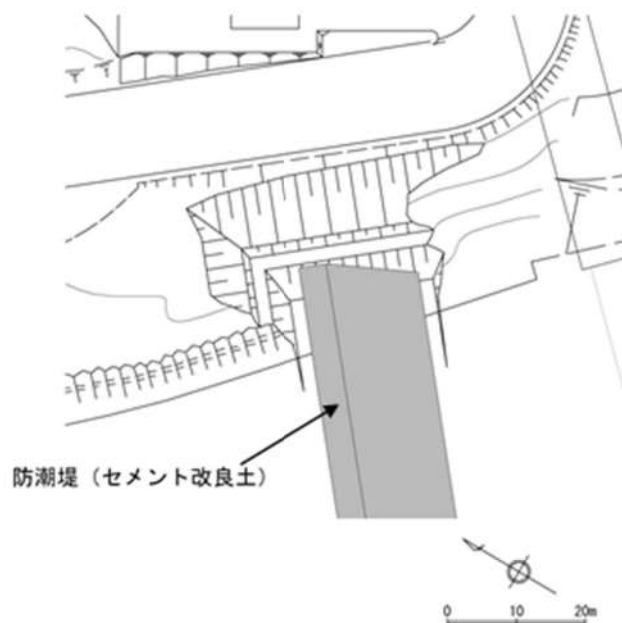
図 2.1. a. c-9 防潮堤（茶津側）端部の擦り付け構造
