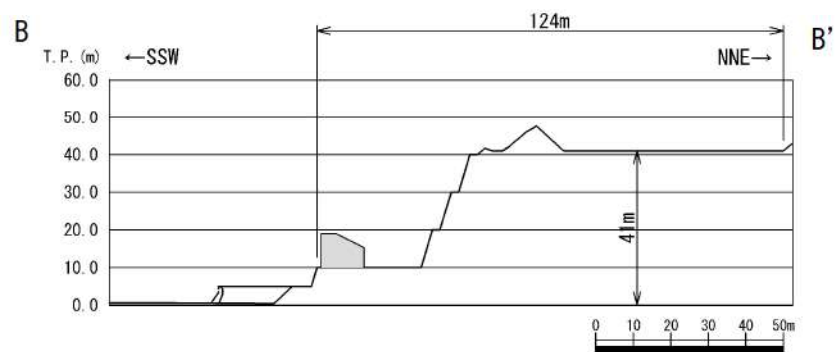
B-B' 断面
