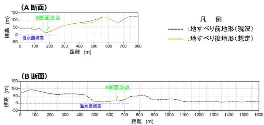
図 2. 1. b. b-4 地滑り地形③の断面図
