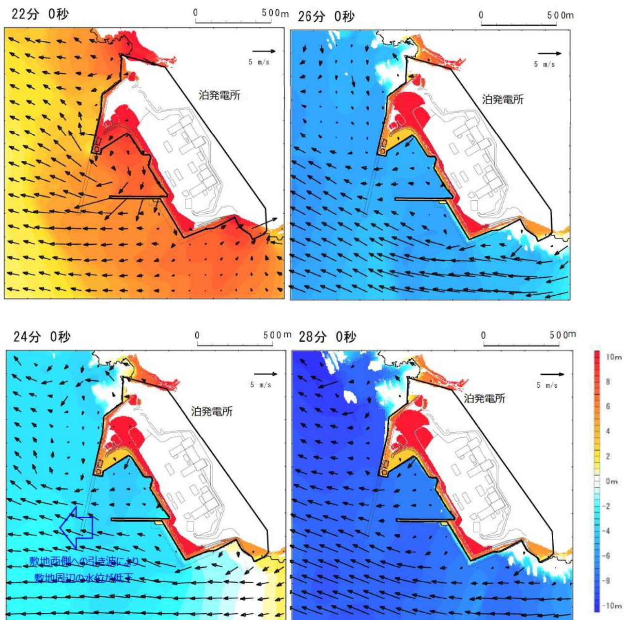
図1.2. a-1 (3) 水位変動量・流速分布の経時変化 (スナップショット) (基準津波 (波源F, 北防波堤損傷) ※ 1, 2 ) (拡大図その2)
