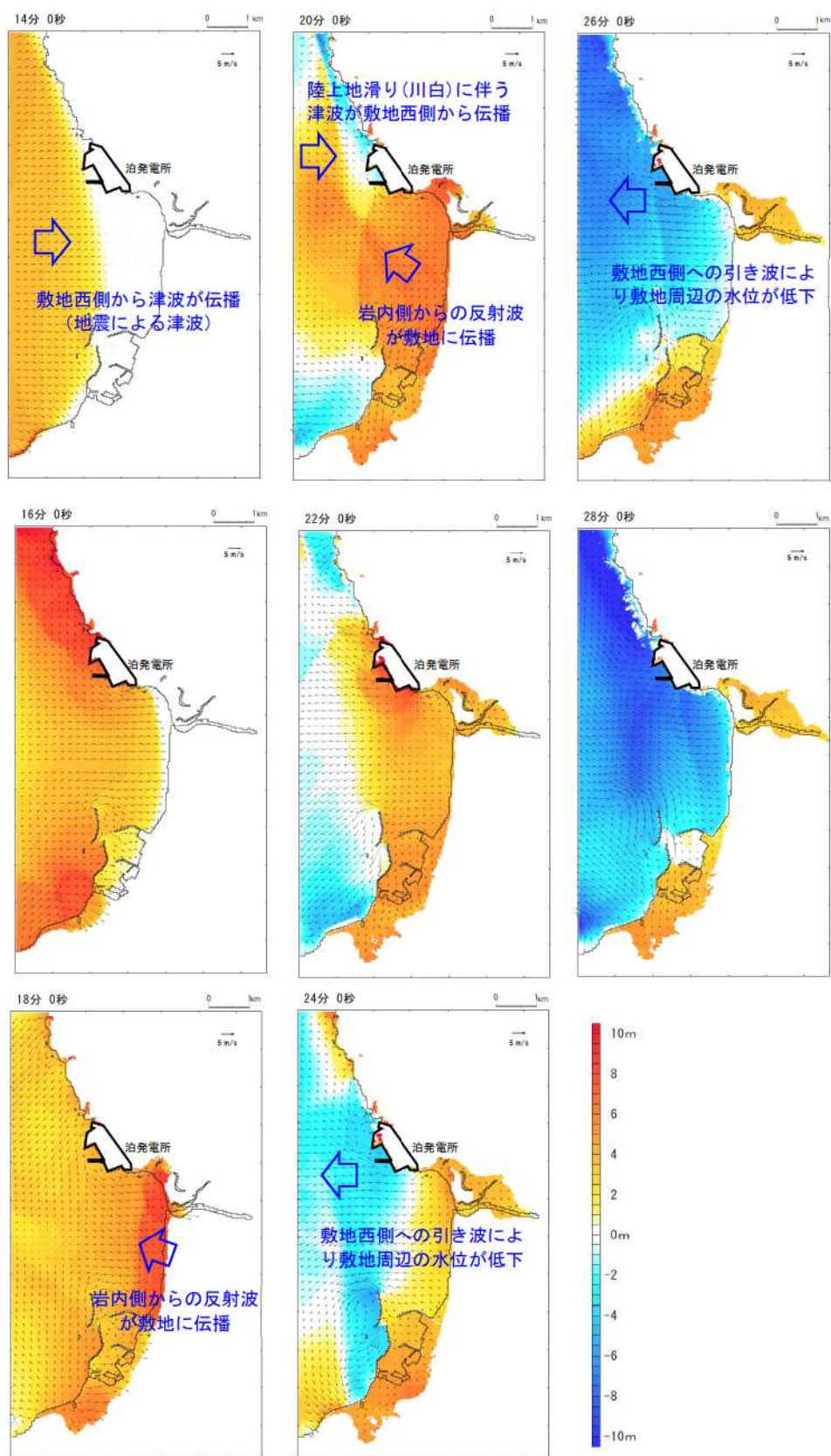
図 1.2. a-1 (1) 水位変動量・流速分布の経時変化 (スナップショット) (基準津波 (波源 F, 北防波堤損傷) ※) ※現時点における最大ケース
