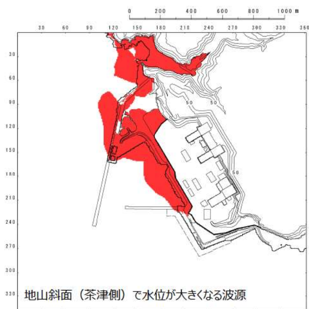
図 2.1. a. b-3 (1) 最大水位上昇量分布図 (基準津波：波源D，北及び南防波堤損傷) (■ T. P. 10. 0m 以上表示)
