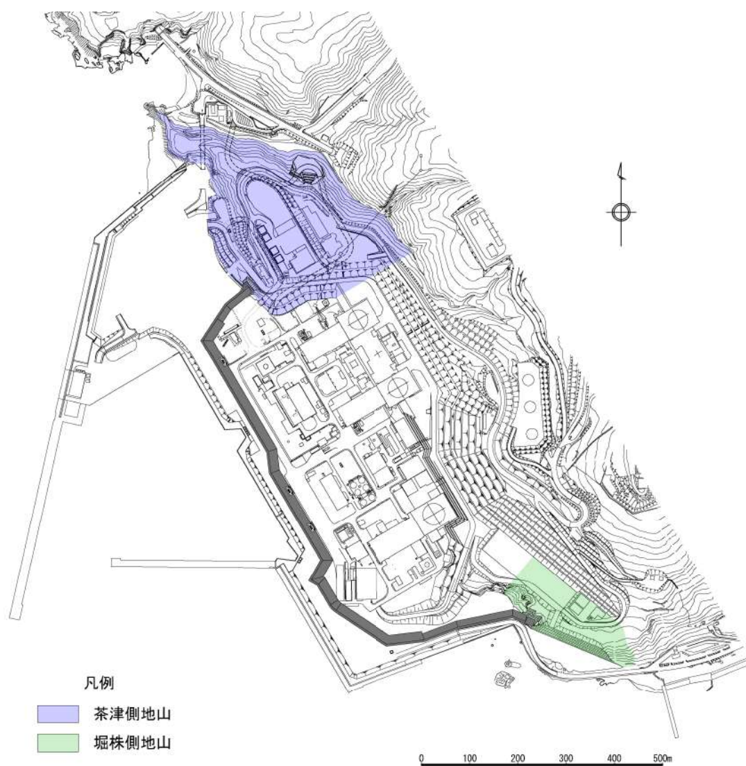
図 2.1. a. b-4 防潮堤（茶津側）及び防潮堤（堀株側）の地山
