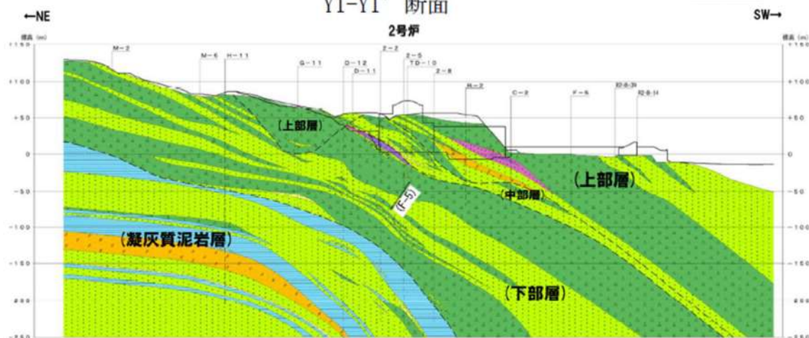
Y2-Y2' 断面
