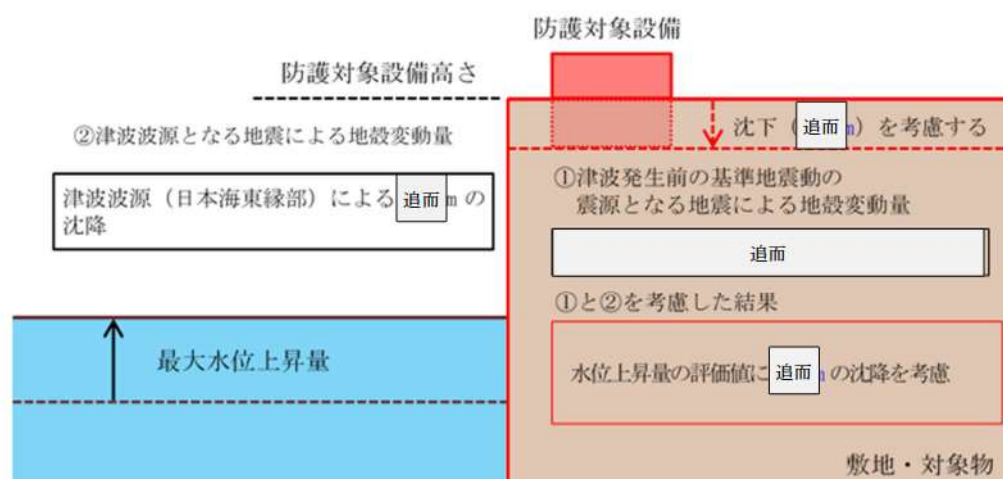
【水位上昇側】
