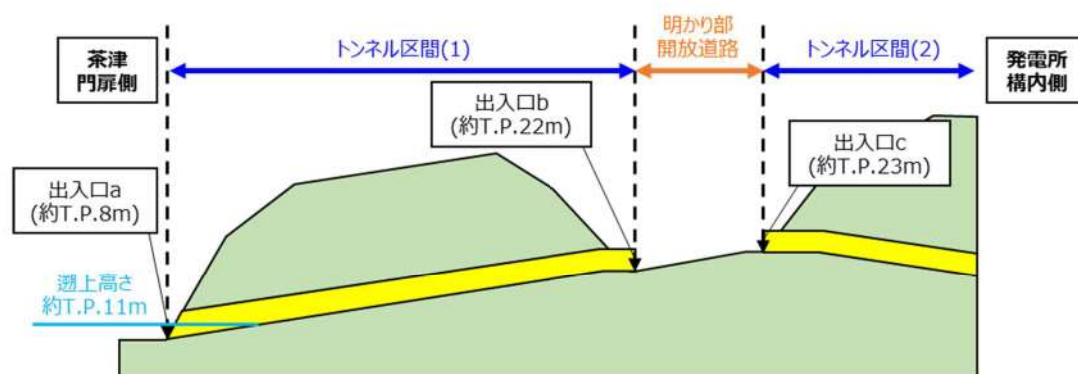
図 1.2. c-1 (3) 茶津入構トンネル断面図
