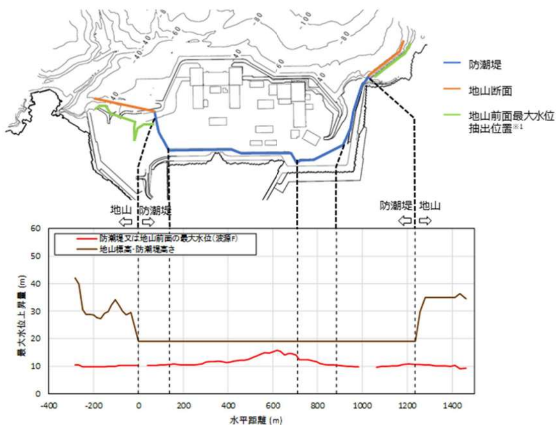
図 1. 2. b-2 防潮堤沿いの最大水位縦断図 ※2 (基準津波 (波源 F, 北防波堤損傷) ※3 )
