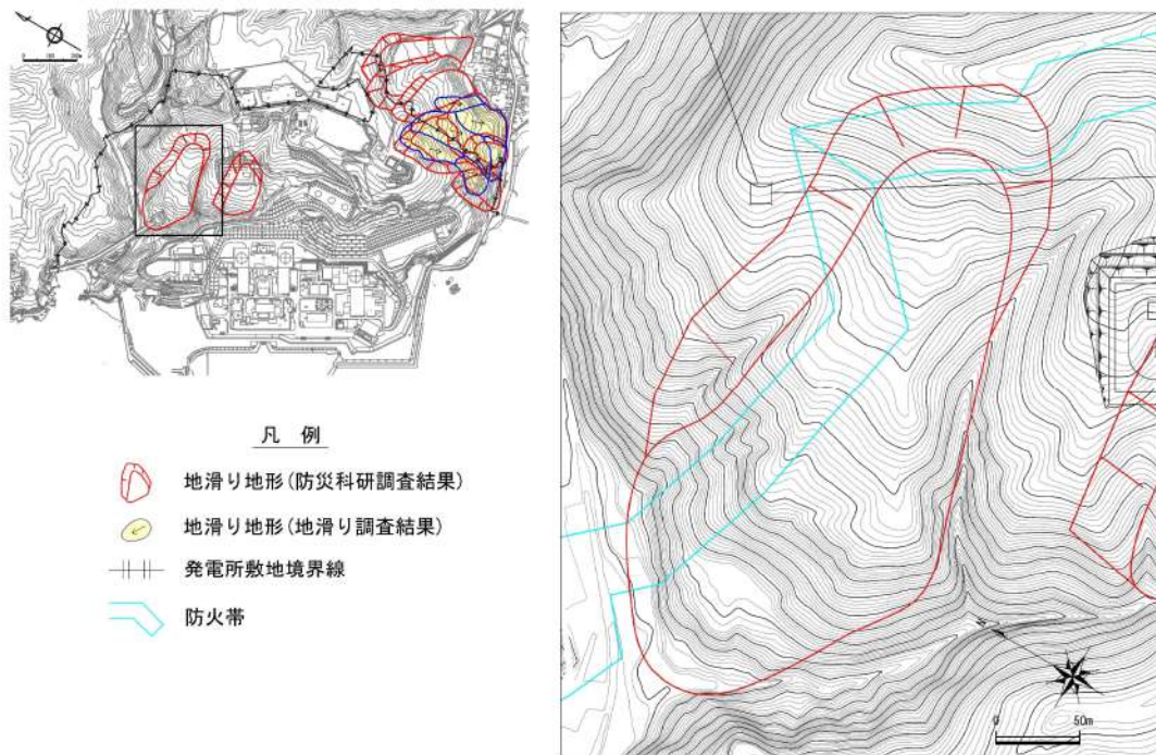
図 2.1.b.a-5 地滑り地形③分布図
