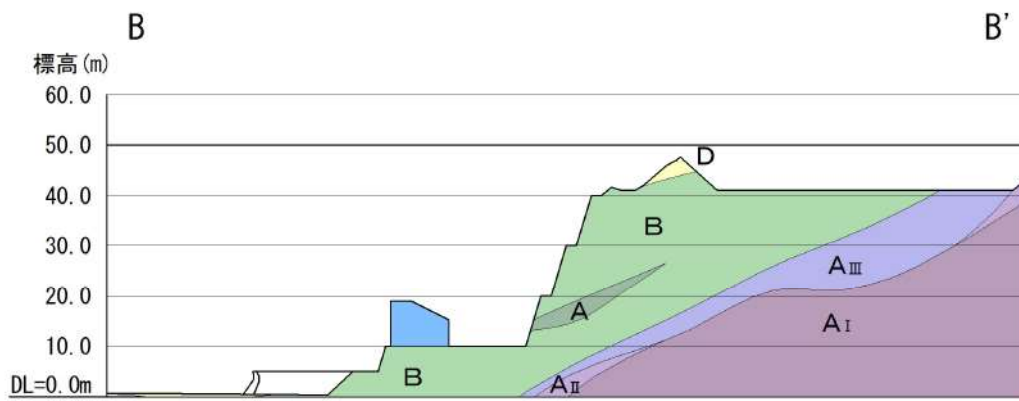
岩盤分類図 (B-B' 断面)
