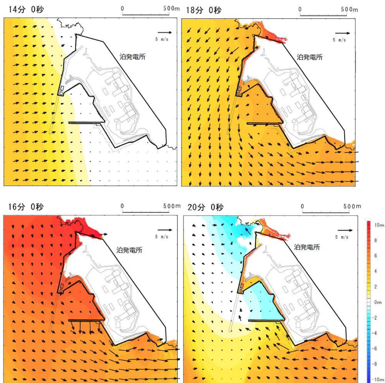
図1.2. a-1 (2) 水位変動量・流速分布の経時変化 (スナップショット) (基準津波 (波源F, 北防波堤損傷) ※) (拡大図その1) ※現時点における最大ケース
