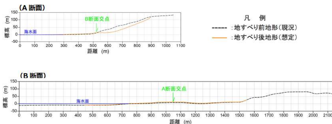
図 2. 1. b. b-2 地滑り地形①の断面図
