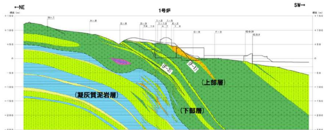
Y1-Y1' 断面
