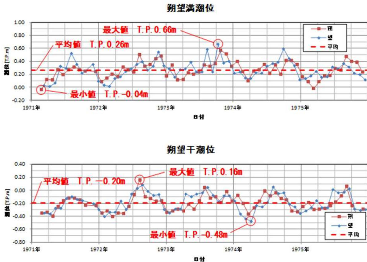
第 1.5-3 図 各月の朔望満干潮位 (1971 年 3 月～1975 年 12 月)
