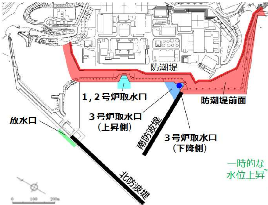
基準津波の抽出位置
