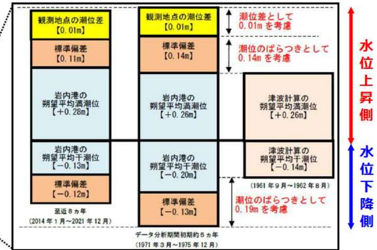
潮位変動の概念図
