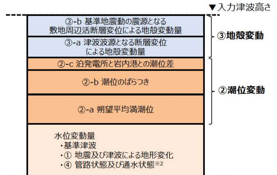
入力津波設定(水位上昇側)の概念図
