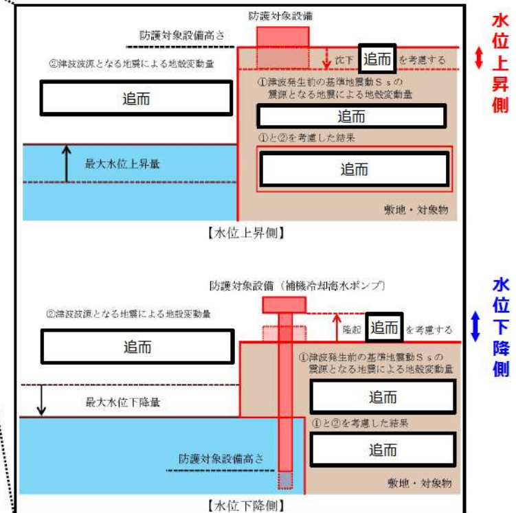
地殻変動の概念図
