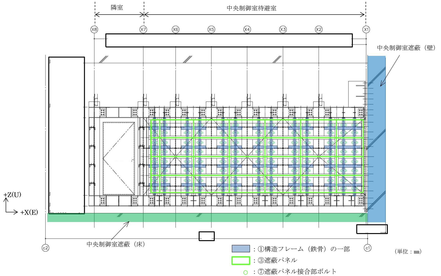
図 2-5 Y1 通り壁部における③遮蔽パネルの接合イメージ
