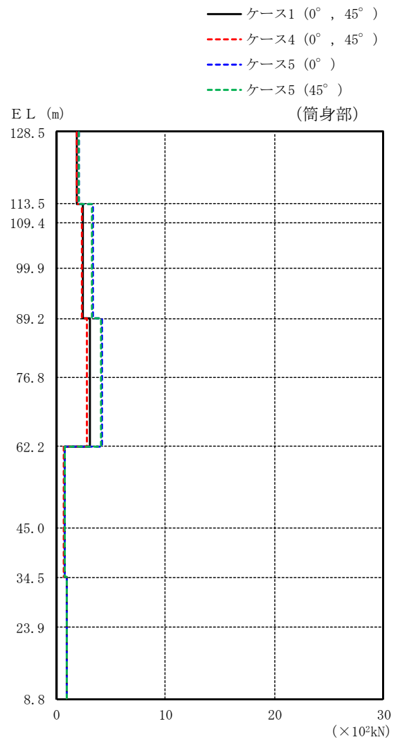
図 4-13(2) 最大応答せん断力 (基準地震動 S_s - D , 水平方向)
