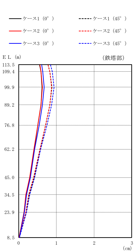
図 2-56(1) 最大応答変位 (弾性設計用地震動 S d - N 1, 鉛直方向)
