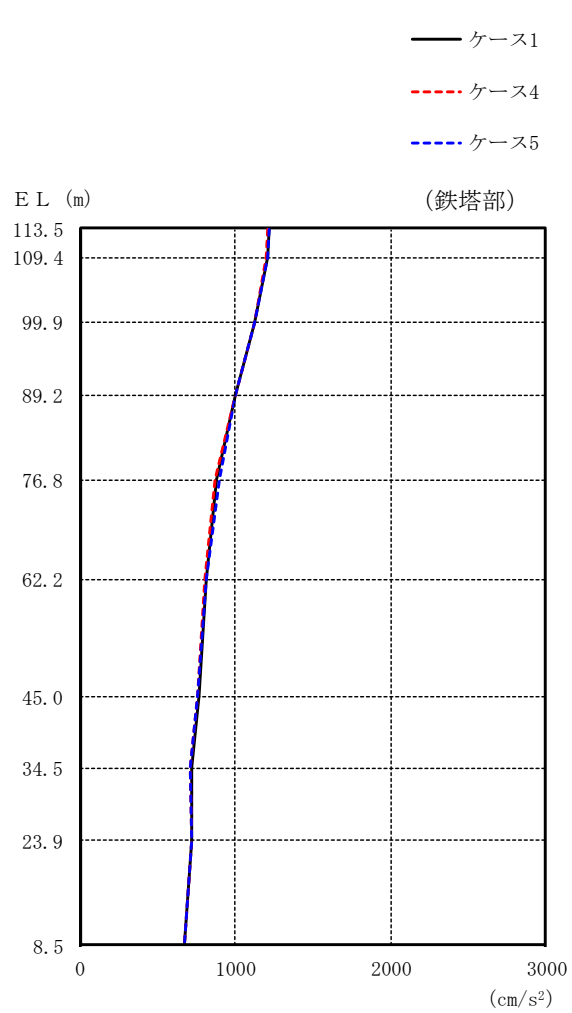
図 2-83(1) 最大応答加速度 (基準地震動 S s - N 2, 鉛直方向)
