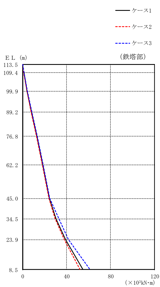
図 2-14(1) 最大応答曲げモーメント (基準地震動 S_s - F2 , NS 方向)
