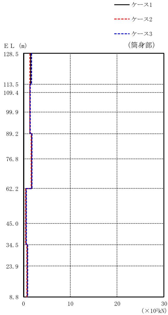
図 2-10(2) 最大応答せん断力 (基準地震動 S_s - F_2 , NS 方向)
