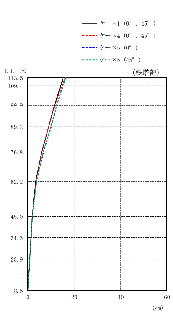
図 4-12(1) 最大応答変位 (基準地震動 S_s - D , 水平方向)
