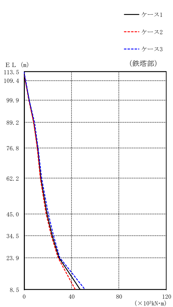
図 2-14(3) 最大応答曲げモーメント (基準地震動 S_s - F2 , EW方向)
