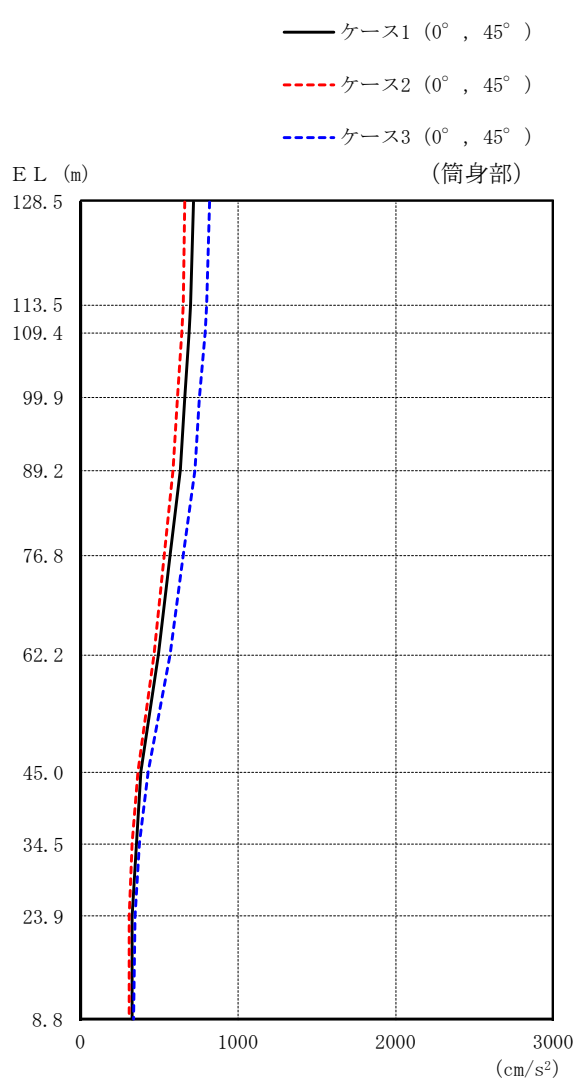
図 2-49(2) 最大応答加速度 (弾性設計用地震動 S d - D, 鉛直方向)
