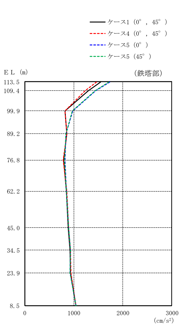
図 2-64(1) 最大応答加速度 (基準地震動 S s - D, 水平方向)
