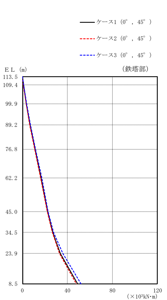
図 2-48(1) 最大応答曲げモーメント (弾性設計用地震動 S d - 1, 水平方向)
