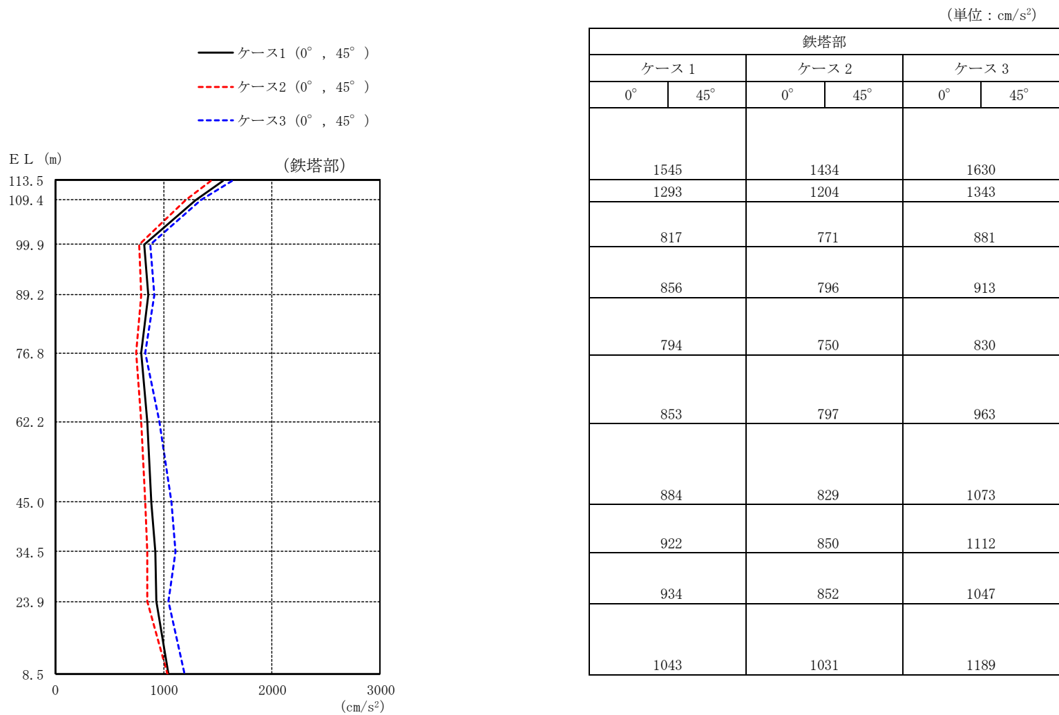
図 4-4(1) 最大応答加速度 (基準地震動 S_s - D , 水平方向)
