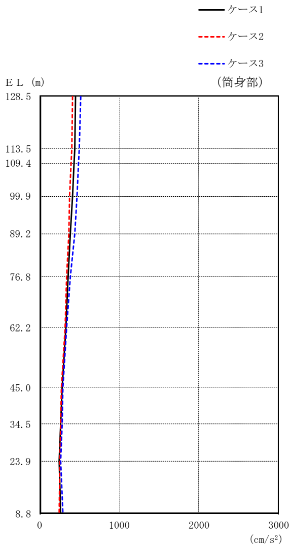
図 2-50(2) 最大応答加速度 (弾性設計用地震動 S d - F 2, 鉛直方向)
