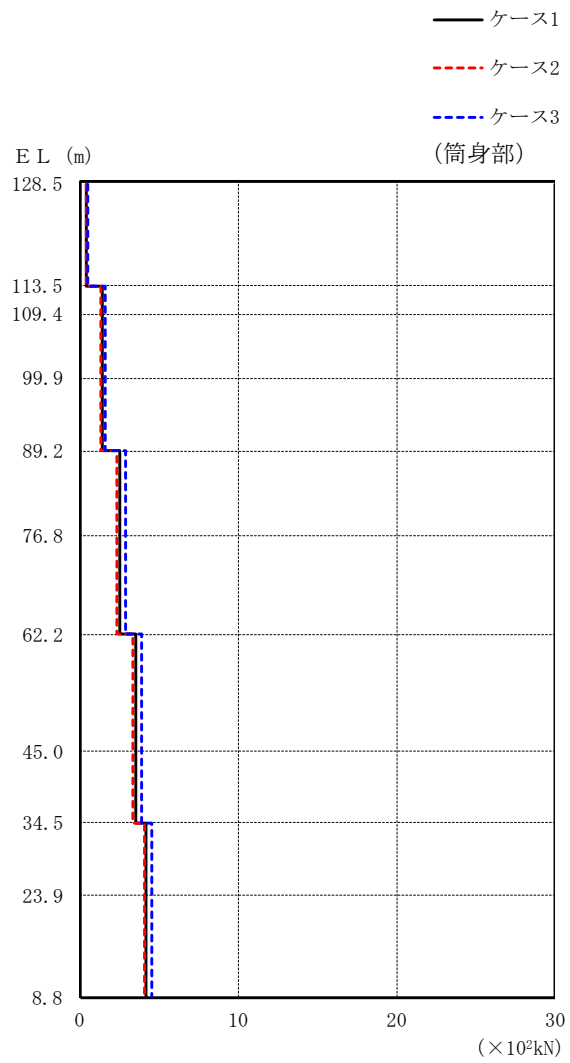
図 2-60(2) 最大応答軸力 (弾性設計用地震動 S d - F 2, 鉛直方向)
