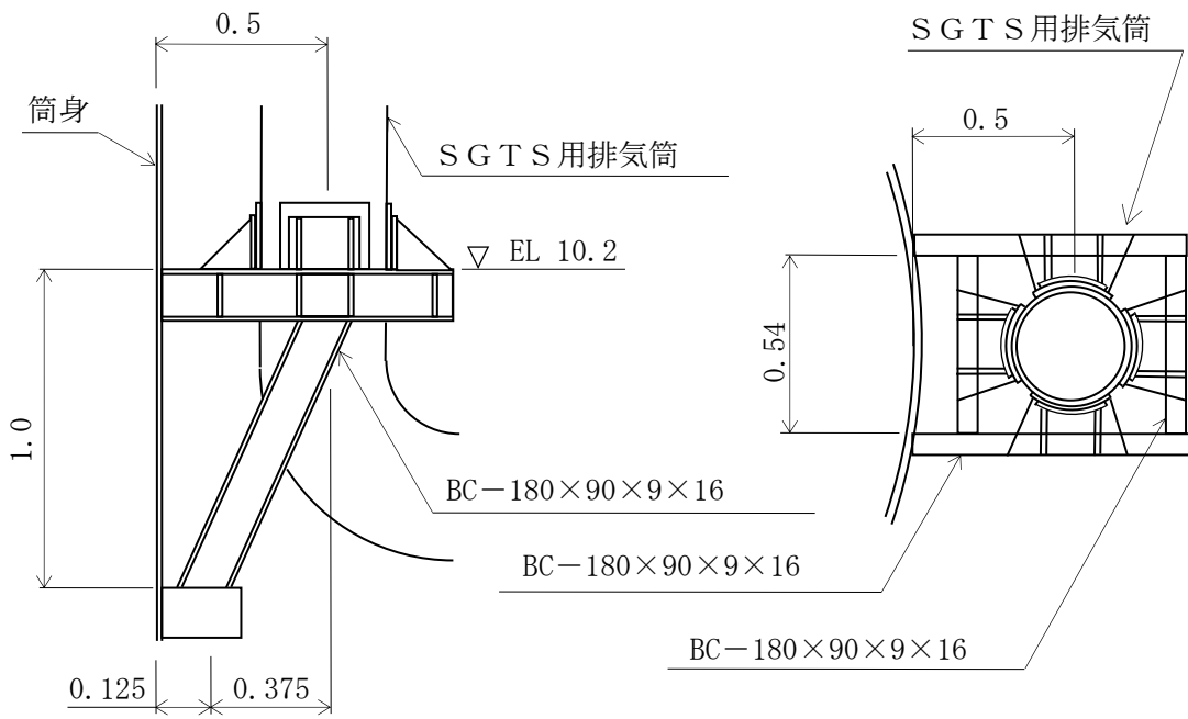
(b) 補強後 (今回工認)
