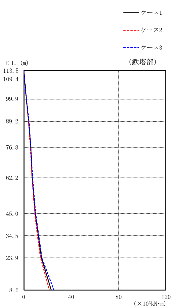
図 2-45(3) 最大応答曲げモーメント (弾性設計用地震動 S d - F 2, E W 方向)
