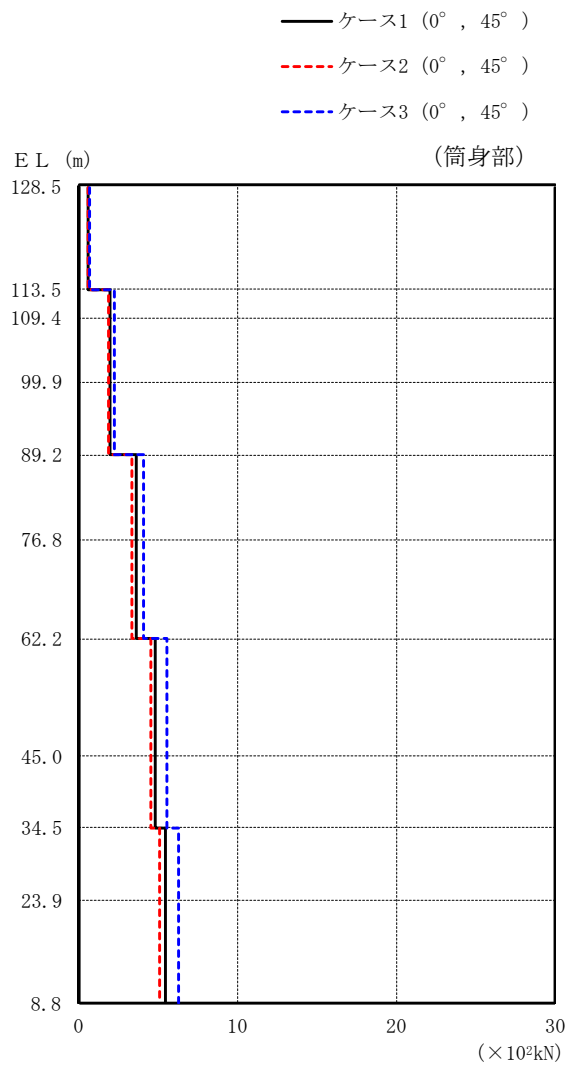
図 2-61(2) 最大応答軸力 (弾性設計用地震動 S d - N 1, 鉛直方向)
