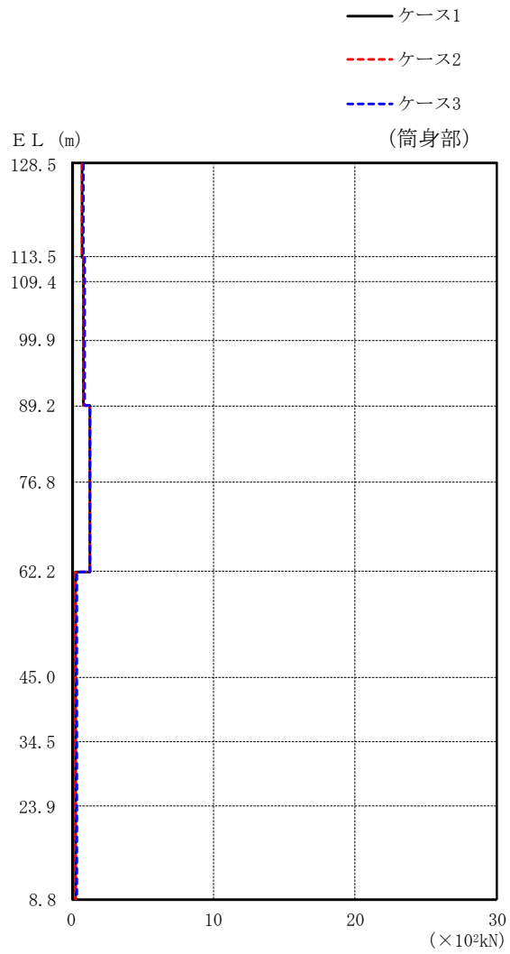
図 2-42 (2) 最大応答せん断力 (弾性設計用地震動 S d - N 2, NS 方向)
