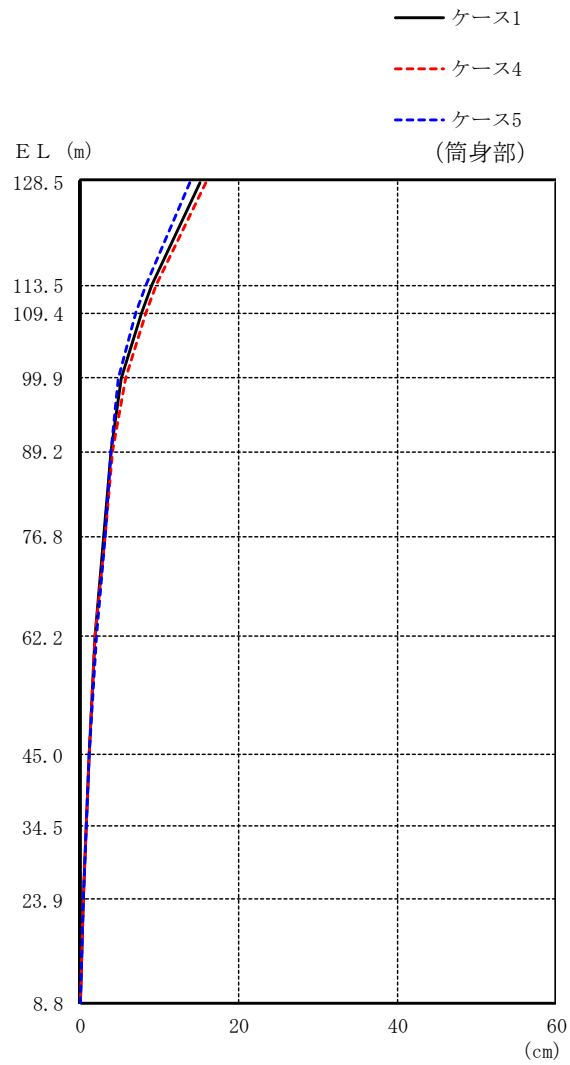
図 2-69(2) 最大応答変位 (基準地震動 S s - F 2, NS 方向)
