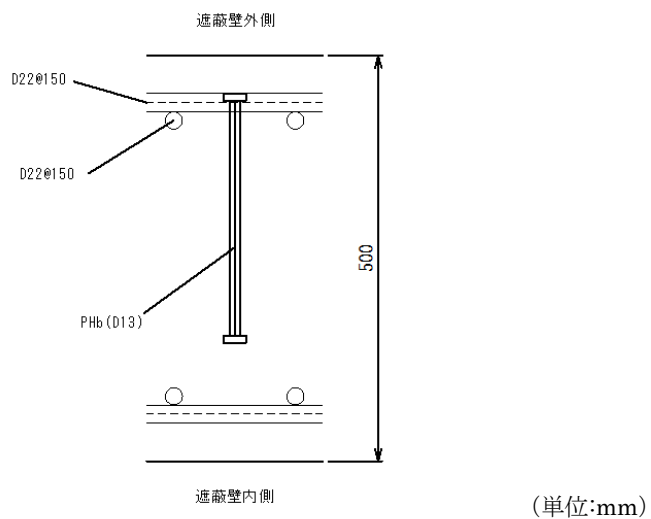
図 1.2-6(3) 復水貯蔵タンク遮蔽壁 概略配筋図 (PHb 工法)
