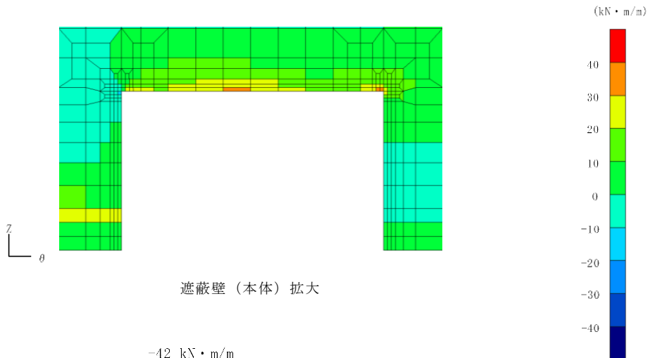
遮蔽壁（本体）
