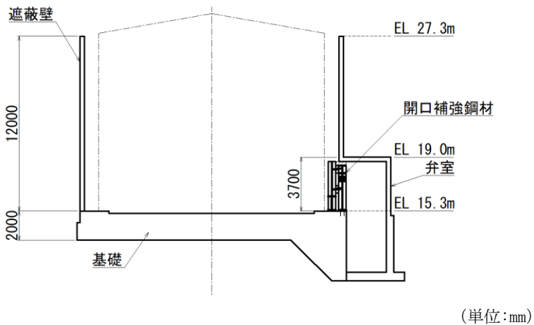
図 2.2-3 補助復水貯蔵タンク遮蔽壁 断面図 (A-A 断面, 東西)
