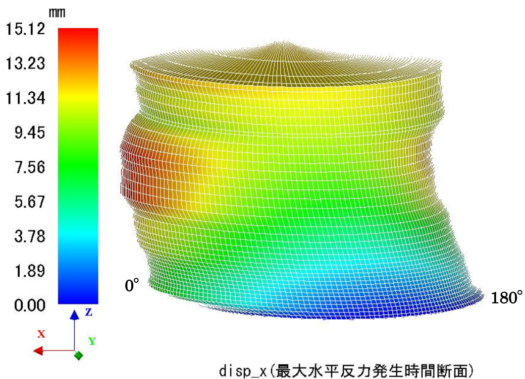
図 5-6 最大水平反力発生時水平 X 方向変位分布 (変形倍率 200 倍)
