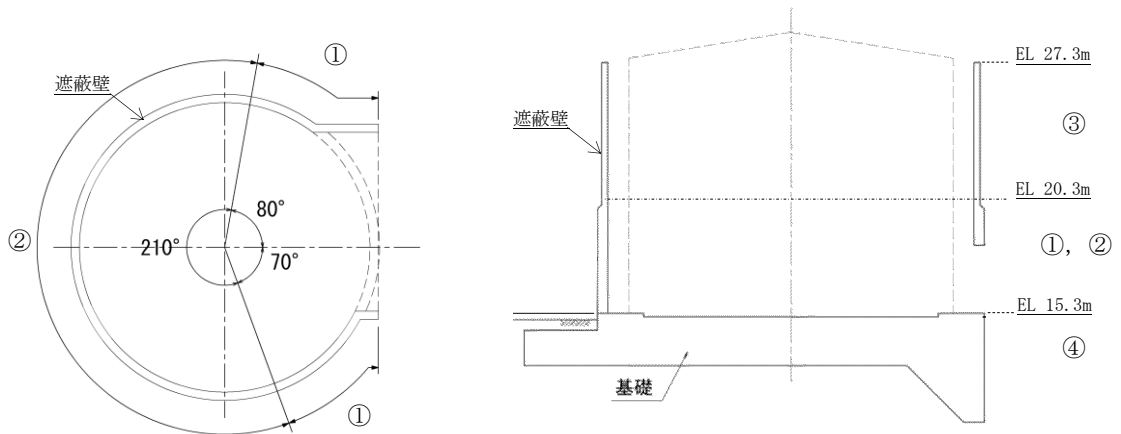
(遮蔽壁，基礎)
