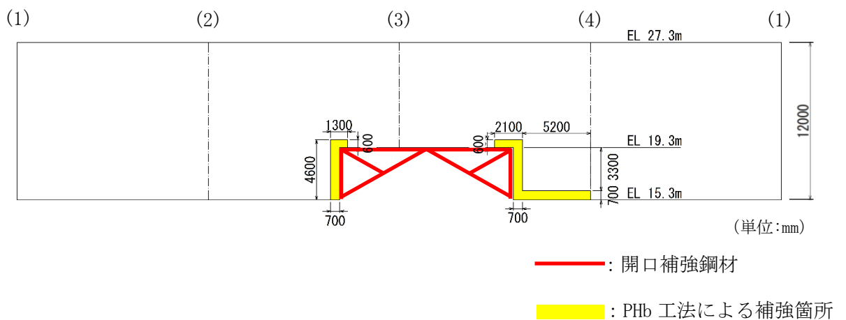
図 1.2-4 復水貯蔵タンク遮蔽壁 Phb 工法による耐震補強箇所及び開口補強鋼材概念図 (展開図)
