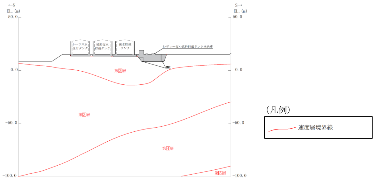
(速度層図)
