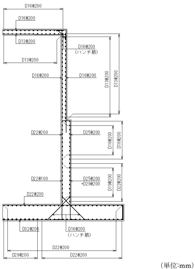
図 1.2-6(4) 復水貯蔵タンク遮蔽壁 概略配筋図 (弁室)
