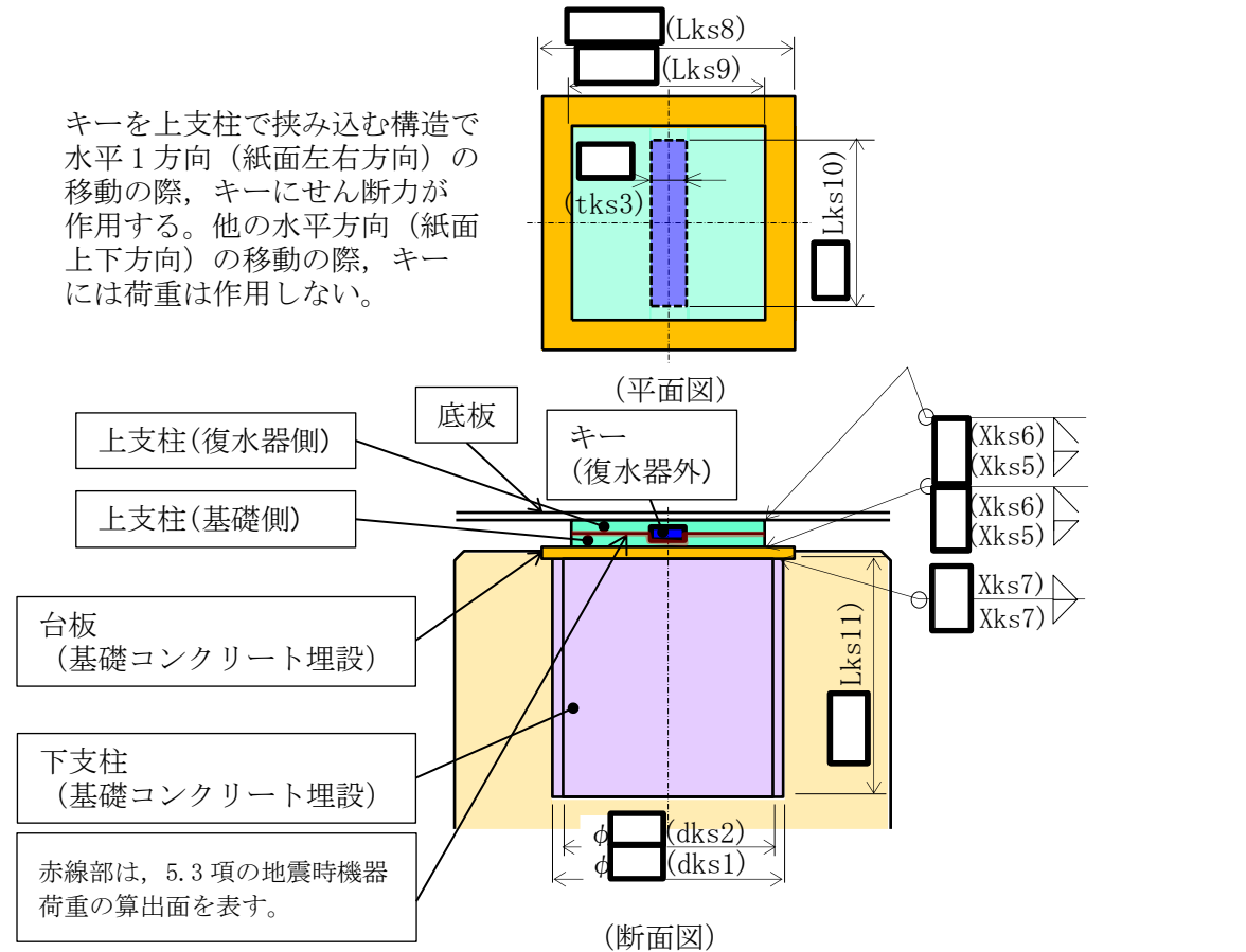
第 7.12-17 図 キーサポート⑩⑪平面図，断面図
