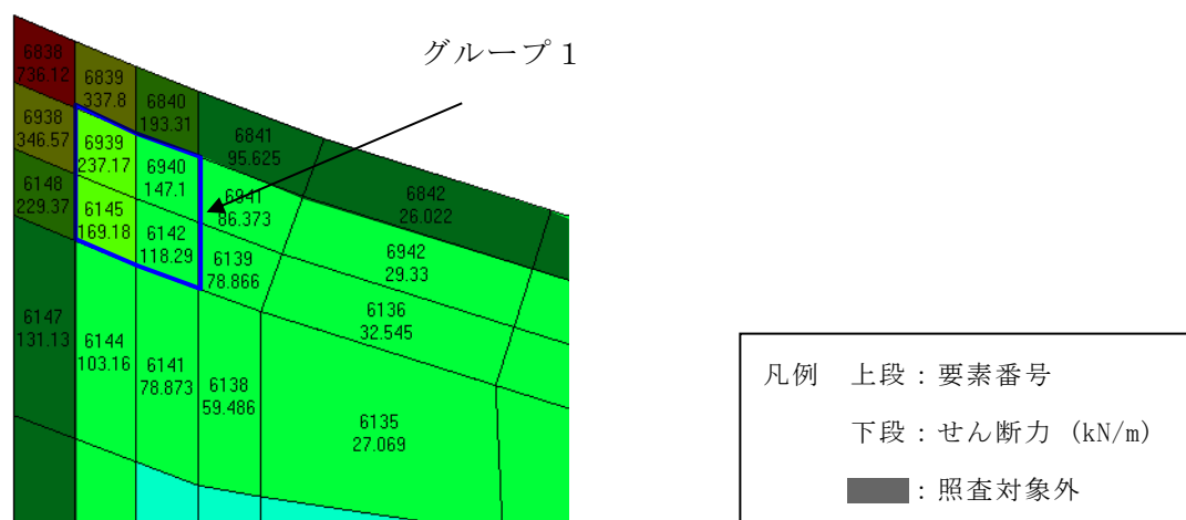
(b) せん断力分布拡大図（遮蔽壁（開口部頂版））
