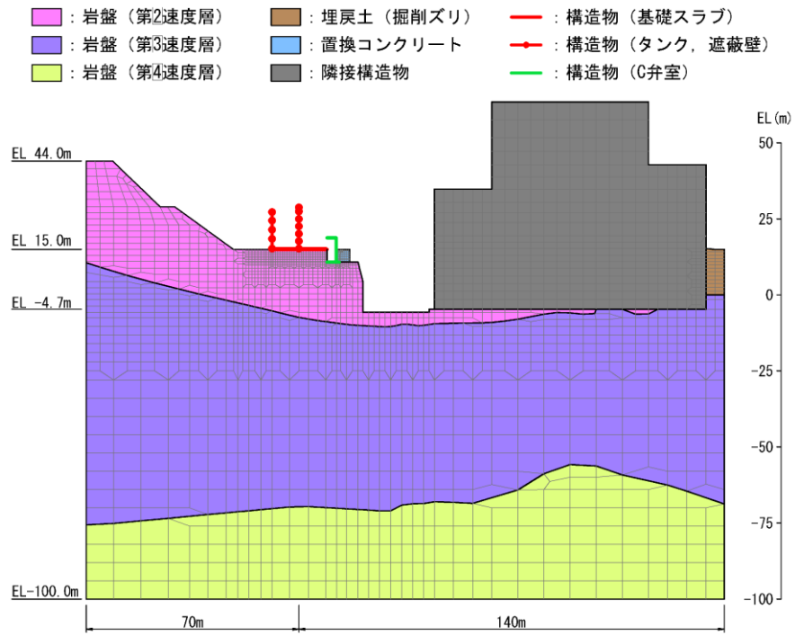
(全体図)
