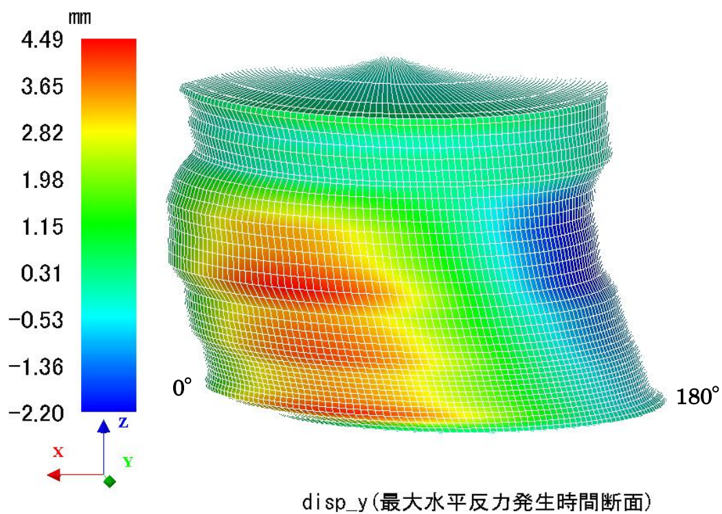
図 5-7 最大水平反力発生時水平 Y 方向変位分布 (変形倍率 200 倍)
