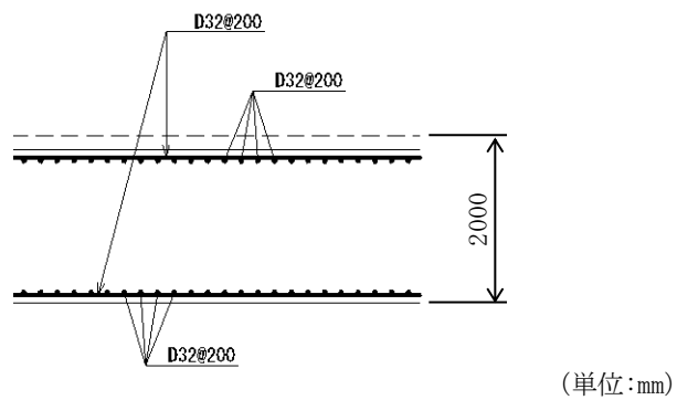
図 2.2-6(2) 補助復水貯蔵タンク遮蔽壁 概略配筋図 (基礎)
