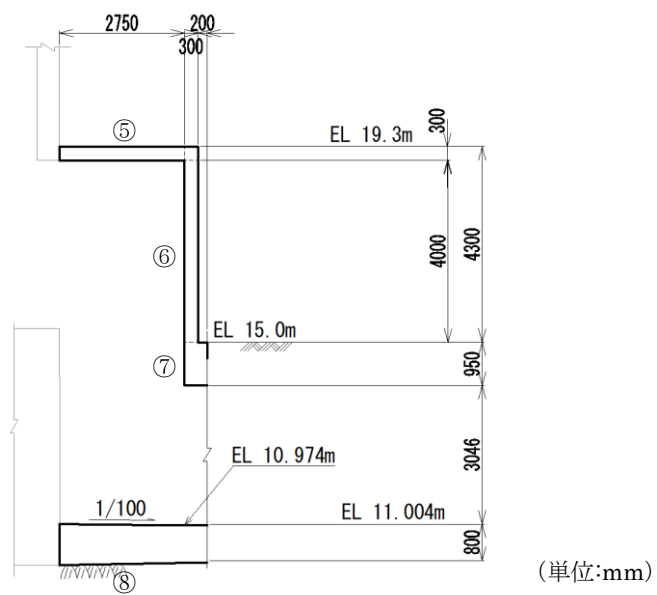
(弁室)
