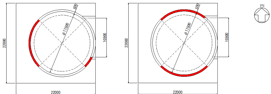
南北方向加振時の 有効せん断断面積
