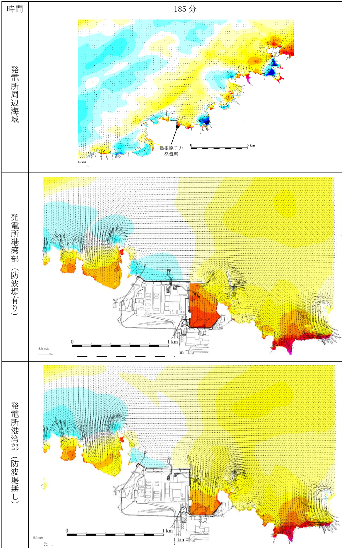
図 1-171 基準津波 1 の水位変動・流向ベクトル
