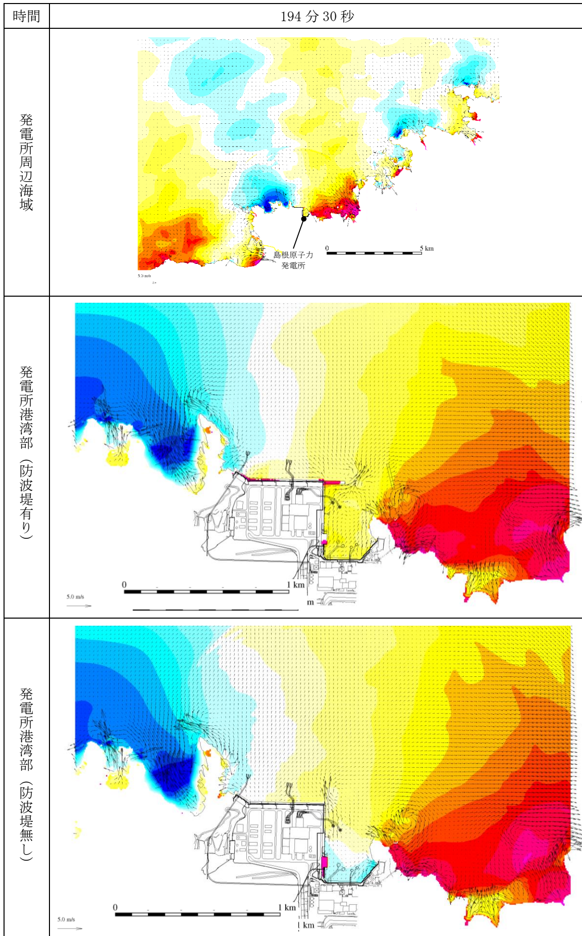
図 1-190 基準津波 1 の水位変動・流向ベクトル
