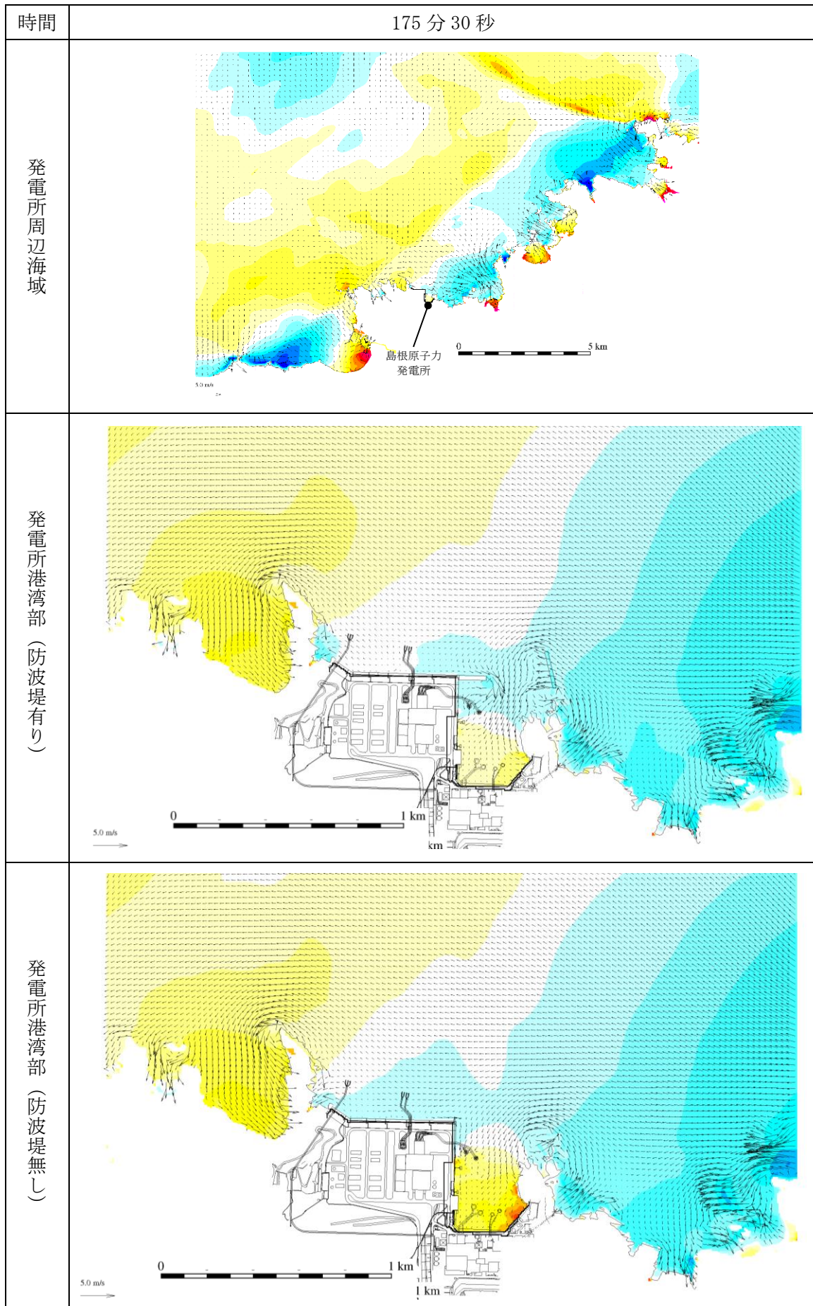
図 1-152 基準津波 1 の水位変動・流向ベクトル
