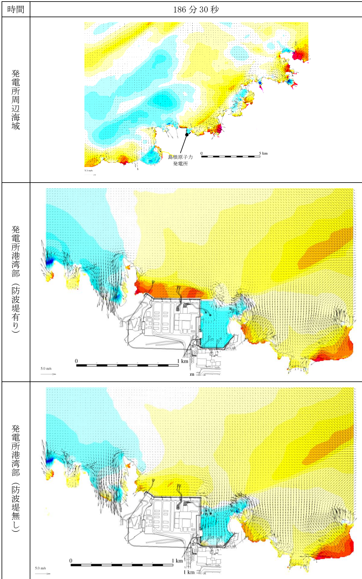
図 1-174 基準津波 1 の水位変動・流向ベクトル
