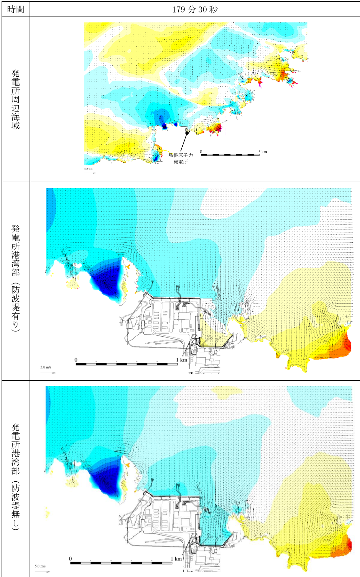
図 1-160 基準津波 1 の水位変動・流向ベクトル
