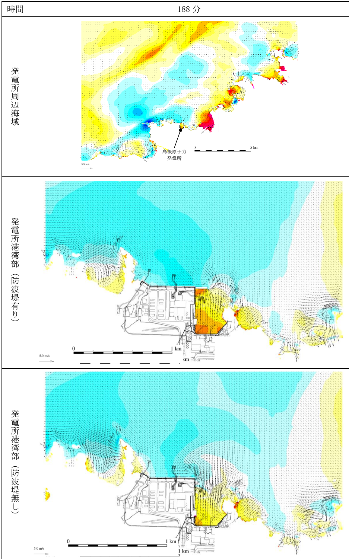
図 1-177 基準津波 1 の水位変動・流向ベクトル
