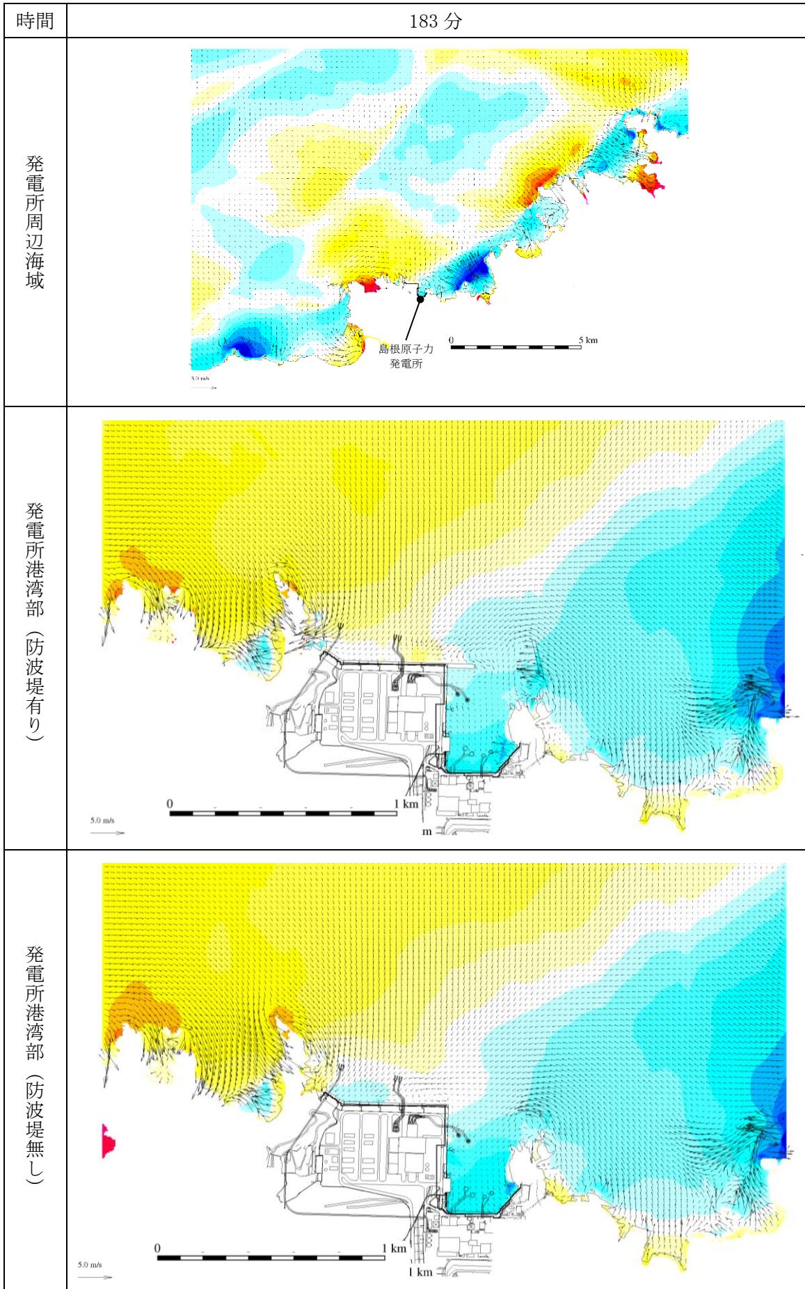
図 1-167 基準津波 1 の水位変動・流向ベクトル
