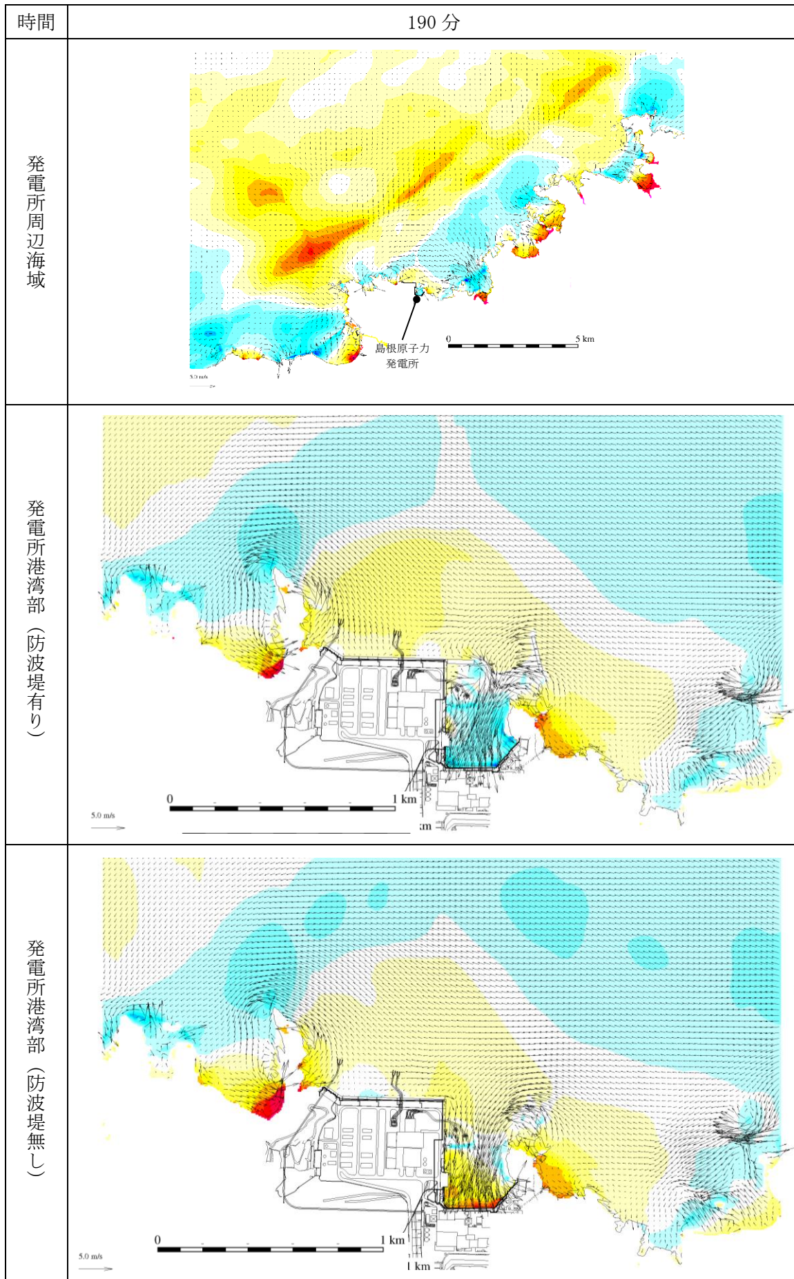
図 1-181 基準津波 1 の水位変動・流向ベクトル
