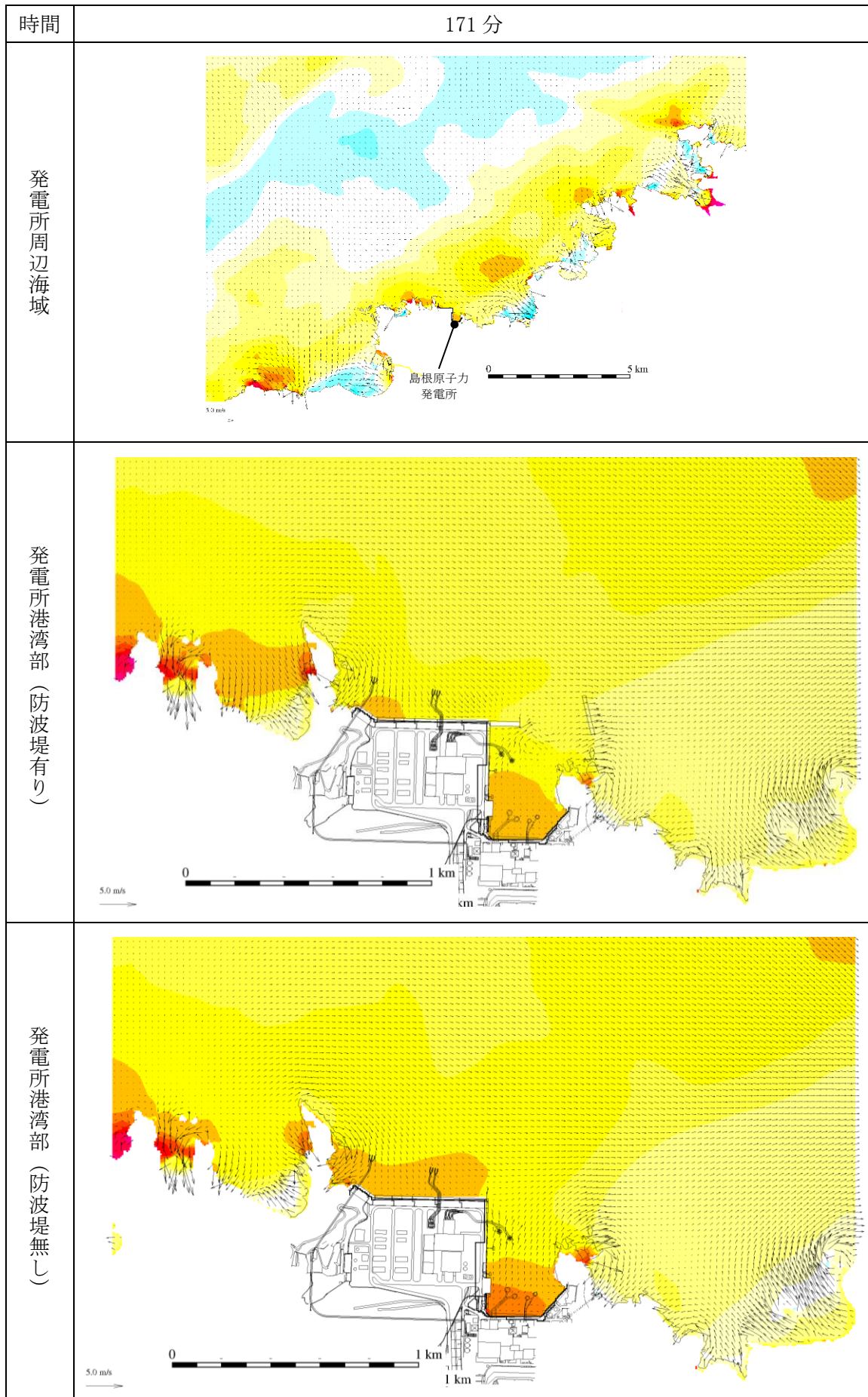
図 1-143 基準津波 1 の水位変動・流向ベクトル
