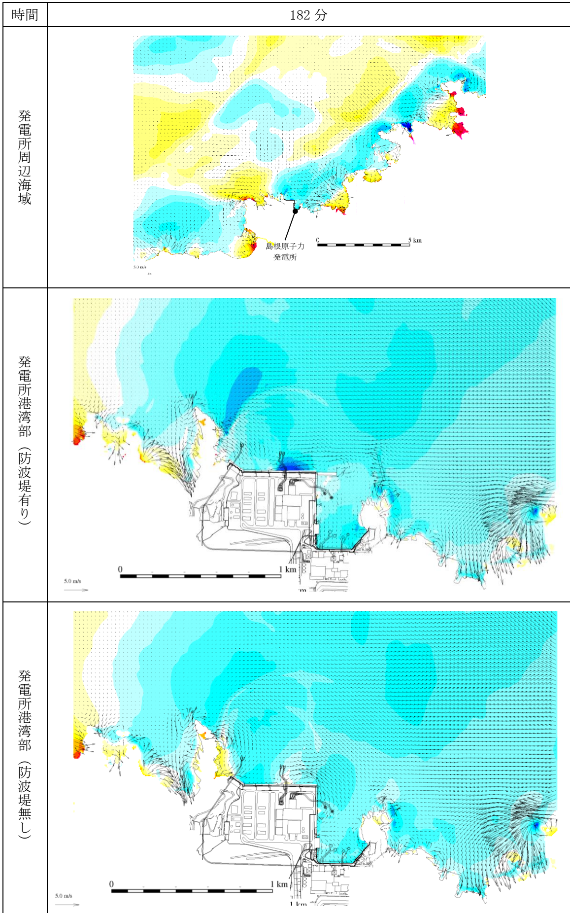
図 1-165 基準津波 1 の水位変動・流向ベクトル
