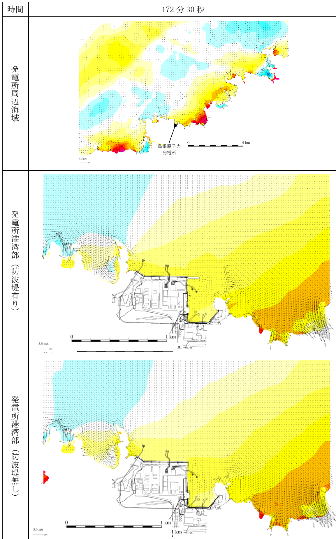
図 1-146 基準津波 1 の水位変動・流向ベクトル
