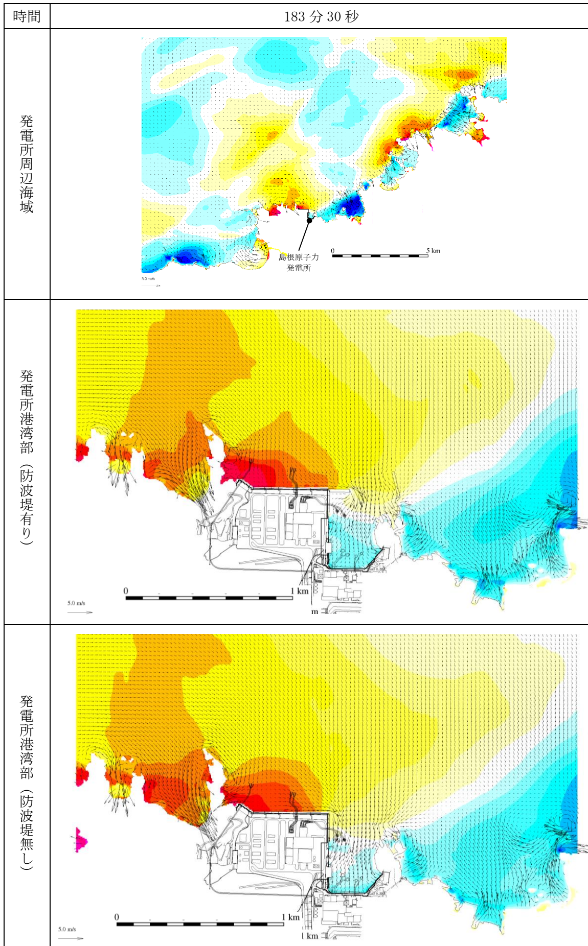
図 1-168 基準津波 1 の水位変動・流向ベクトル
