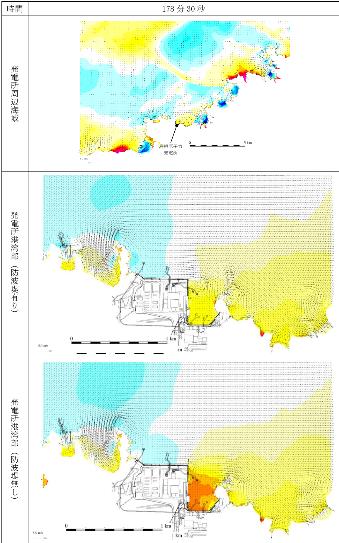
図 1-158 基準津波 1 の水位変動・流向ベクトル
