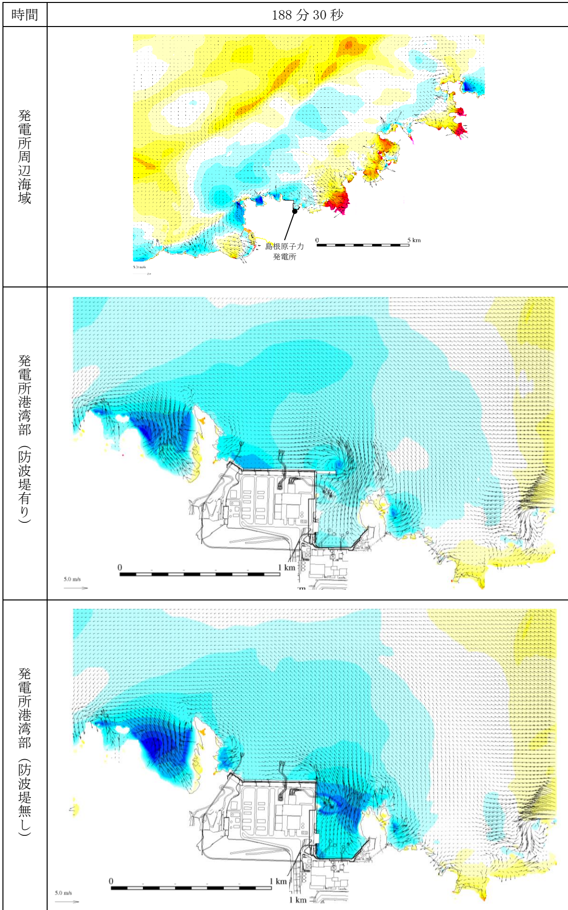
図 1-178 基準津波 1 の水位変動・流向ベクトル
