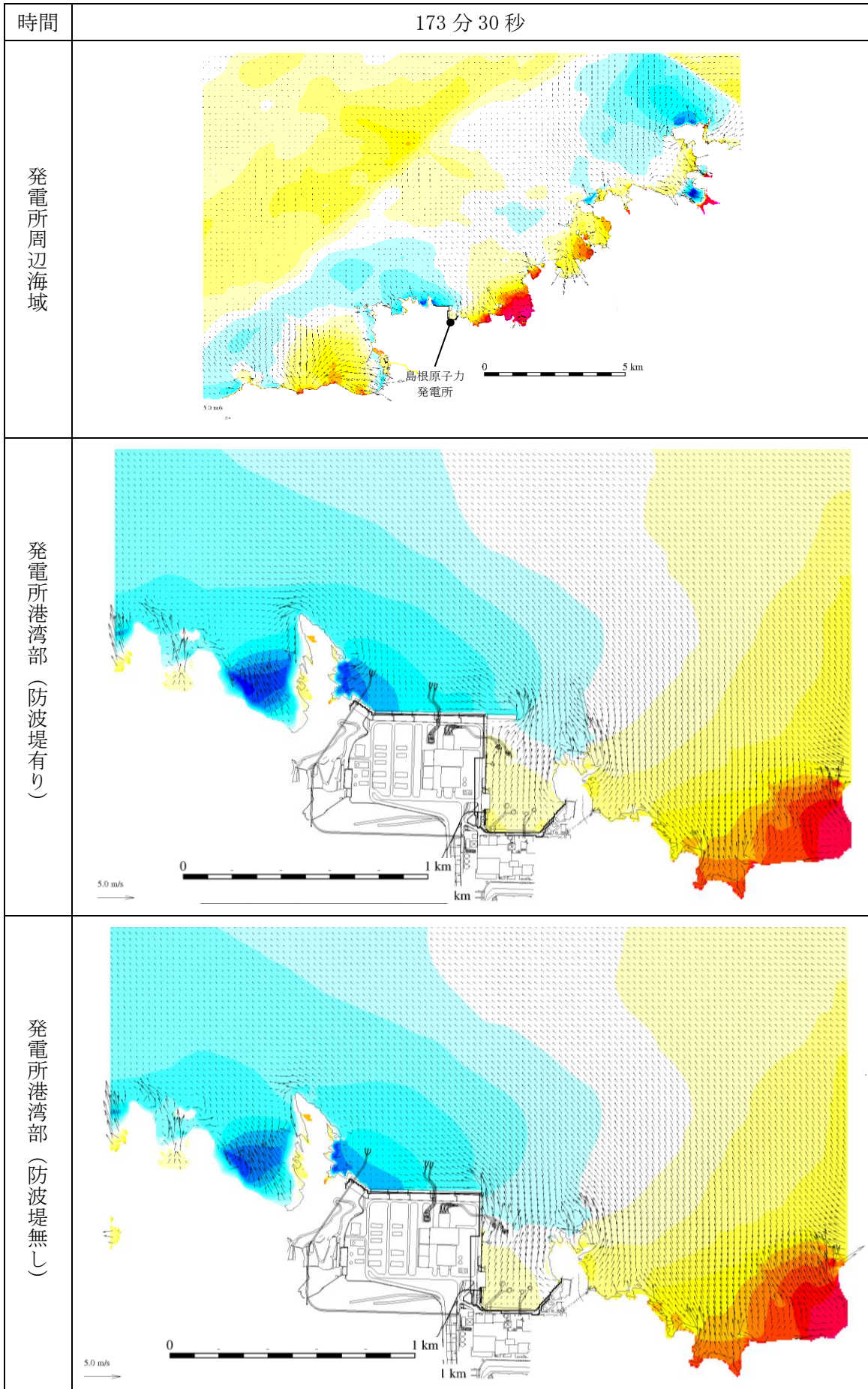
図 1-148 基準津波 1 の水位変動・流向ベクトル
