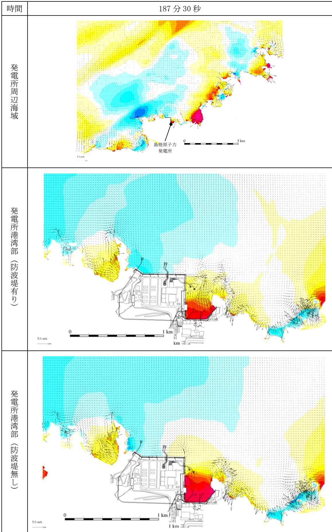
図 1-176 基準津波 1 の水位変動・流向ベクトル
