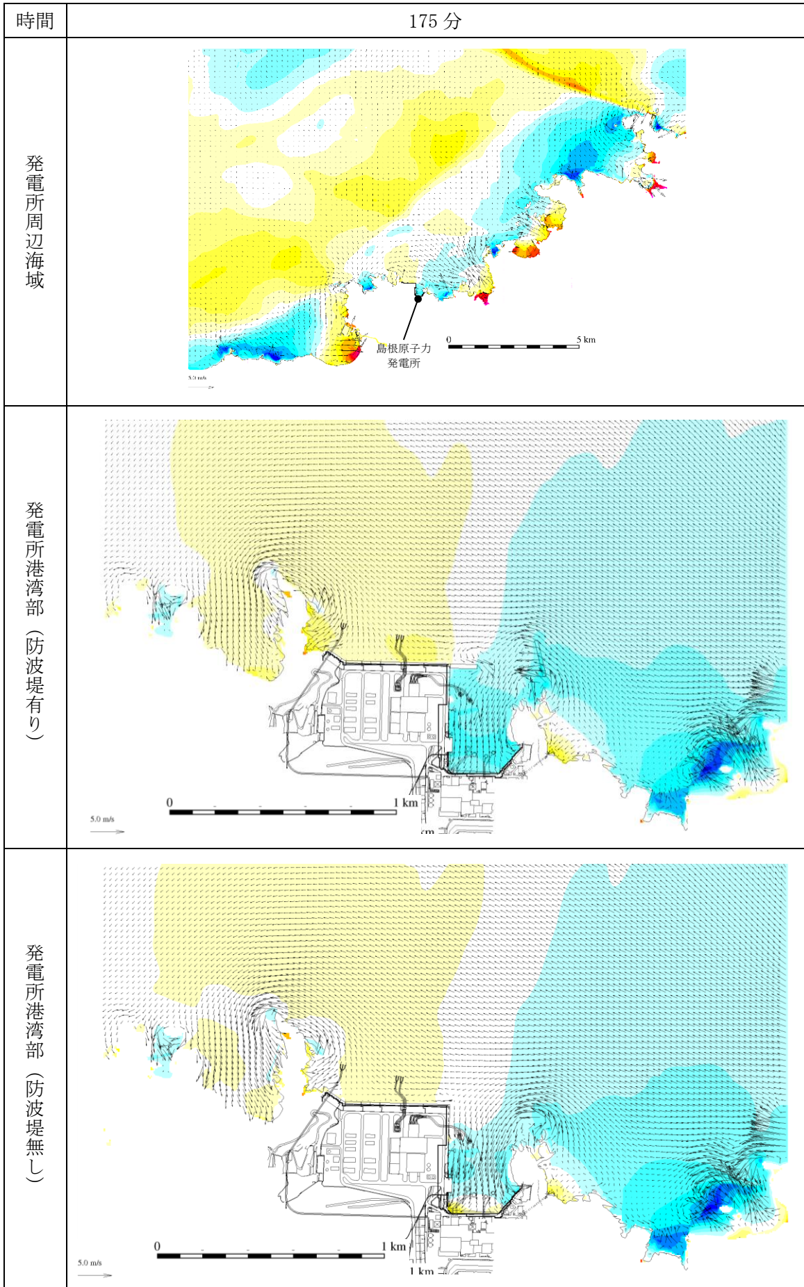
図 1-151 基準津波 1 の水位変動・流向ベクトル
