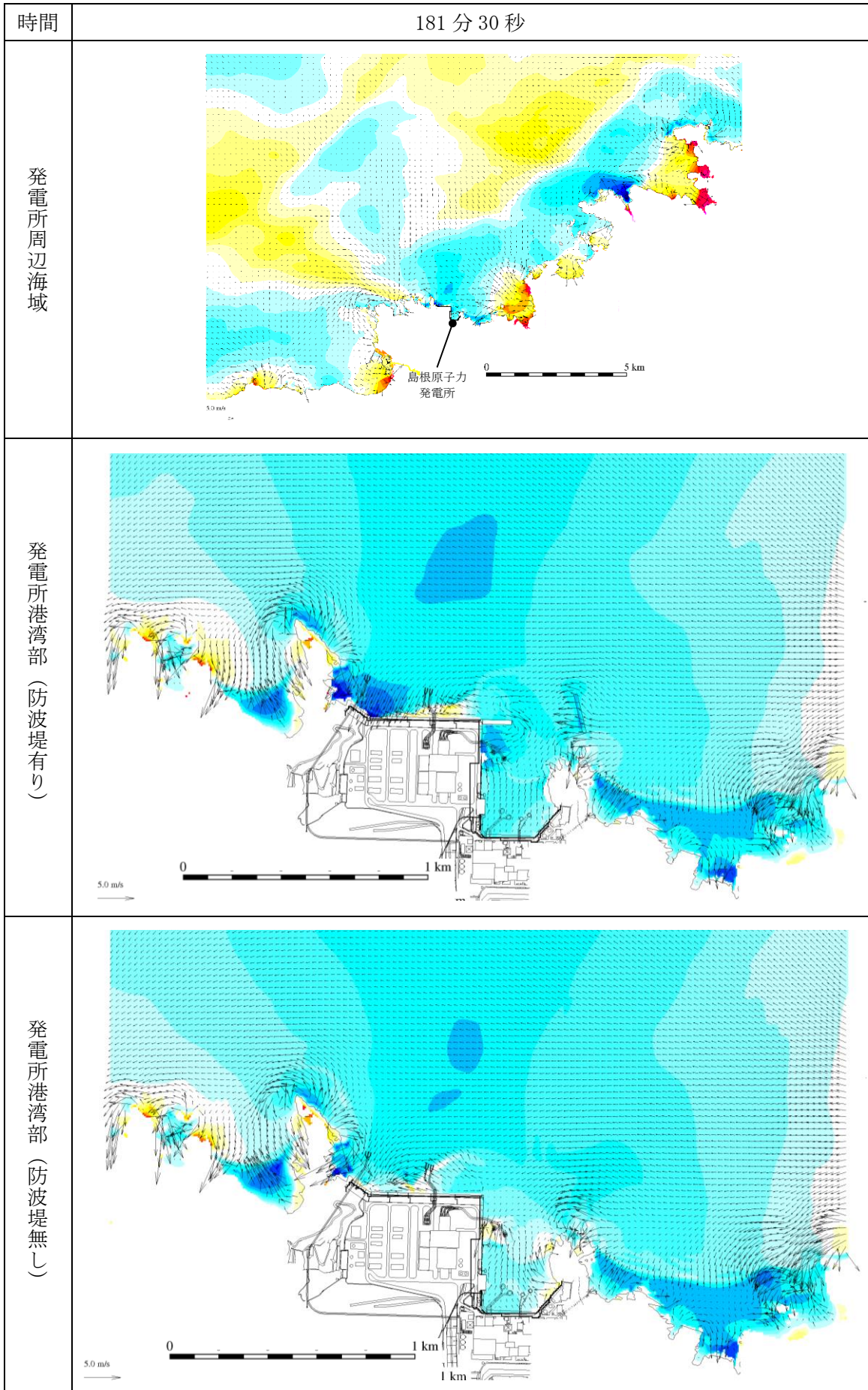
図 1-164 基準津波 1 の水位変動・流向ベクトル
