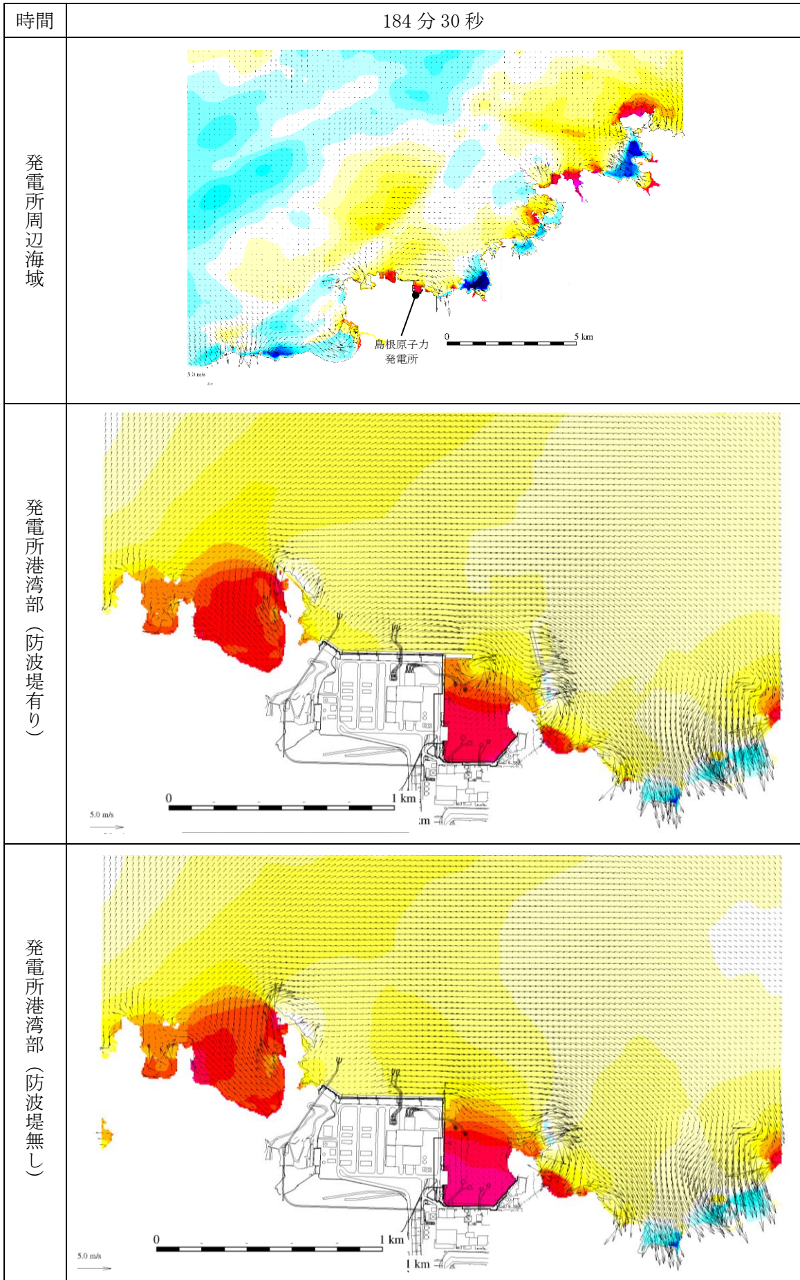
図 1-170 基準津波 1 の水位変動・流向ベクトル
