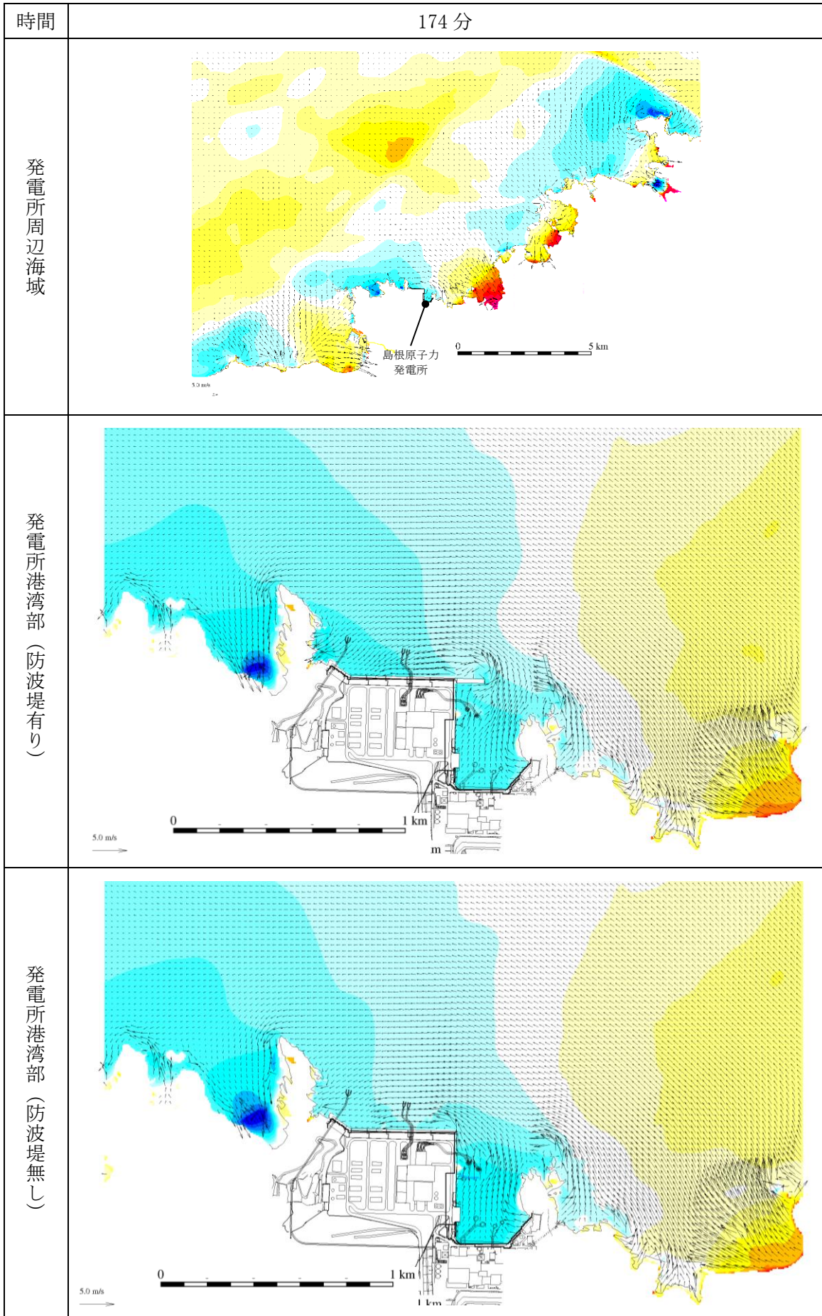
図 1-149 基準津波 1 の水位変動・流向ベクトル
