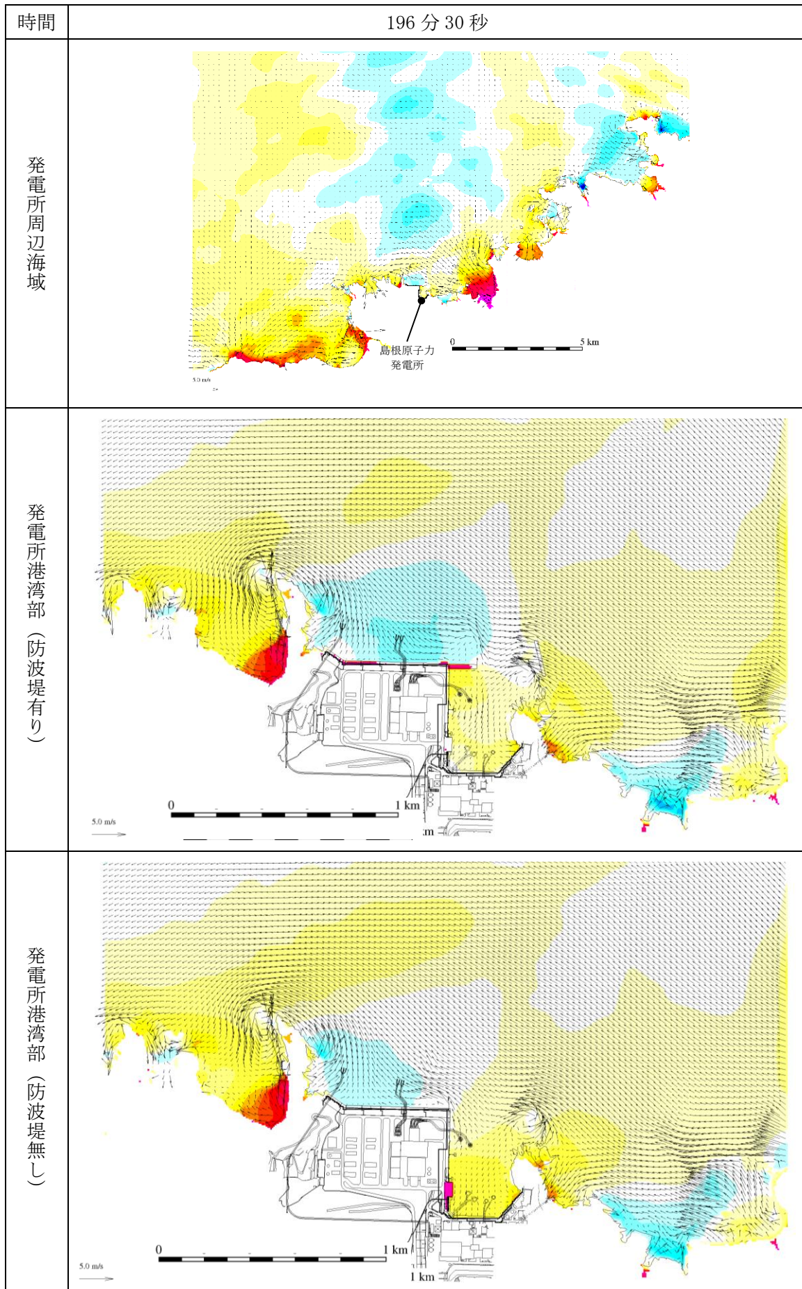
図 1-194 基準津波 1 の水位変動・流向ベクトル
