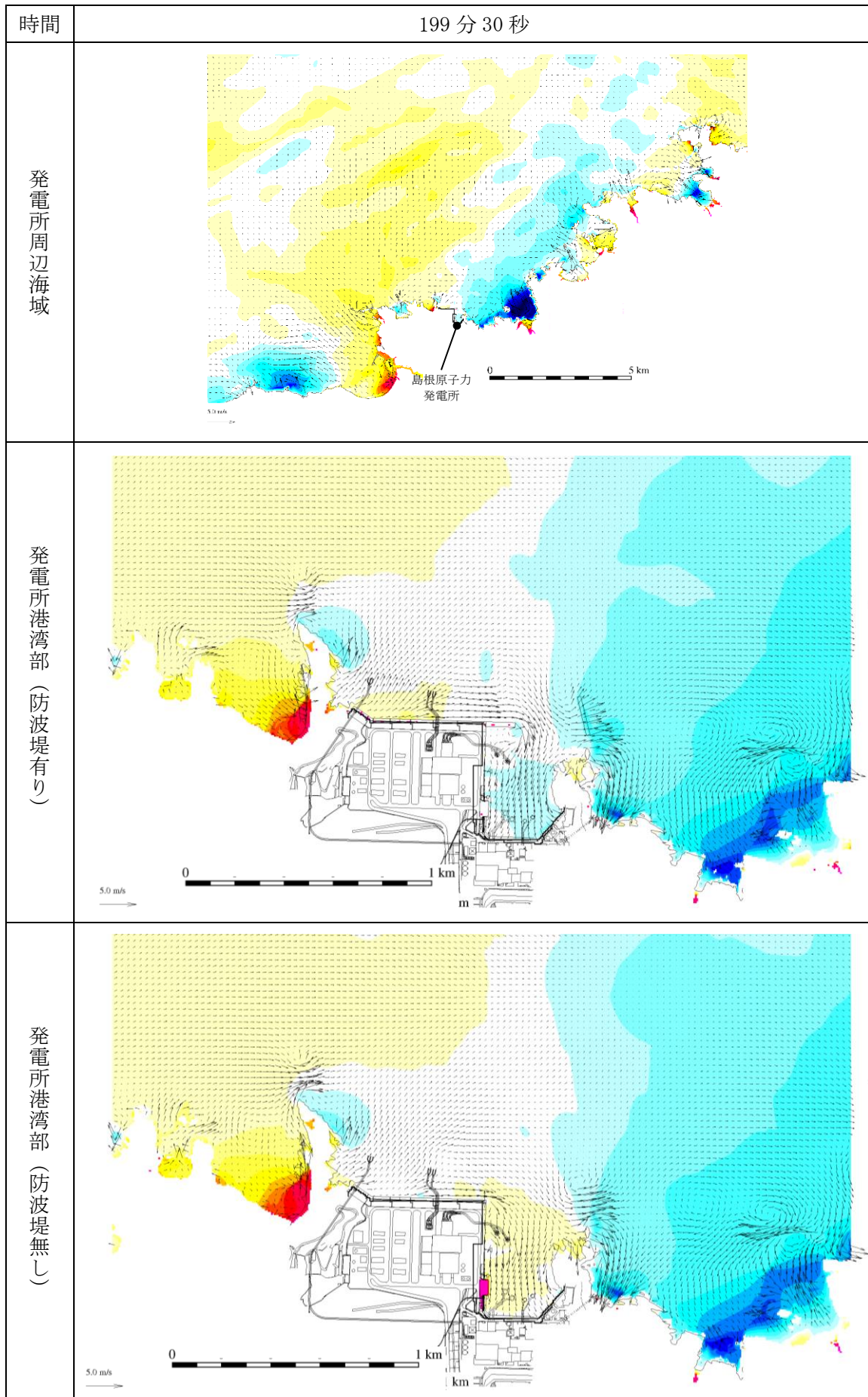
図 1-200 基準津波 1 の水位変動・流向ベクトル
