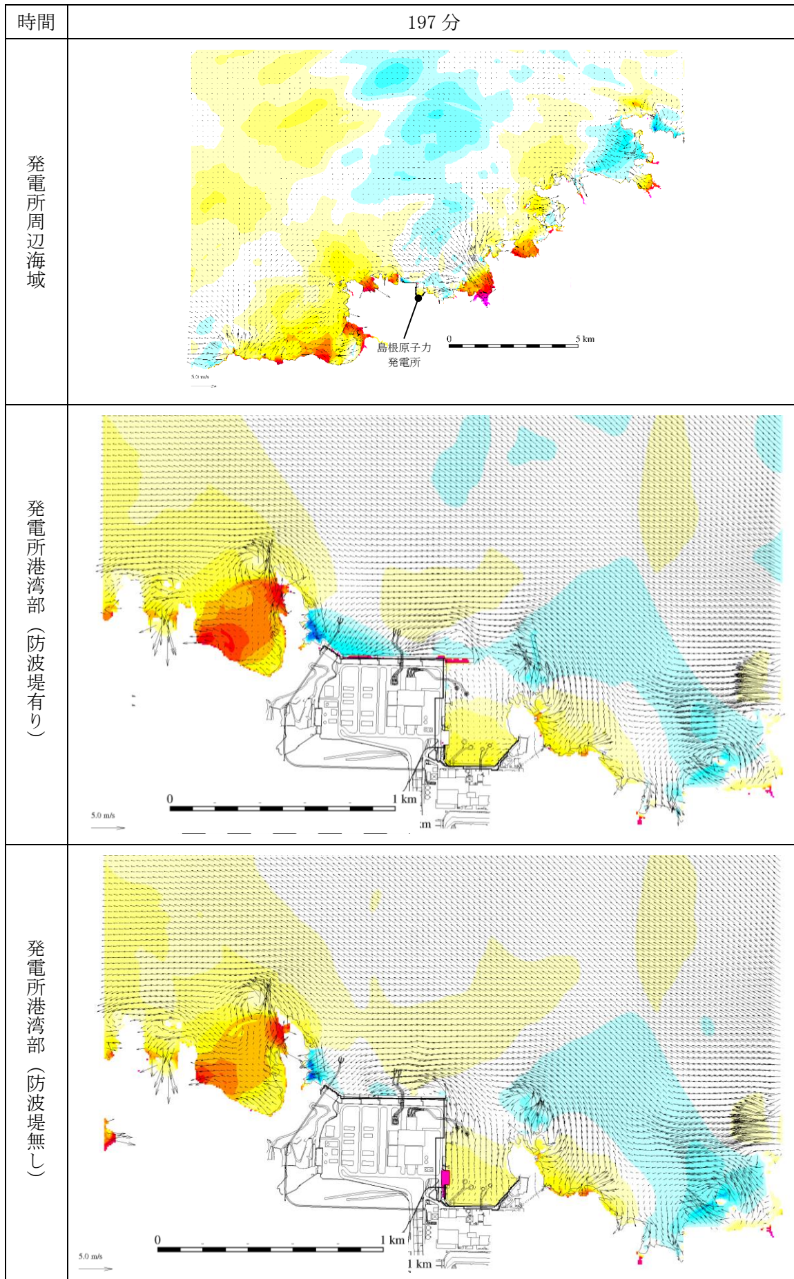
図 1-195 基準津波 1 の水位変動・流向ベクトル
