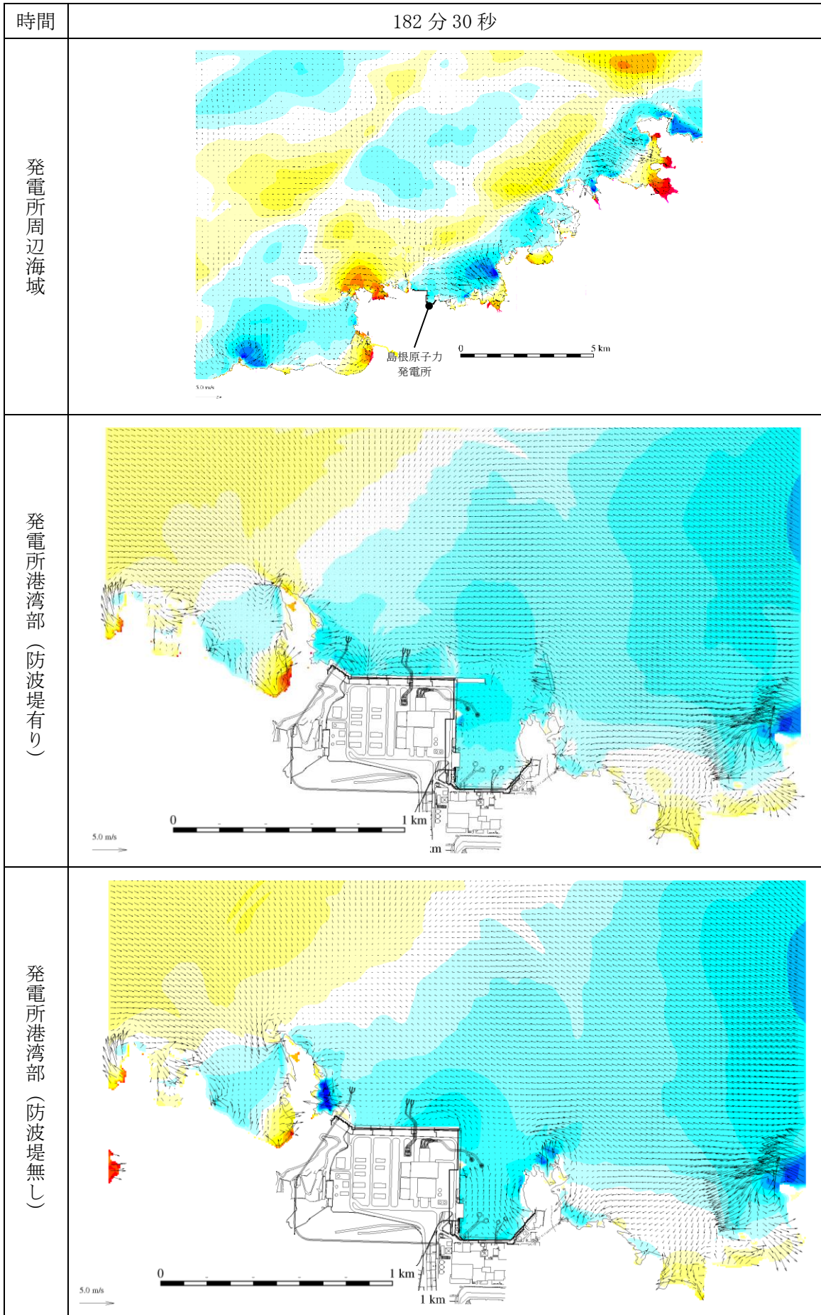
図 1-166 基準津波 1 の水位変動・流向ベクトル
