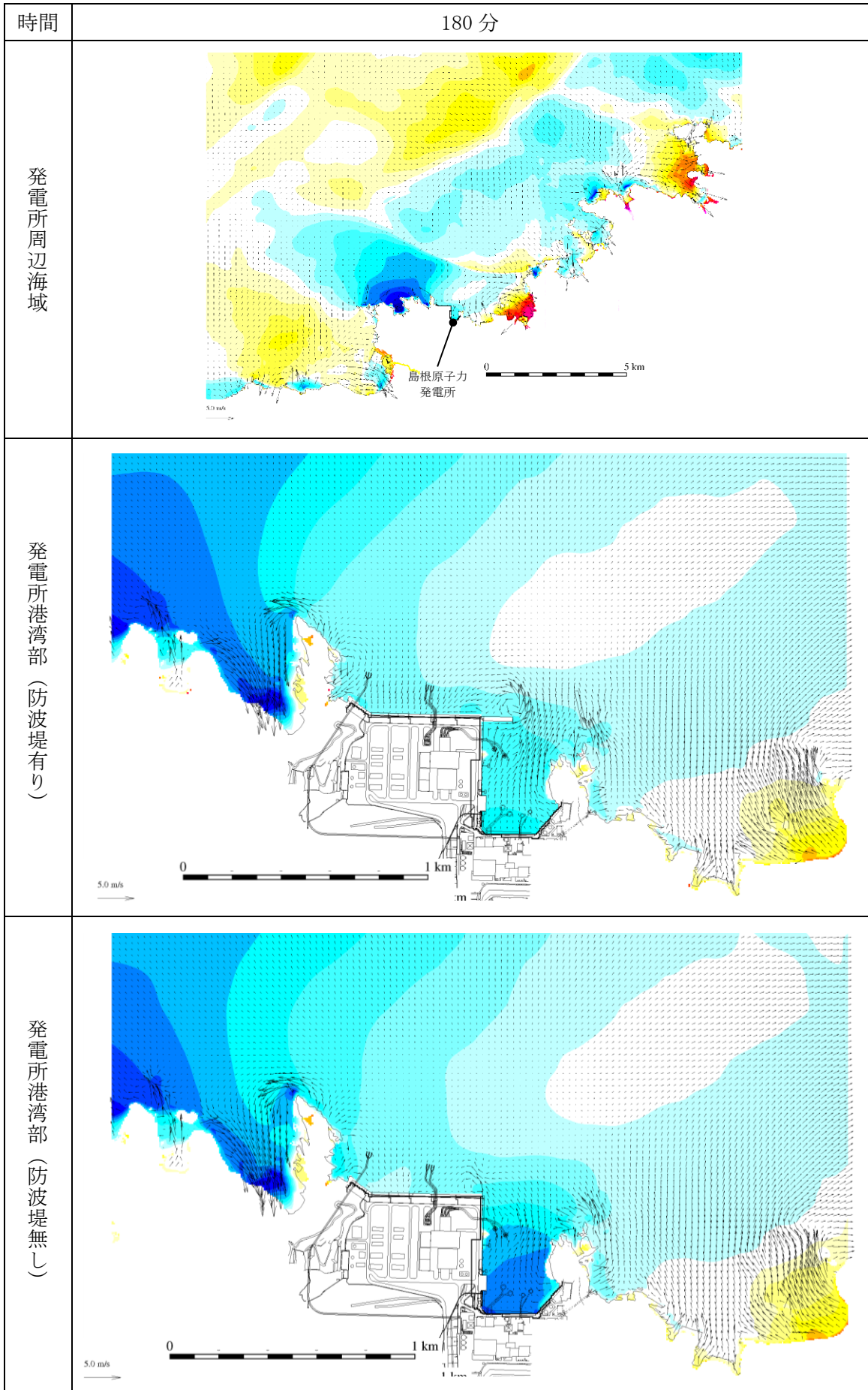
図 1-161 基準津波 1 の水位変動・流向ベクトル
