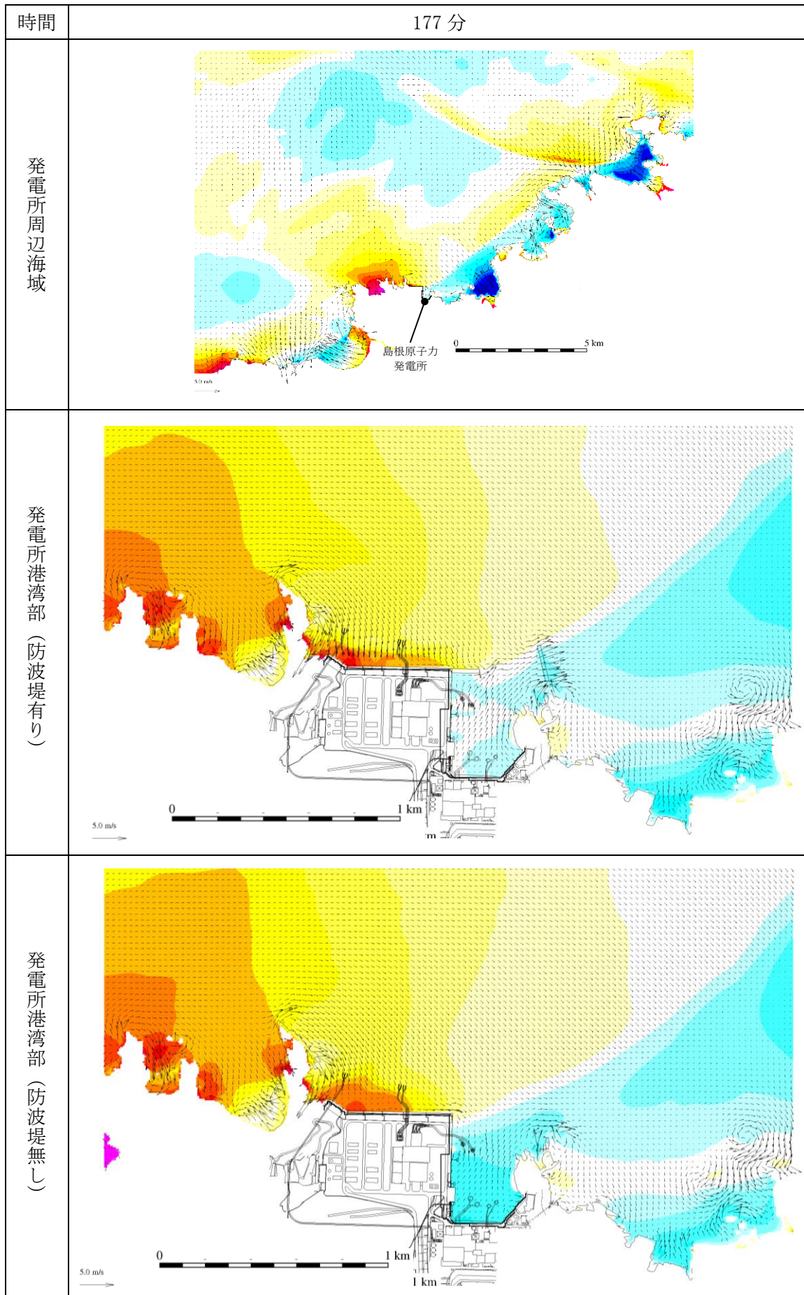
図 1-155 基準津波 1 の水位変動・流向ベクトル
