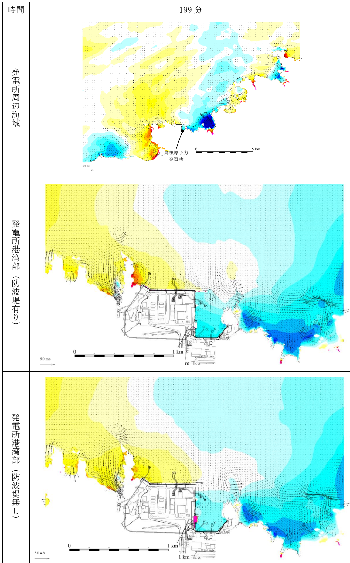
図 1-199 基準津波 1 の水位変動・流向ベクトル
