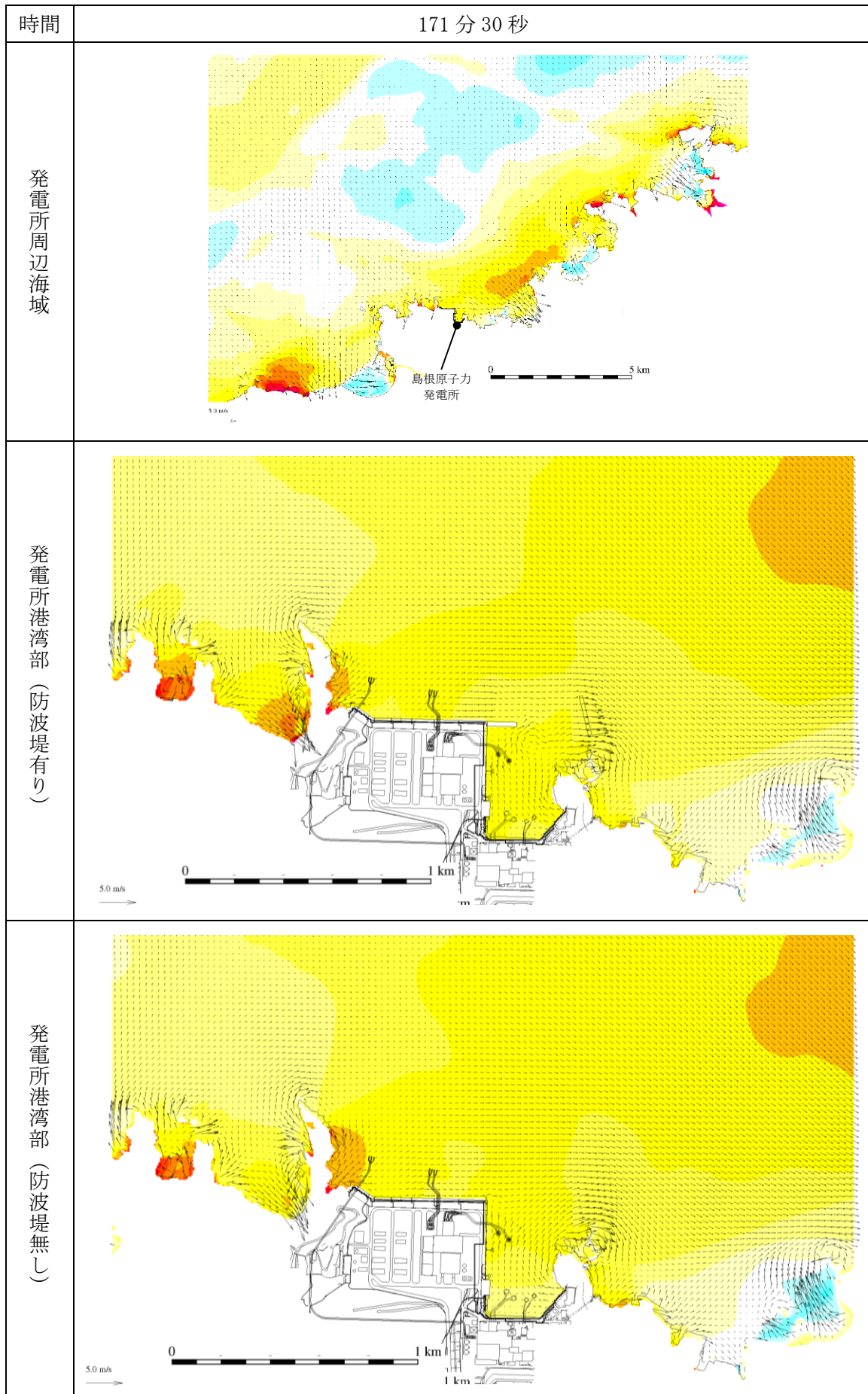
図 1-144 基準津波 1 の水位変動・流向ベクトル
