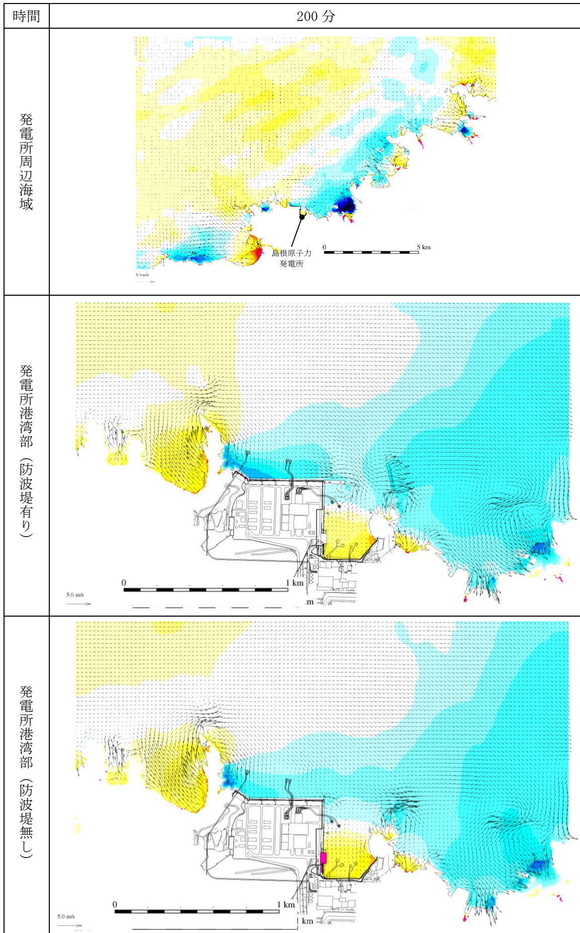
図 1-201 基準津波 1 の水位変動・流向ベクトル
