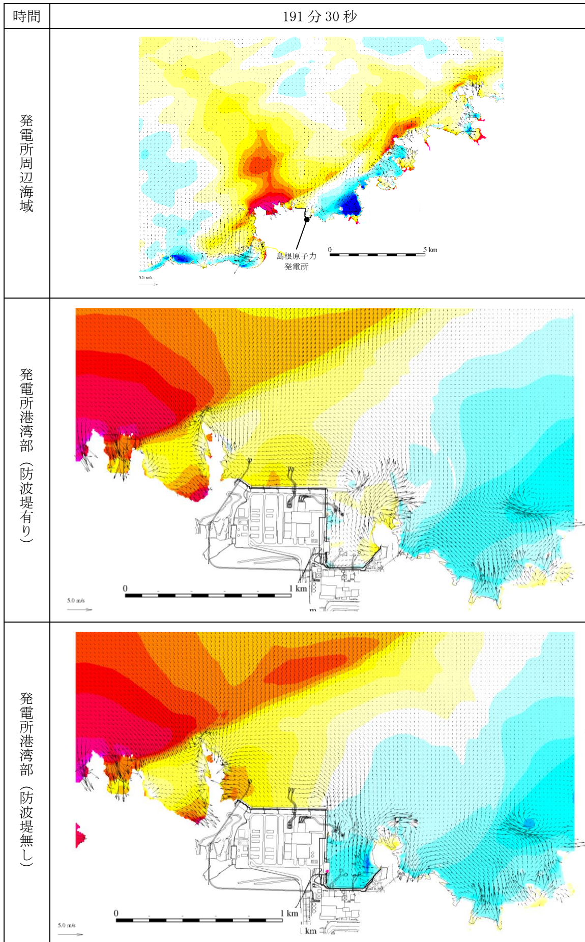
図 1-184 基準津波 1 の水位変動・流向ベクトル
