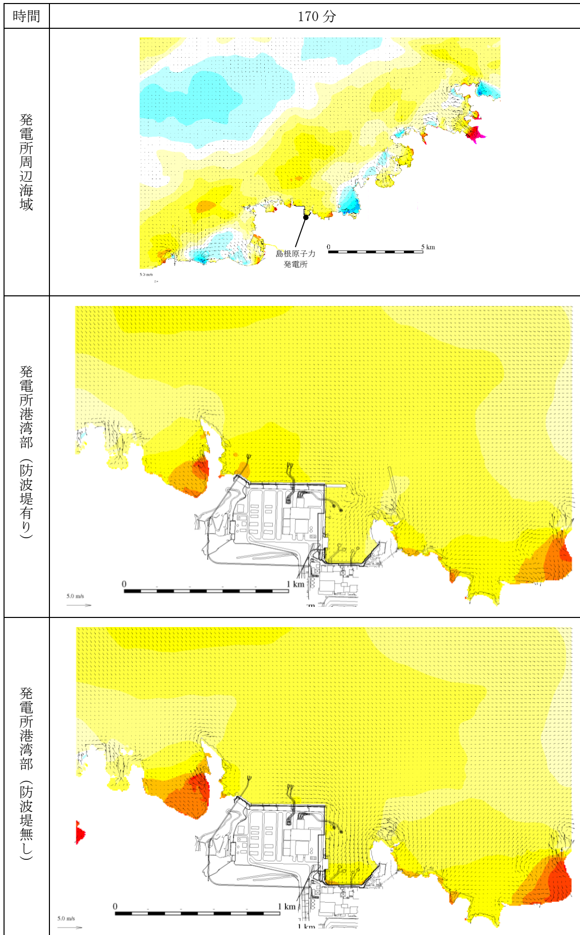
図 1-141 基準津波 1 の水位変動・流向ベクトル
