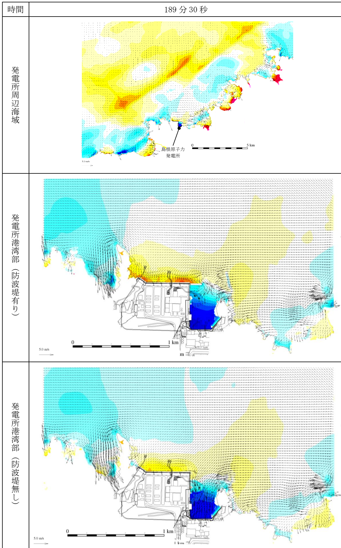
図 1-180 基準津波 1 の水位変動・流向ベクトル
