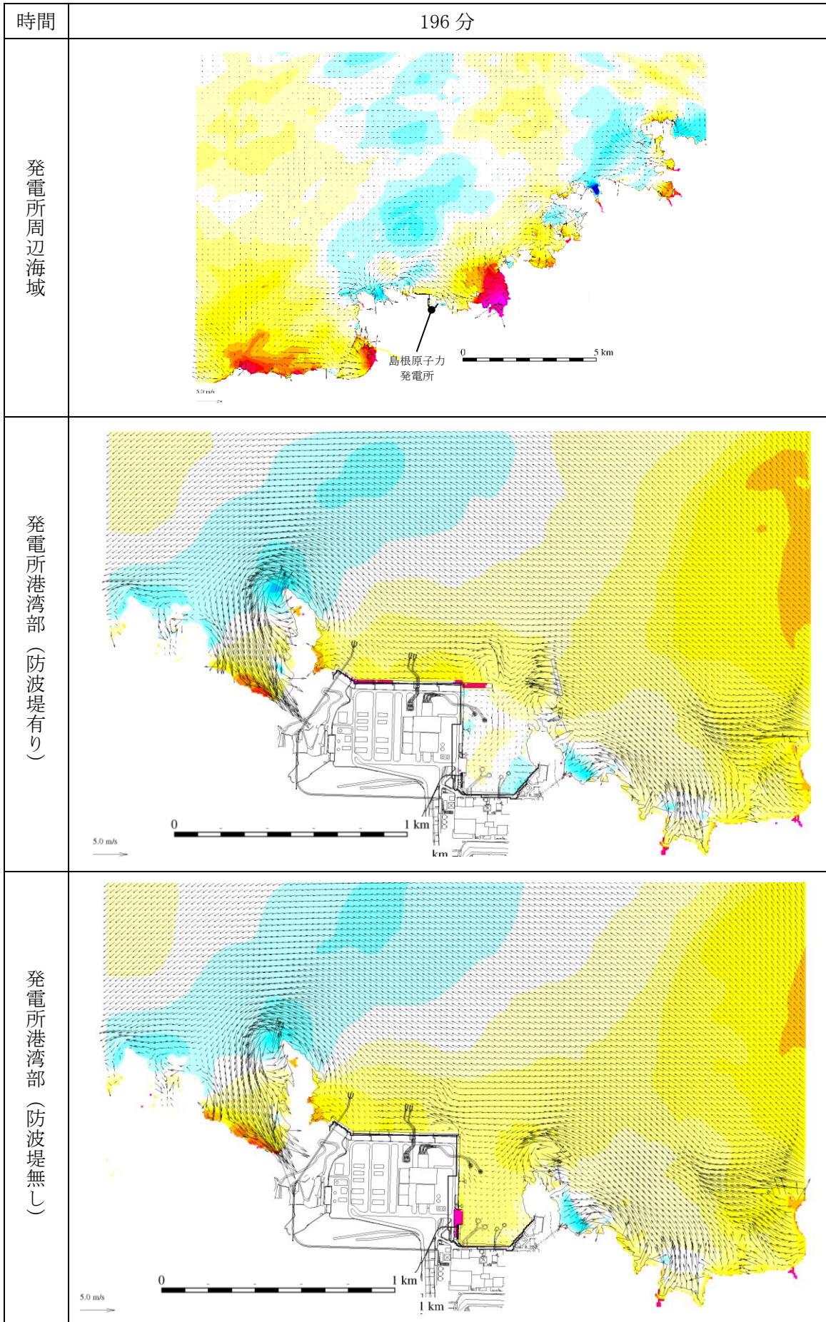
図 1-193 基準津波 1 の水位変動・流向ベクトル
