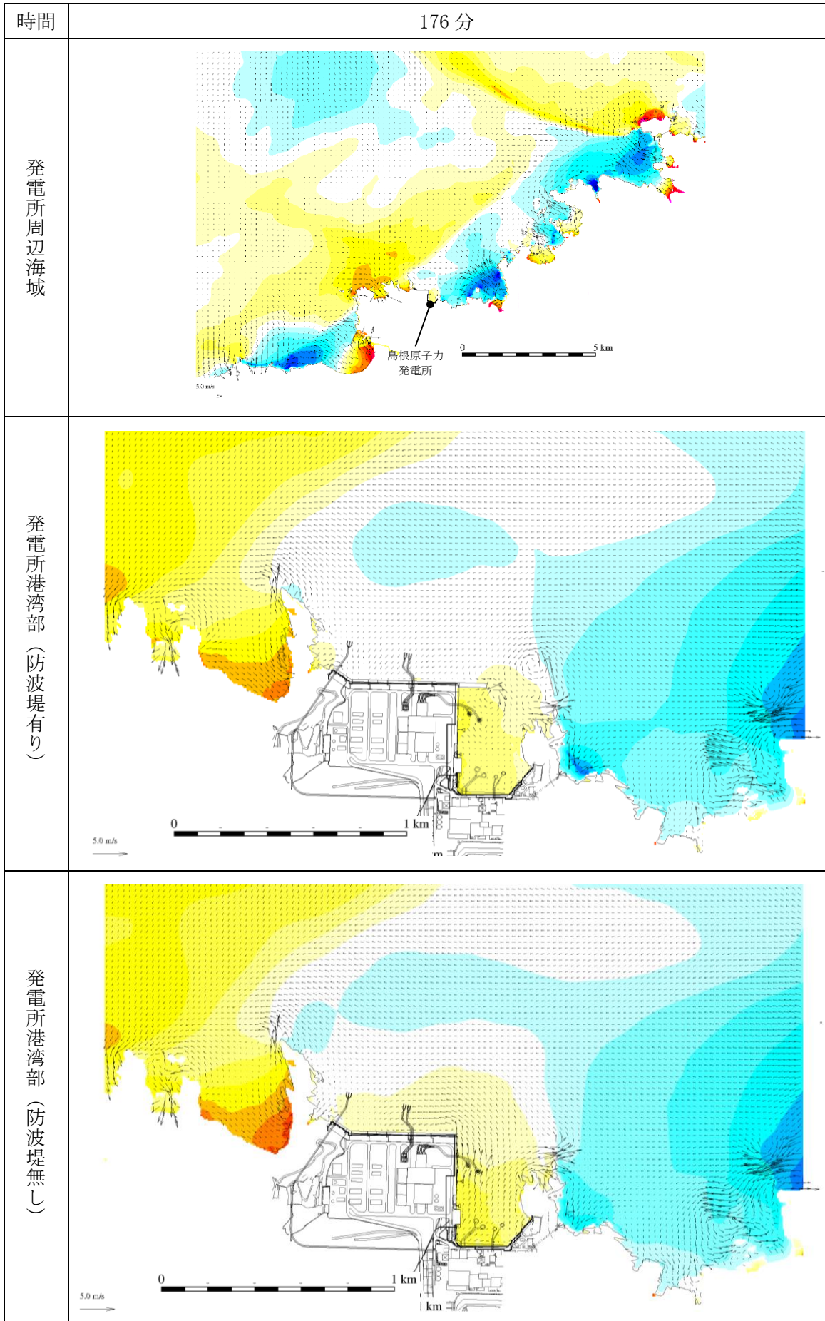
図 1-153 基準津波 1 の水位変動・流向ベクトル
