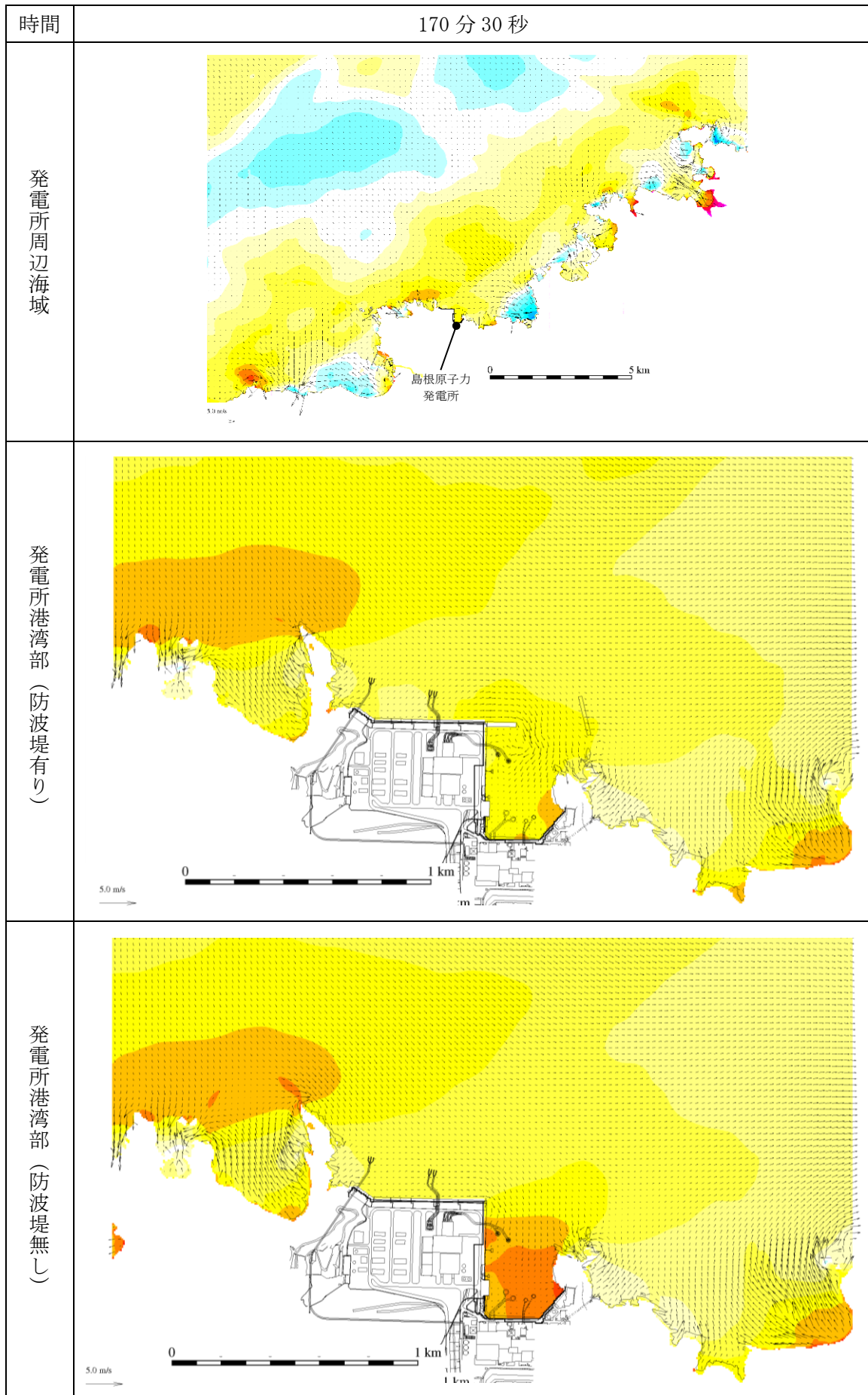
図 1-142 基準津波 1 の水位変動・流向ベクトル
