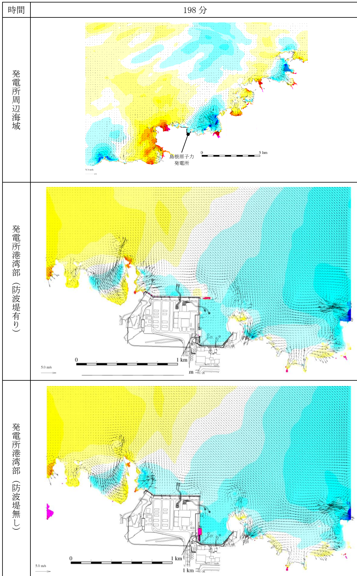
図 1-197 基準津波 1 の水位変動・流向ベクトル
