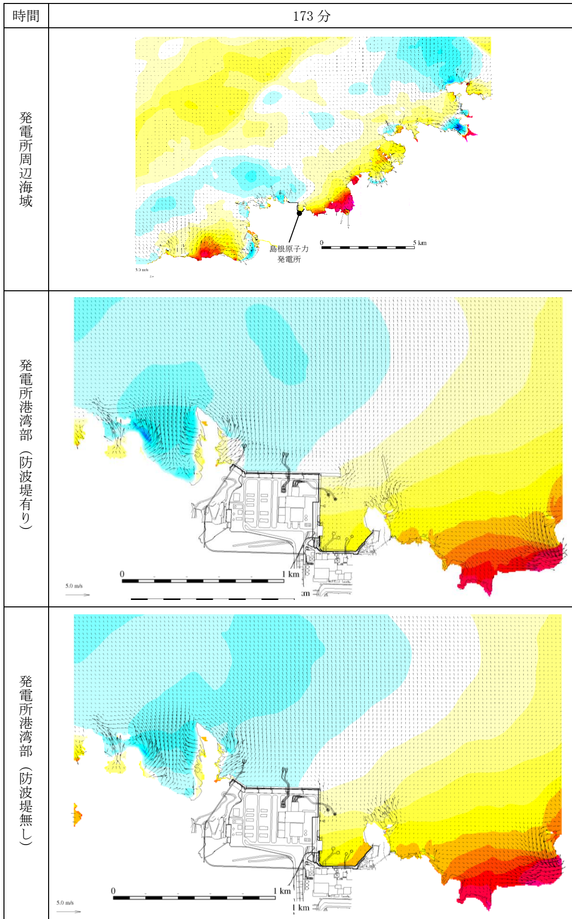
図 1-147 基準津波 1 の水位変動・流向ベクトル
