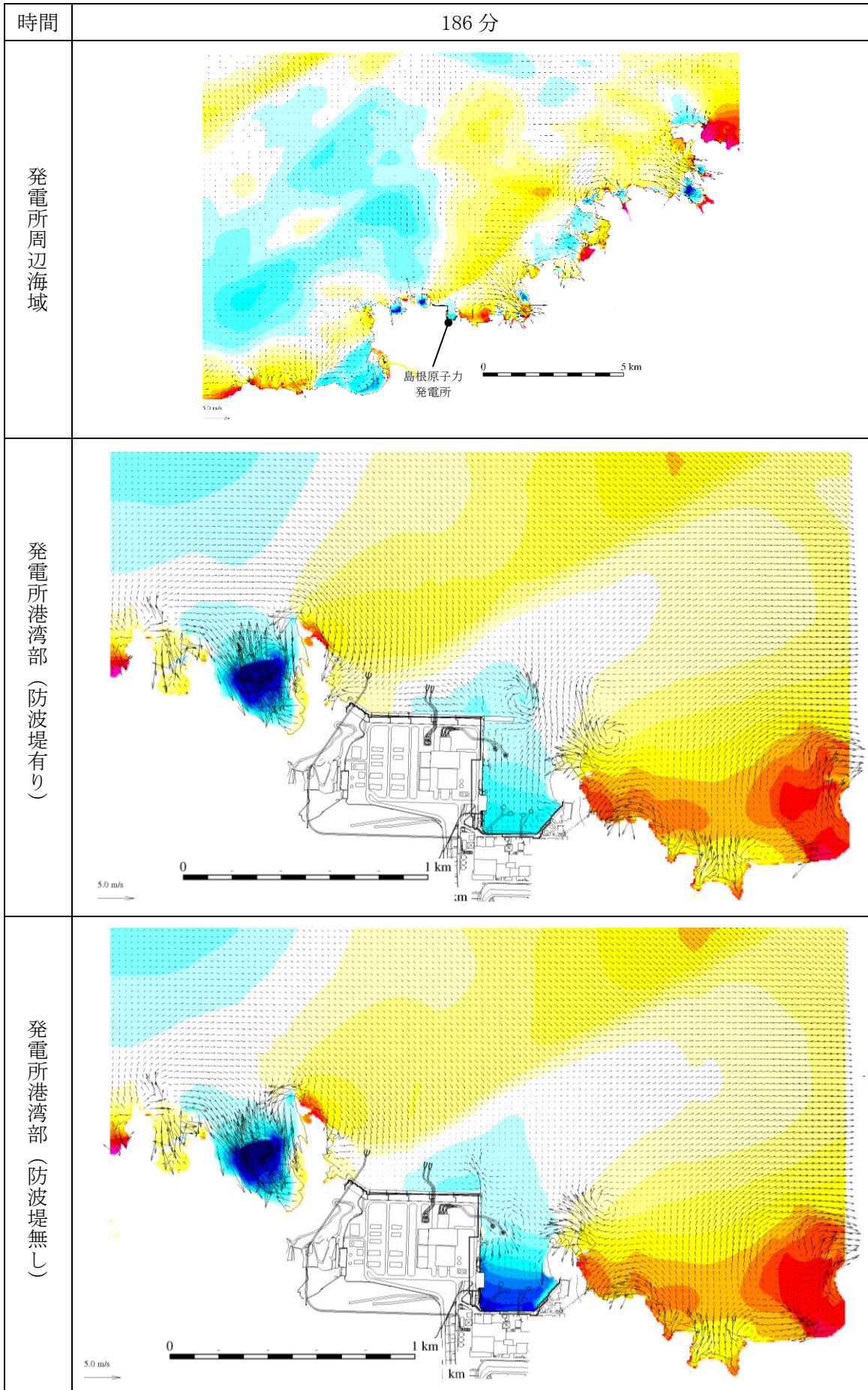
図 1-173 基準津波 1 の水位変動・流向ベクトル
