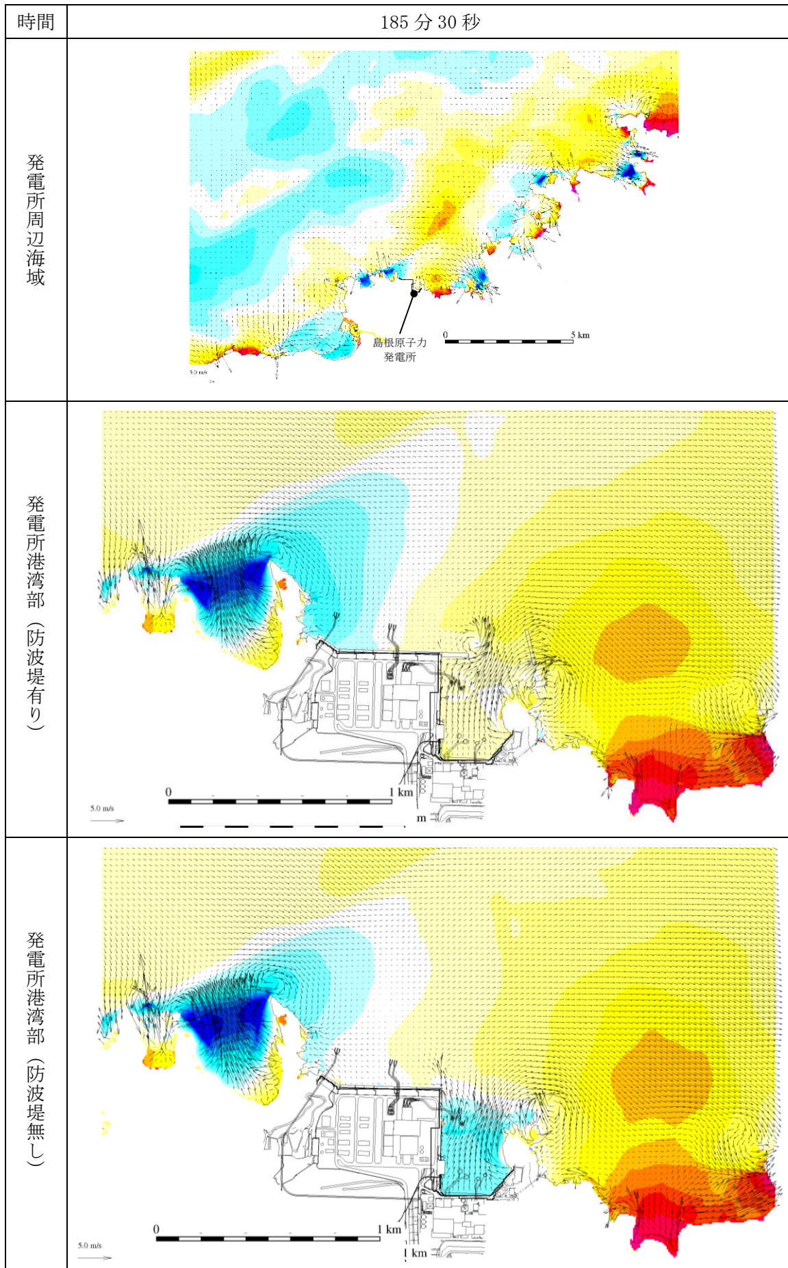
図 1-172 基準津波 1 の水位変動・流向ベクトル
