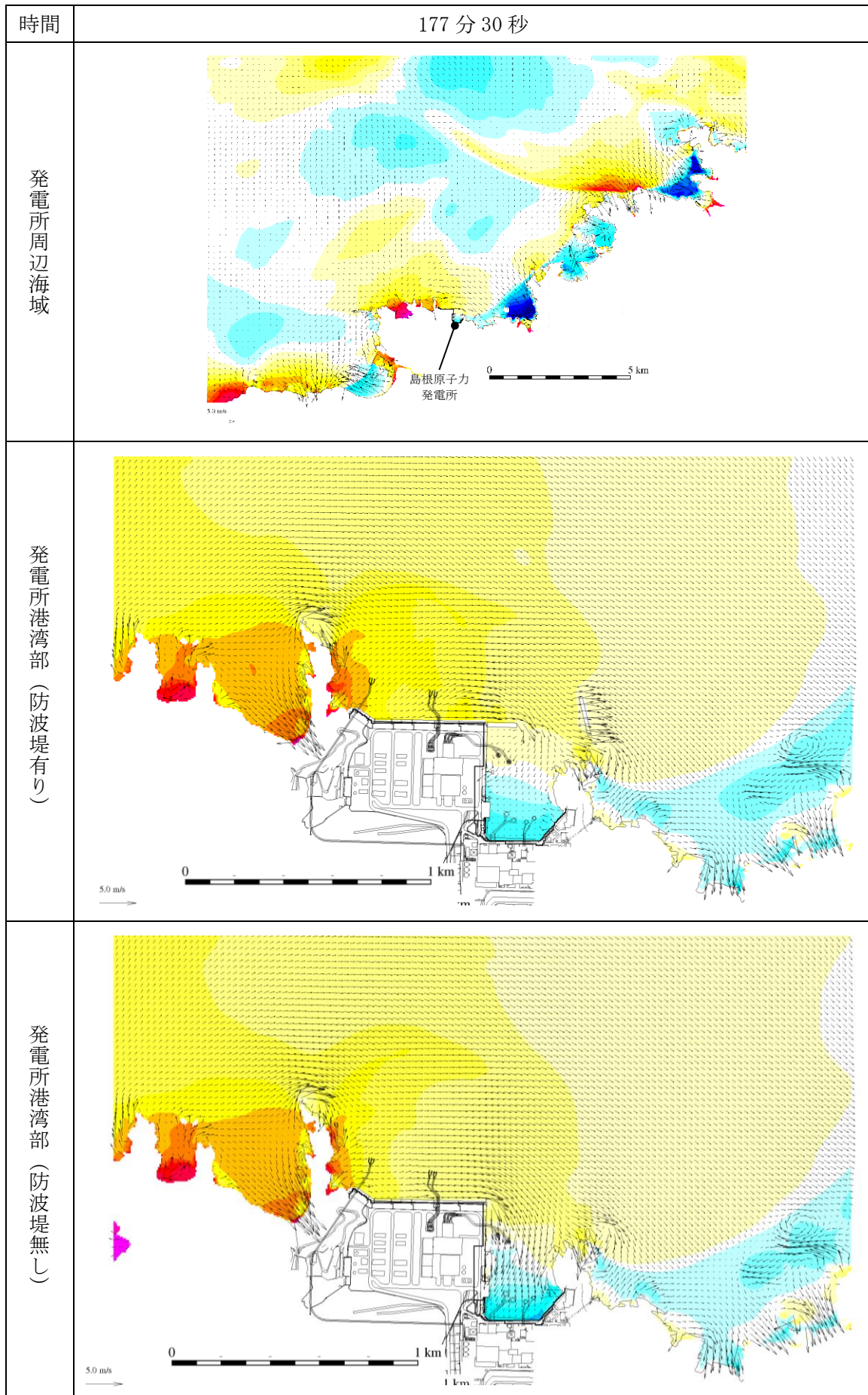
図 1-156 基準津波 1 の水位変動・流向ベクトル
