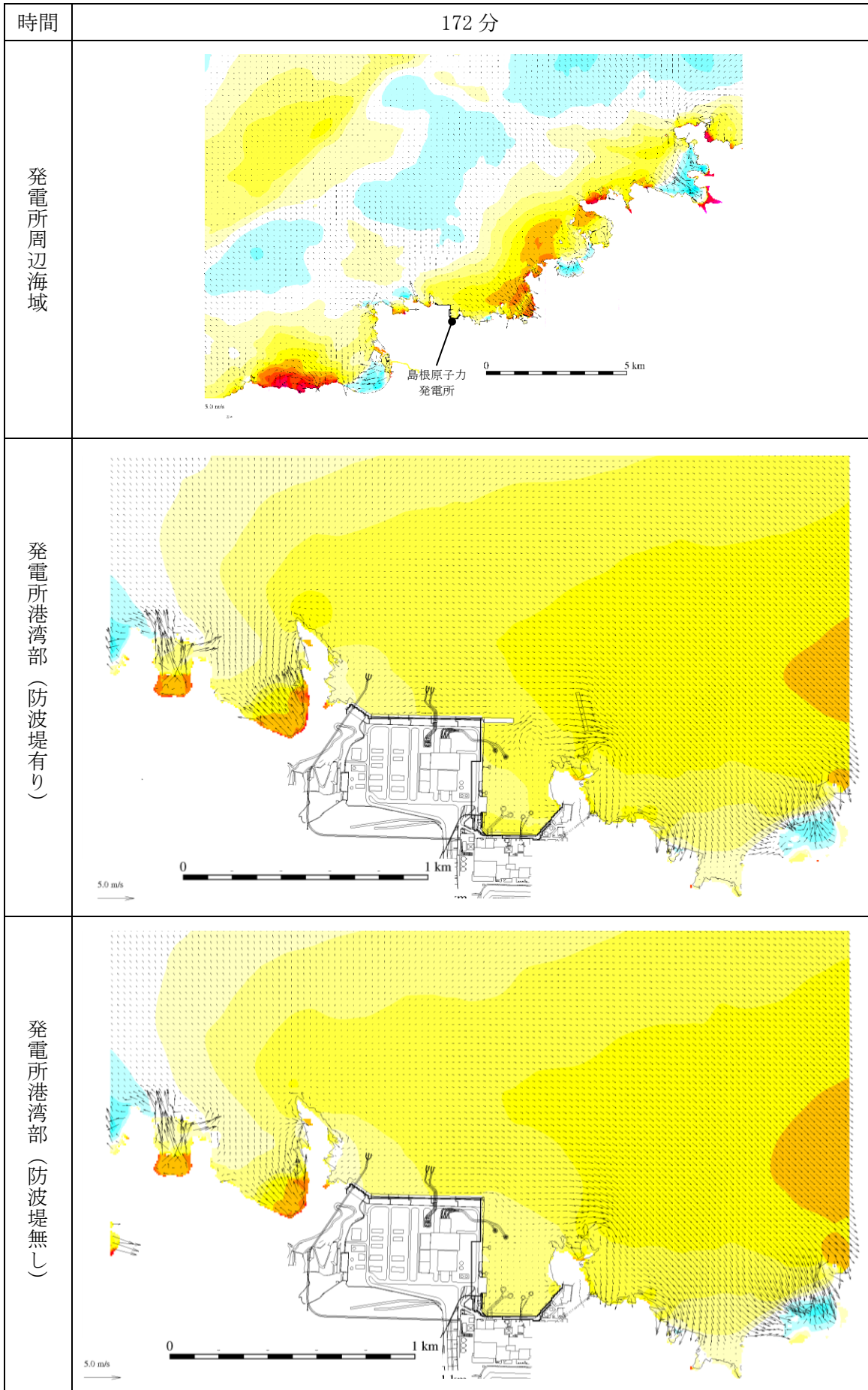
図 1-145 基準津波 1 の水位変動・流向ベクトル
