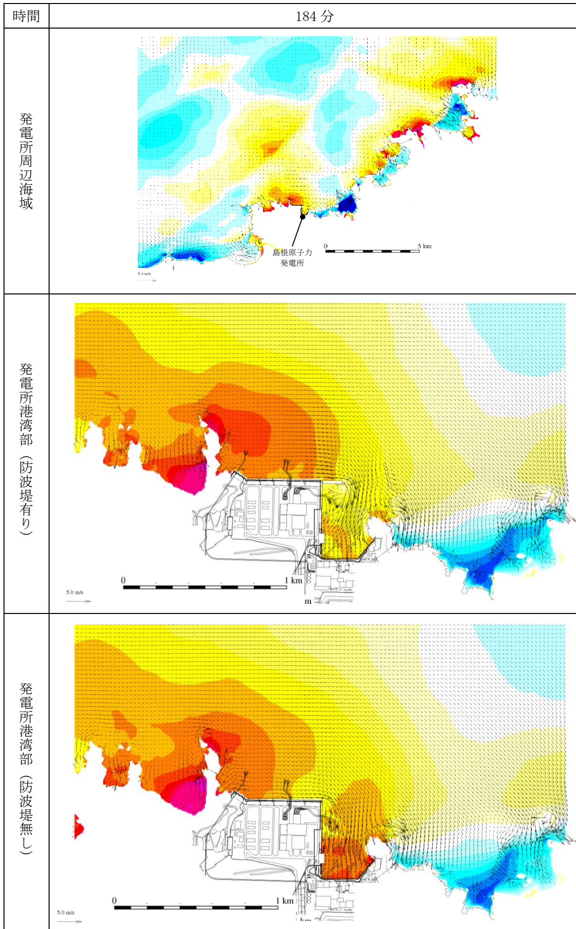
図 1-169 基準津波 1 の水位変動・流向ベクトル
