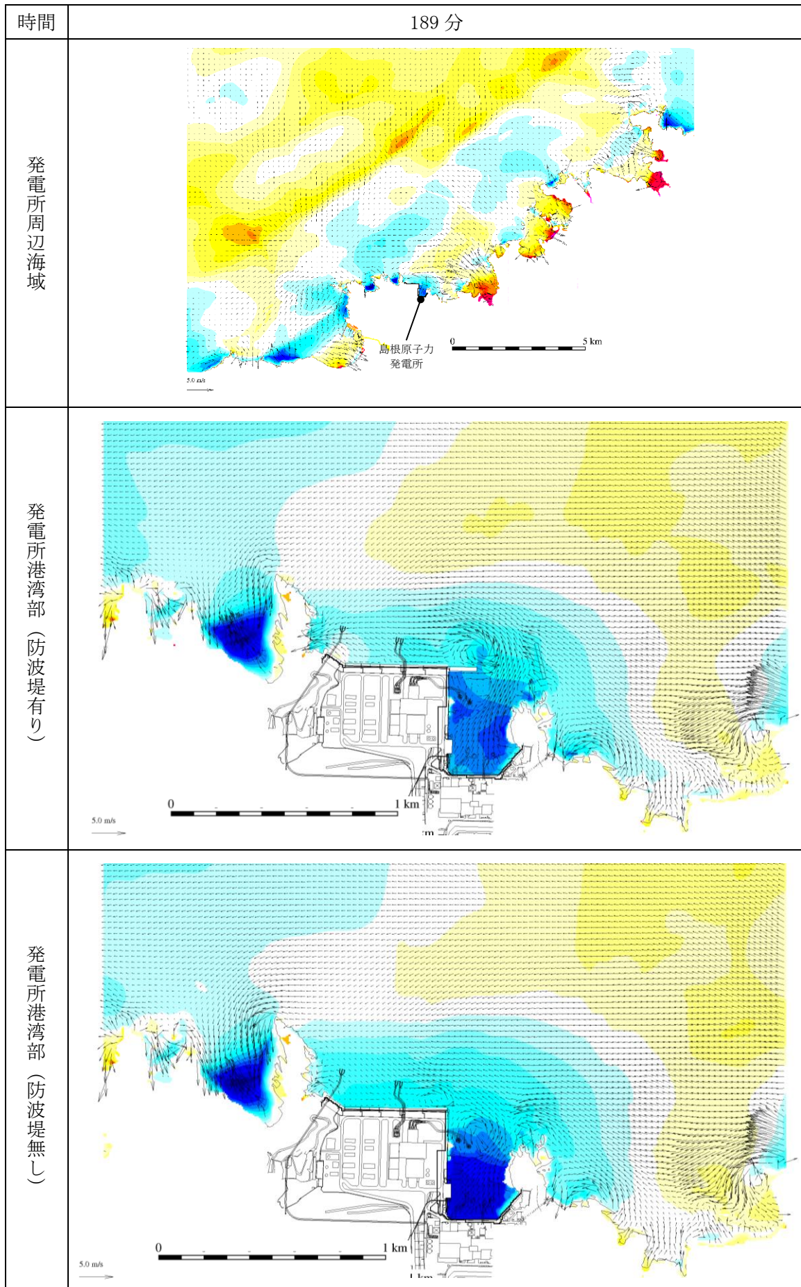
図 1-179 基準津波 1 の水位変動・流向ベクトル
