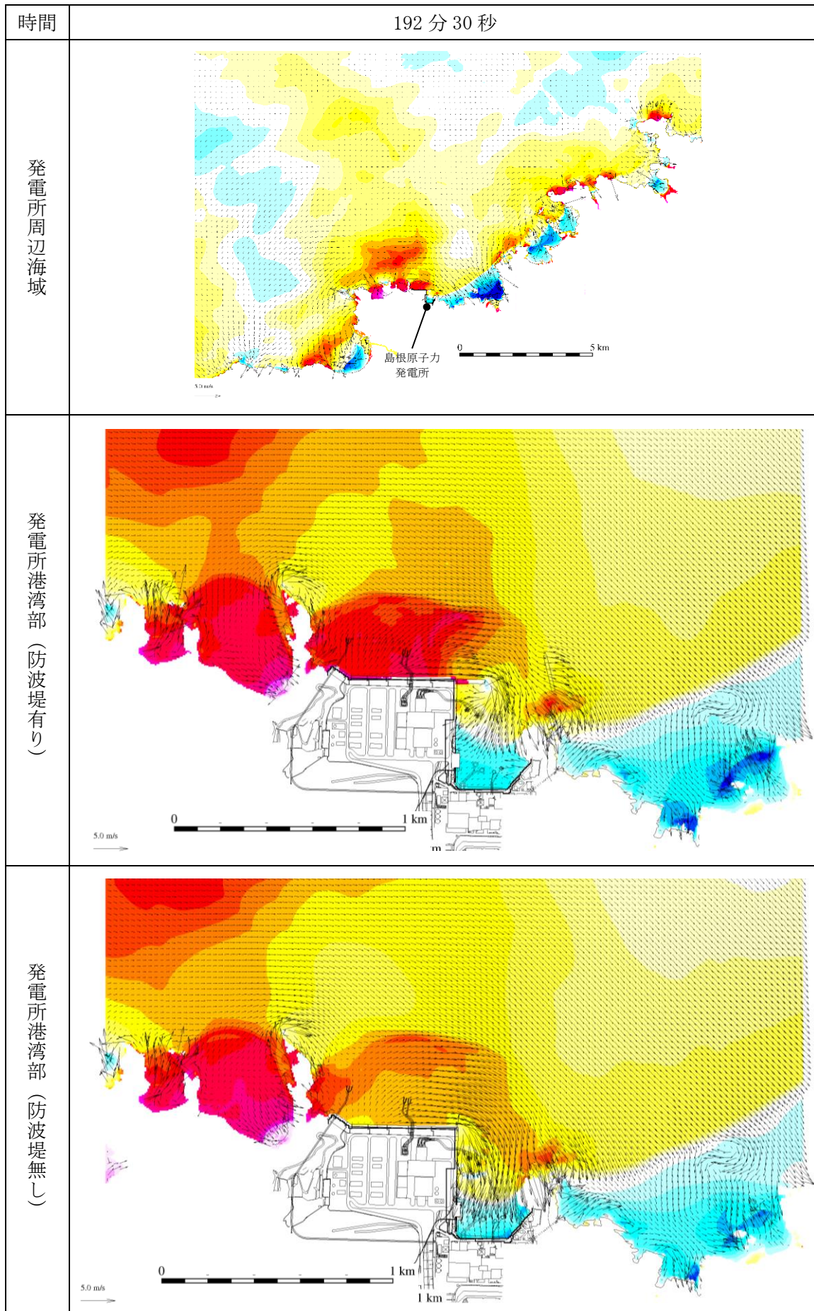
図 1-186 基準津波 1 の水位変動・流向ベクトル
