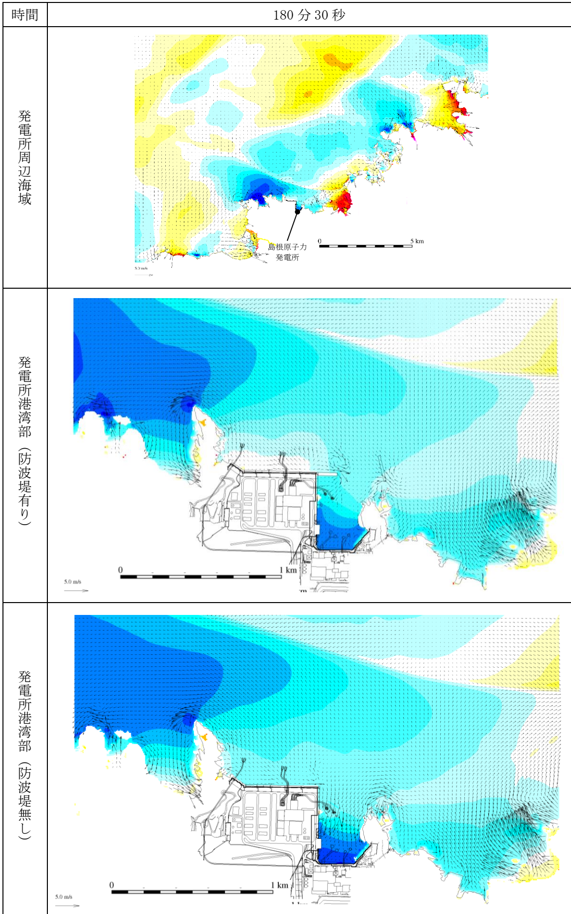
図 1-162 基準津波 1 の水位変動・流向ベクトル
