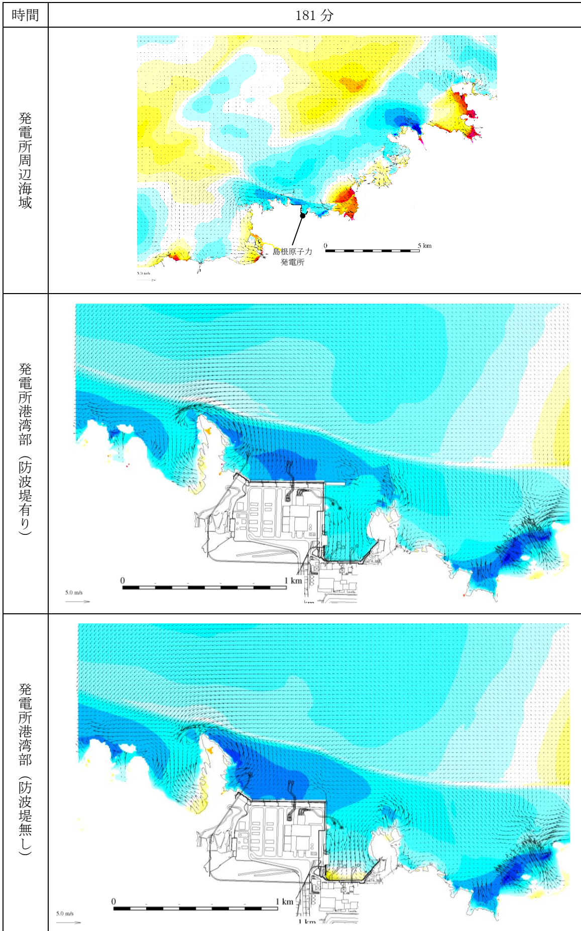
図 1-163 基準津波 1 の水位変動・流向ベクトル
