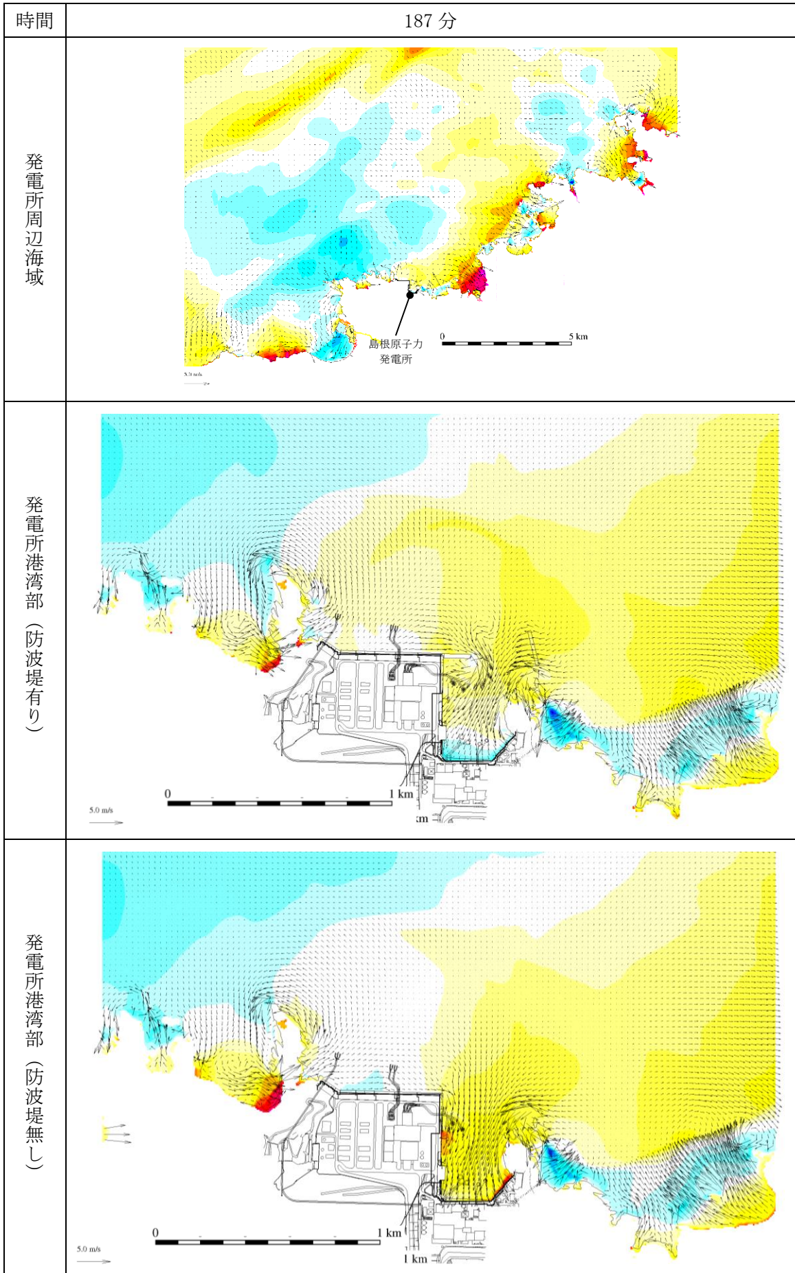
図 1-175 基準津波 1 の水位変動・流向ベクトル
