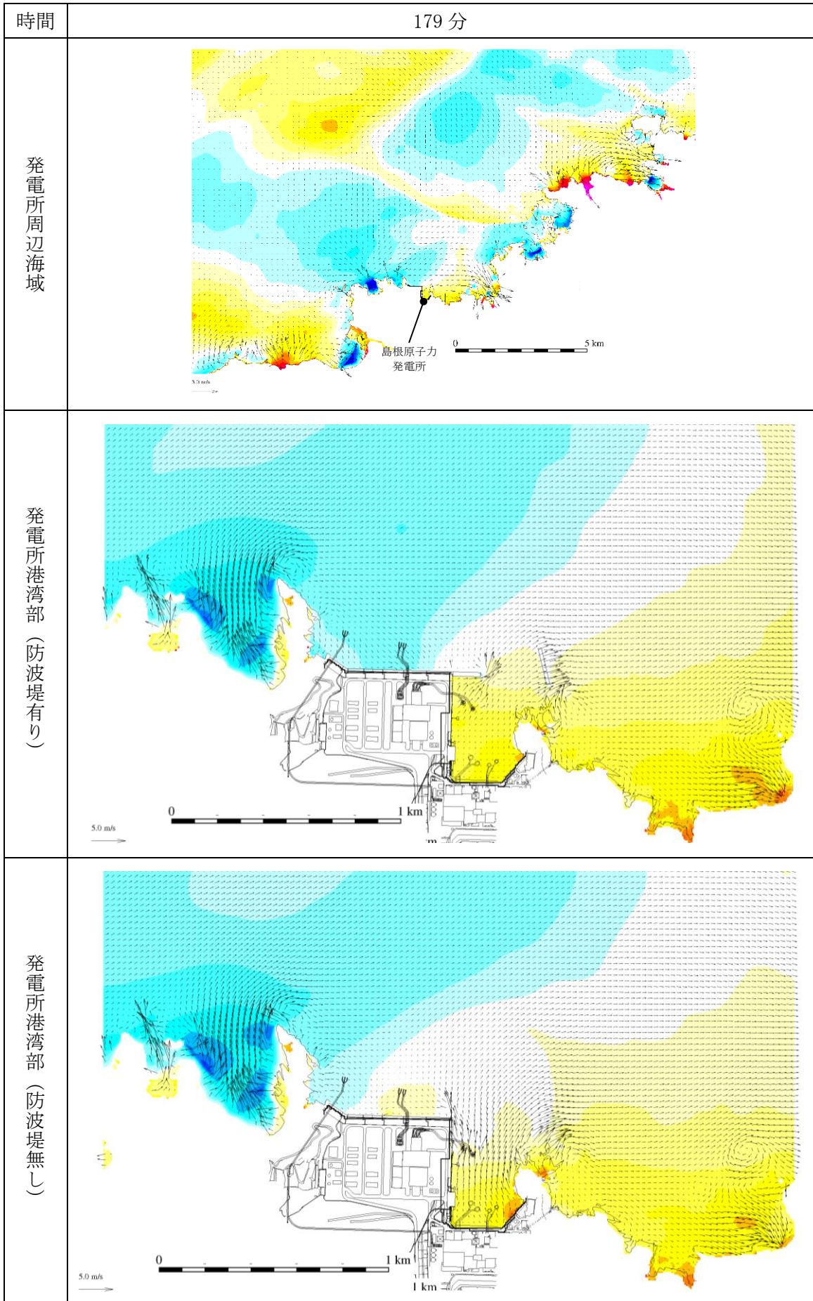
図 1-159 基準津波 1 の水位変動・流向ベクトル
