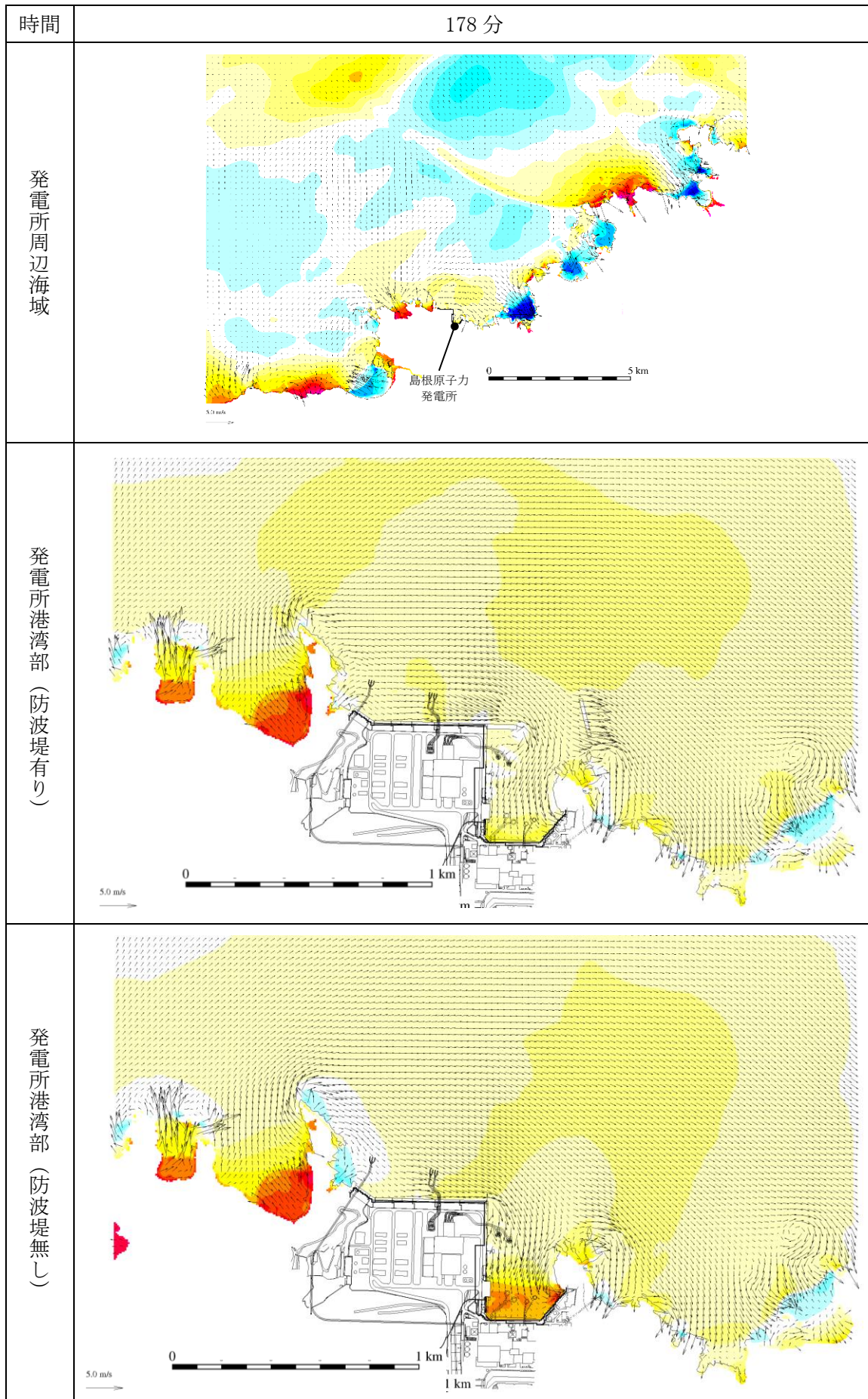
図 1-157 基準津波 1 の水位変動・流向ベクトル
