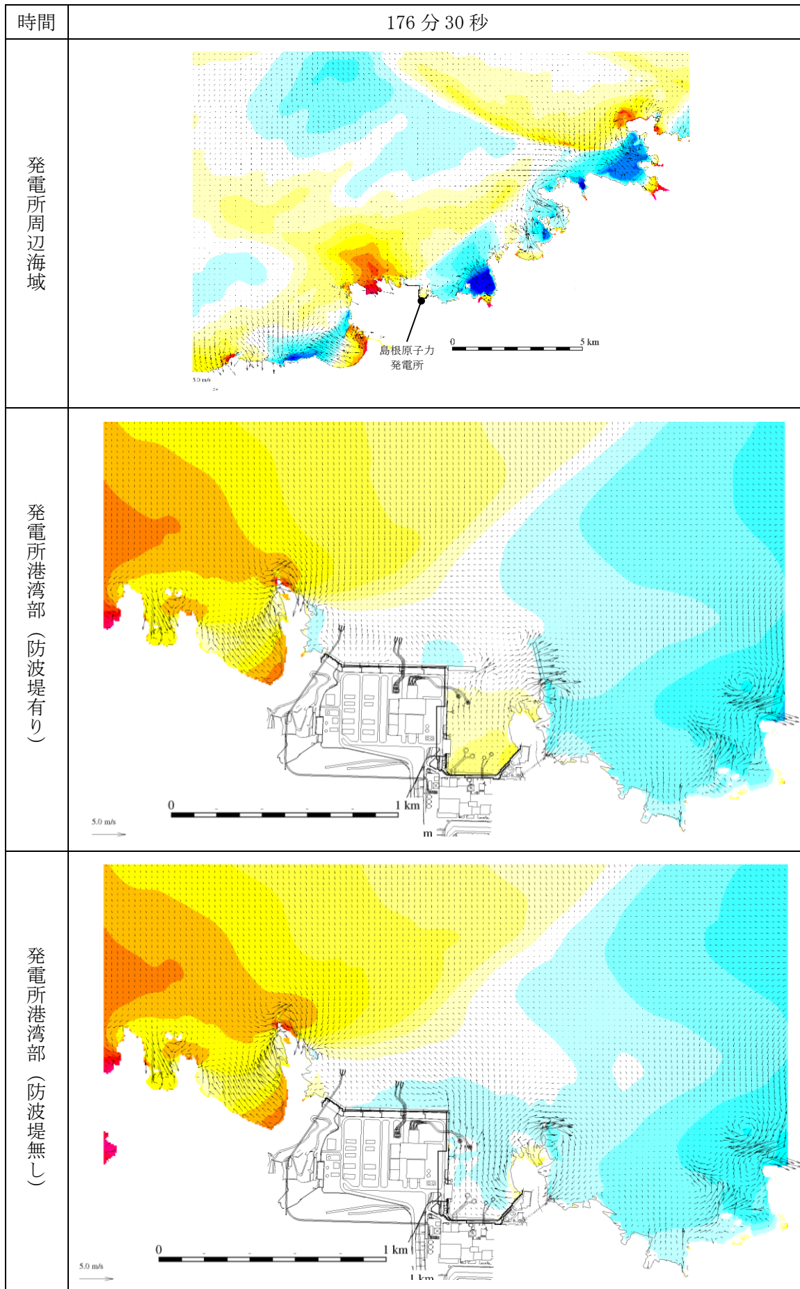
図 1-154 基準津波 1 の水位変動・流向ベクトル
