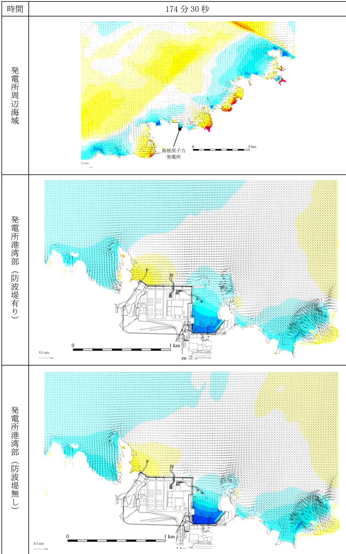
図 1-150 基準津波 1 の水位変動・流向ベクトル
