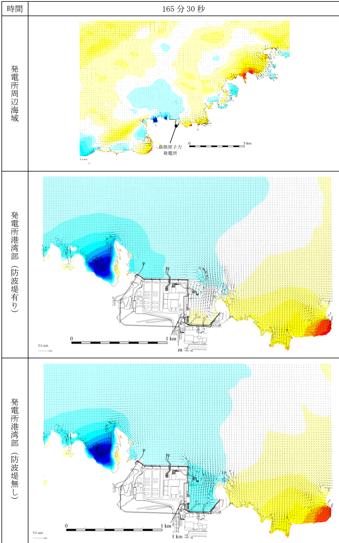
図 1-132 基準津波 1 の水位変動・流向ベクトル
