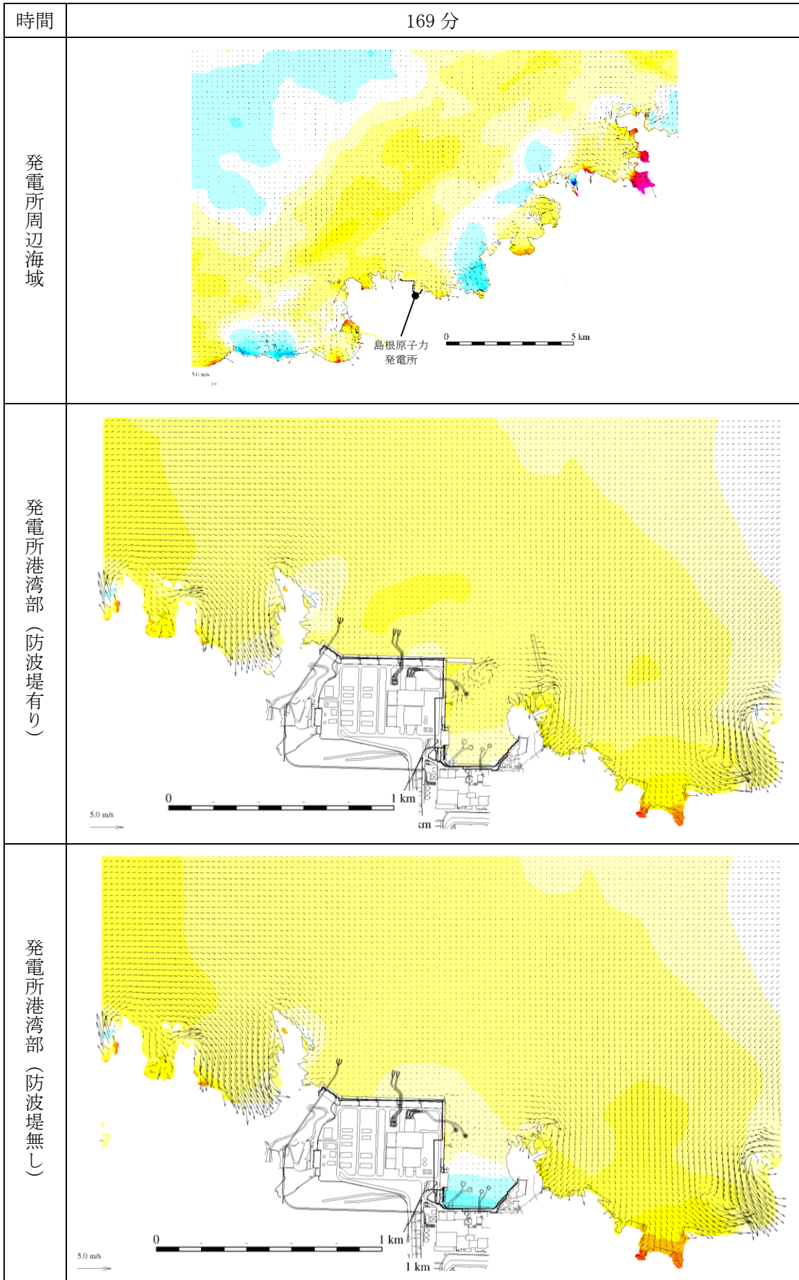
図 1-139 基準津波 1 の水位変動・流向ベクトル
