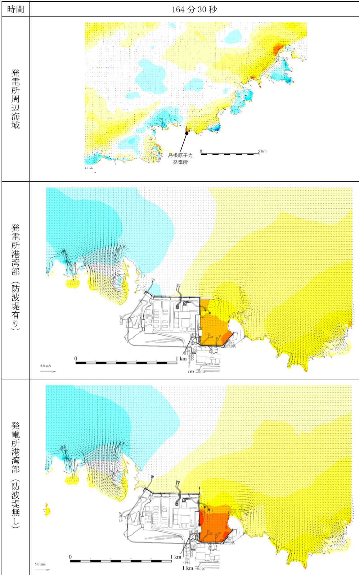
図 1-130 基準津波 1 の水位変動・流向ベクトル
