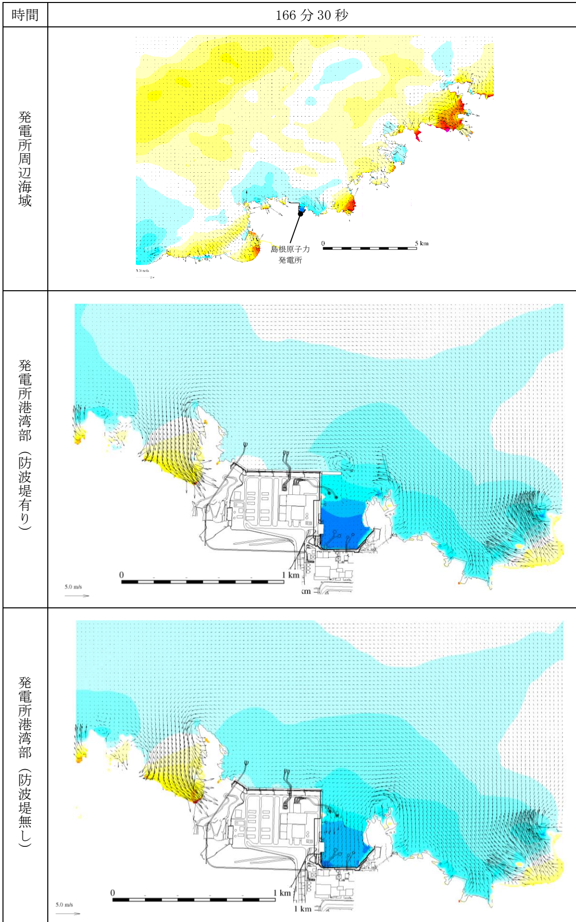
図 1-134 基準津波 1 の水位変動・流向ベクトル
