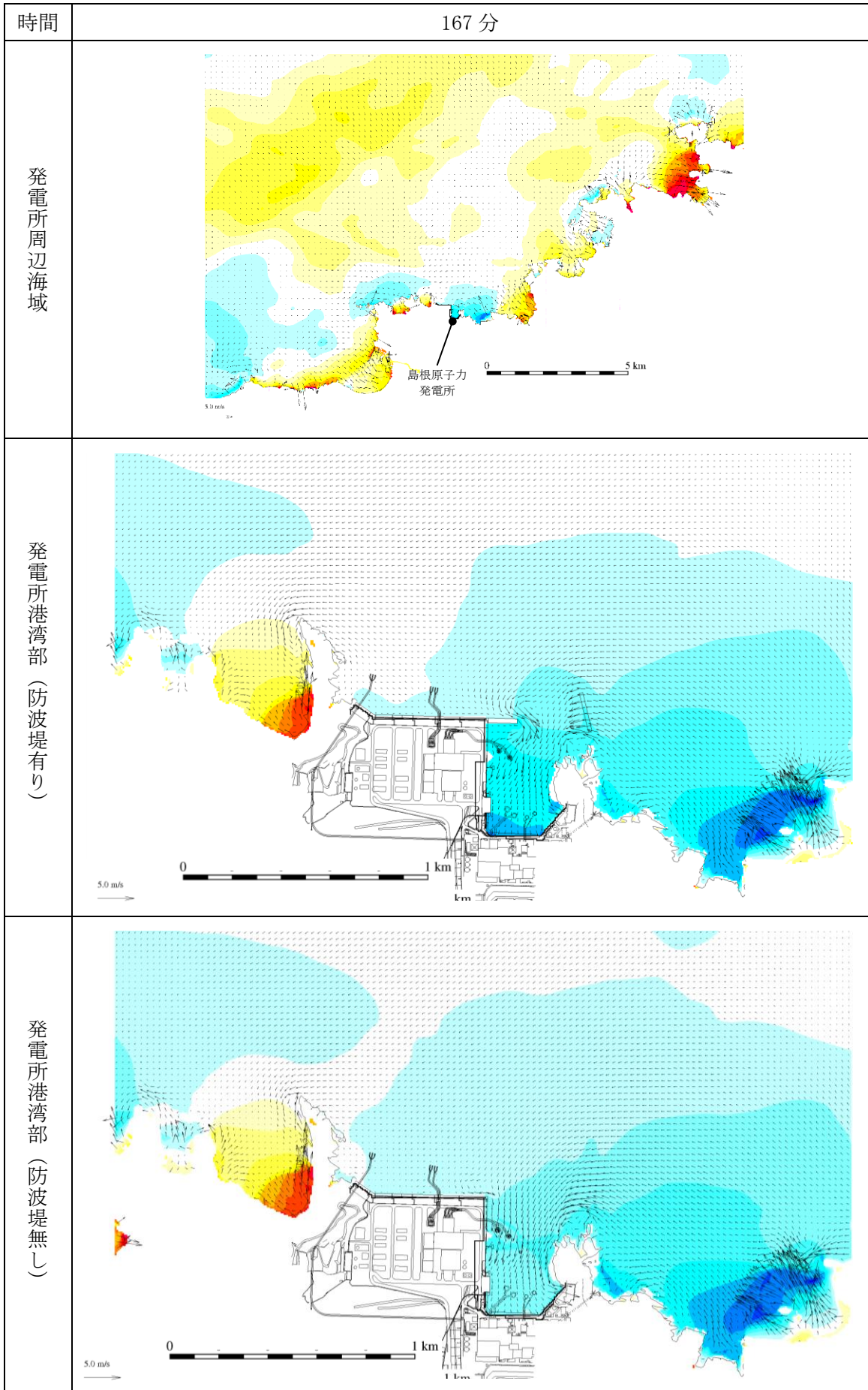
図 1-135 基準津波 1 の水位変動・流向ベクトル
