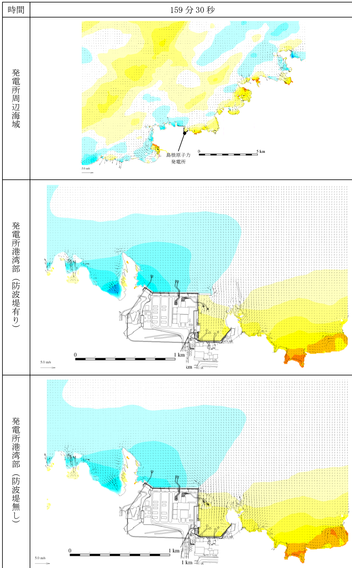
図 1-120 基準津波 1 の水位変動・流向ベクトル
