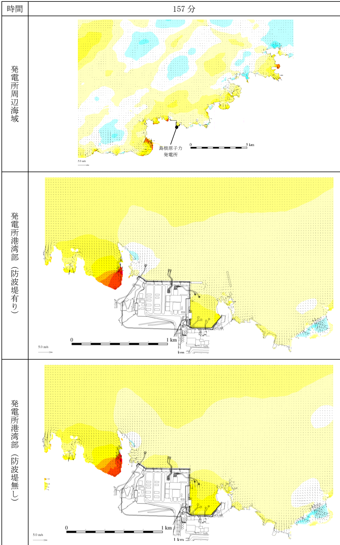
図 1-115 基準津波 1 の水位変動・流向ベクトル
