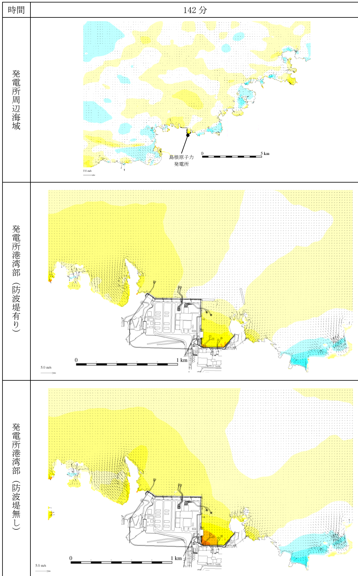
図 1-85 基準津波 1 の水位変動・流向ベクトル
