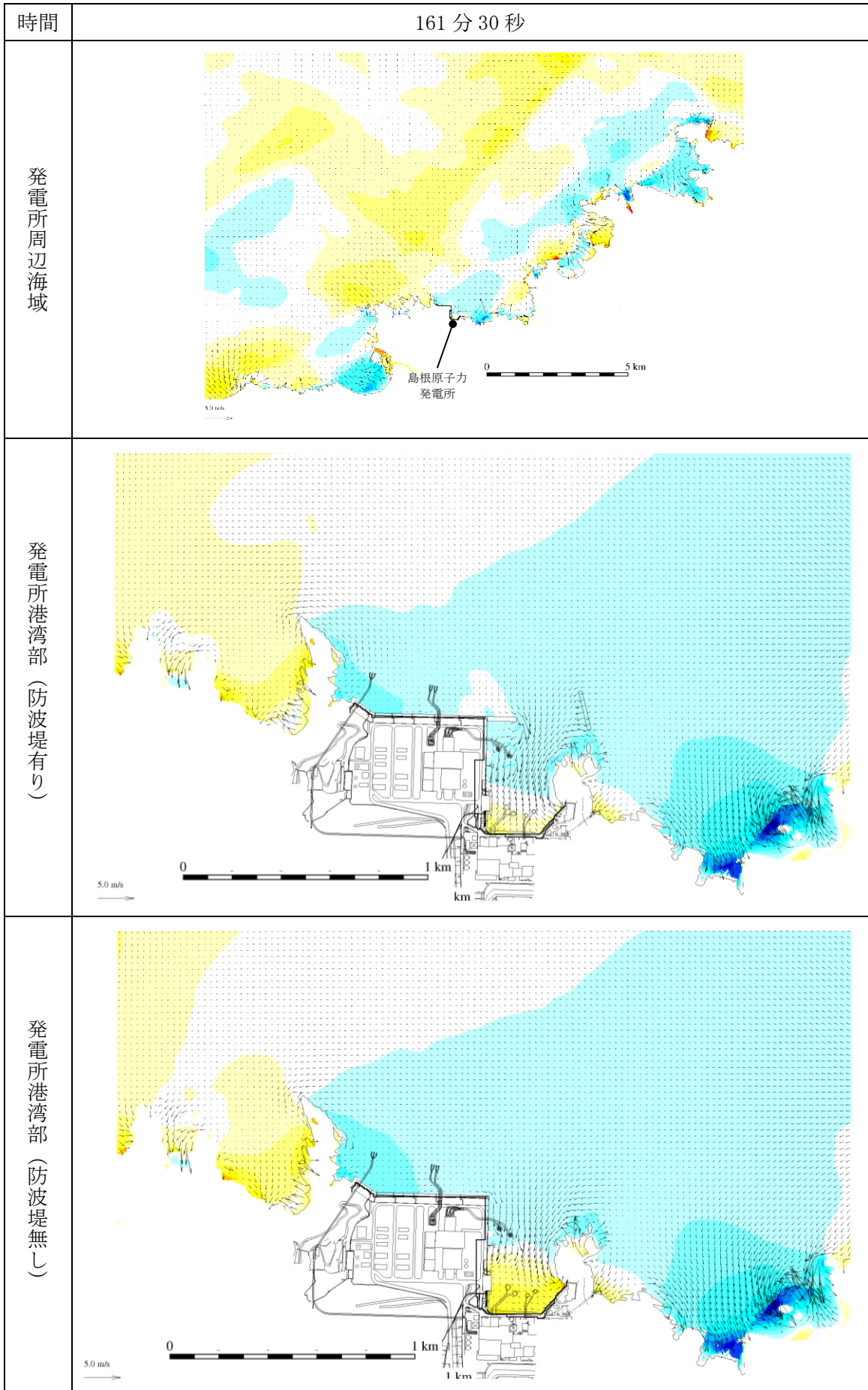
図 1-124 基準津波 1 の水位変動・流向ベクトル
