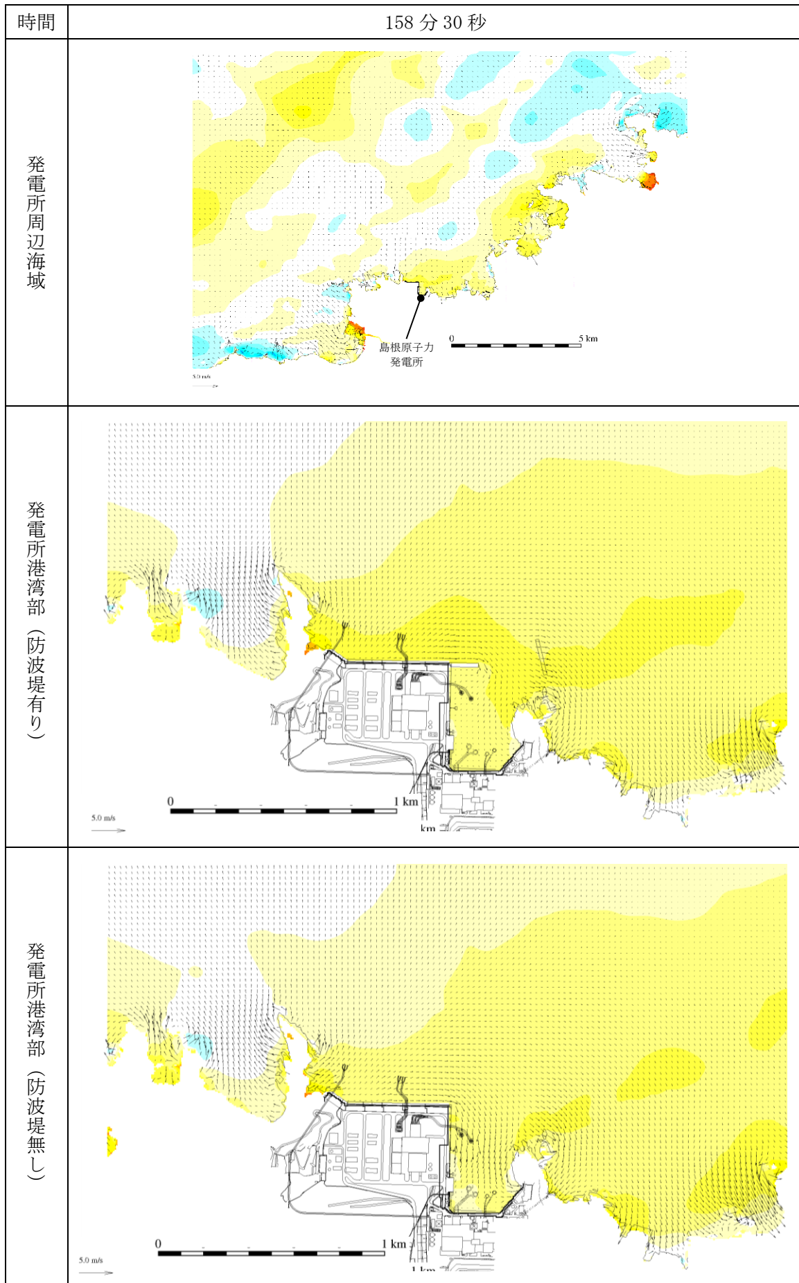
図 1-118 基準津波 1 の水位変動・流向ベクトル
