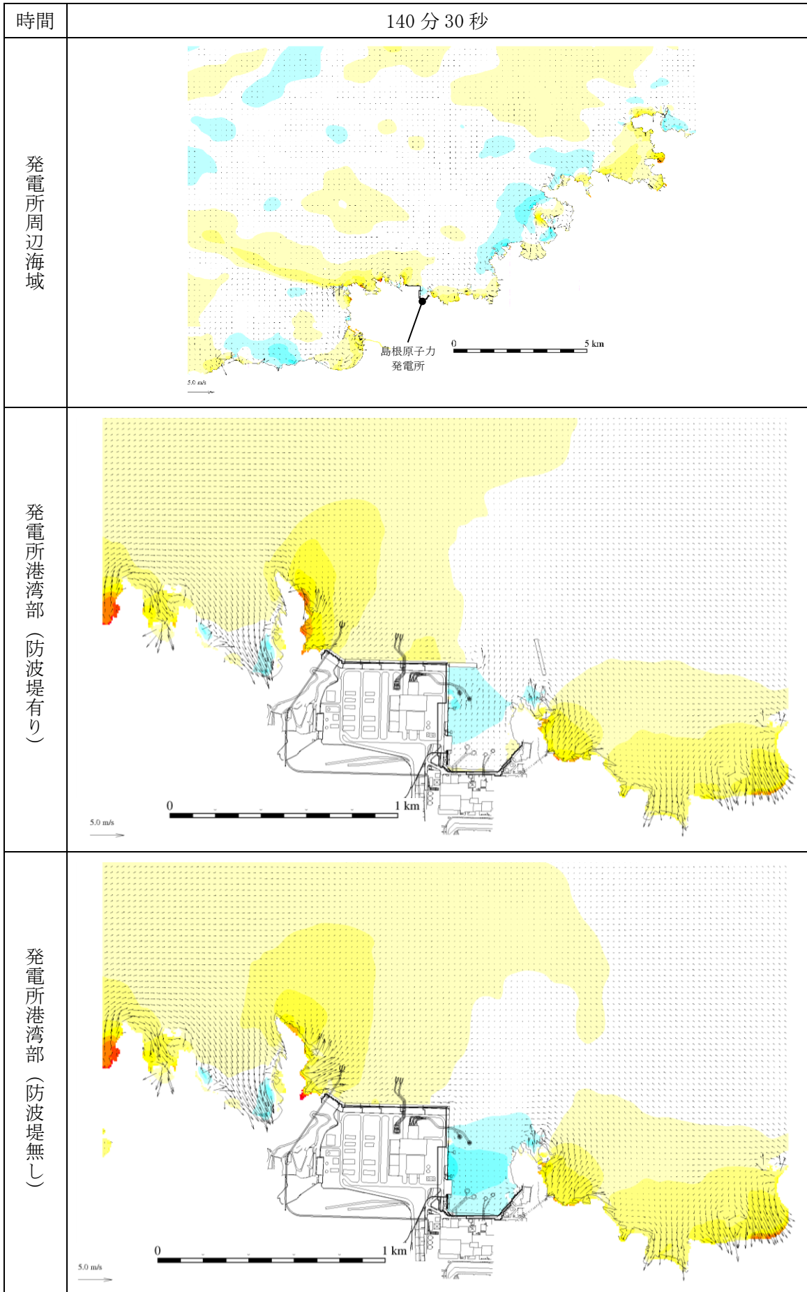
図 1-82 基準津波 1 の水位変動・流向ベクトル
