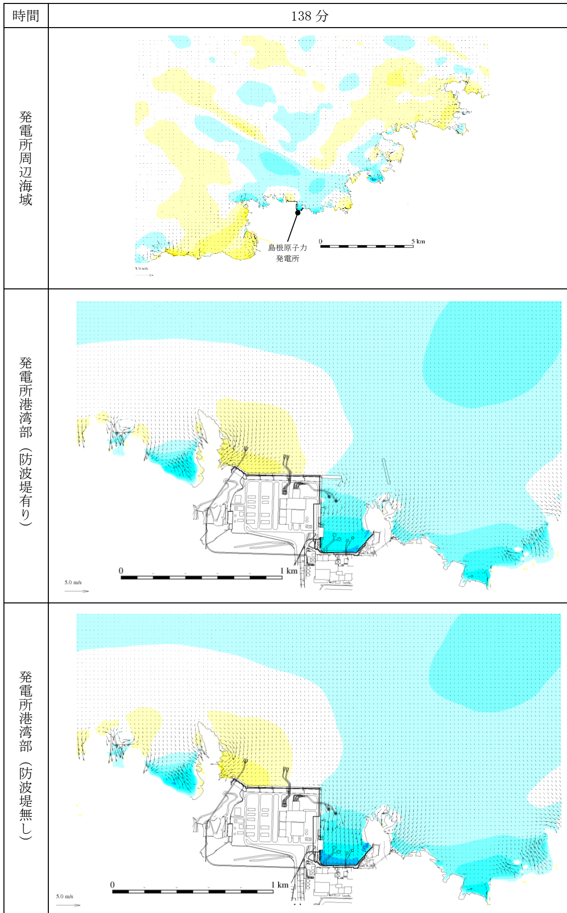
図 1-77 基準津波 1 の水位変動・流向ベクトル
