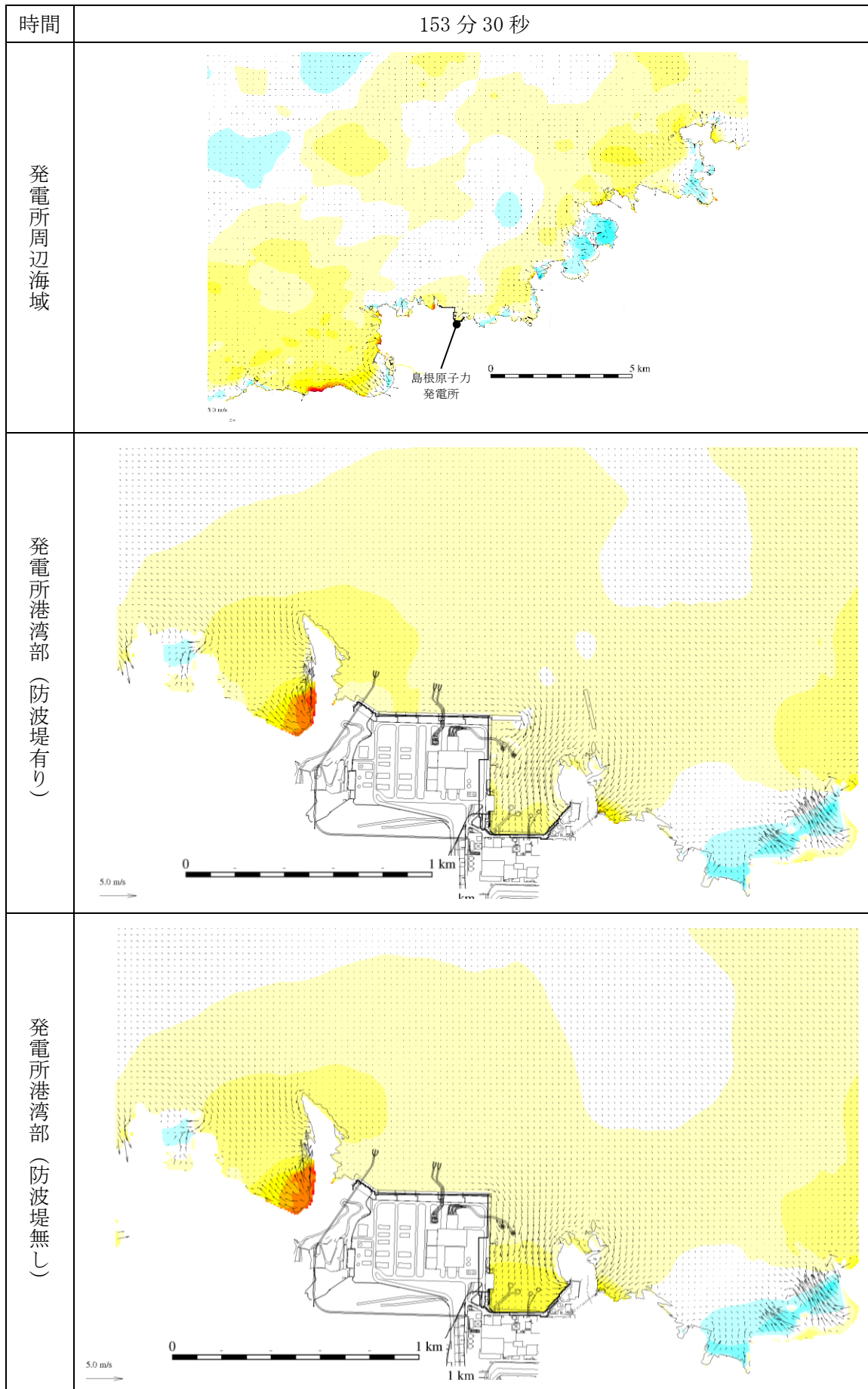
図 1-108 基準津波 1 の水位変動・流向ベクトル
