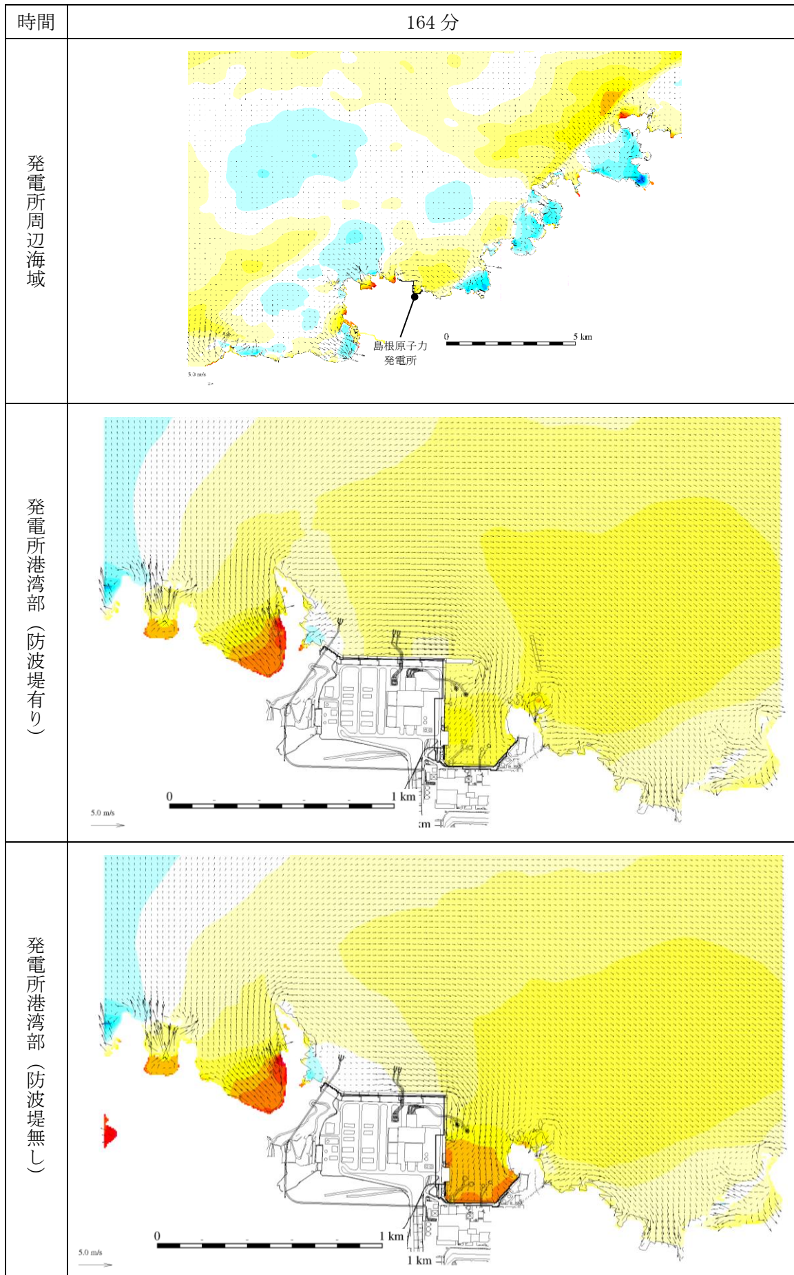
図 1-129 基準津波 1 の水位変動・流向ベクトル
