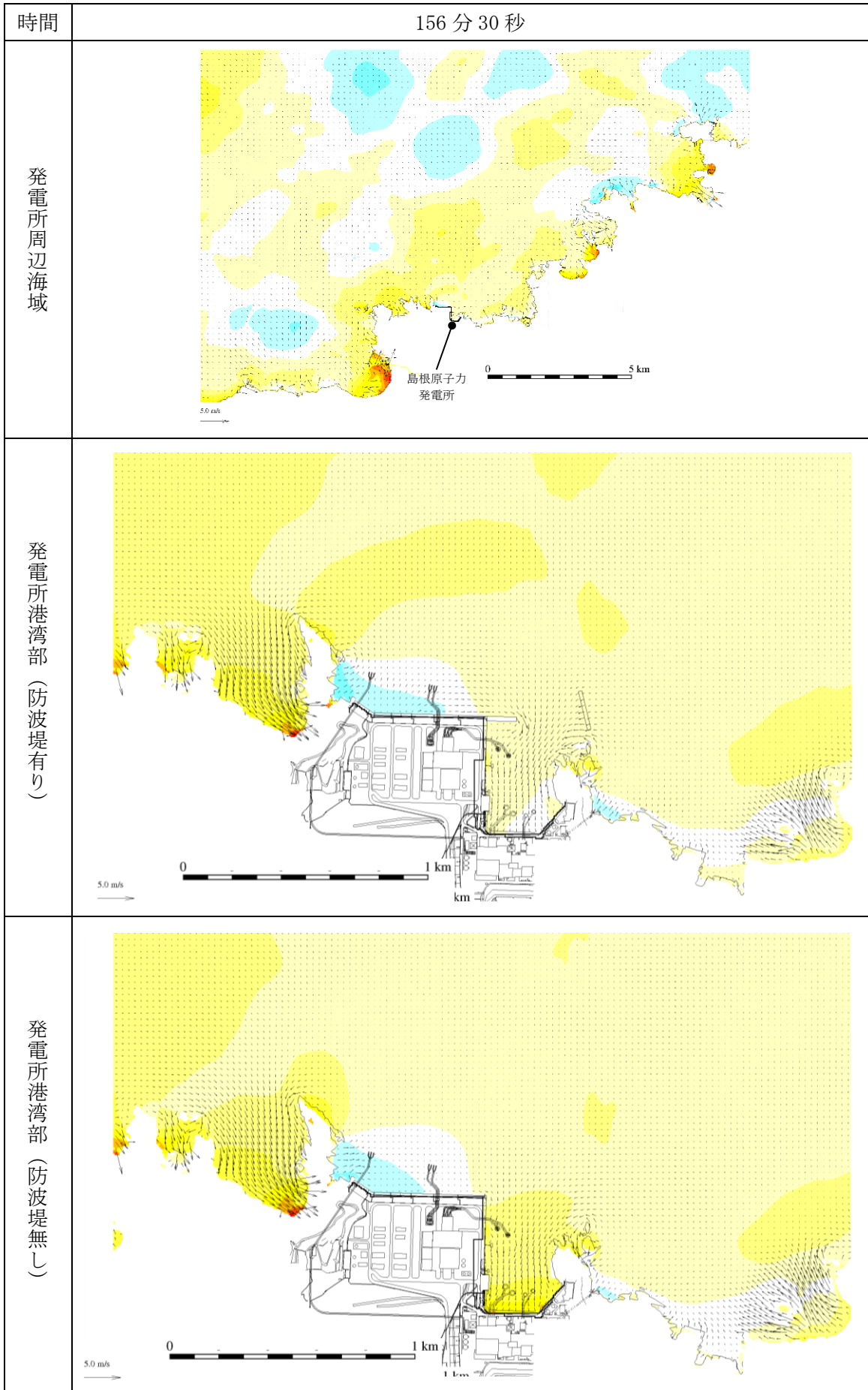
図 1-114 基準津波 1 の水位変動・流向ベクトル
