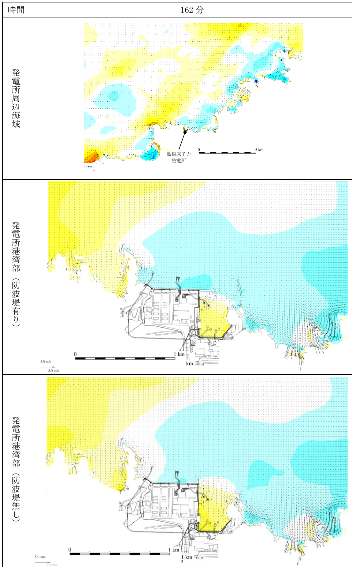
図 1-125 基準津波 1 の水位変動・流向ベクトル
