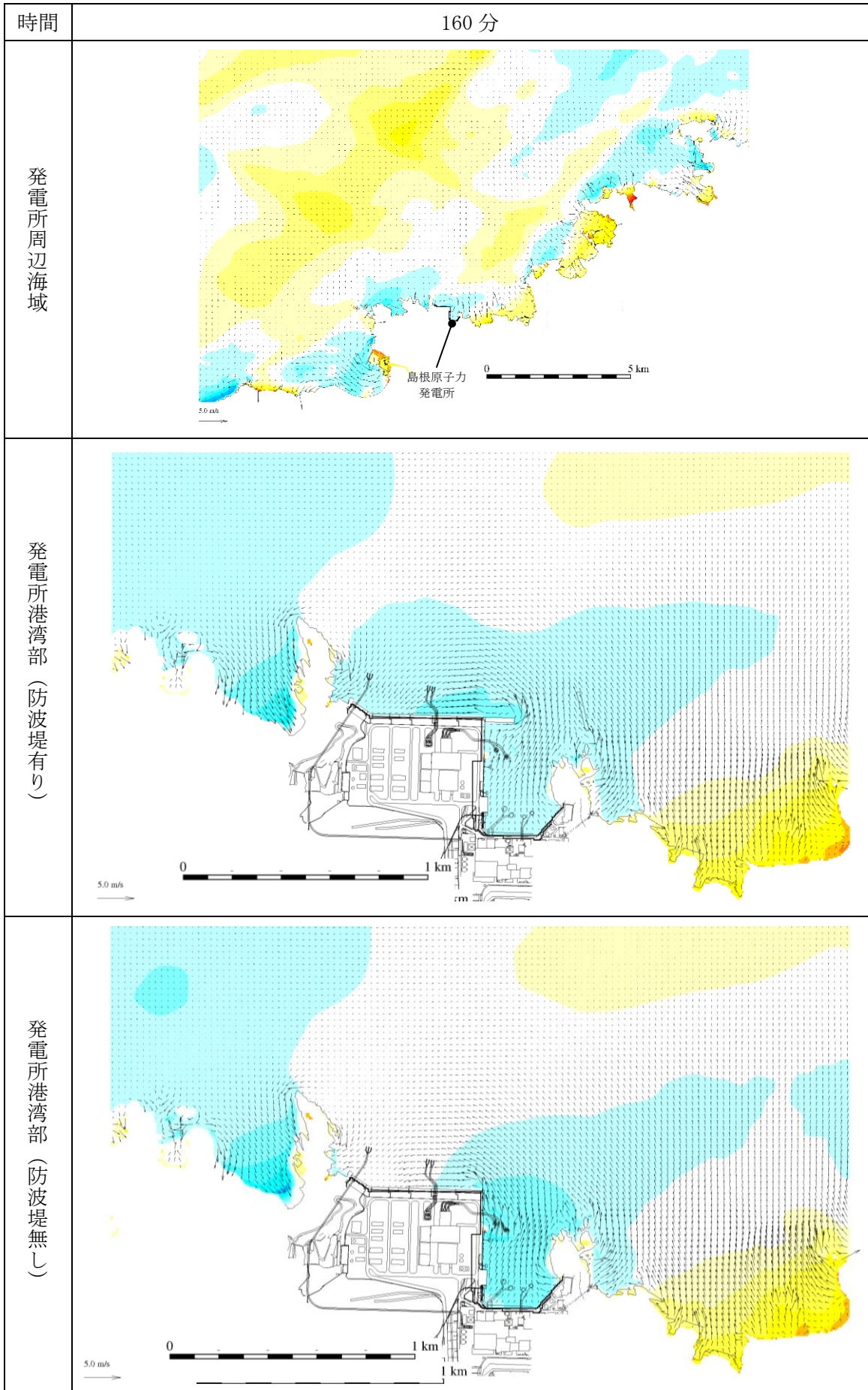
図 1-121 基準津波 1 の水位変動・流向ベクトル
