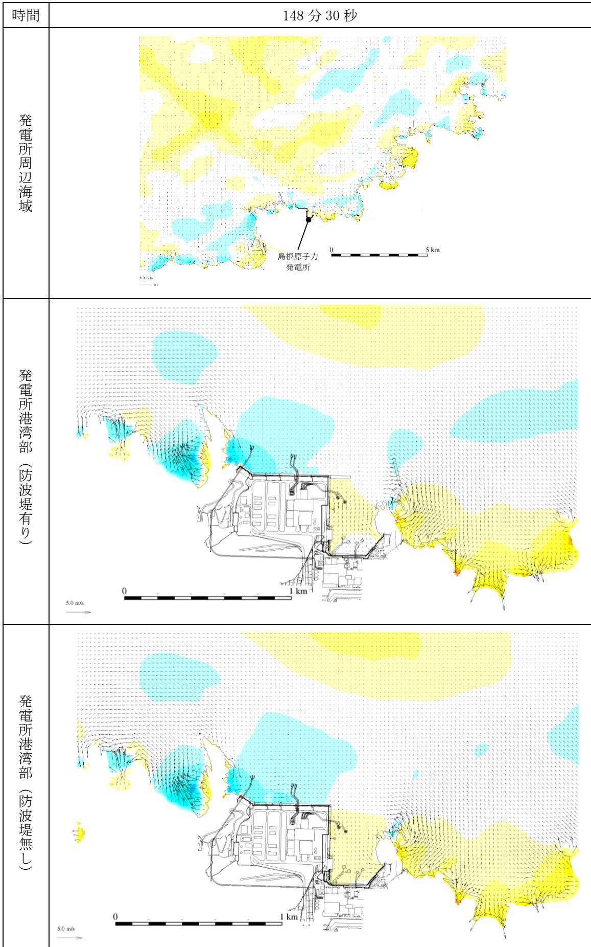
図 1-98 基準津波 1 の水位変動・流向ベクトル
