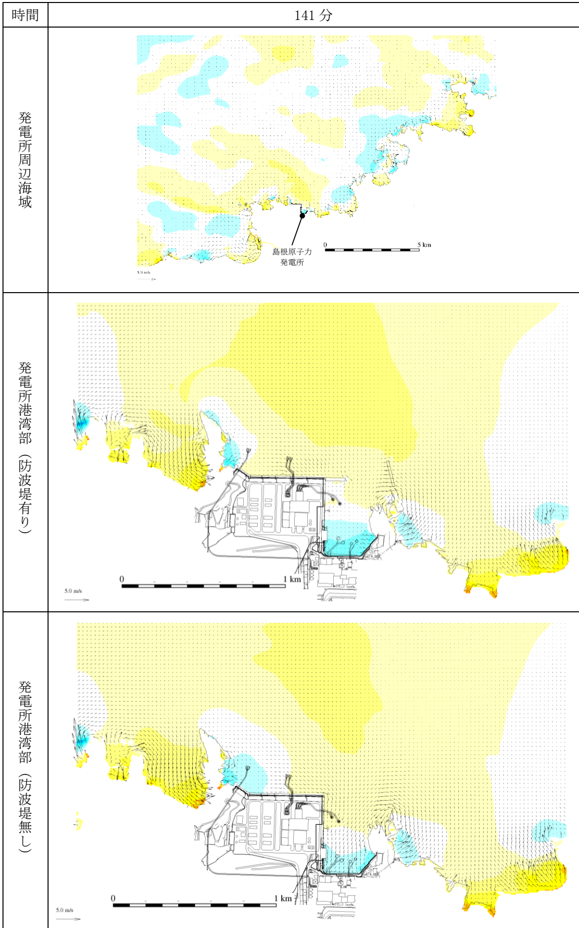
図 1-83 基準津波 1 の水位変動・流向ベクトル
