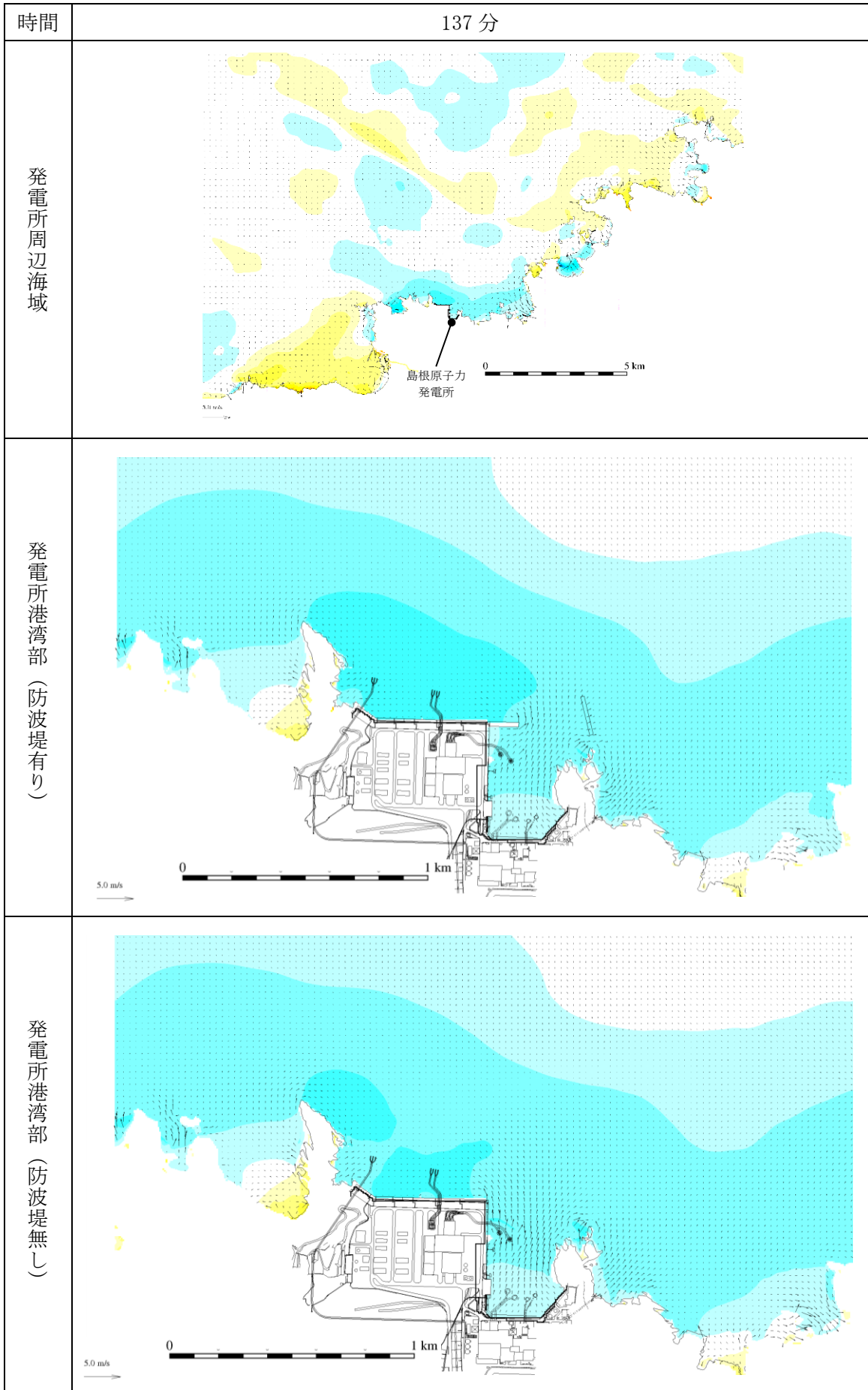
図 1-75 基準津波 1 の水位変動・流向ベクトル
