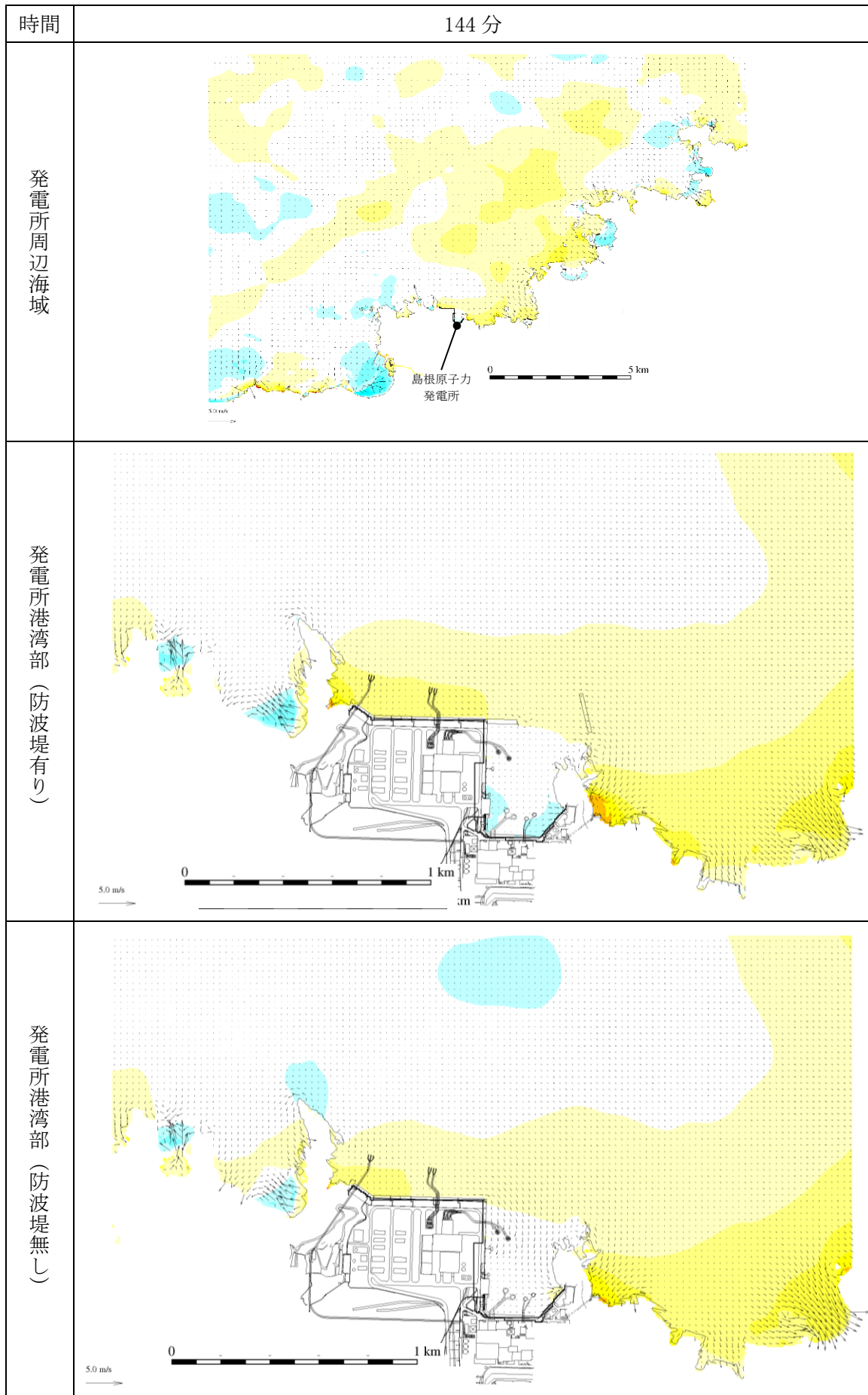
図 1-89 基準津波 1 の水位変動・流向ベクトル
