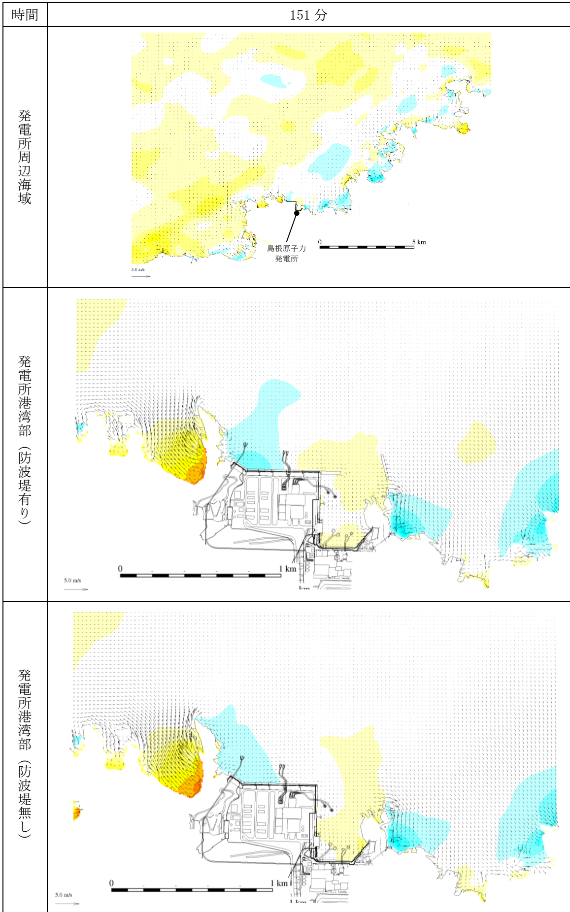
図 1-103 基準津波 1 の水位変動・流向ベクトル
