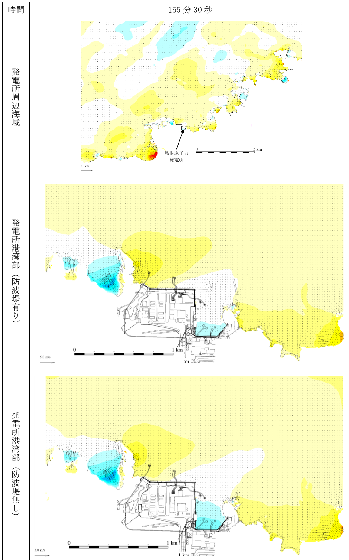
図 1-112 基準津波 1 の水位変動・流向ベクトル
