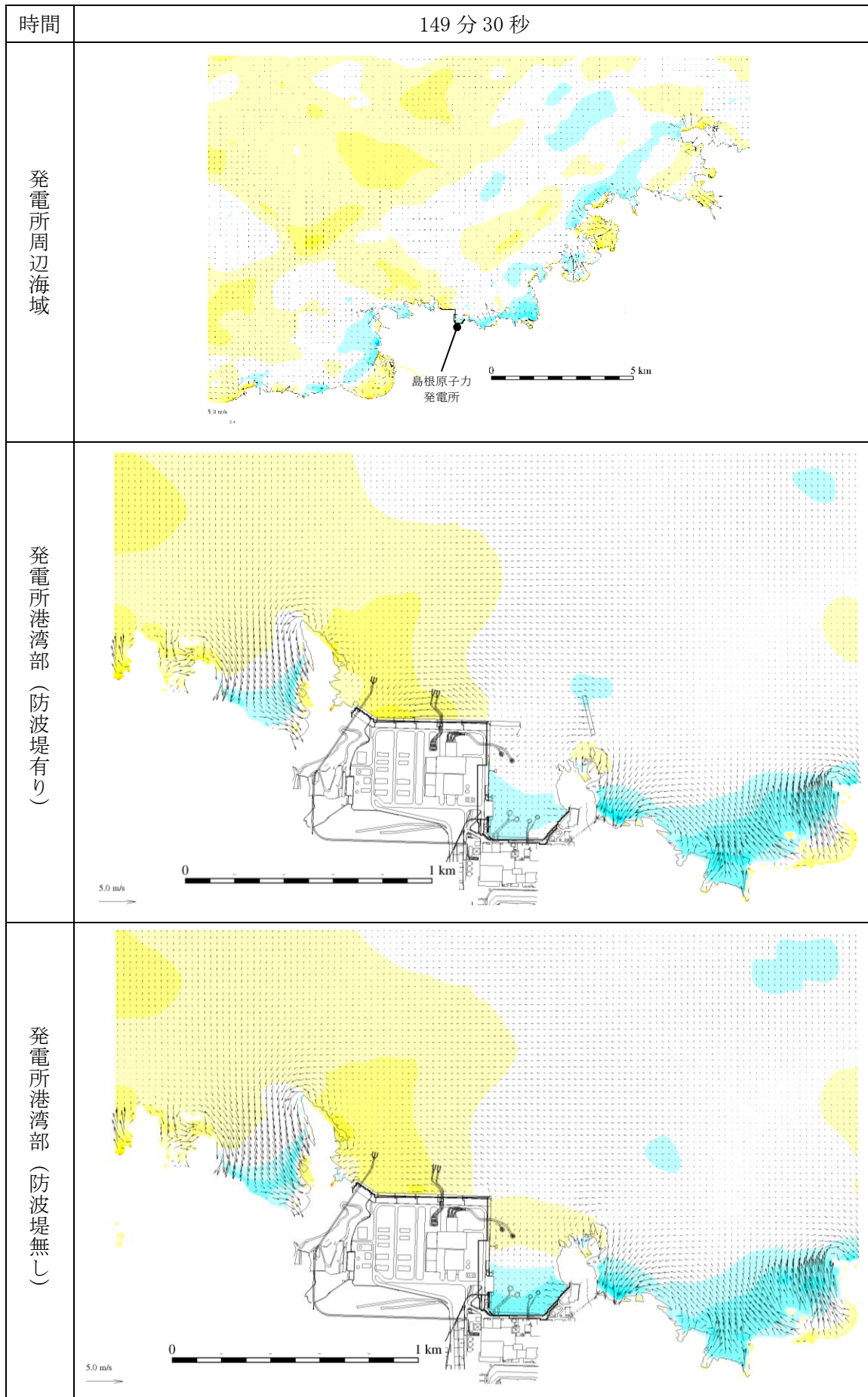
図 1-100 基準津波 1 の水位変動・流向ベクトル
