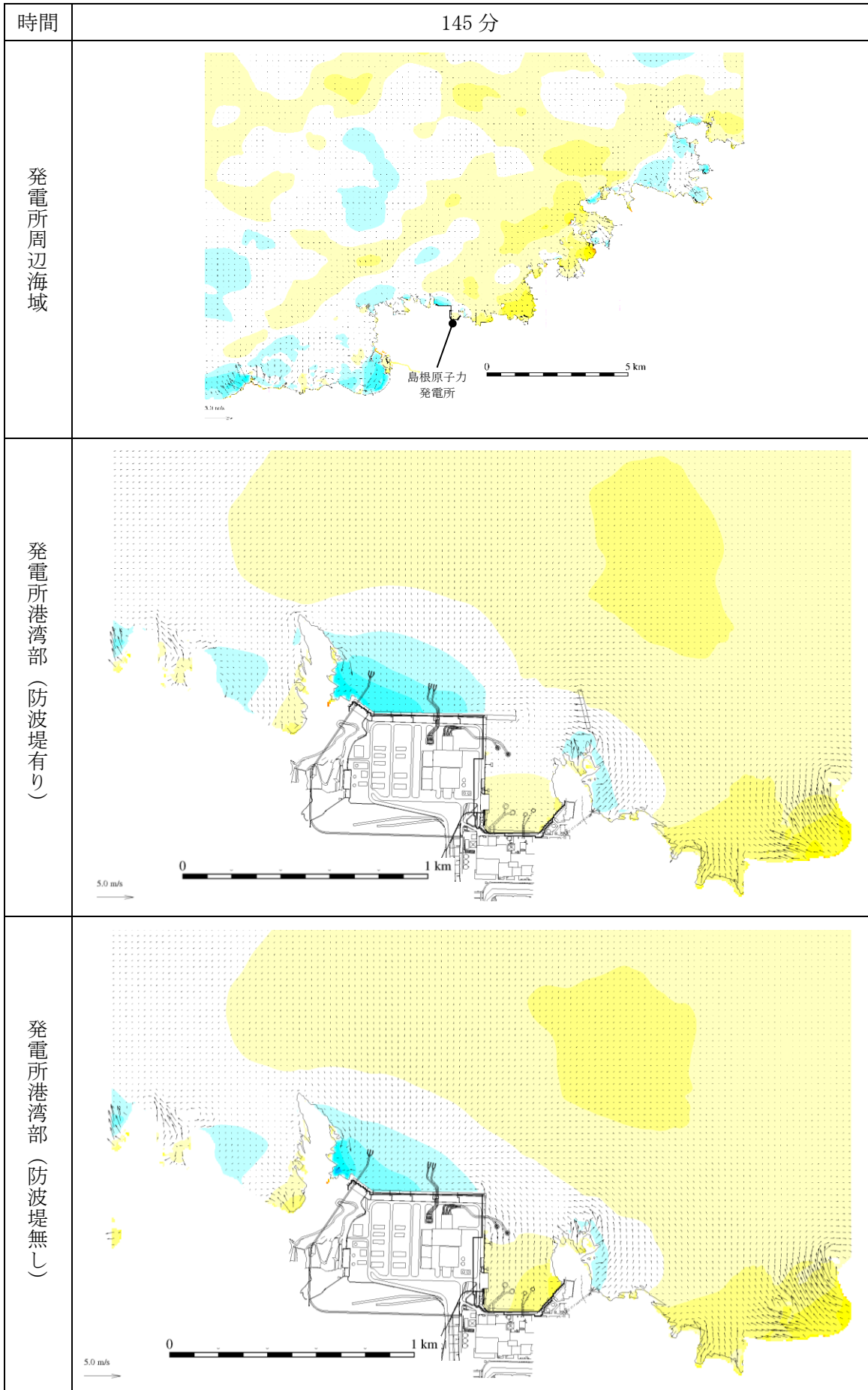
図 1-91 基準津波 1 の水位変動・流向ベクトル
