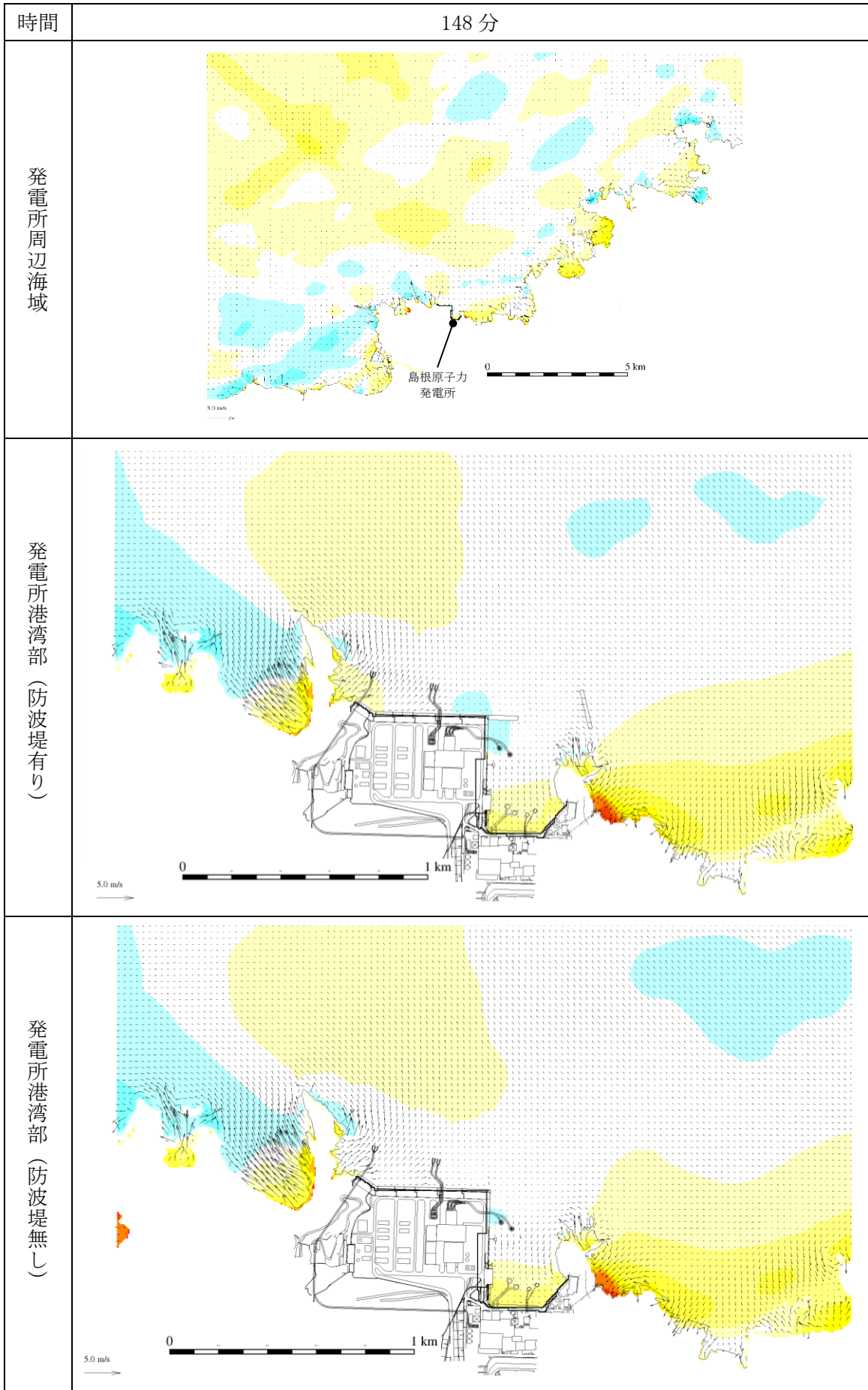
図 1-97 基準津波 1 の水位変動・流向ベクトル
