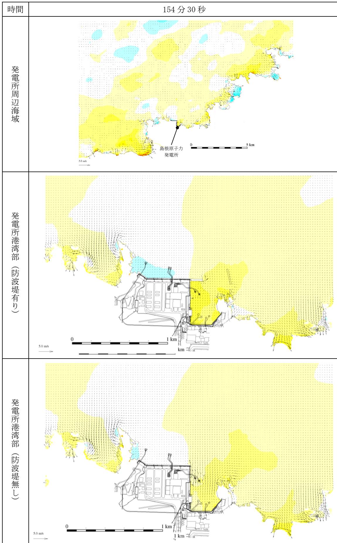
図 1-110 基準津波 1 の水位変動・流向ベクトル
