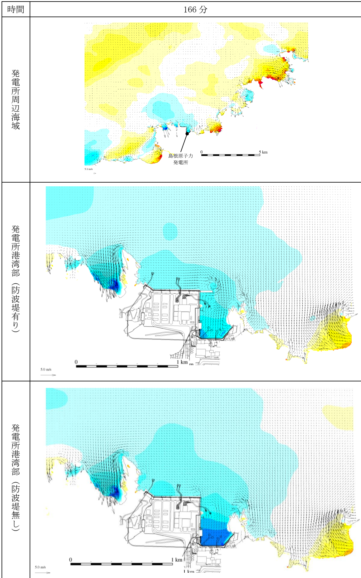
図 1-133 基準津波 1 の水位変動・流向ベクトル
