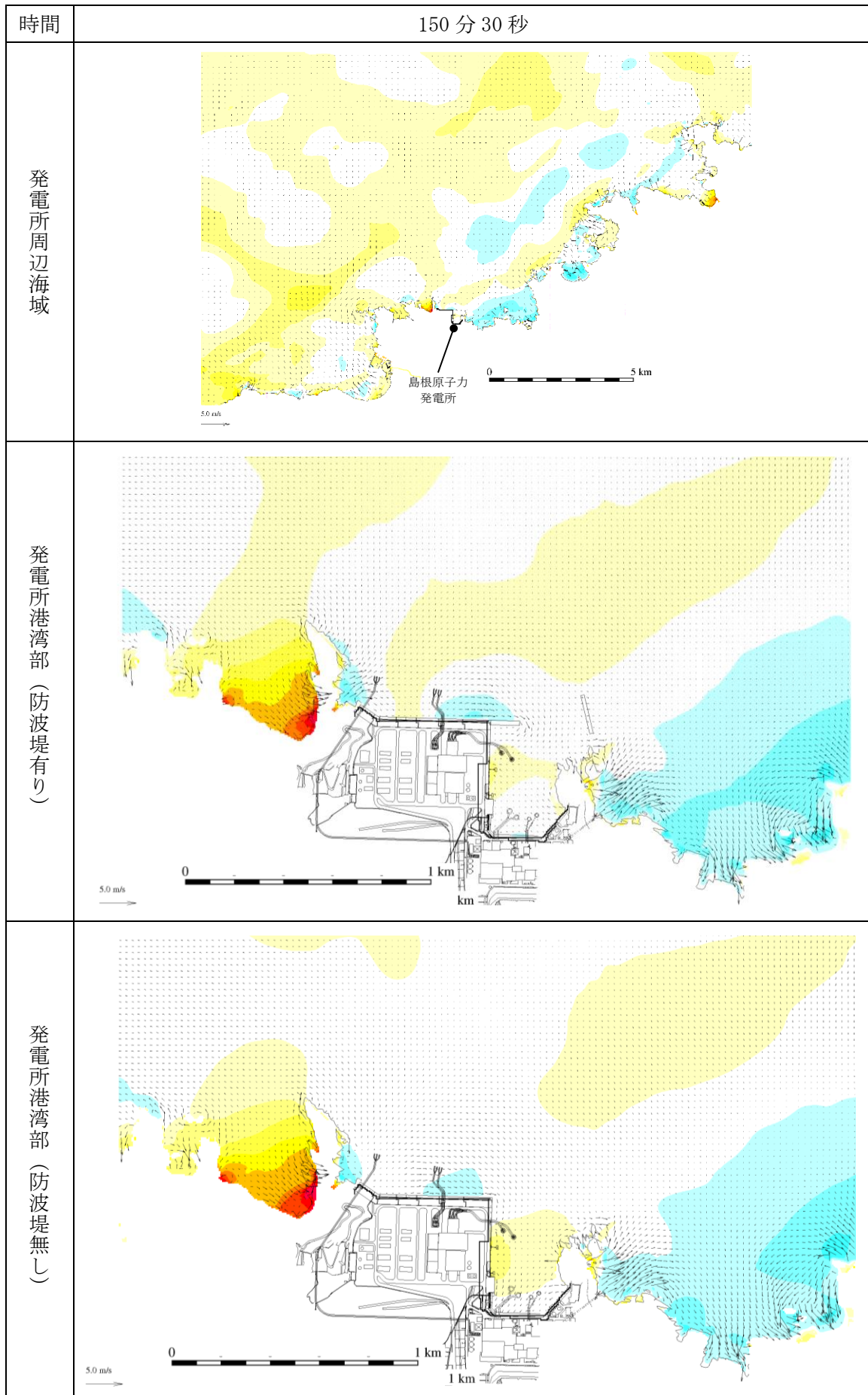
図 1-102 基準津波 1 の水位変動・流向ベクトル
