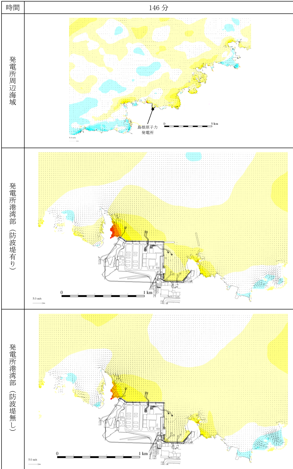
図 1-93 基準津波 1 の水位変動・流向ベクトル
