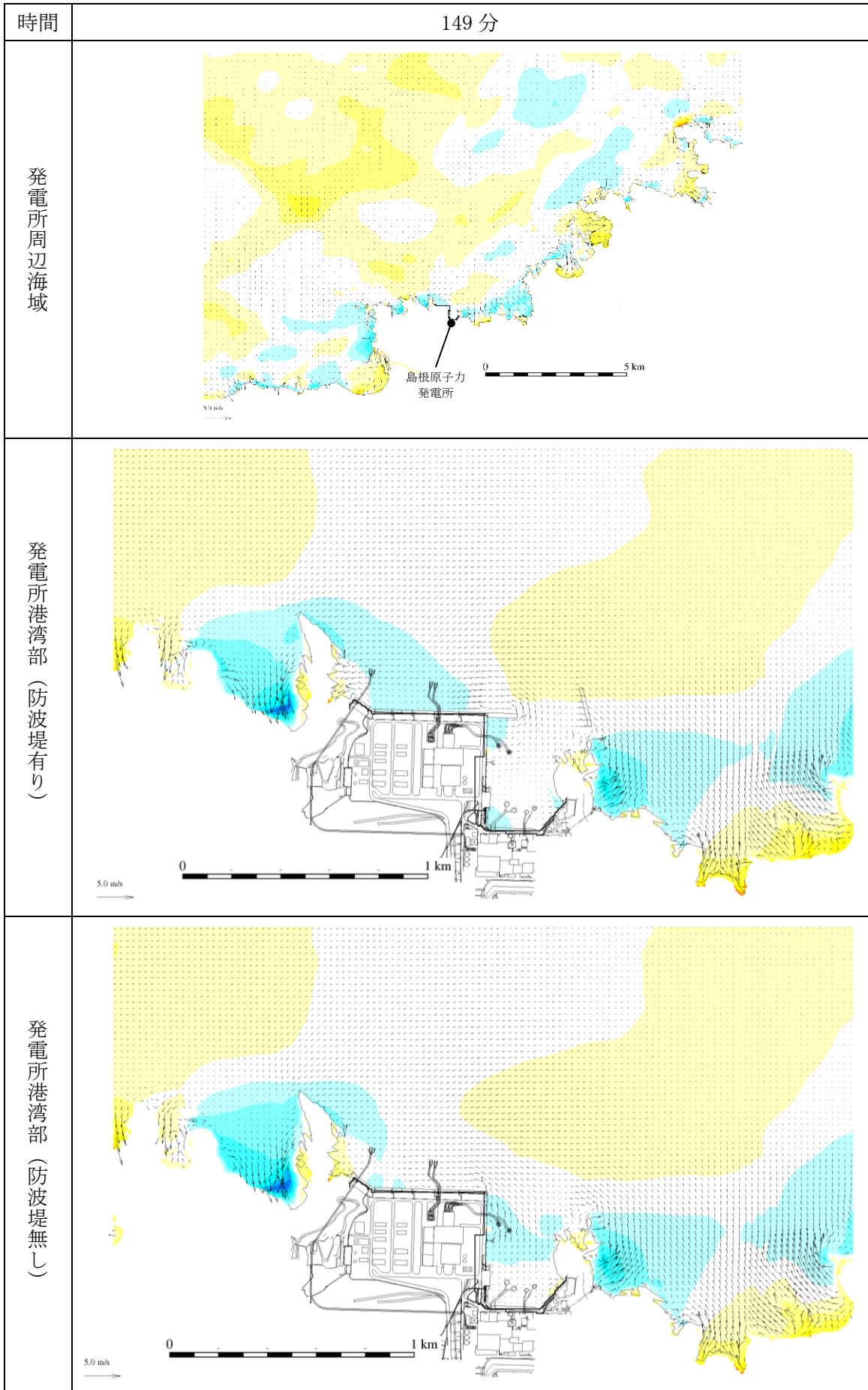
図 1-99 基準津波 1 の水位変動・流向ベクトル
