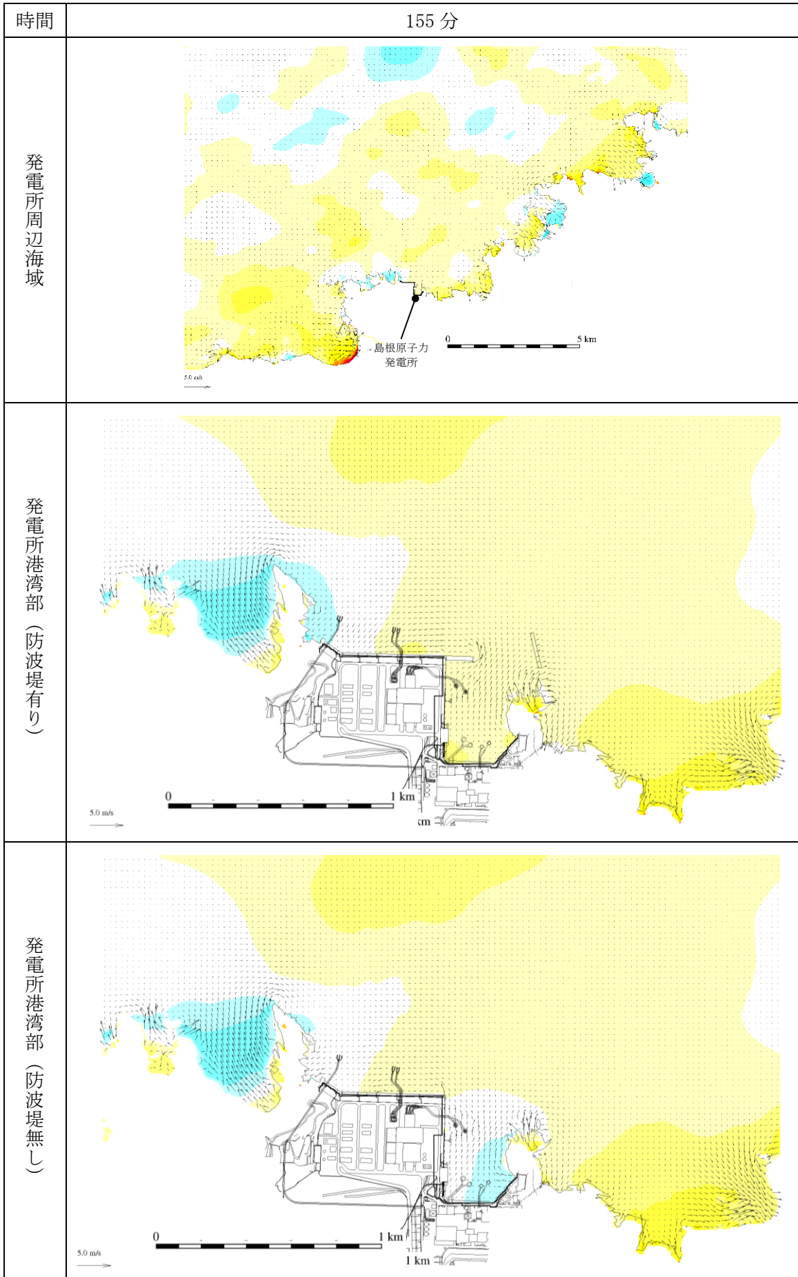
図 1-111 基準津波 1 の水位変動・流向ベクトル
