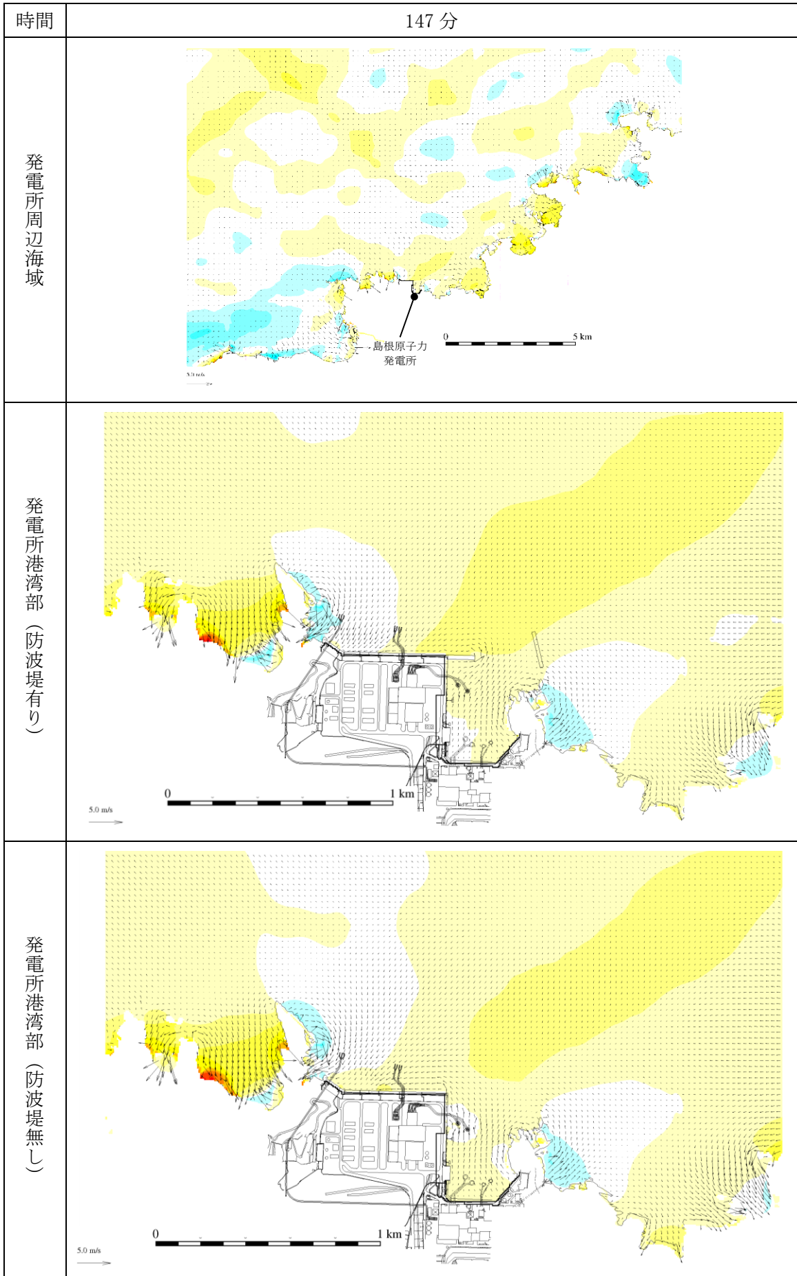
図 1-95 基準津波 1 の水位変動・流向ベクトル
