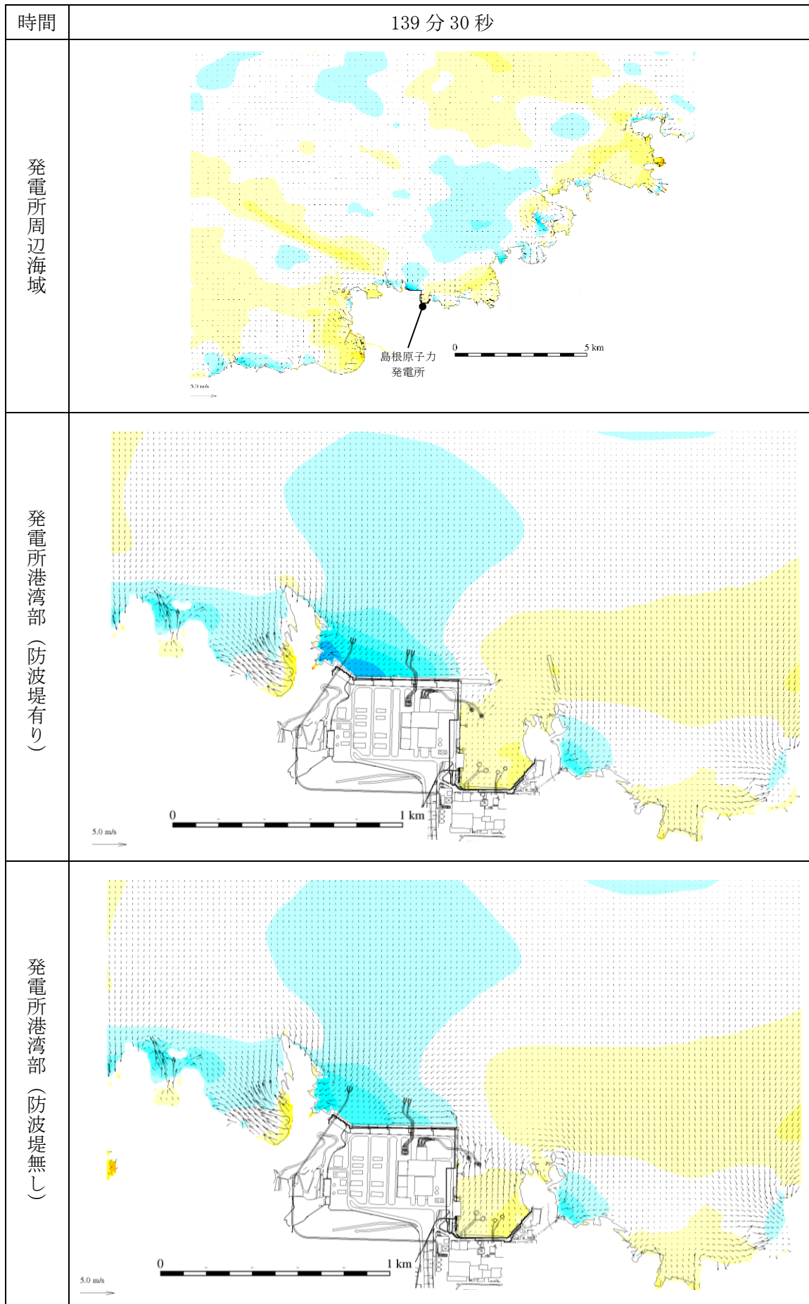
図 1-80 基準津波 1 の水位変動・流向ベクトル
