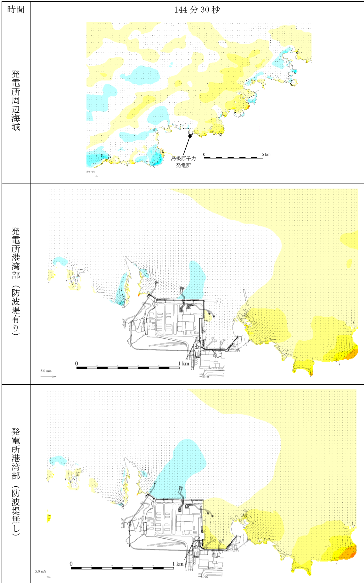
図 1-90 基準津波 1 の水位変動・流向ベクトル
