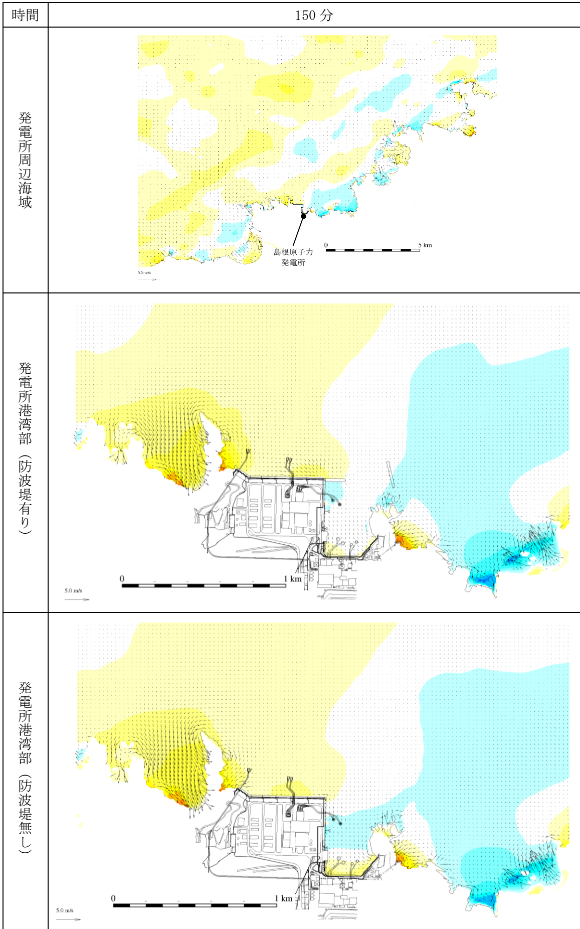
図 1-101 基準津波 1 の水位変動・流向ベクトル
