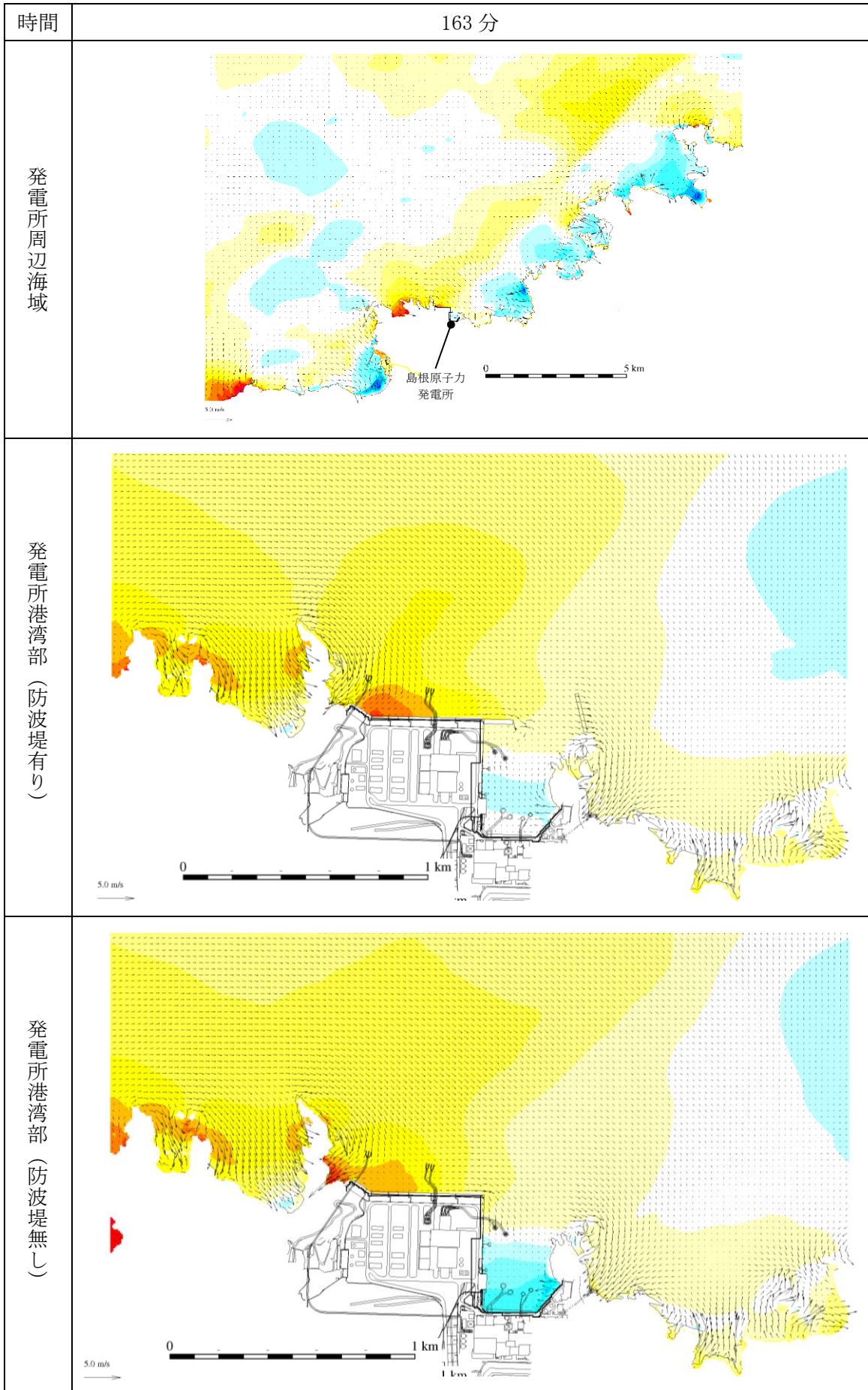
図 1-127 基準津波 1 の水位変動・流向ベクトル
