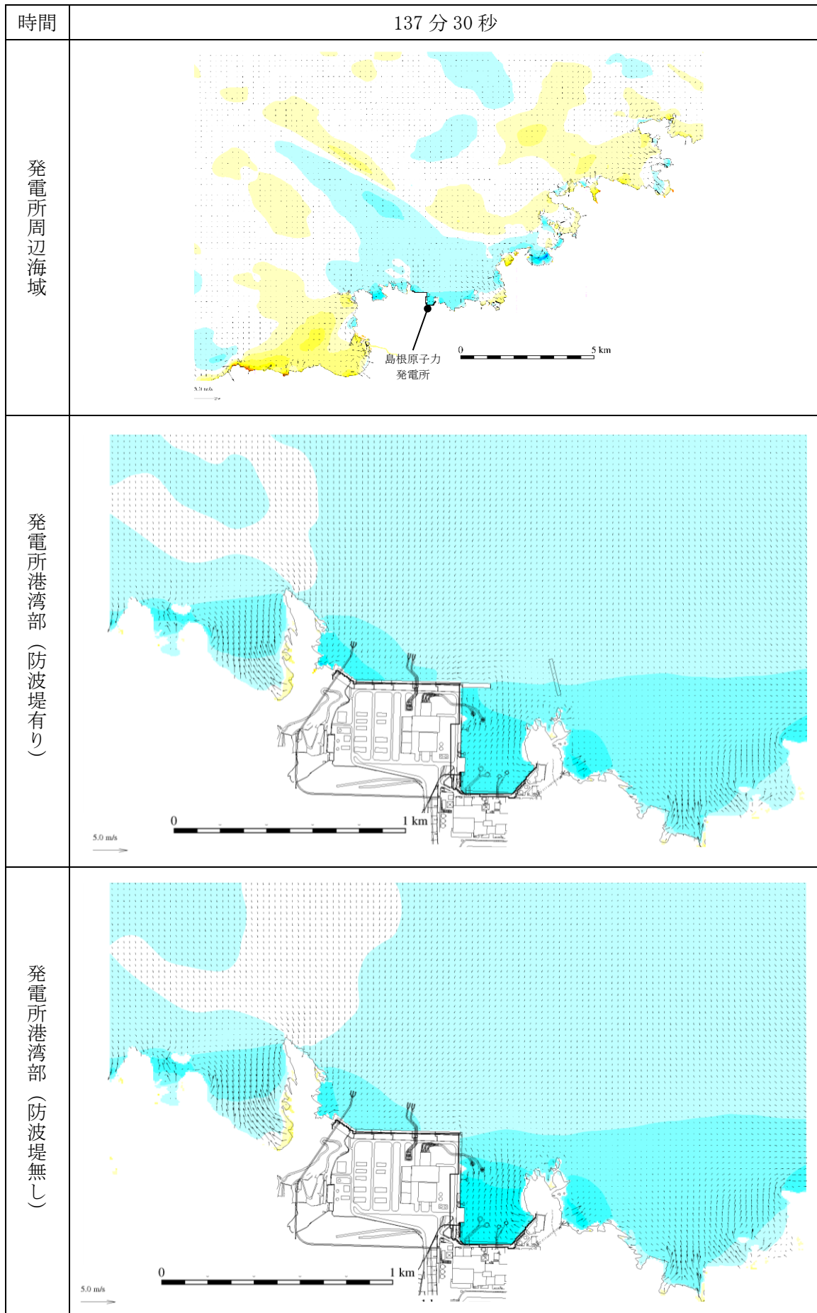
図 1-76 基準津波 1 の水位変動・流向ベクトル
