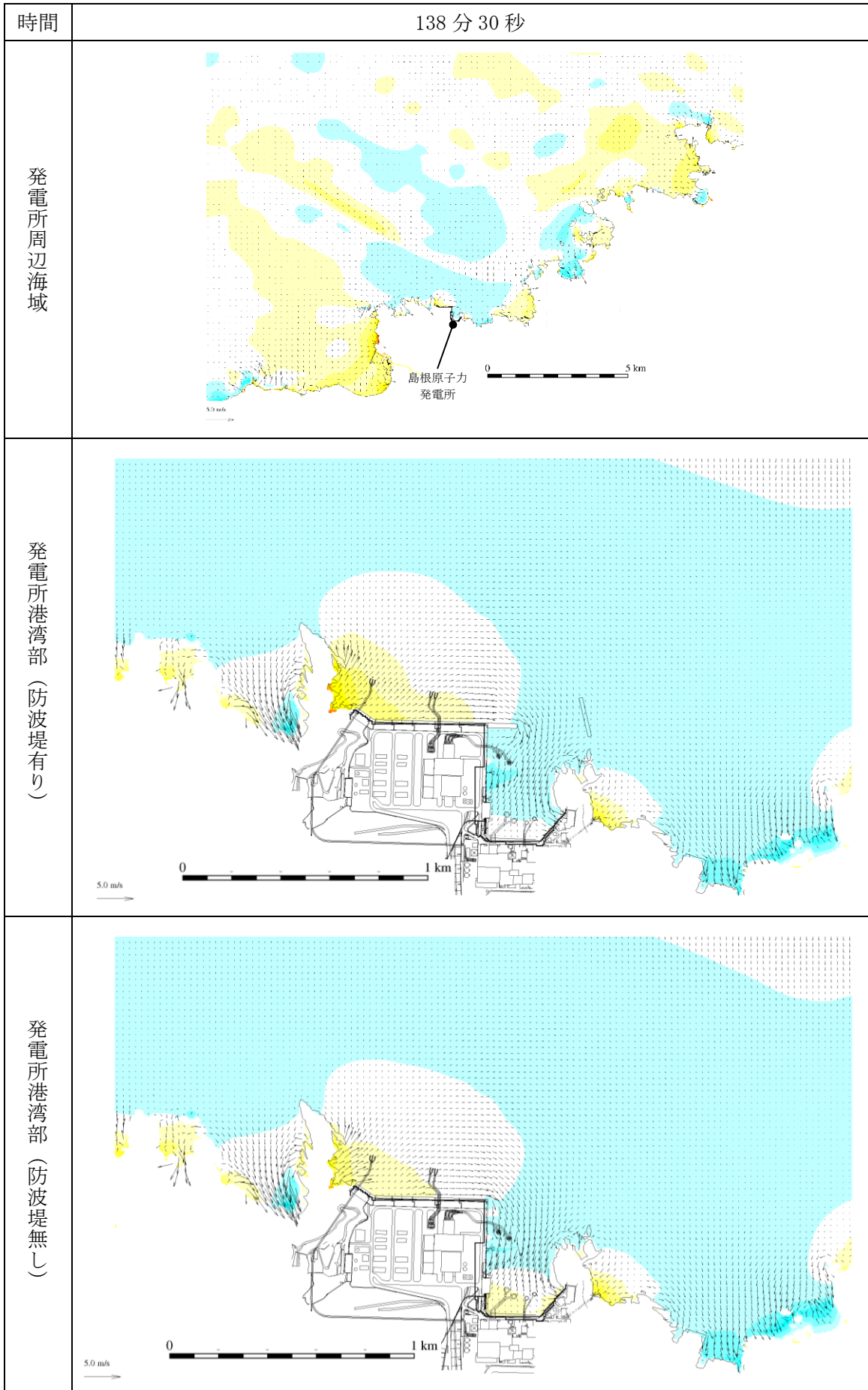
図 1-78 基準津波 1 の水位変動・流向ベクトル
