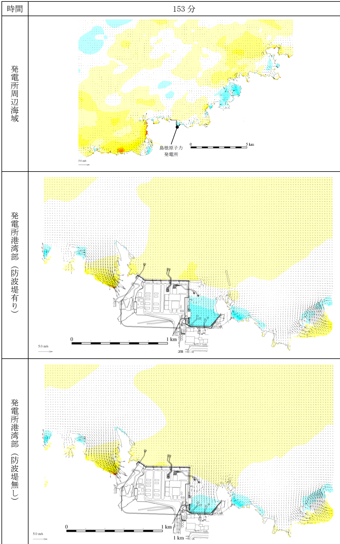
図 1-107 基準津波 1 の水位変動・流向ベクトル
