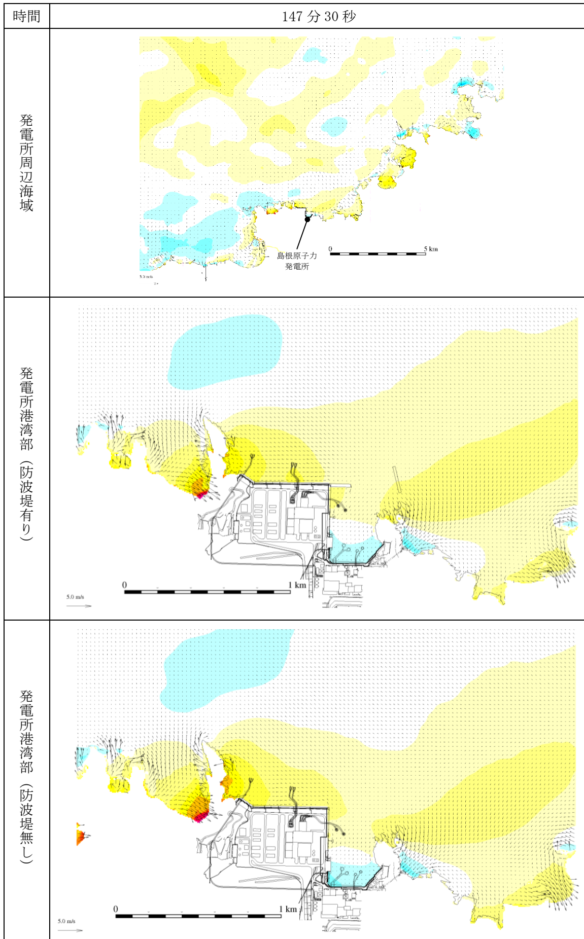
図 1-96 基準津波 1 の水位変動・流向ベクトル
