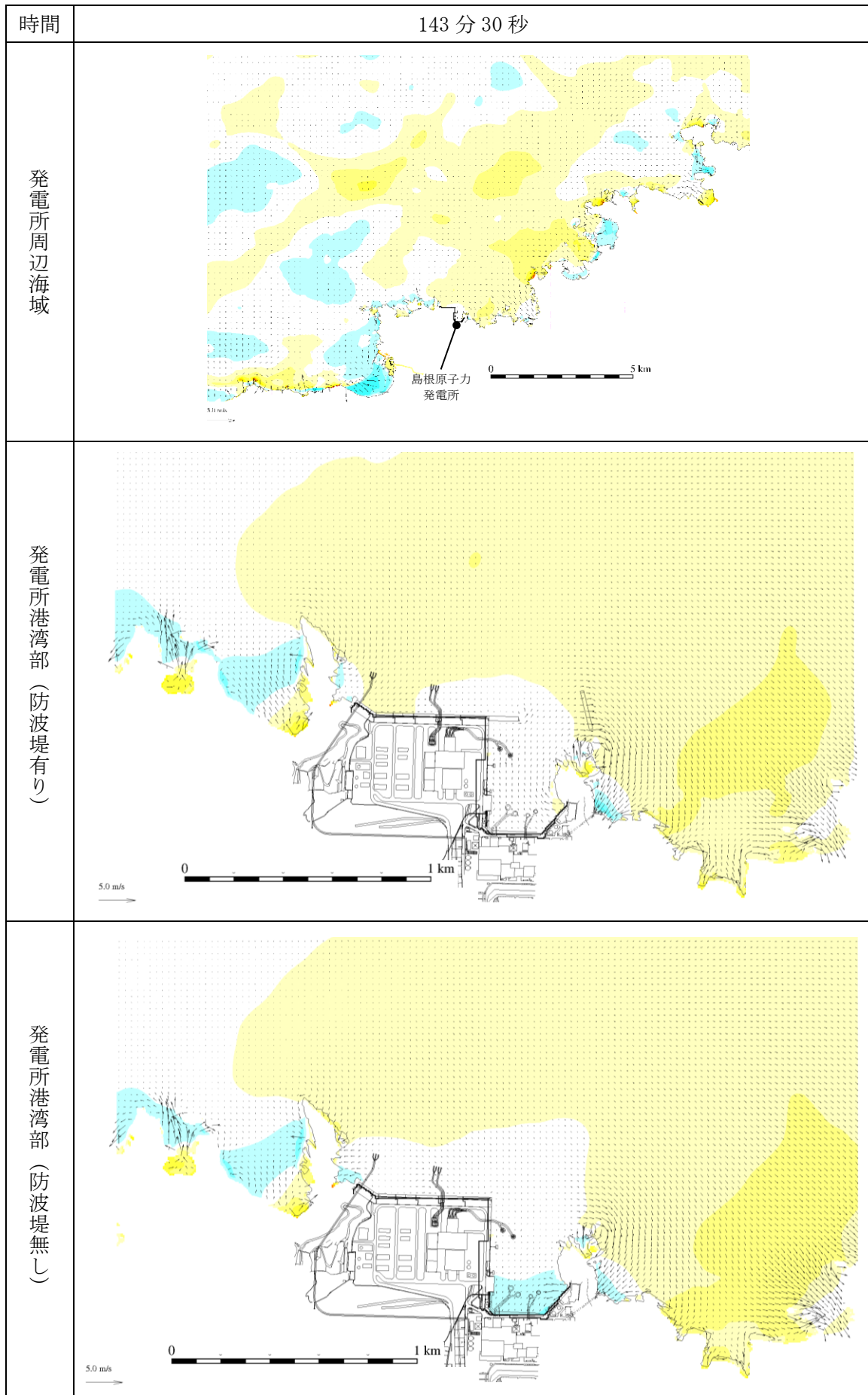
図 1-88 基準津波 1 の水位変動・流向ベクトル
