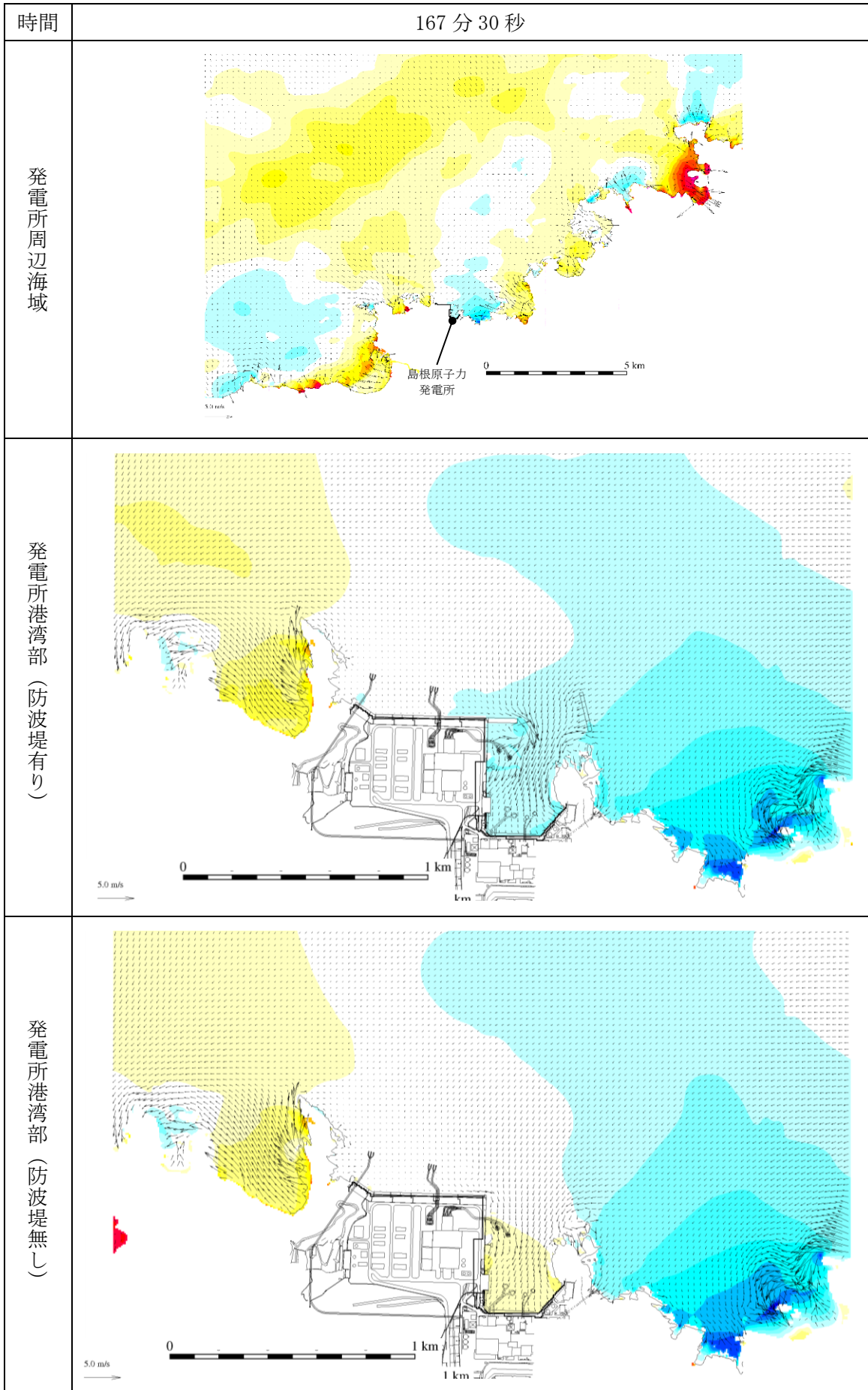
図 1-136 基準津波 1 の水位変動・流向ベクトル
