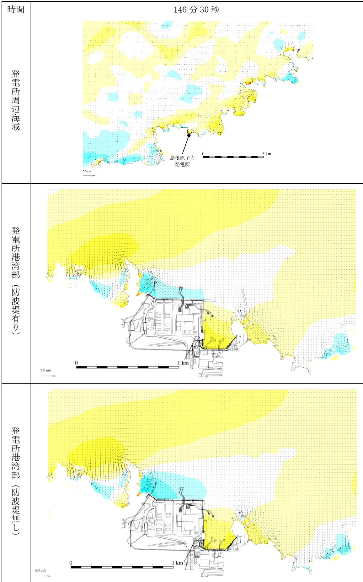
図 1-94 基準津波 1 の水位変動・流向ベクトル
