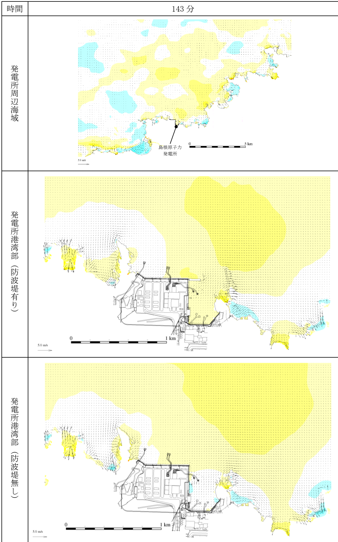
図 1-87 基準津波 1 の水位変動・流向ベクトル
