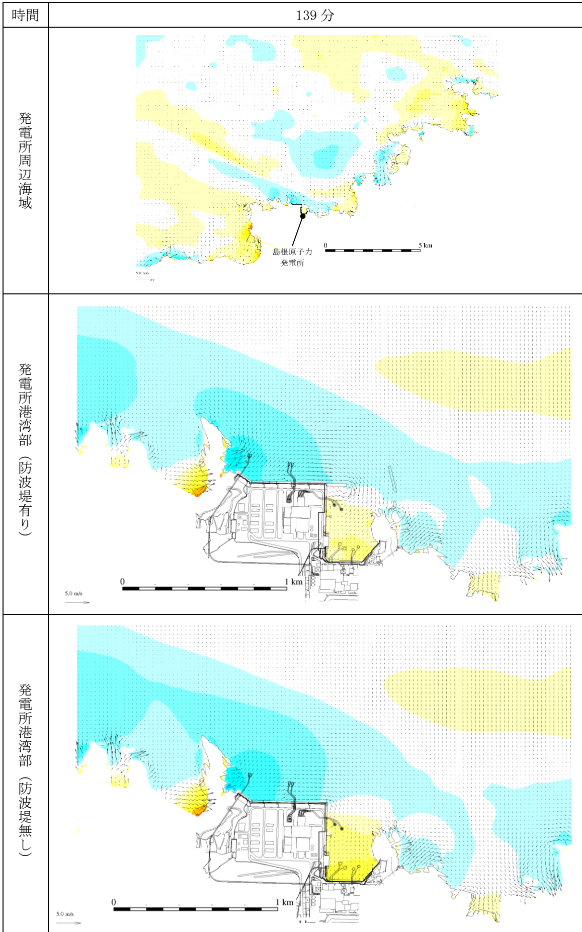
図 1-79 基準津波 1 の水位変動・流向ベクトル
