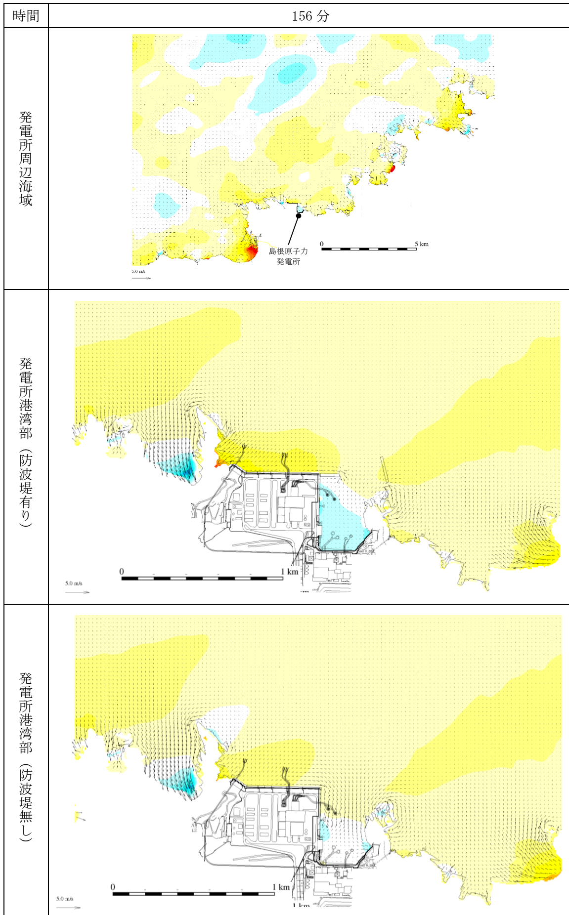
図 1-113 基準津波 1 の水位変動・流向ベクトル
