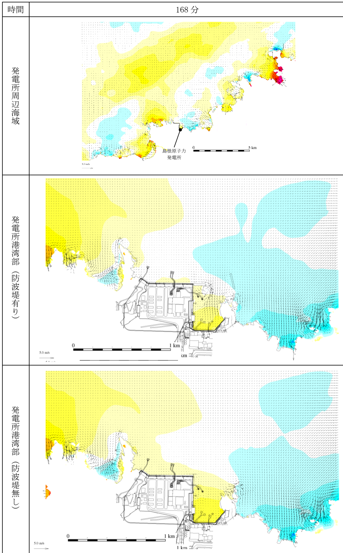
図 1-137 基準津波 1 の水位変動・流向ベクトル
