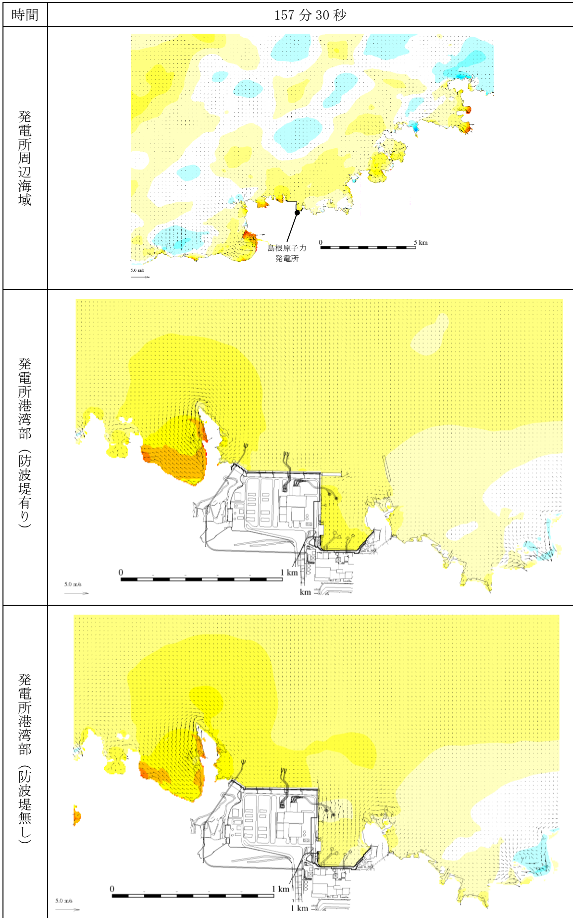
図 1-116 基準津波 1 の水位変動・流向ベクトル
