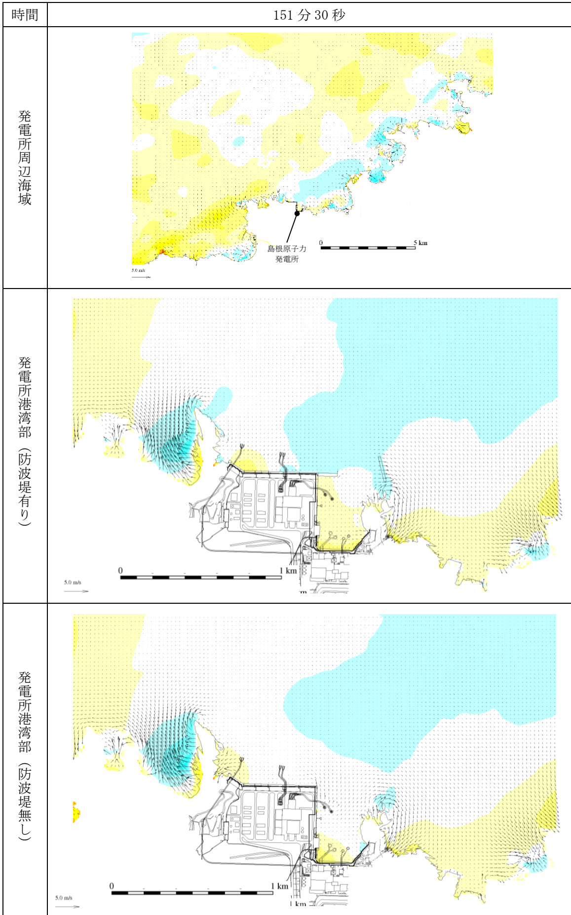
図 1-104 基準津波 1 の水位変動・流向ベクトル
