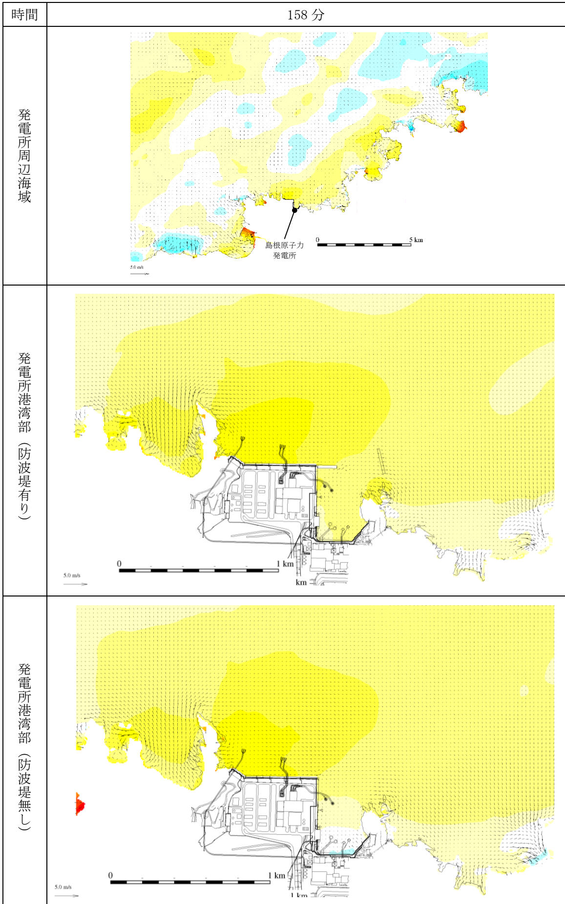
図 1-117 基準津波 1 の水位変動・流向ベクトル
