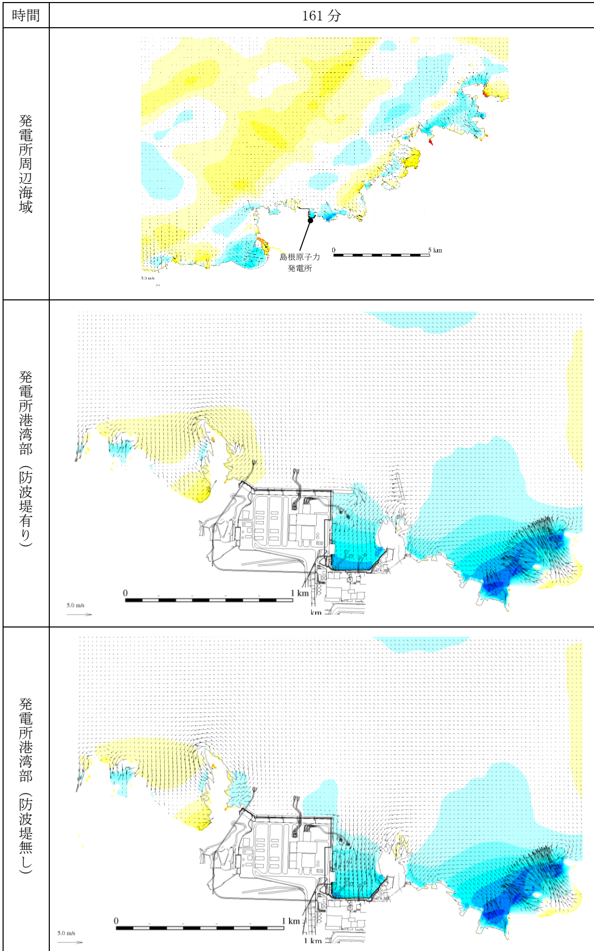
図 1-123 基準津波 1 の水位変動・流向ベクトル
