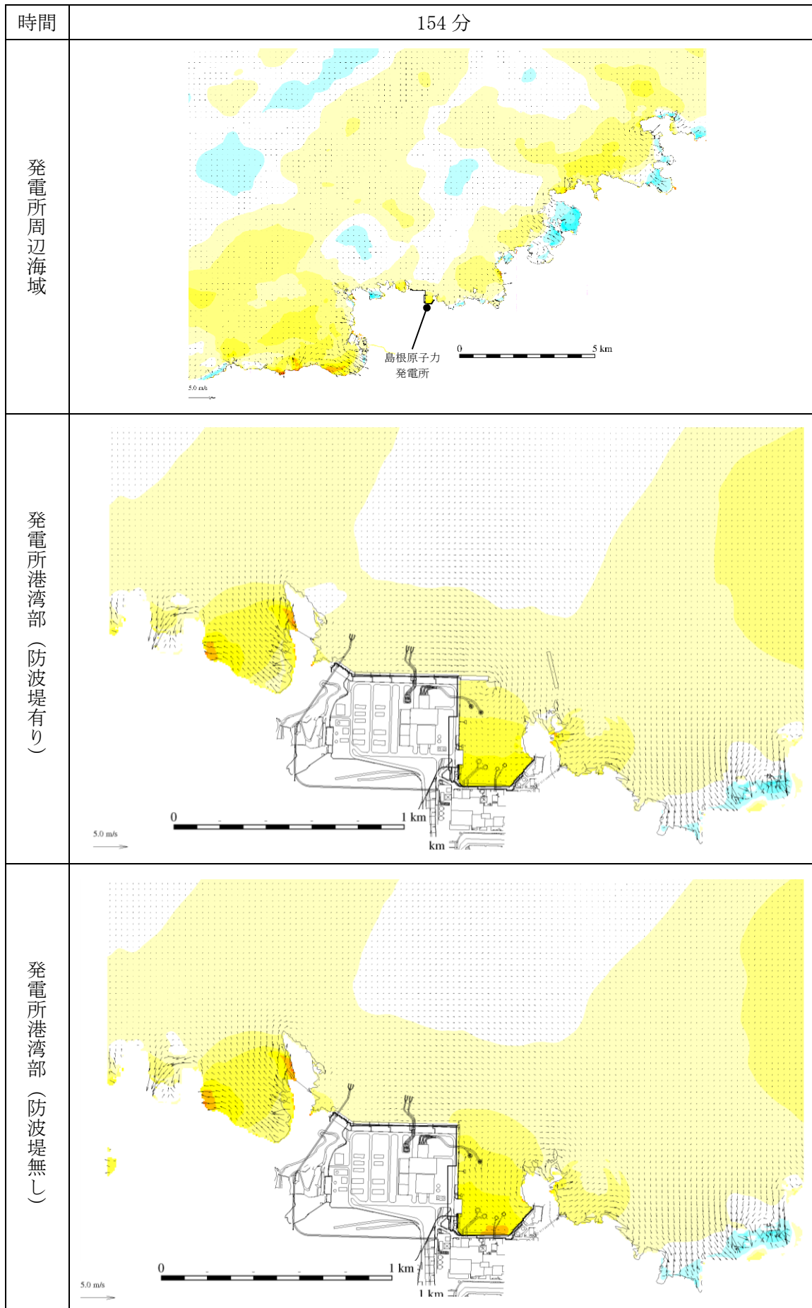
図 1-109 基準津波 1 の水位変動・流向ベクトル
