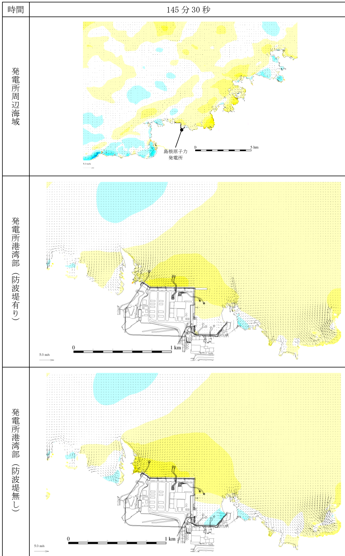
図 1-92 基準津波 1 の水位変動・流向ベクトル
