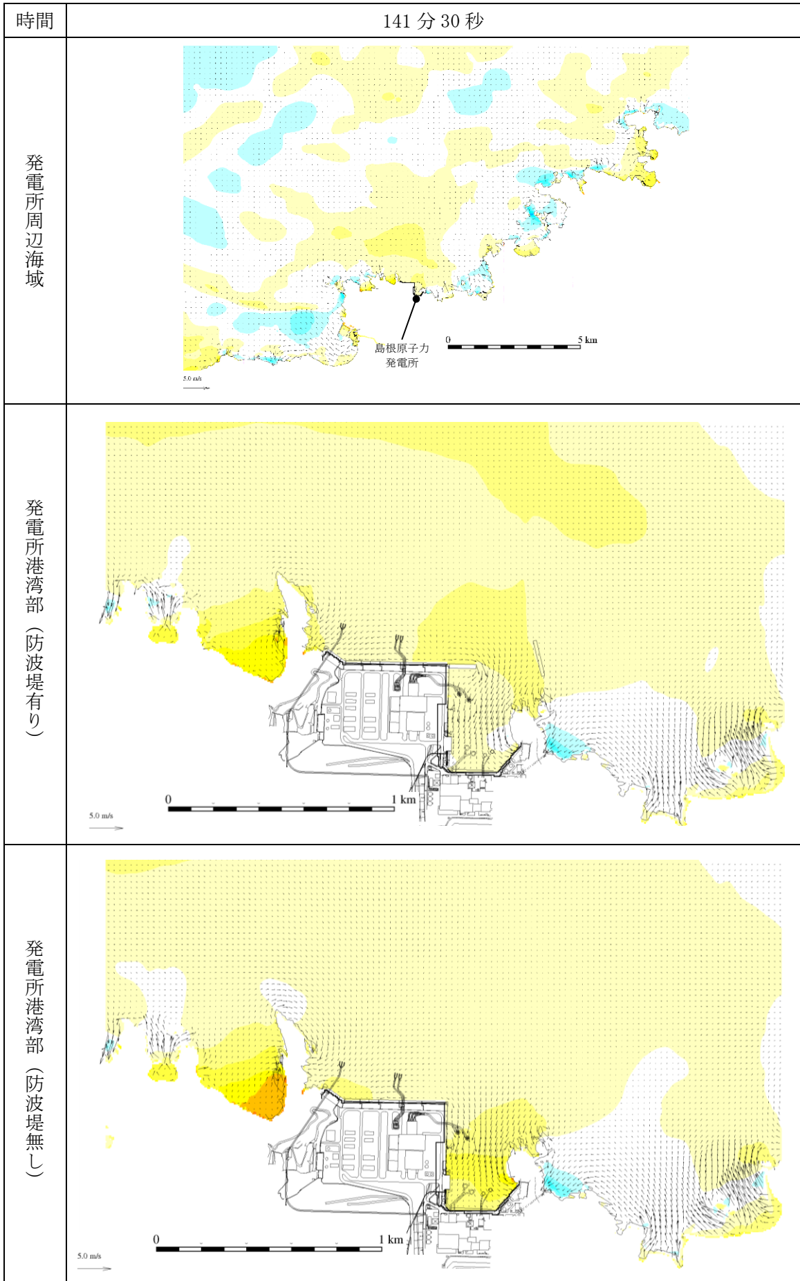
図 1-84 基準津波 1 の水位変動・流向ベクトル
