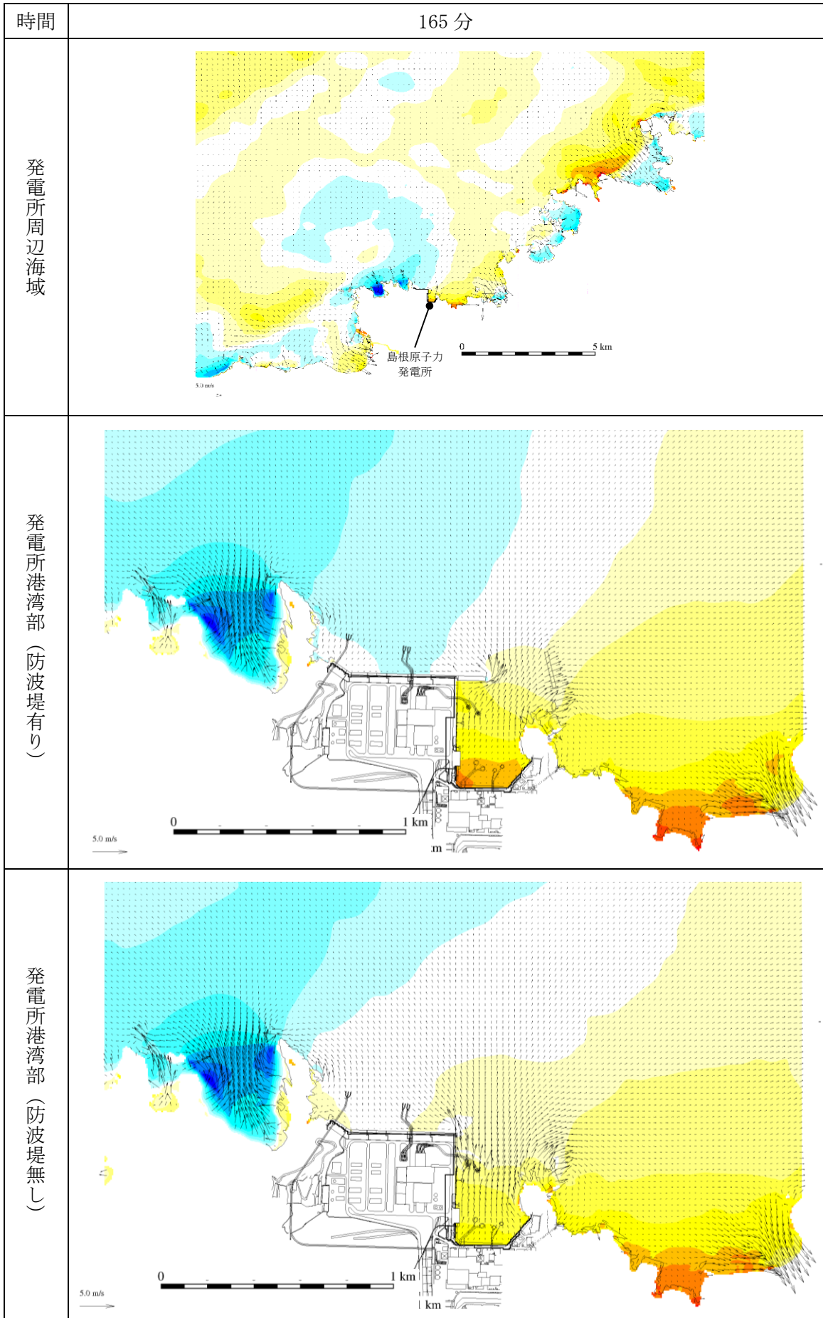
図 1-131 基準津波 1 の水位変動・流向ベクトル
