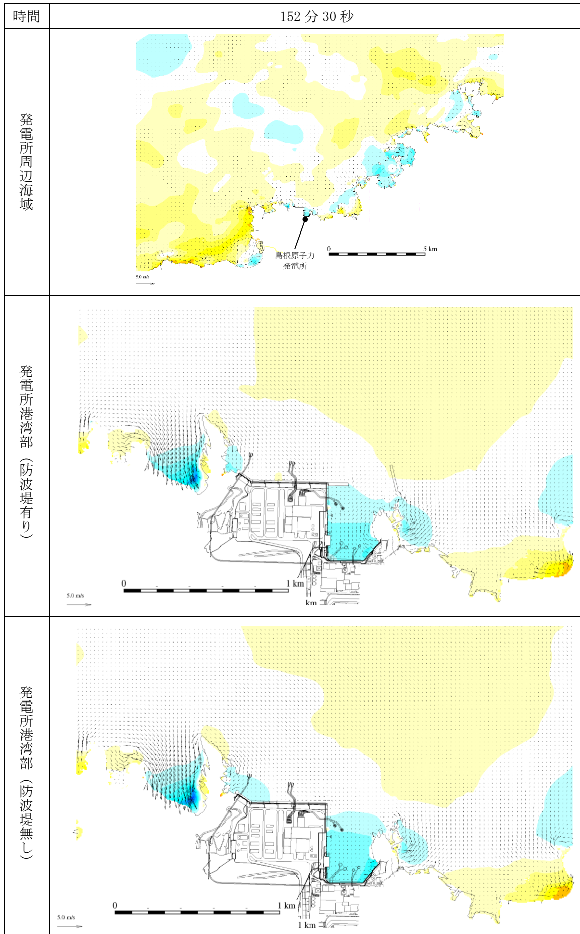
図 1-106 基準津波 1 の水位変動・流向ベクトル
