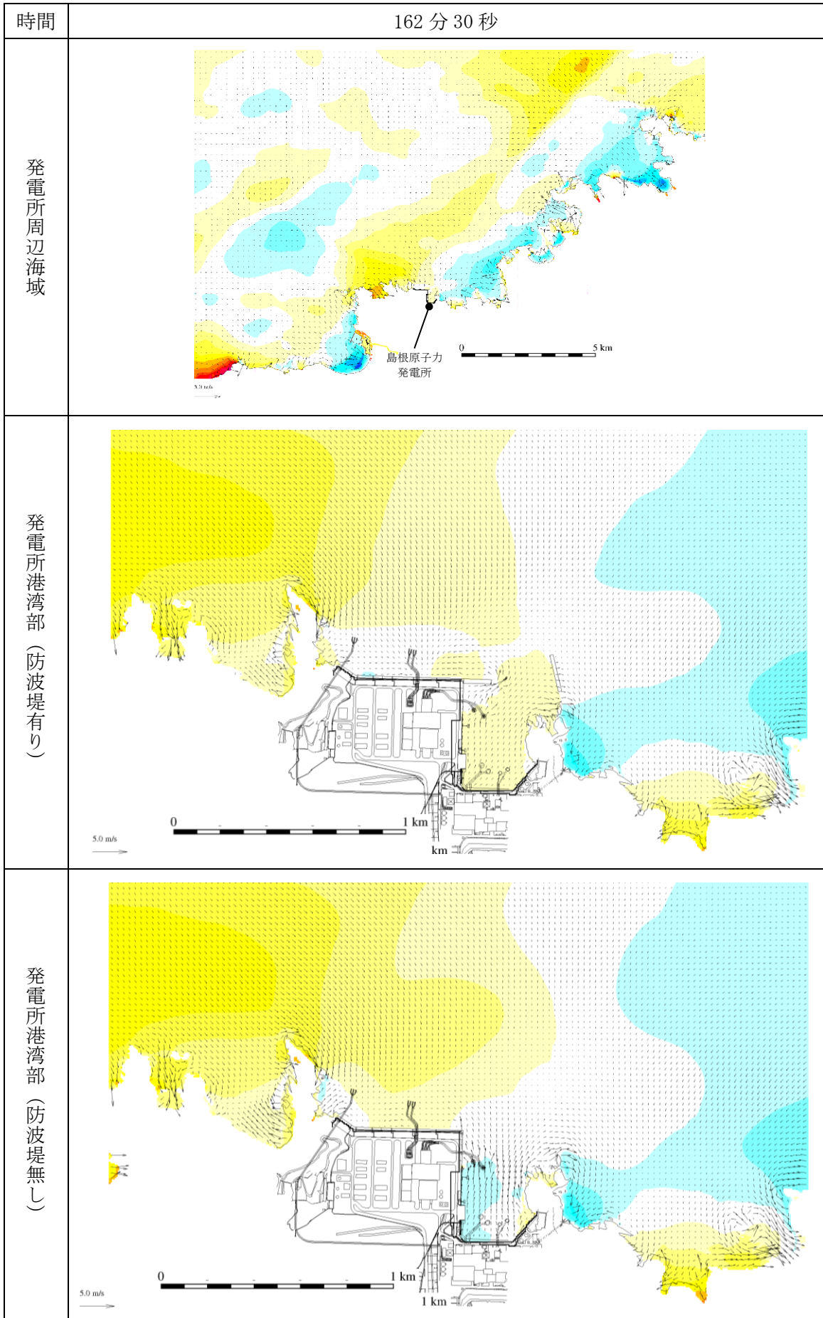
図 1-126 基準津波 1 の水位変動・流向ベクトル
