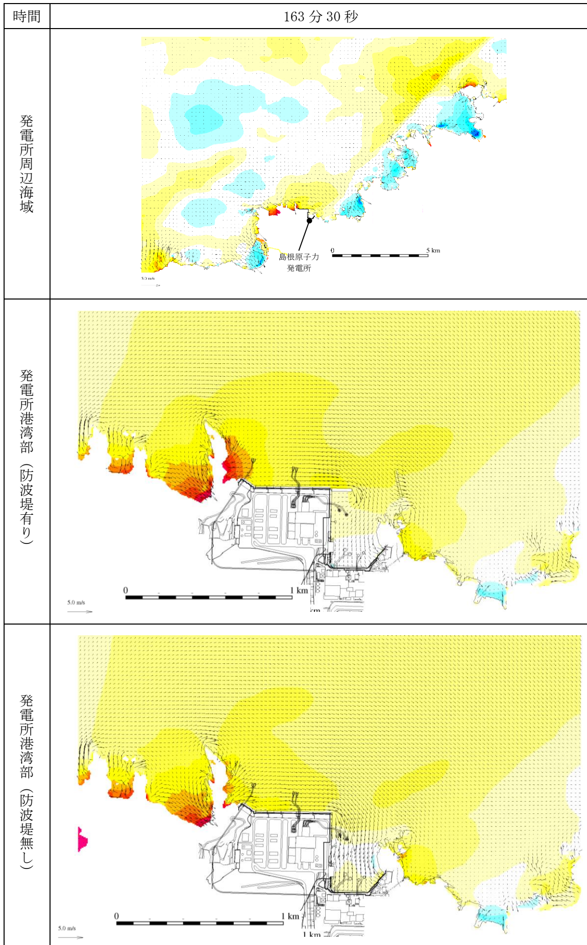
図 1-128 基準津波 1 の水位変動・流向ベクトル
