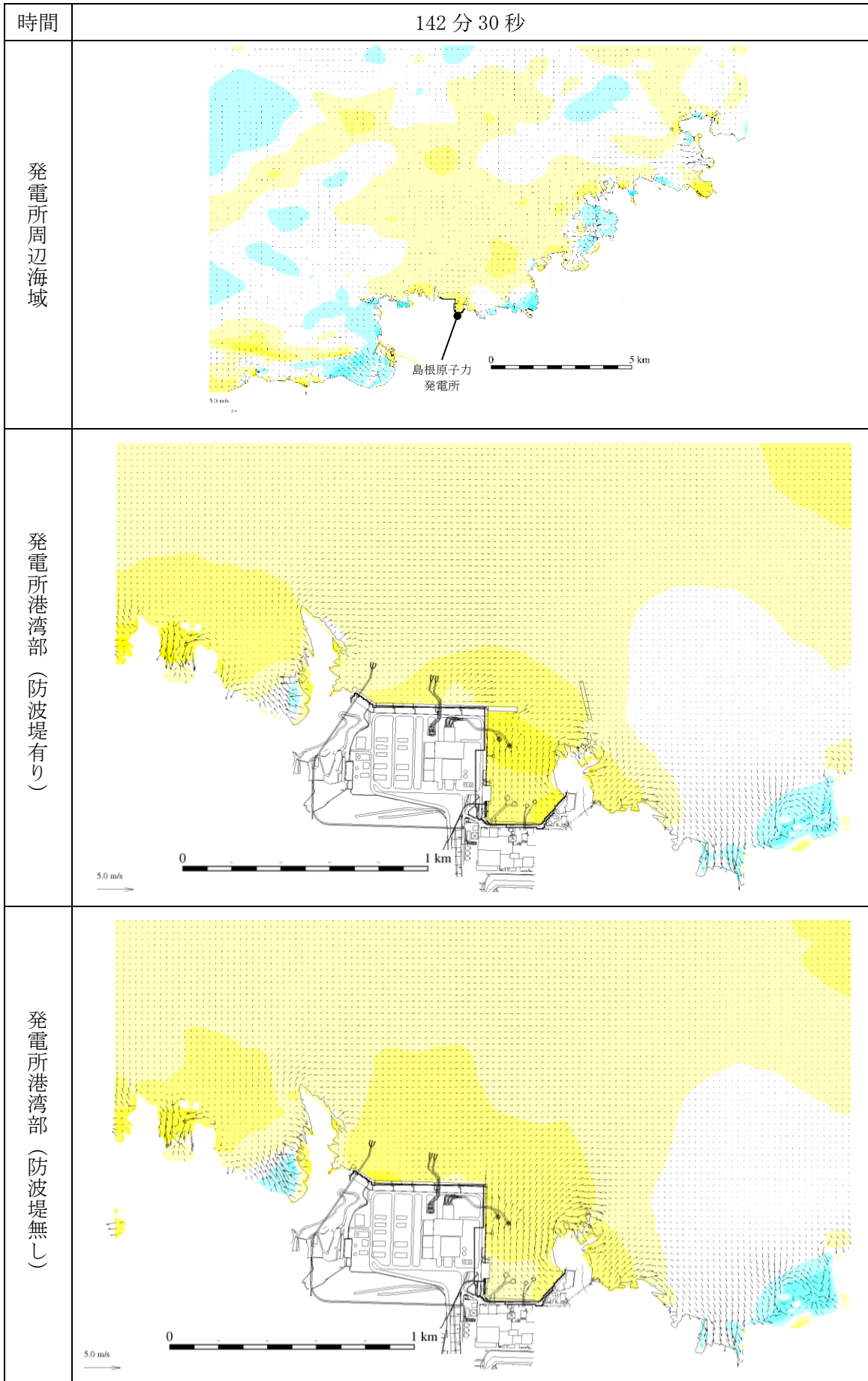
図 1-86 基準津波 1 の水位変動・流向ベクトル
