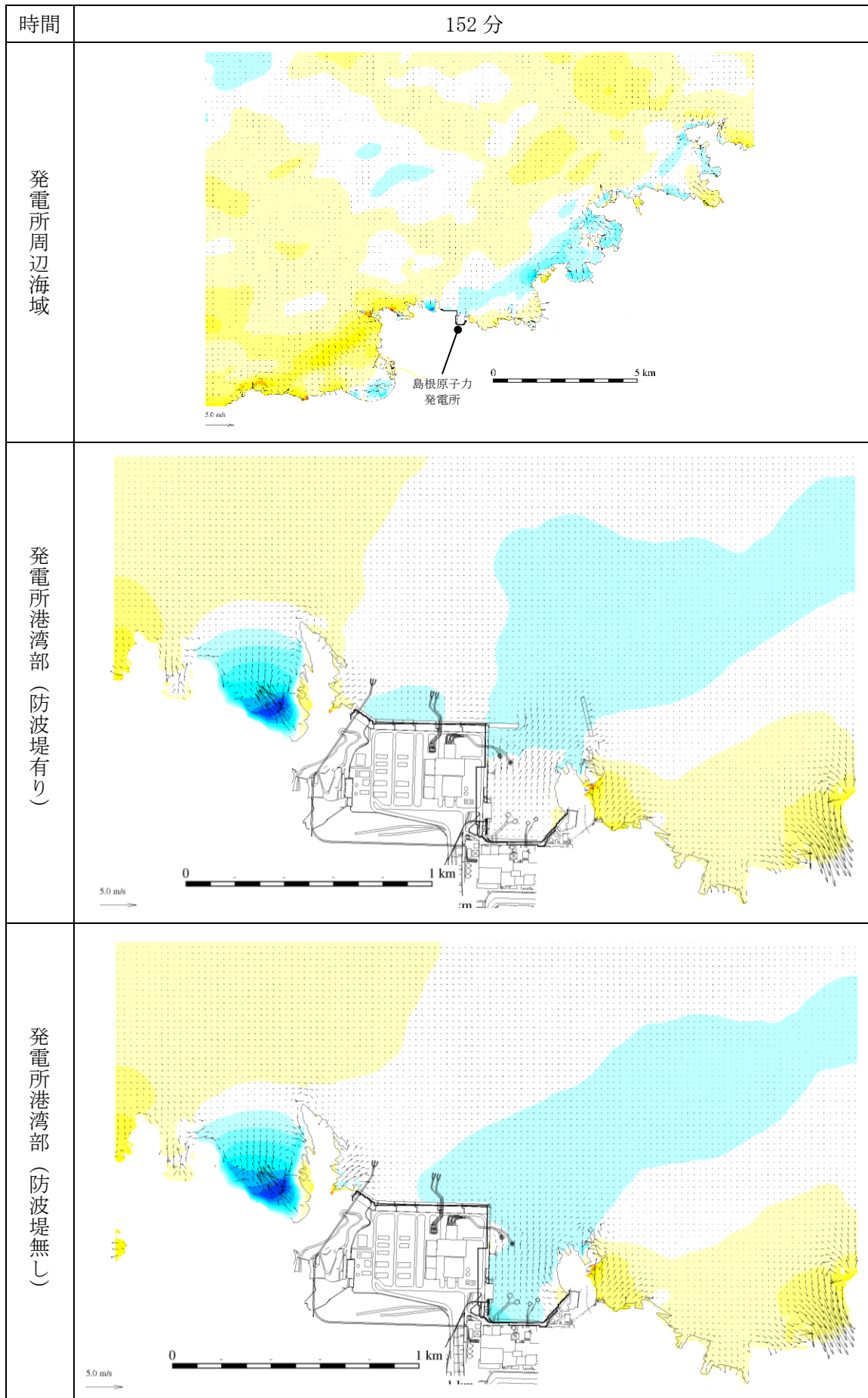
図 1-105 基準津波 1 の水位変動・流向ベクトル
