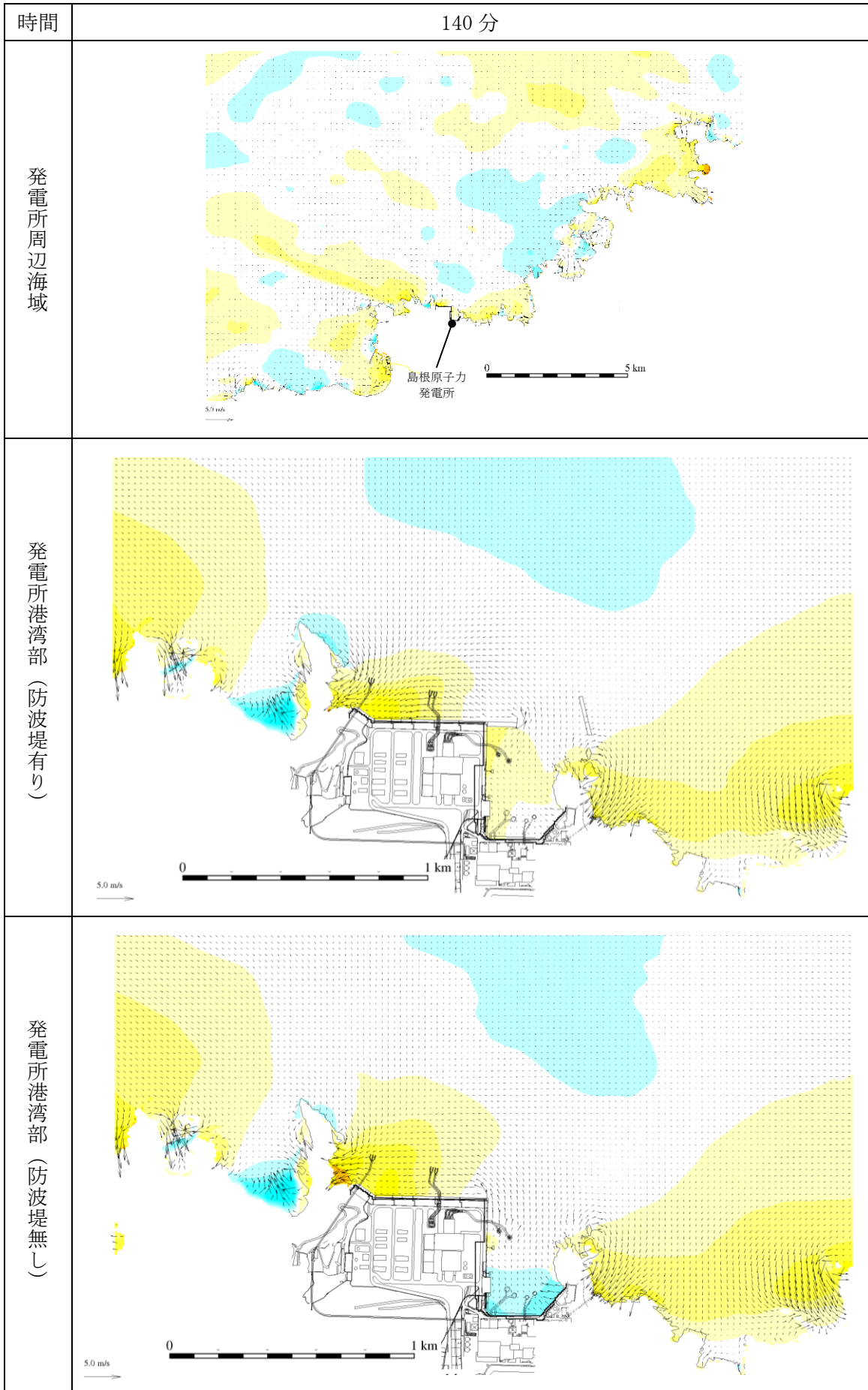
図 1-81 基準津波 1 の水位変動・流向ベクトル
