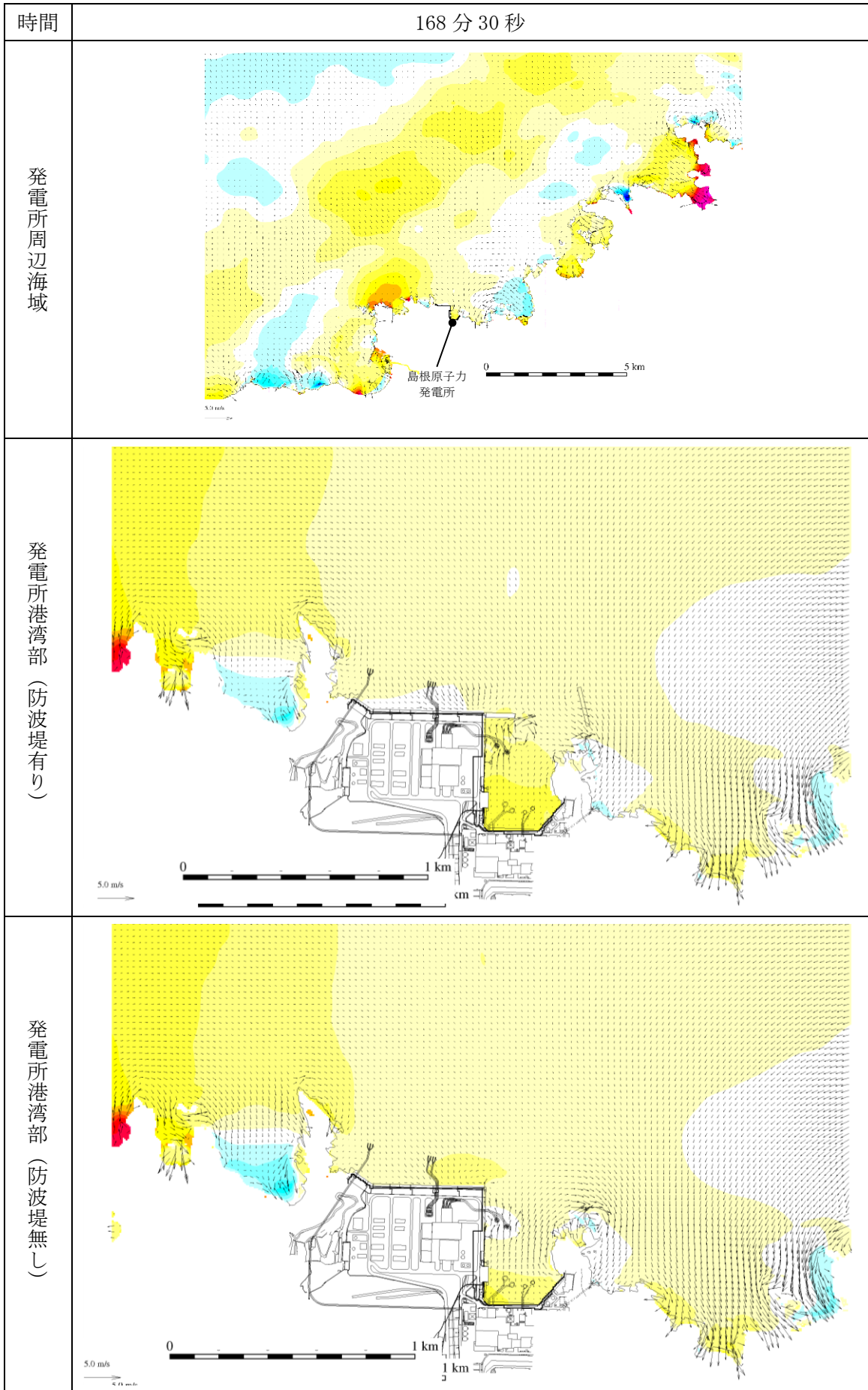
図 1-138 基準津波 1 の水位変動・流向ベクトル
