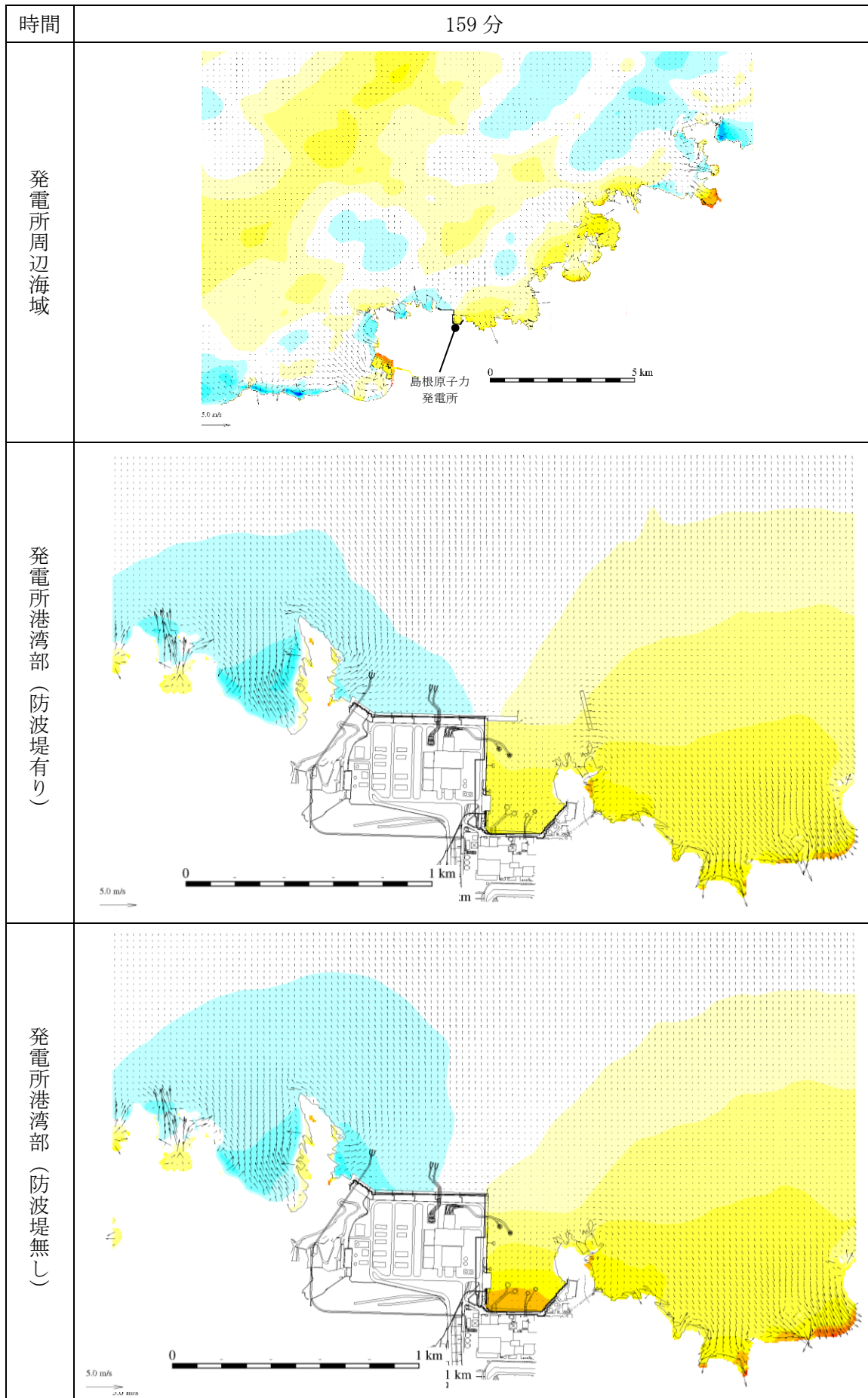
図 1-119 基準津波 1 の水位変動・流向ベクトル
