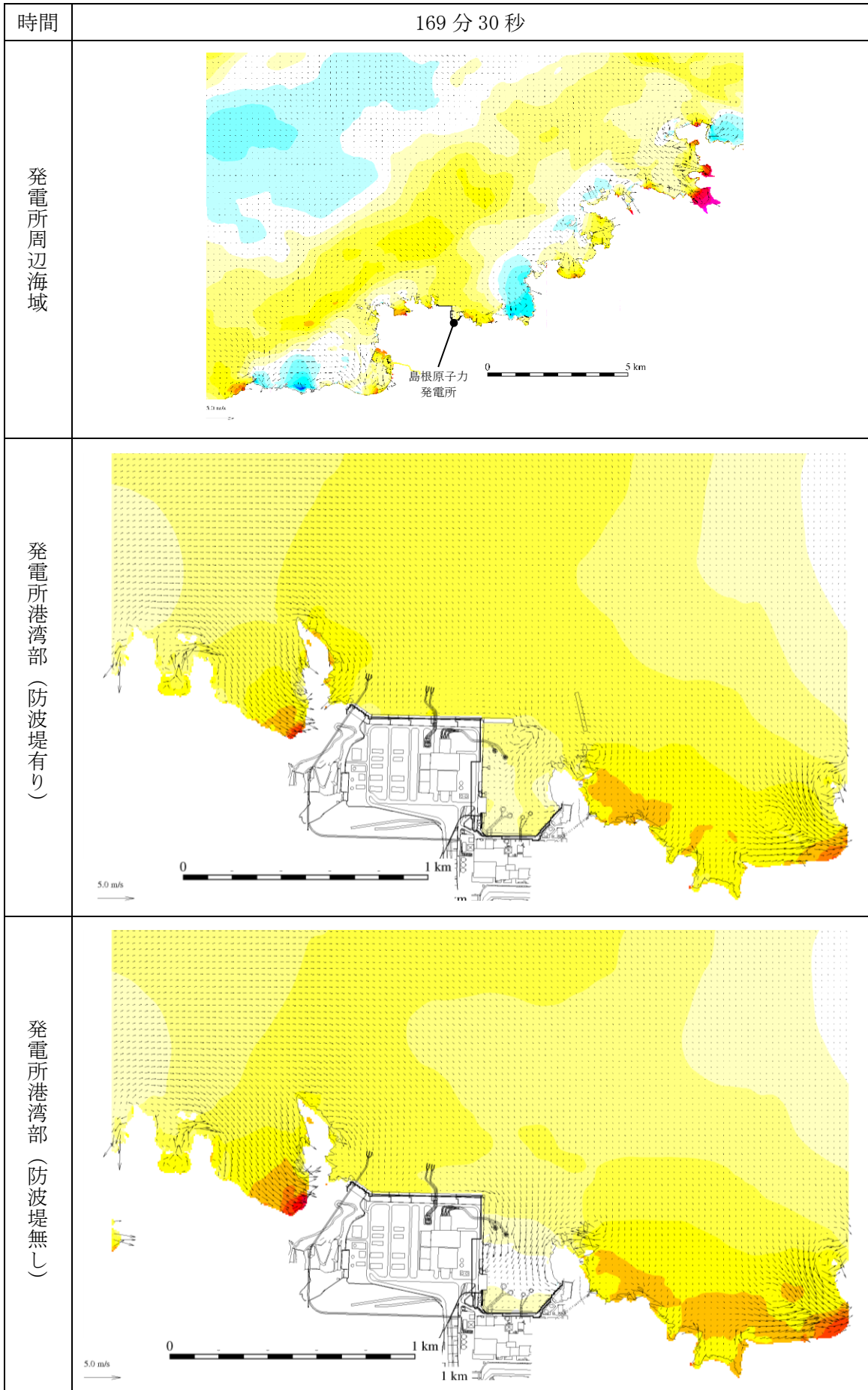
図 1-140 基準津波 1 の水位変動・流向ベクトル
