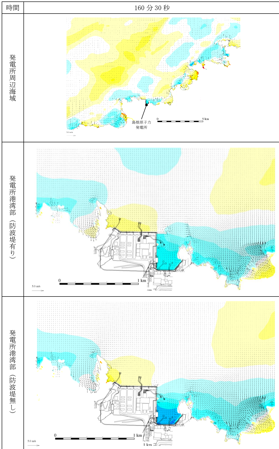
図 1-122 基準津波 1 の水位変動・流向ベクトル
