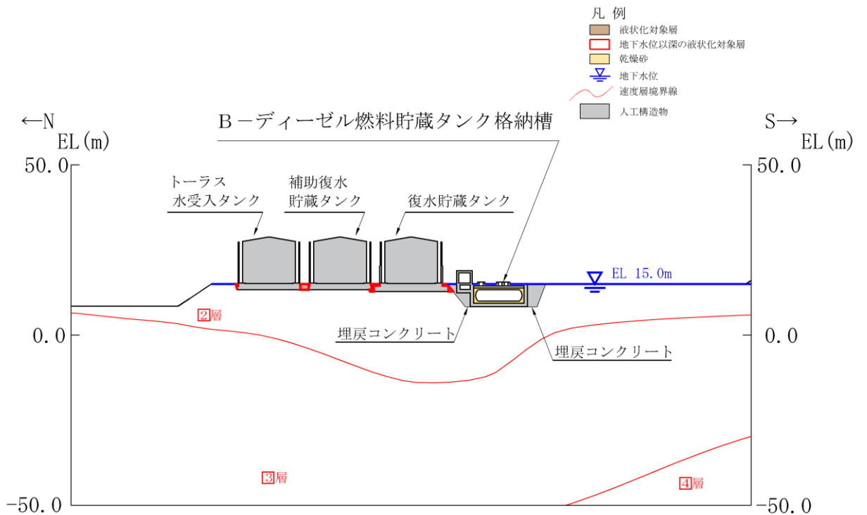
(速度層図)
