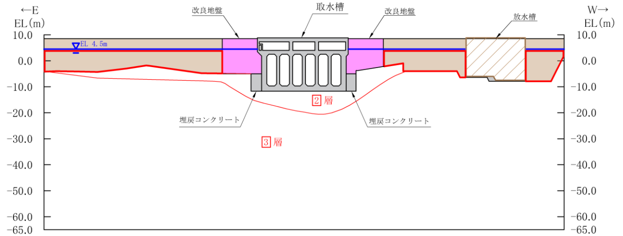
図 4.3-2(21) 取水槽【A-A断面位置】 地質断面図 (⑤有効応力解析)
