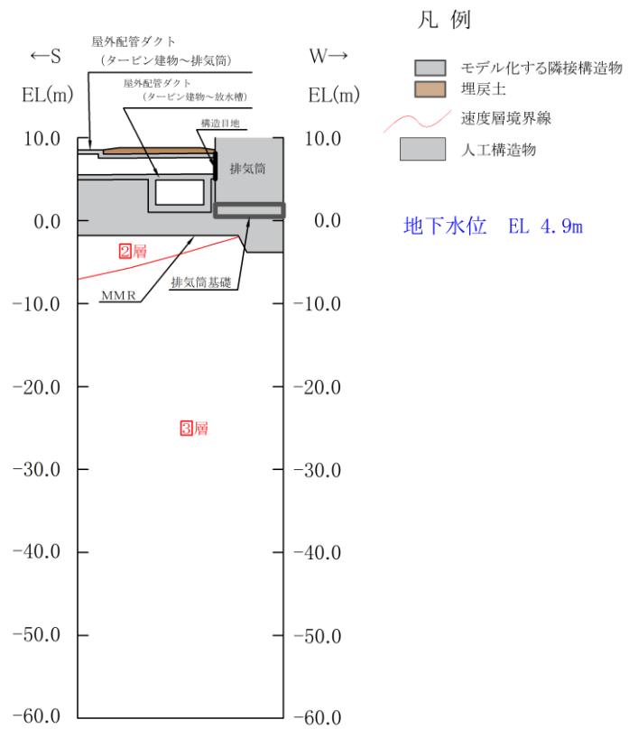
(速度層図)
