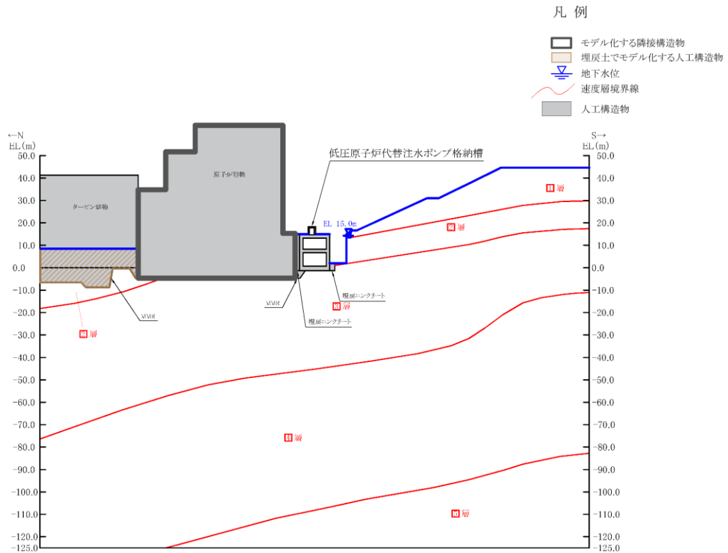
図 8.1-3(9) 隣接構造物としてモデル化する場合の例 (c) 原子炉建物：低圧原子炉代替注水ポンプ格納槽【A-A断面位置】
