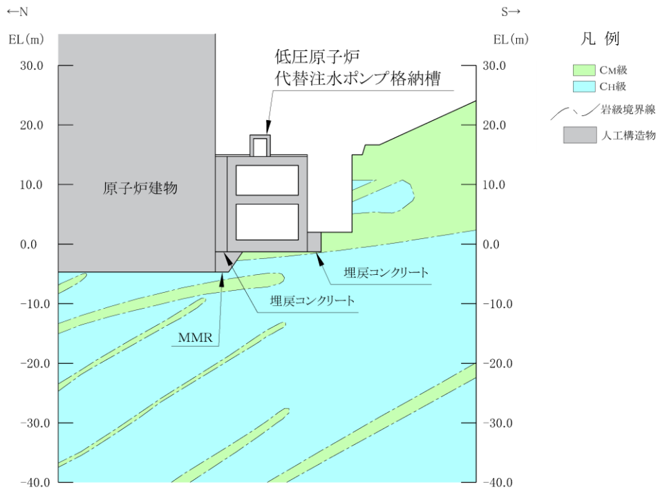
(岩級図)
