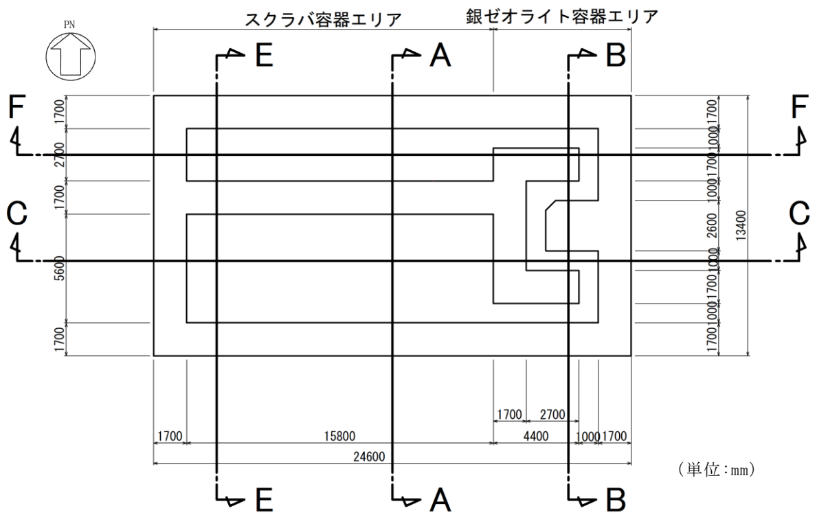
図 2-1 (1) 第 1 ベントフィルタ格納槽 平面図 (EL 3.00m)
