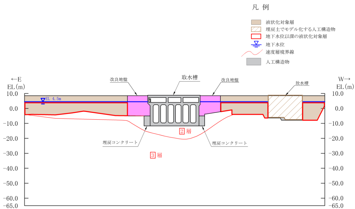
(速度層図)
