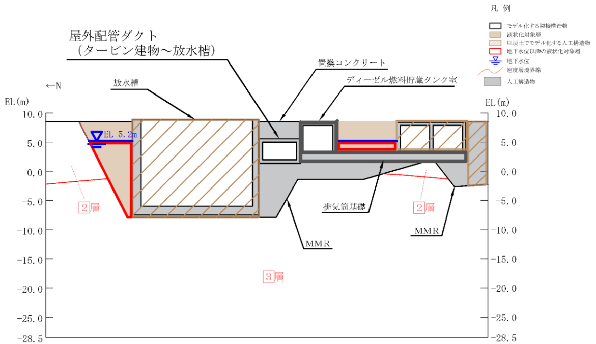
図 8.1-3(2) 隣接構造物としてモデル化する場合の例 (a) 排気筒基礎及びディーゼル燃料貯蔵タンク室：屋外配管ダクト (タービン建物～放水槽) 【A-A断面位置】
