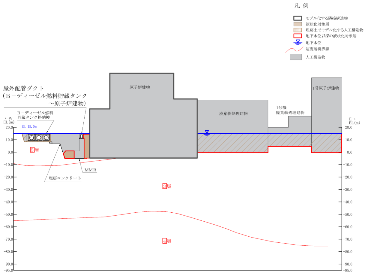
(全体図)
