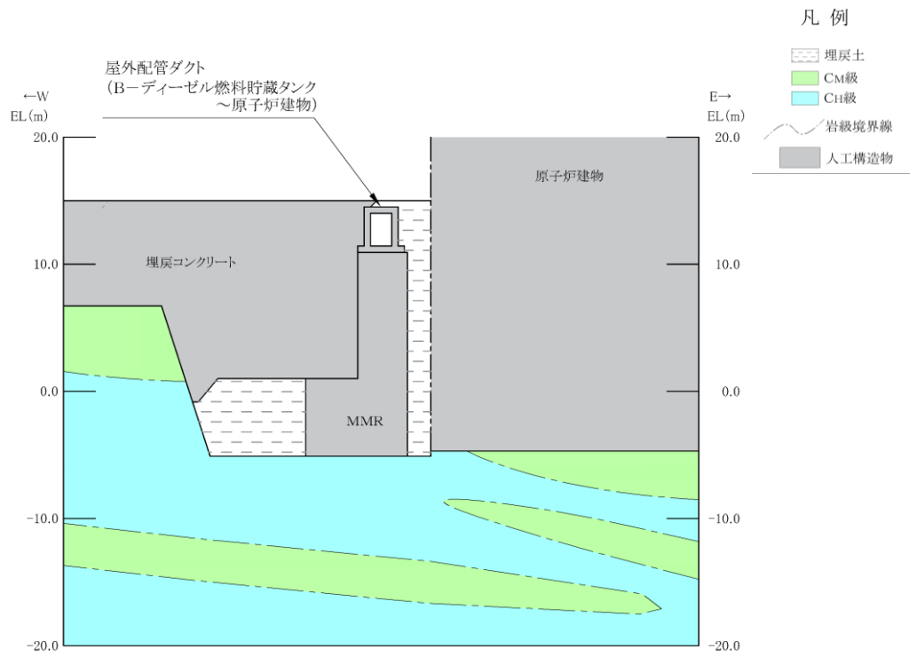
(岩級図)
