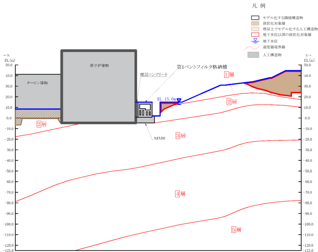
図 8.1-3(7) 隣接構造物としてモデル化する場合の例 (c) 原子炉建物：第1ベントフィルタ格納槽【B-B断面位置】
