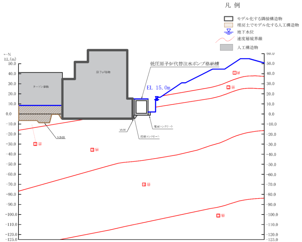
図 4.3-2(16) 低圧原子炉代替注水ポンプ格納槽【B-B断面位置】 地質断面図 (②全応力解析)
