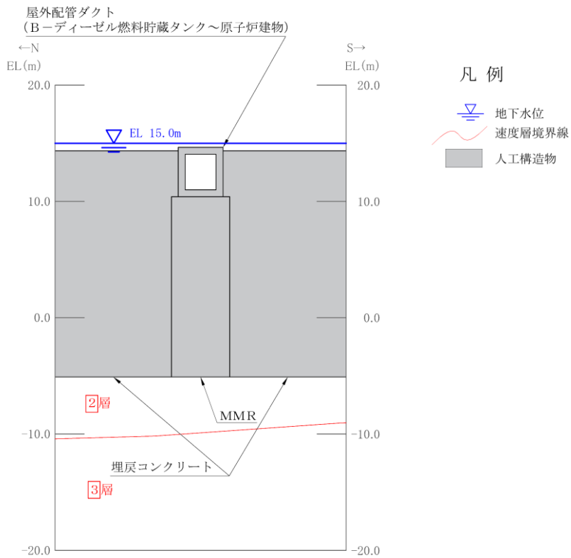
(速度層図)
