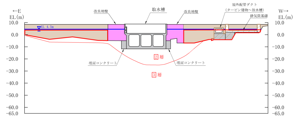
図 4.3-2(22) 取水槽【B-B断面位置】 地質断面図 (⑤有効応力解析)
