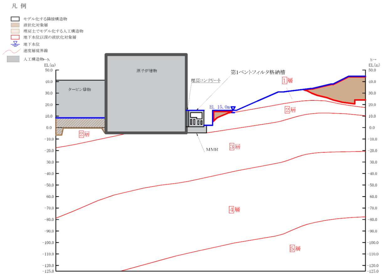
(速度層図)
