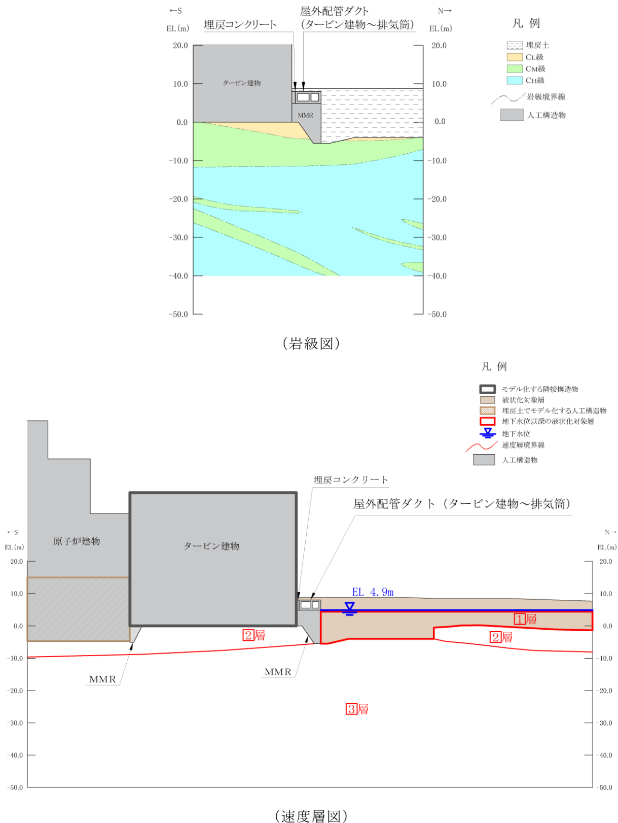
図 4.5-5(1) 屋外配管ダクト (タービン建物～排気筒) 地質断面図 (A-A 断面位置)
