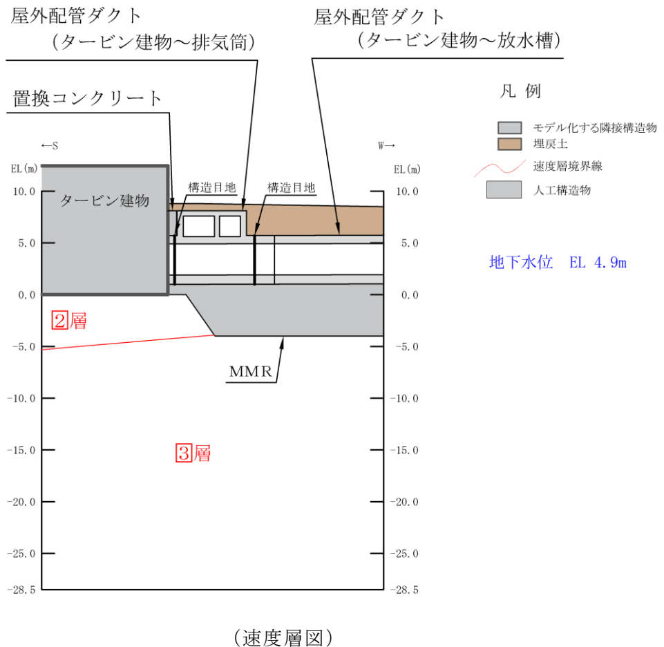
図 4.5-5(2) 屋外配管ダクト (タービン建物～排気筒) 地質断面図 (B-B 断面位置)
