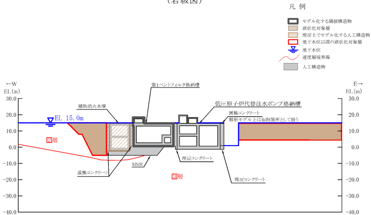
(岩級図)
