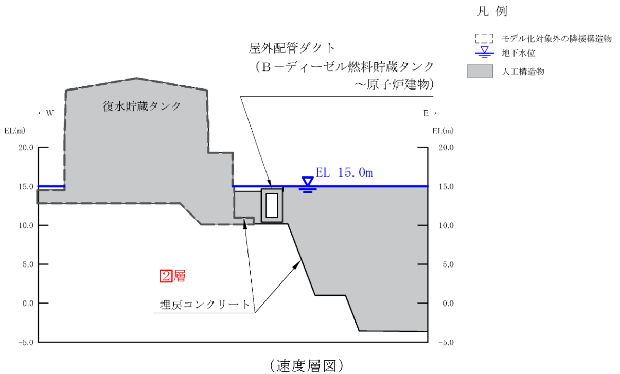
図 4.7-4 (1) 屋外配管ダクト (B-ディーゼル燃料貯蔵タンク～原子炉建物) 地質断面図 (A-A 断面位置)
