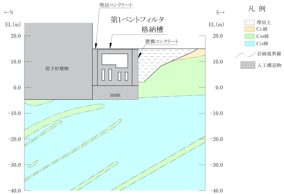
(岩級図)
