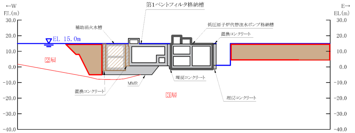
図 4.3-2(26) 第1ベントフィルタ格納槽図【C-C断面位置】 地質断面図 (⑤有効応力解析)
