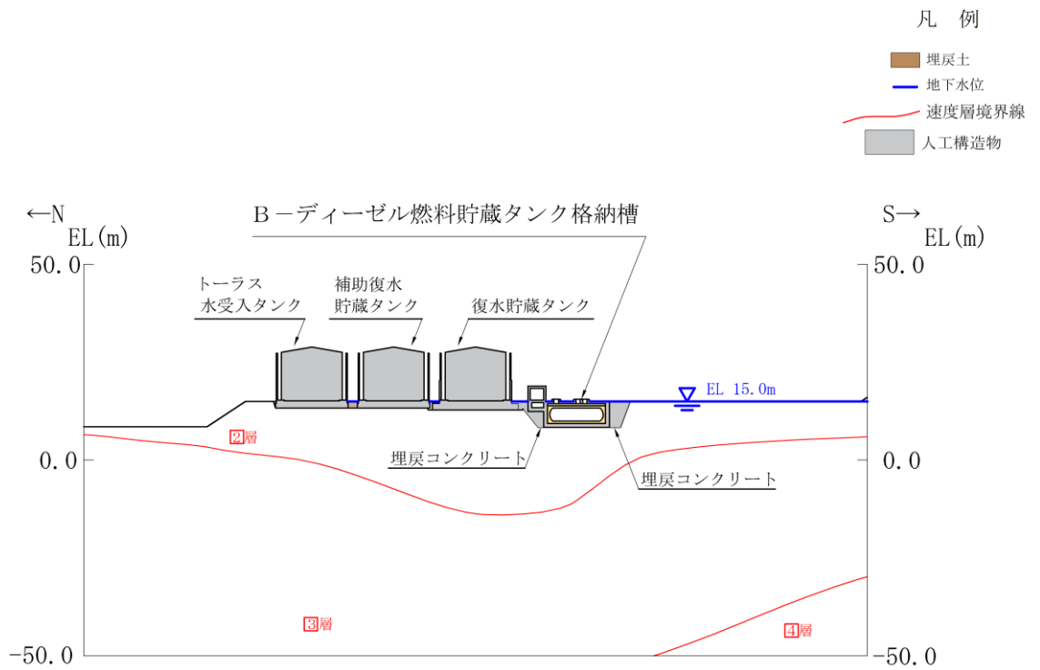
図 4.3-2(10) B-ディーゼル燃料貯蔵タンク格納槽【B-B断面位置】 地質断面図 (②全応力解析)
