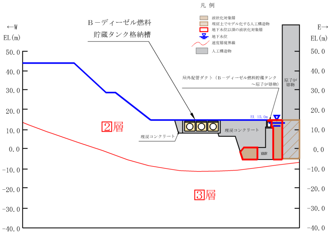
図 2-9 地質断面図 (B-ディーゼル燃料貯蔵タンク格納槽【A-A断面位置】)
