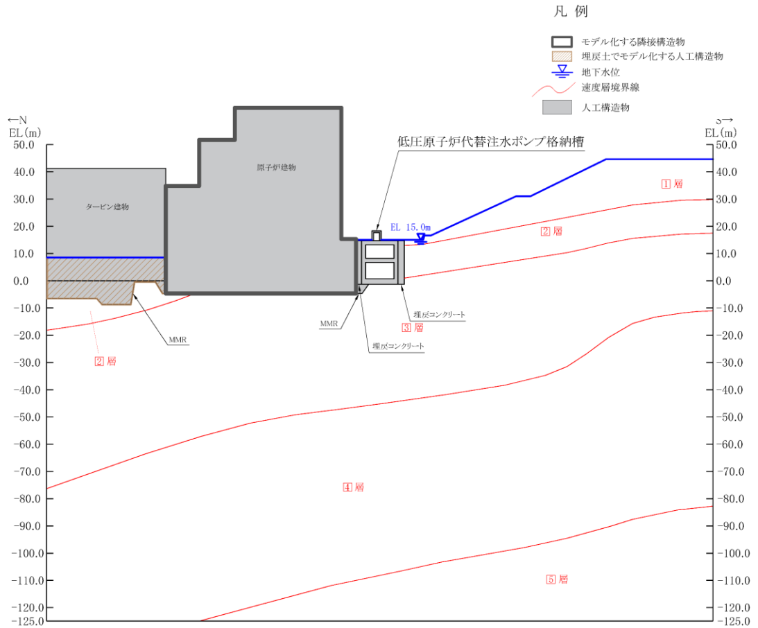
(速度層図)
