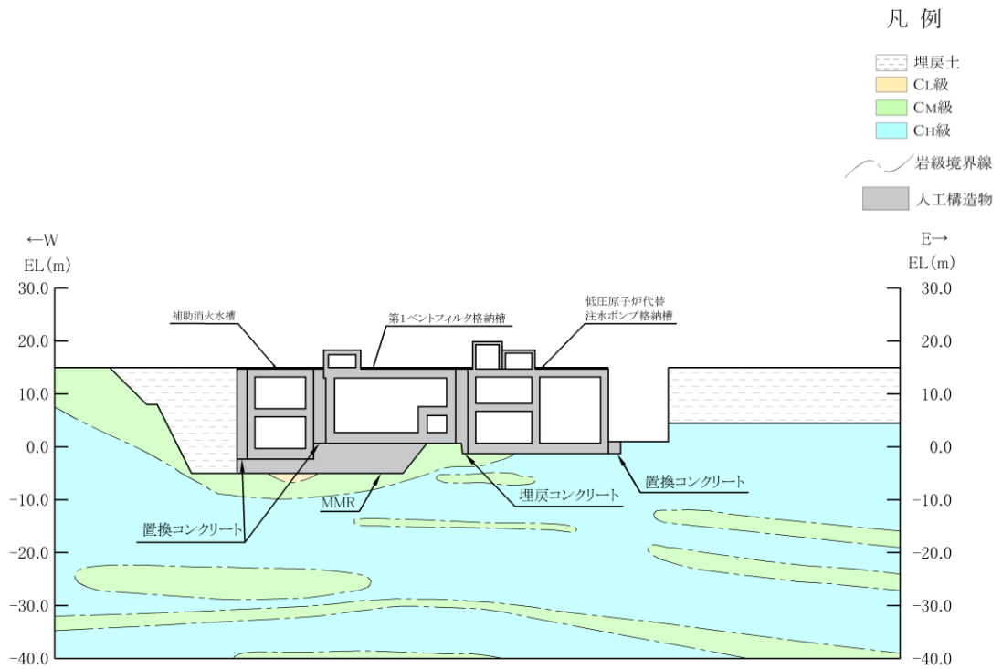
(岩級図)
