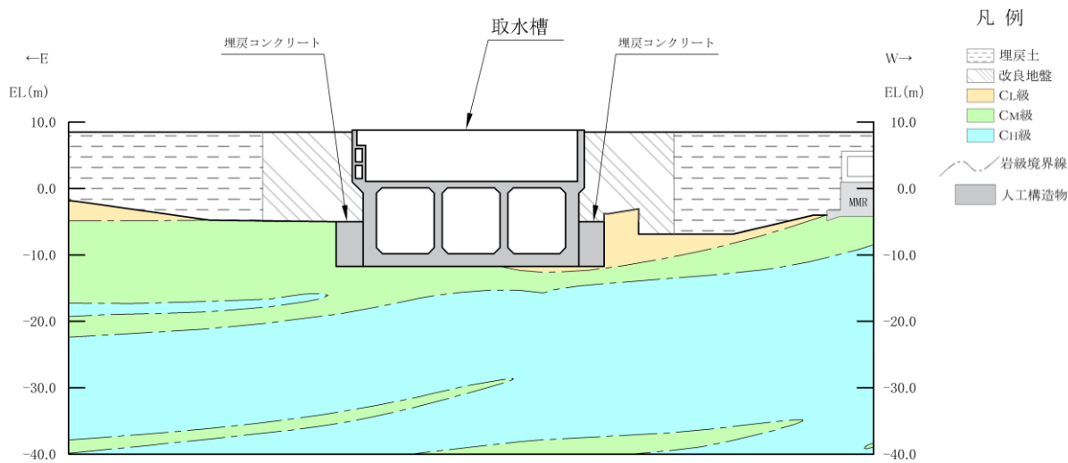
(岩級図)
