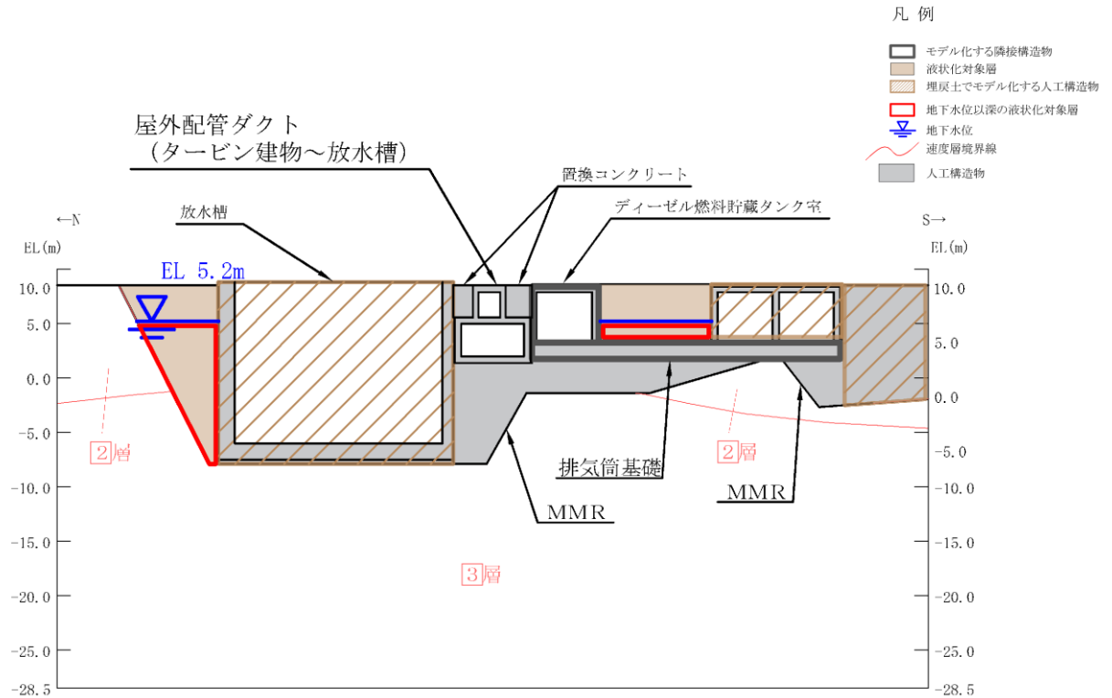
図 8.1-3(3) 隣接構造物としてモデル化する場合の例 (a) 排気筒基礎及びディーゼル燃料貯蔵タンク室：屋外配管ダクト (タービン建物～放水槽) 【B-B断面位置】
