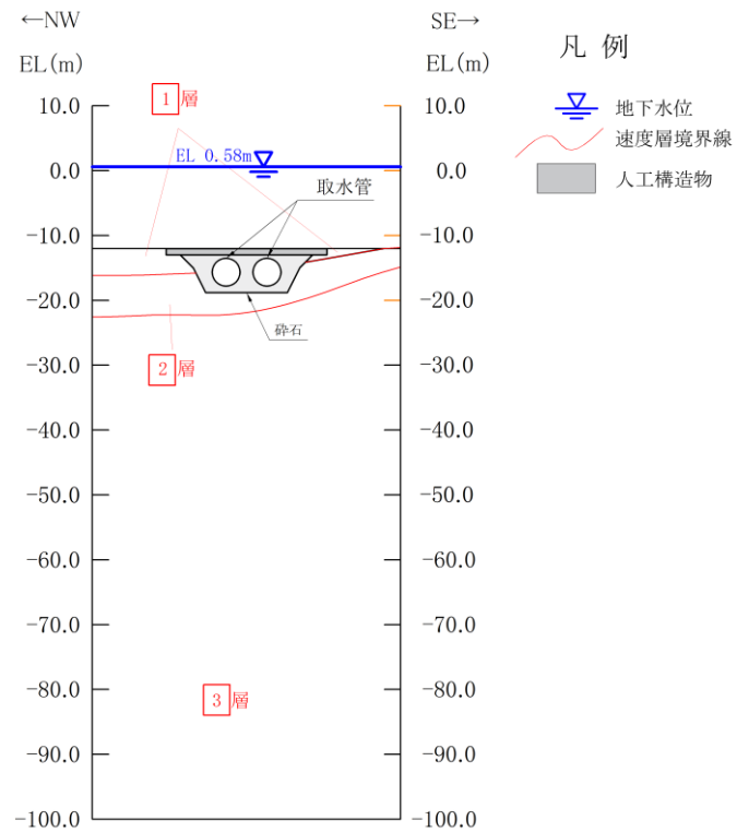
図 4.3-2(9) 取水管【E-E断面位置】 地質断面図 (②全応力解析)
