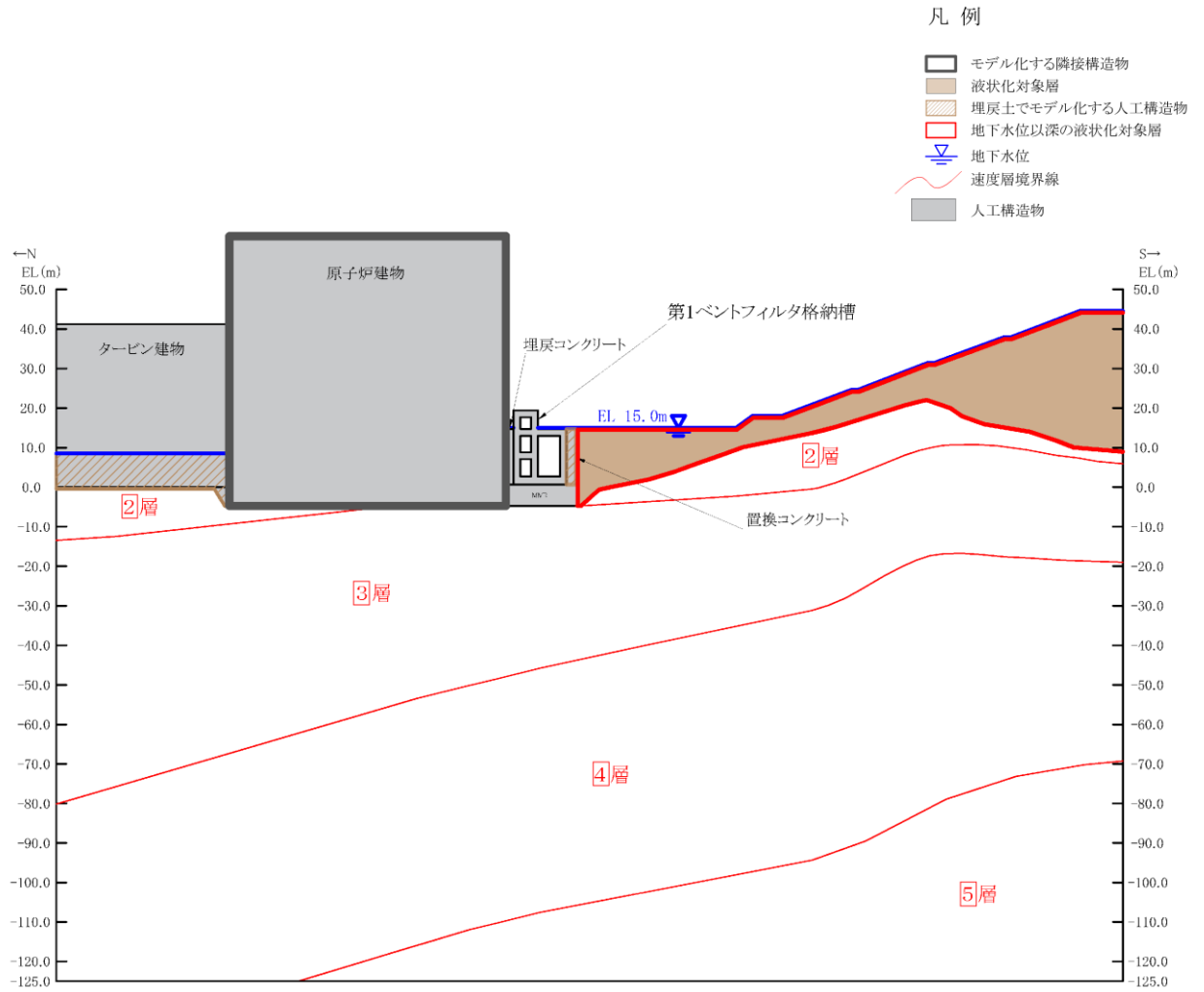
図 2-15 第 1 ベントフィルタ格納槽断面図 (A-A 断面位置)
