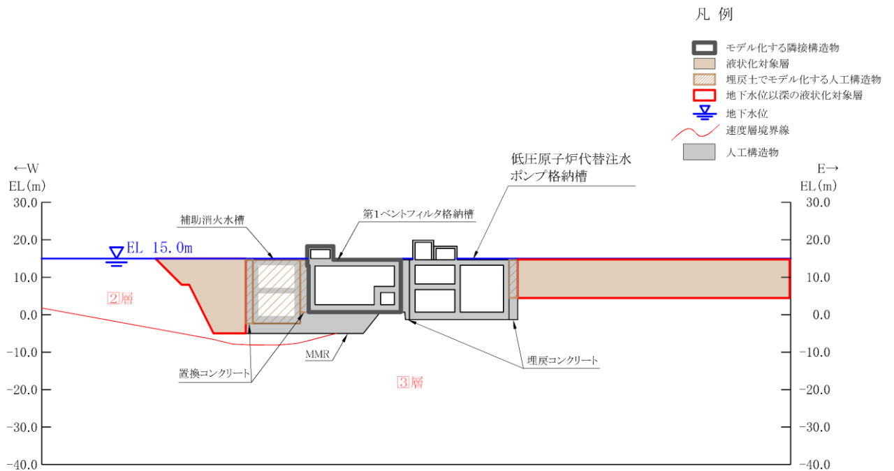
図 2-24 低圧原子炉代替注水ポンプ格納槽 断面図 (C-C 断面位置)
