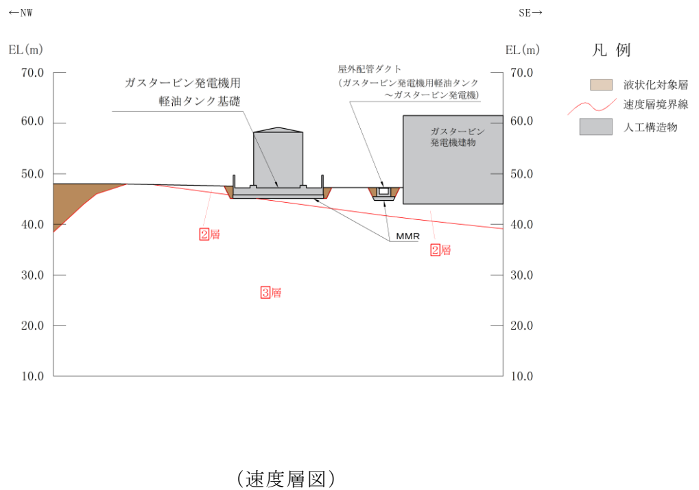
図 4.14—4 (2) ガスタービン発電機用軽油タンク基礎 地質断面図 (B—B 断面位置)
