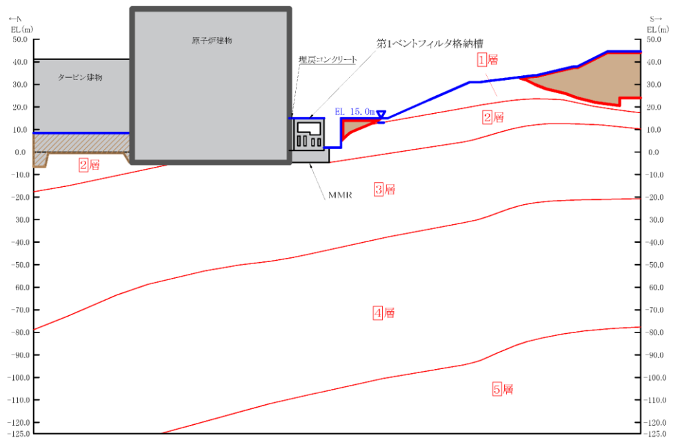
図 4.3-2(14) 第1ベントフィルタ格納槽 地質断面図 【B-B断面位置】 (②全応力解析)
