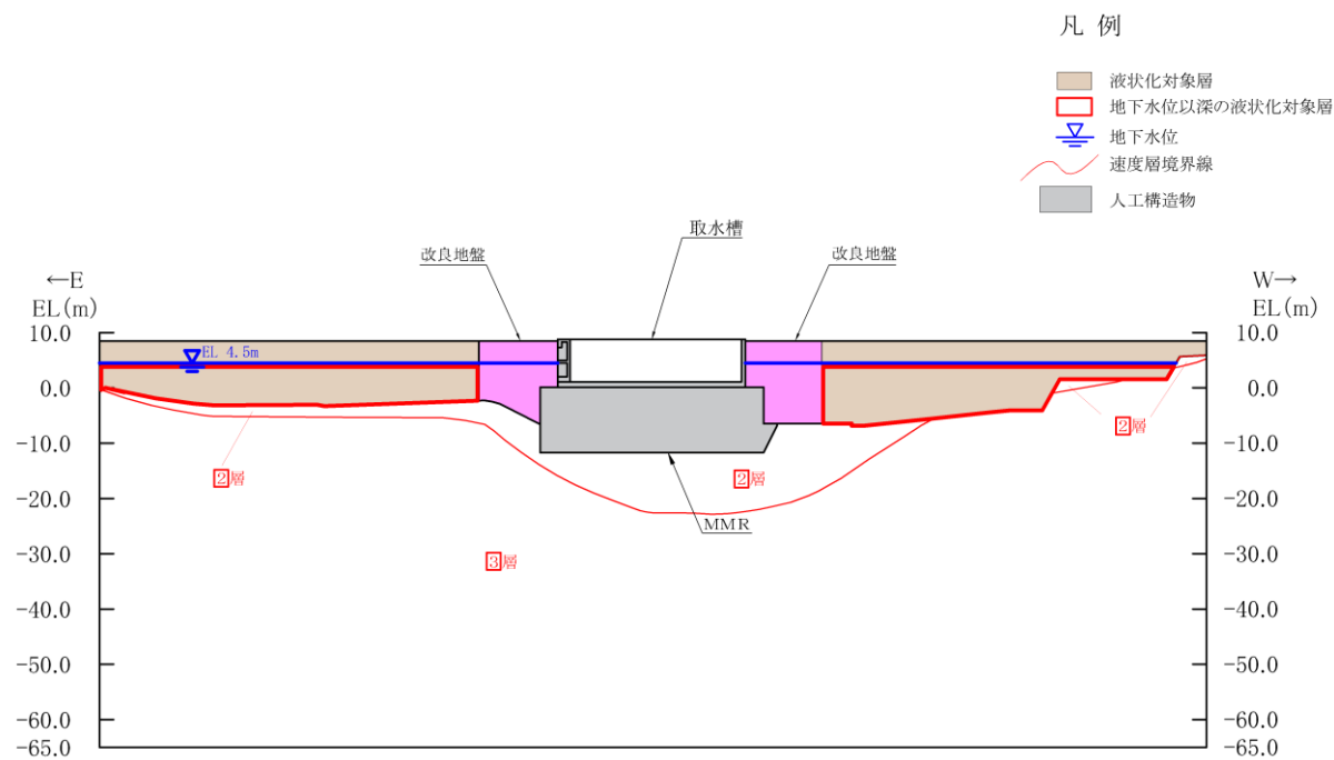
(速度層図)
