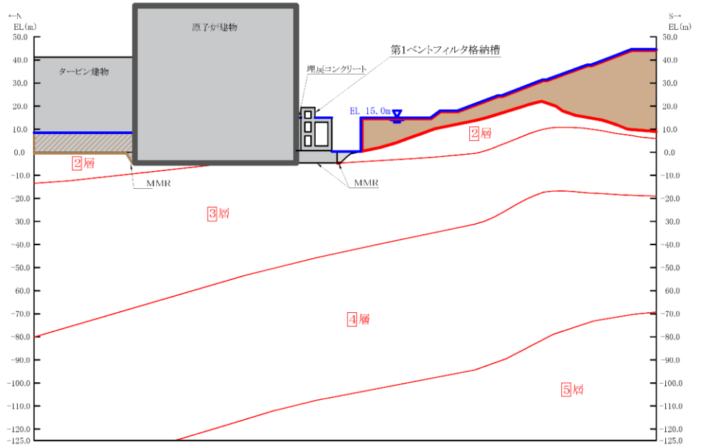
図 4.3-2(13) 第1ベントフィルタ格納槽 地質断面図 【A-A断面位置】 (②全応力解析)
