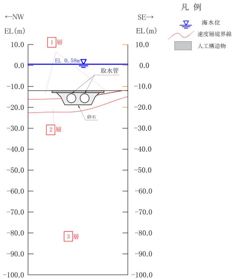
(速度層図)
