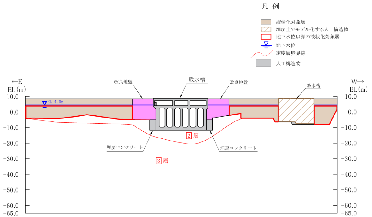
図 8.1-3(12) 埋戻土（非液状化）としてモデル化する場合の例
