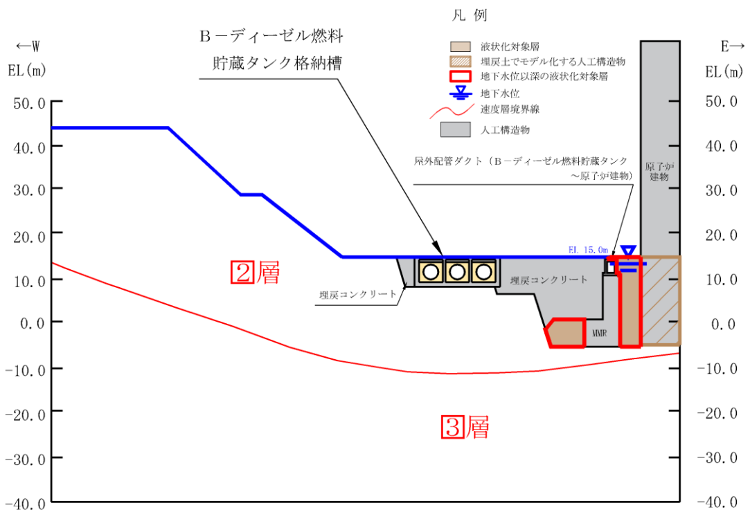
図 4.3-2(19) 屋外配管ダクト（タービン建物～放水槽）【B-B断面位置】 地質断面図（④全応力解析）
