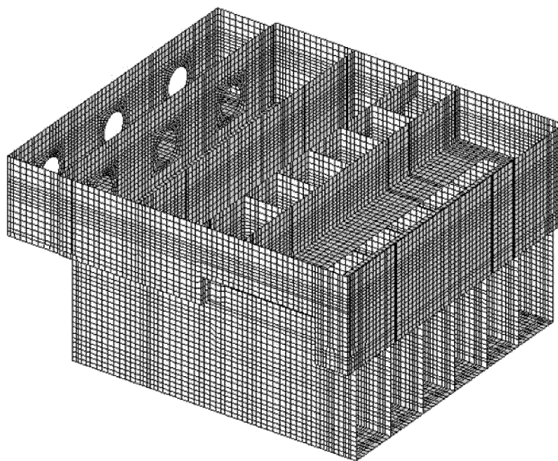
図 4.4-4 取水槽 3次元構造解析モデル
