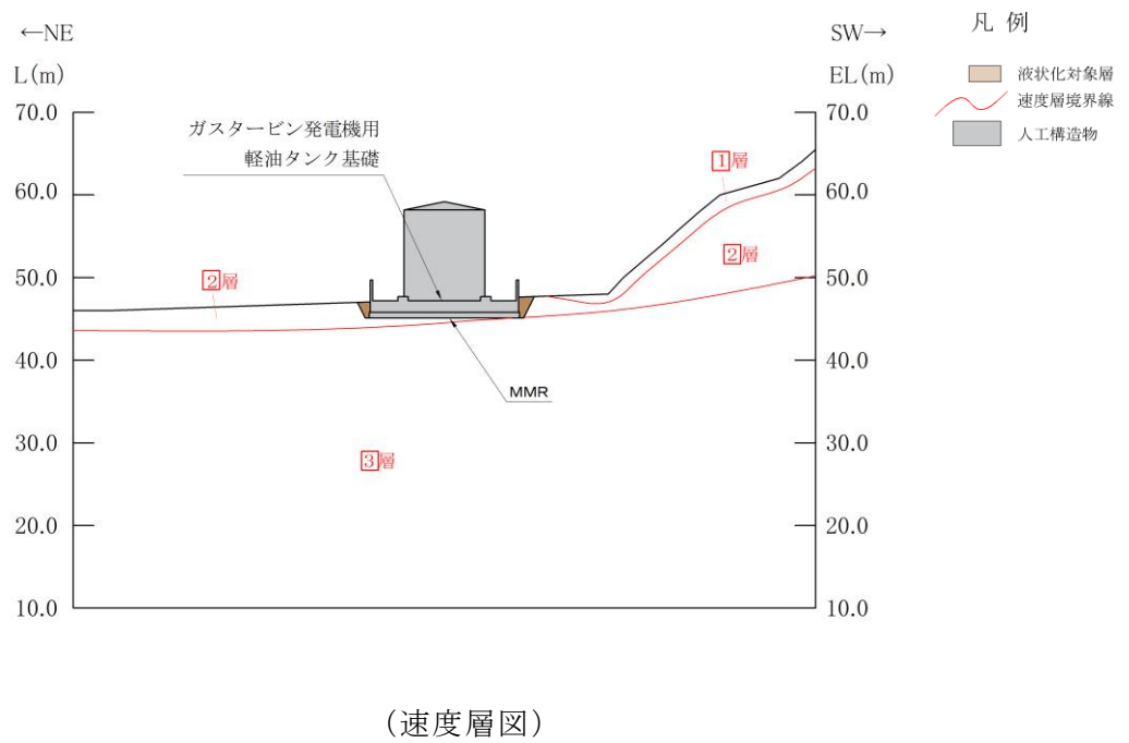
図 4.14-4 (1) ガスタービン発電機用軽油タンク基礎 地質断面図 (A-A断面位置)
