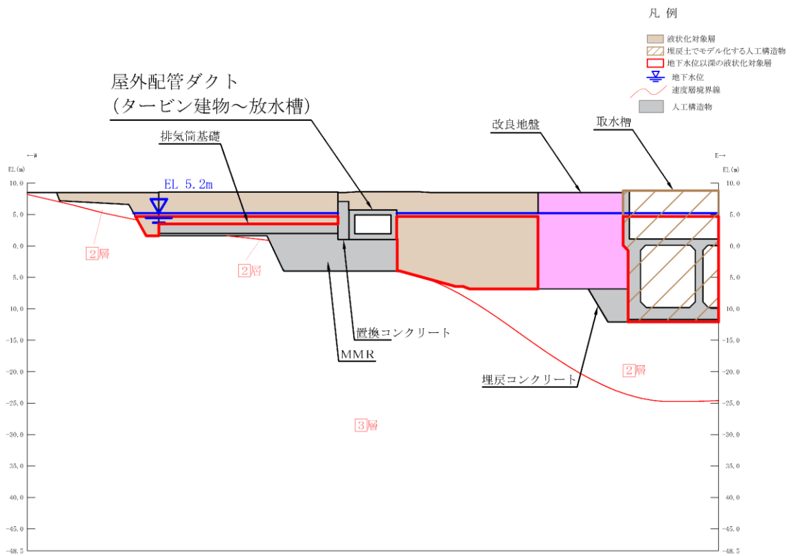
(速度層図)
