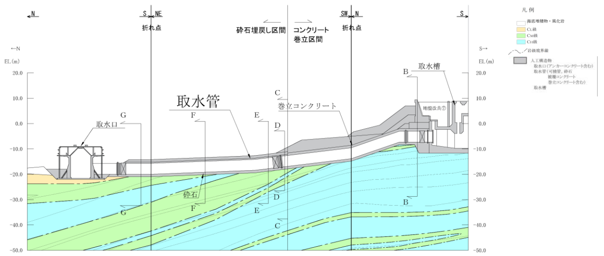
(岩級図)
