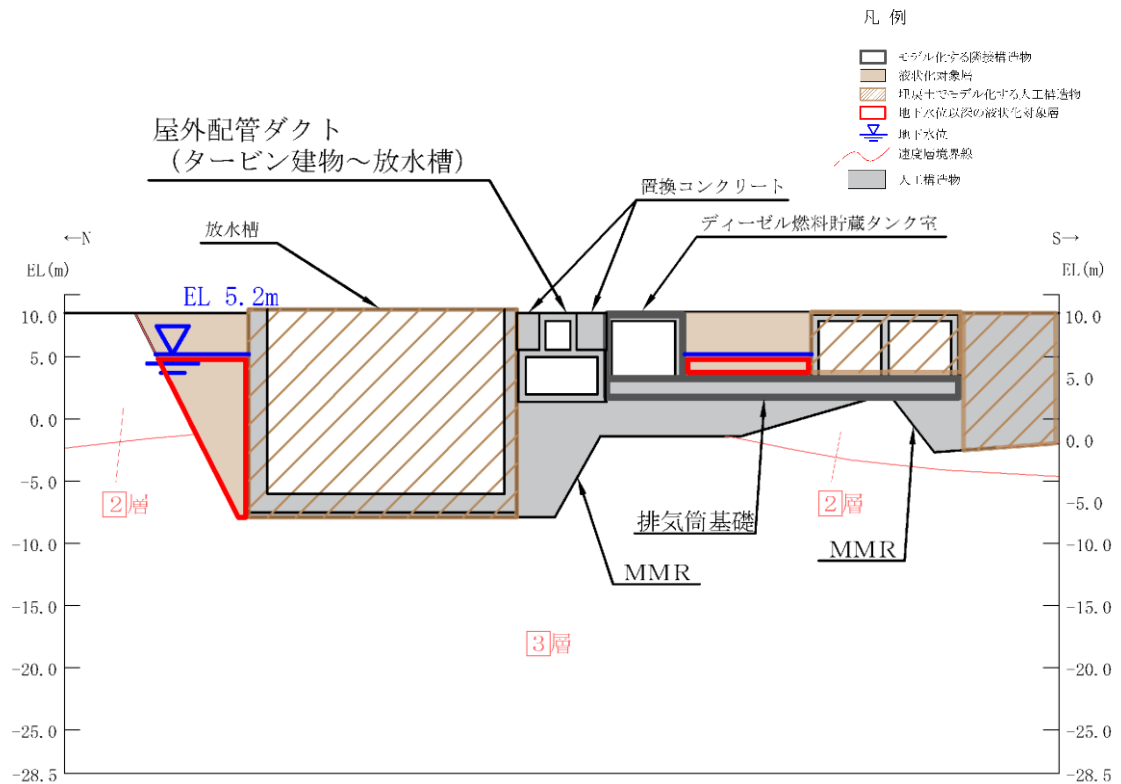
図 2-8 地質断面図 (屋外配管ダクト (タービン建物～放水槽) 【B-B 断面位置】) (参考) 9-9
