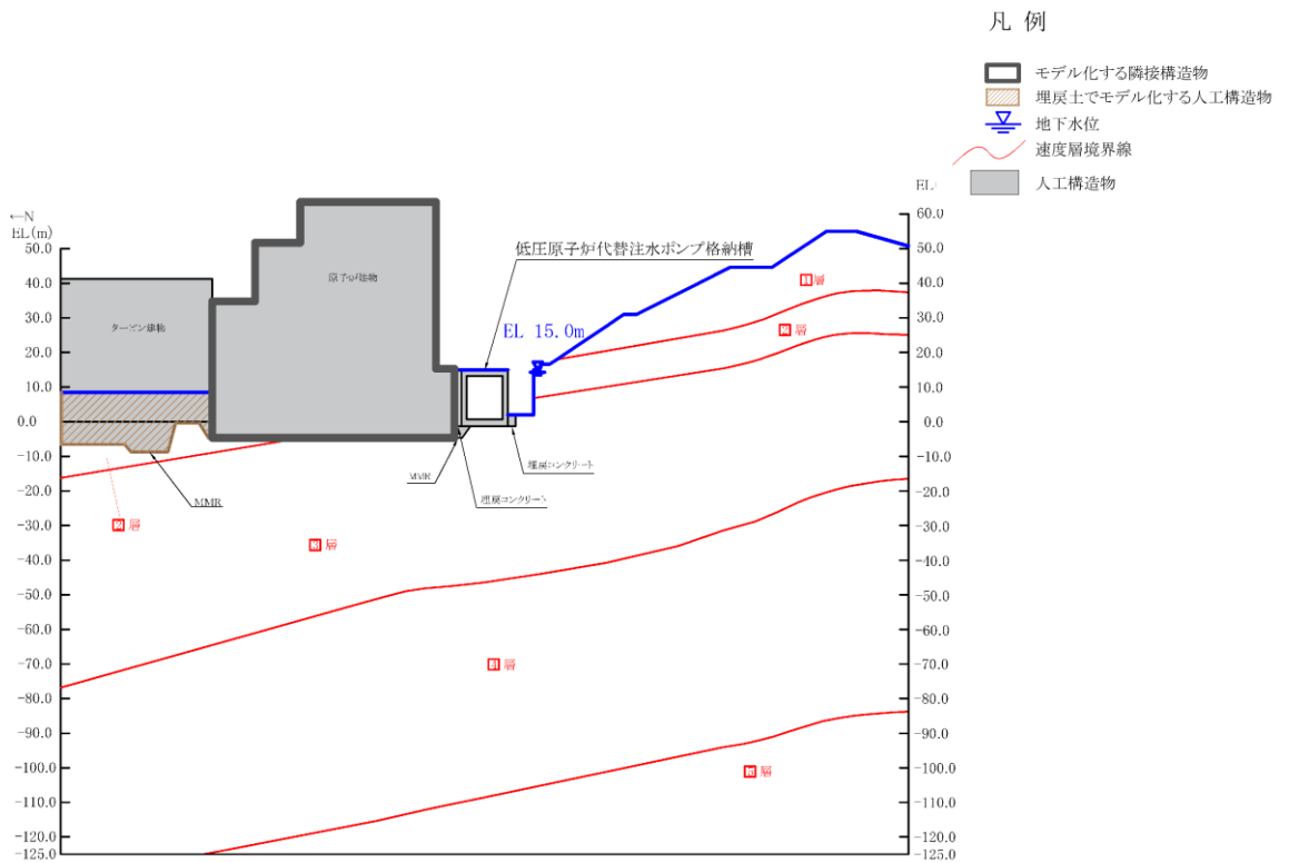
図 8.1-3(10) 隣接構造物としてモデル化する場合の例 (c) 原子炉建物：低圧原子炉代替注水ポンプ格納槽【B-B断面位置】
