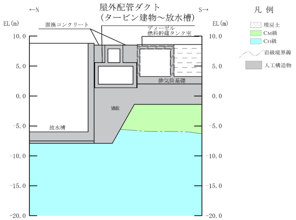
(岩級図)
