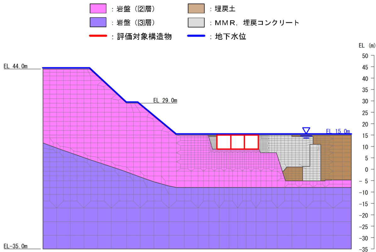
図 3-1 地震応答解析モデル図 (B-ディーゼル燃料貯蔵タンク格納槽 A-A断面)
