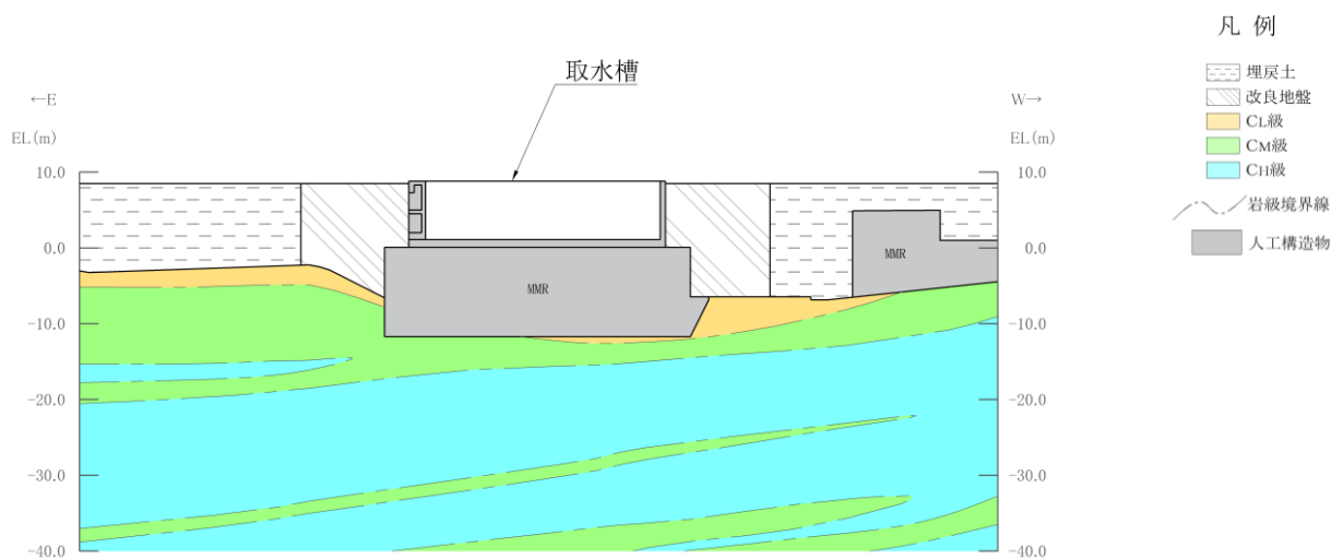
(岩級図)
