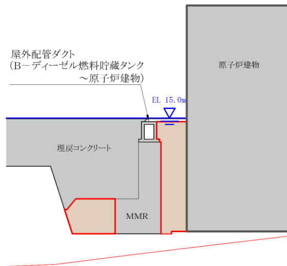
(全体図)
