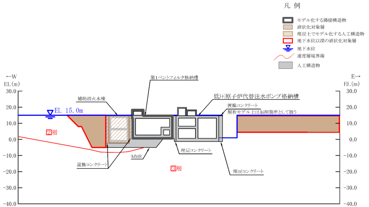
図 8.1-3(11) 隣接構造物としてモデル化する場合の例
