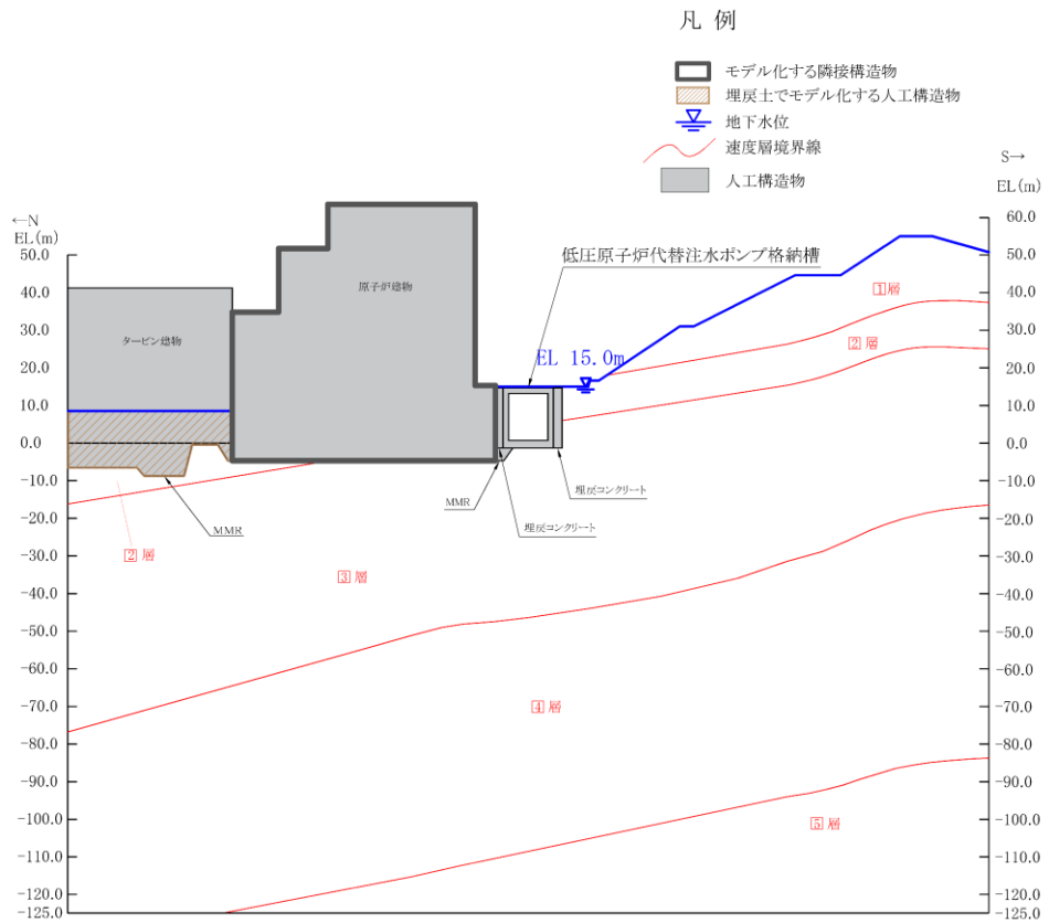
(速度層図)
