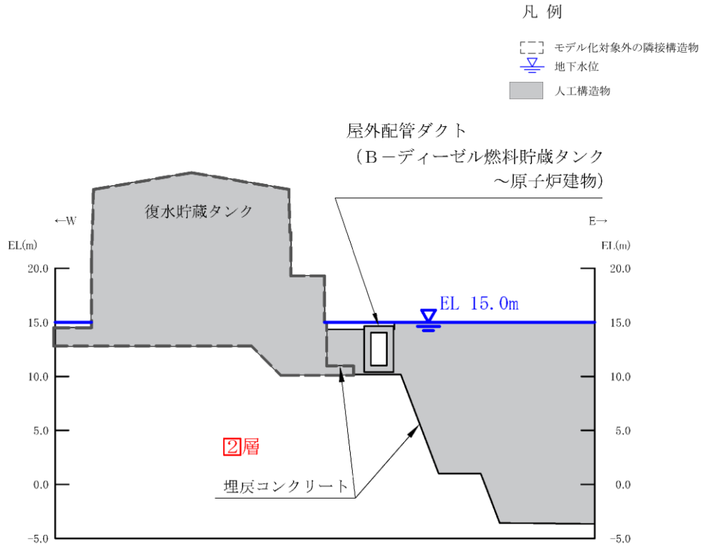
図 4.3-2(11) 屋外配管ダクト (B-ディーゼル燃料貯蔵タンク～原子炉建物) 【A-A断面位置】 地質断面図 (②全応力解析)
