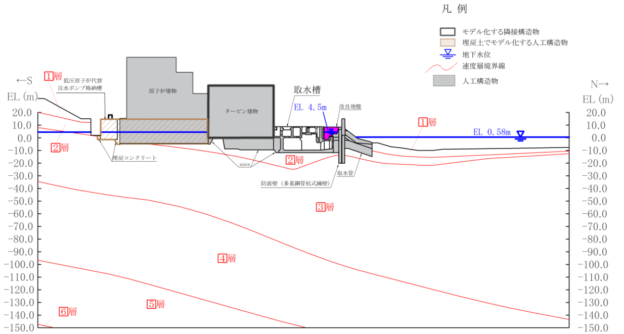
(速度層図)
