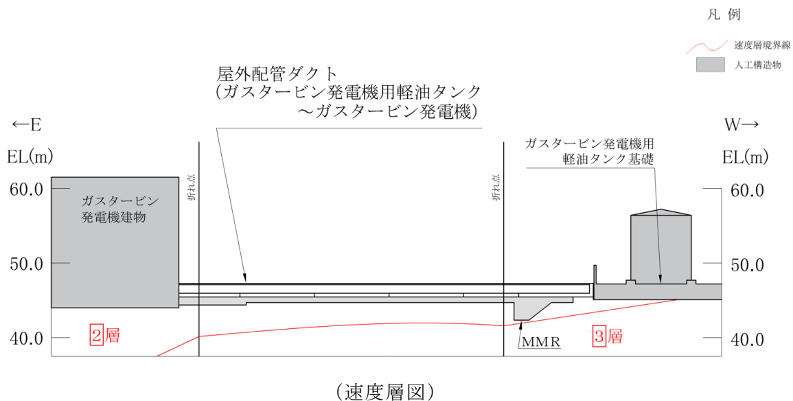
図 4.15-4 (2) 屋外配管ダクト (ガスタービン発電機用軽油タンク～ガスタービン発電機) 地質断面図 (B-B 断面位置)
