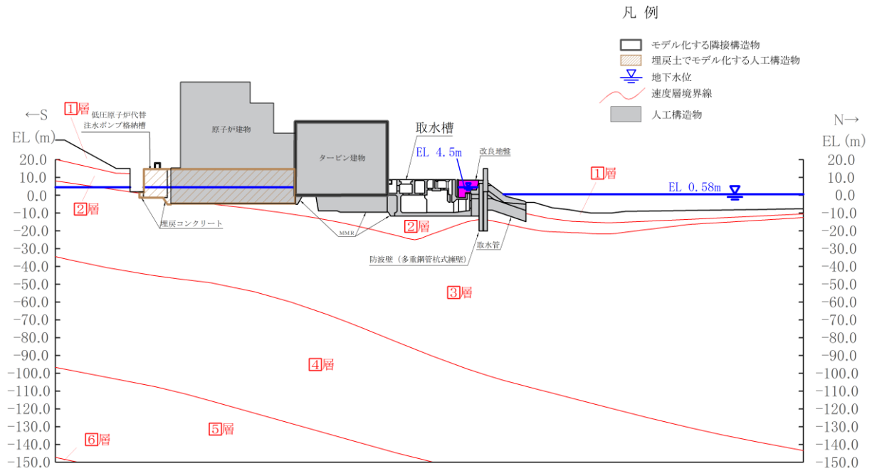
図 8.1-3(1) 隣接構造物としてモデル化する場合の例 (a) タービン建物：取水槽【D-D断面位置】
