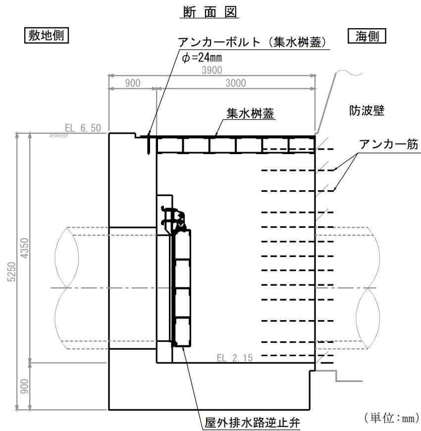
図 6-2(1) 集水樹 (防波壁部, 屋外排水路逆止弁①) 構造図
