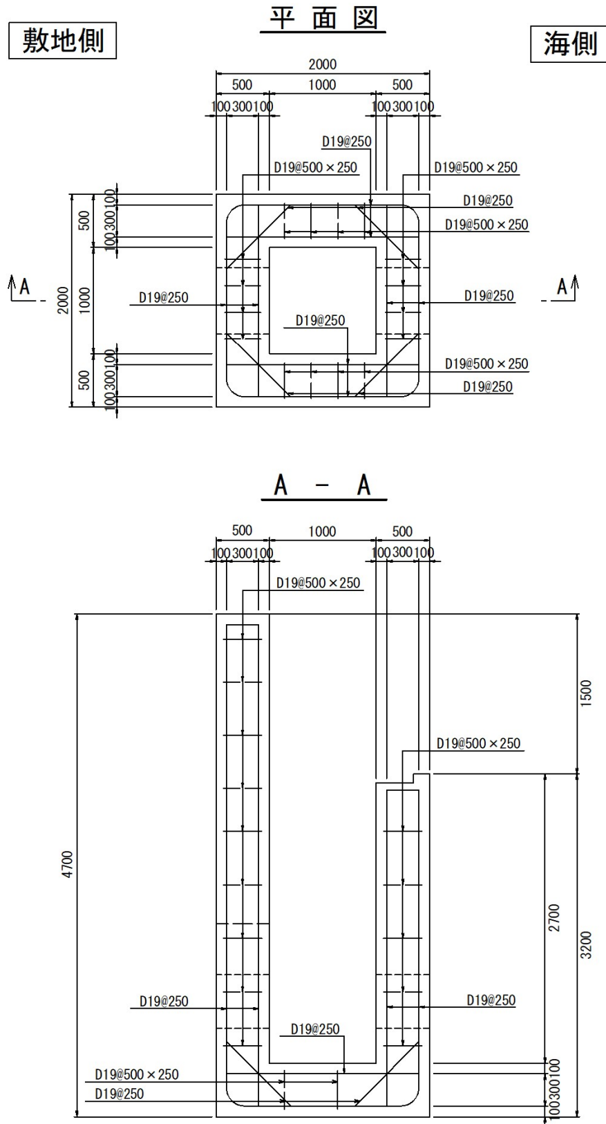
図 8-1(4) 概略配筋図 (集水 枿 (屋外排水路逆止弁⑧-1))
