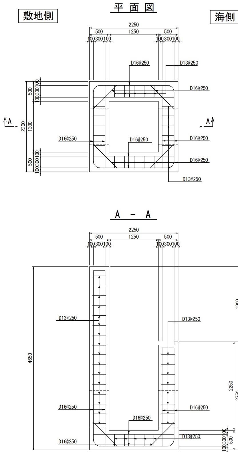
図 8-1(7) 概略配筋図 (集水枿 (屋外排水路逆止弁⑩))
