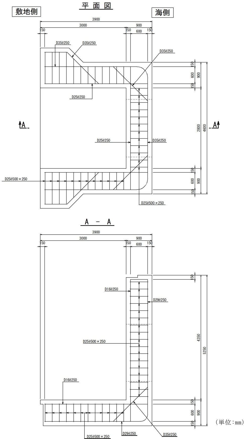
図 8-1(1) 概略配筋図 (集水枿 (屋外排水路逆止弁①))
