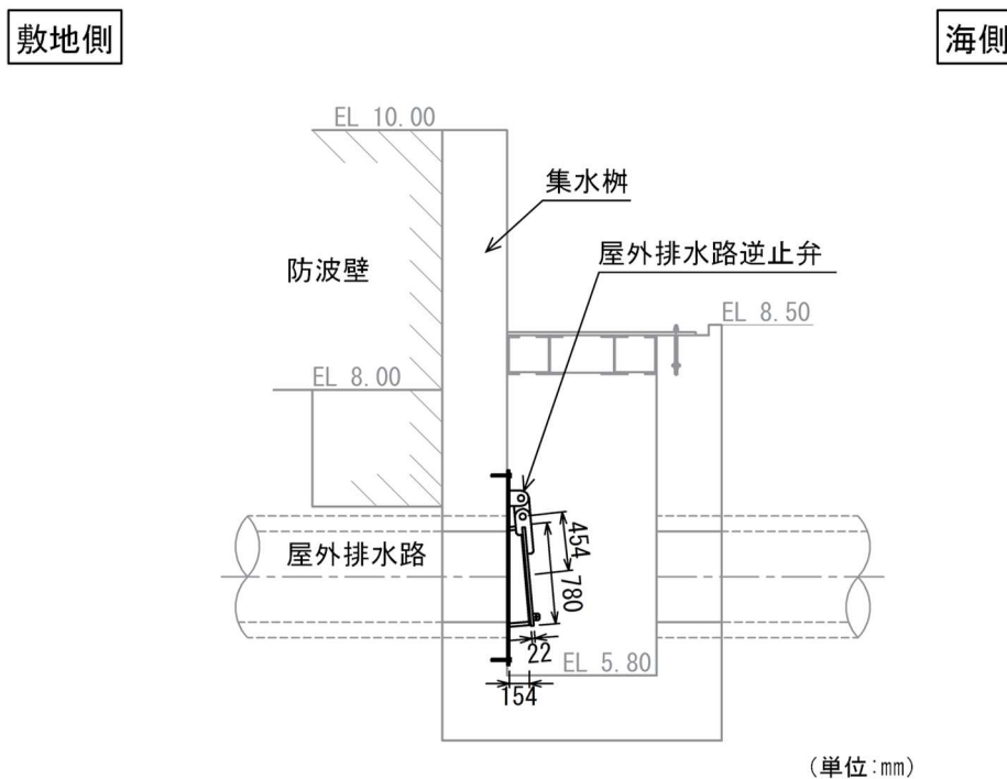
図 2-4(2) 屋外排水路逆止弁⑦の構造概要
