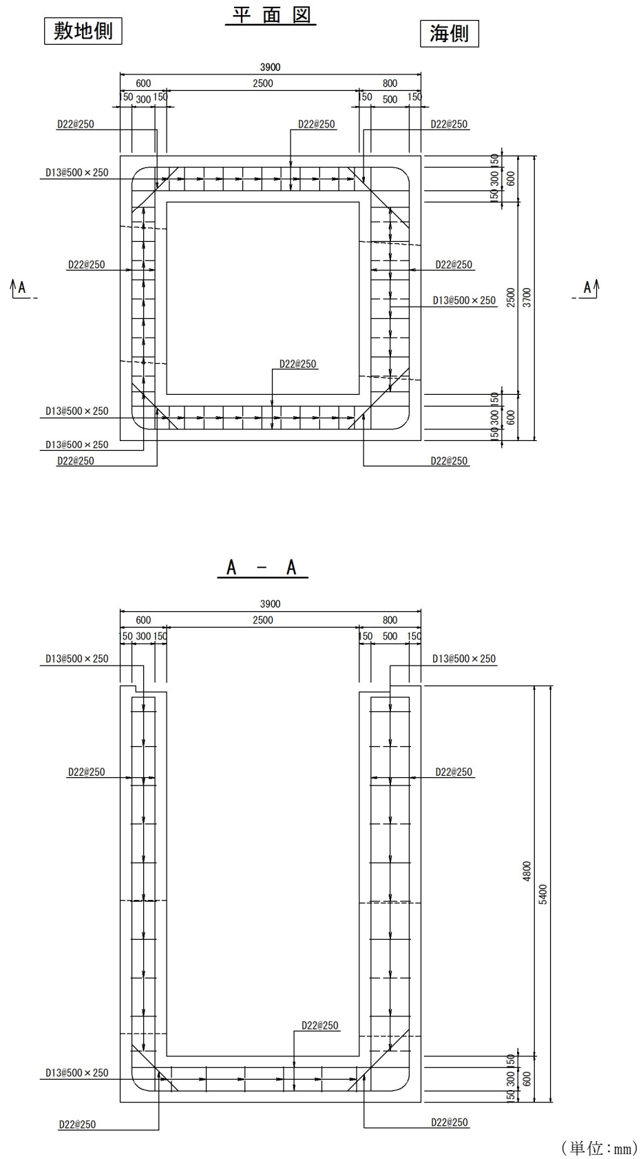
図 8-1(10) 概略配筋図 (集水枡 (屋外排水路逆止弁⑬))
