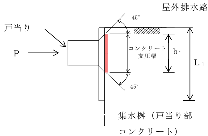
図4-7 集水桝(戸当り部コンクリート)のモデル図
