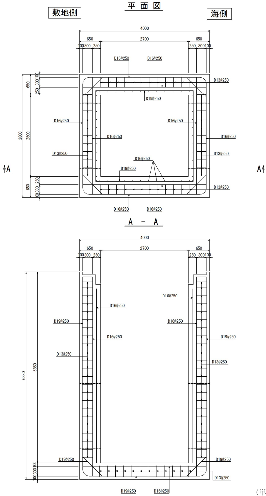
図 8-1(6) 概略配筋図 (集水桝 (屋外排水路逆止弁⑨))
