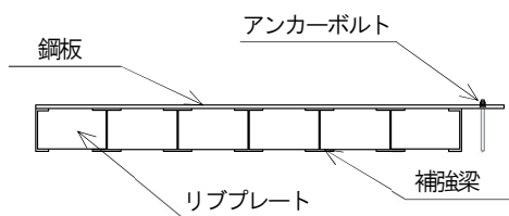
側面図
