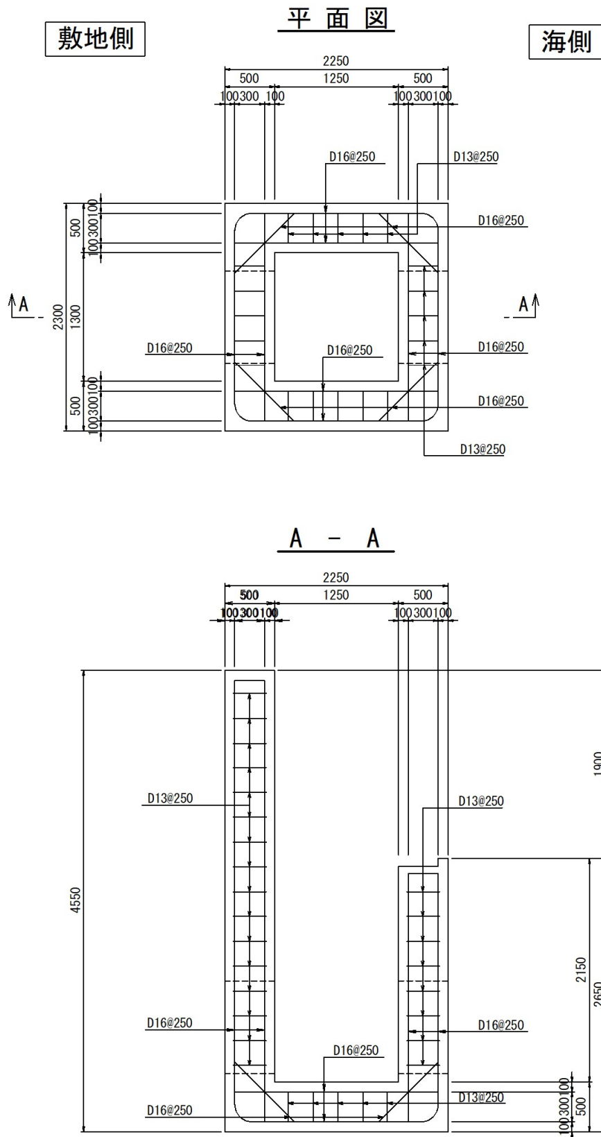
図 8-1(9) 概略配筋図 (集水枿 (屋外排水路逆止弁⑫))
