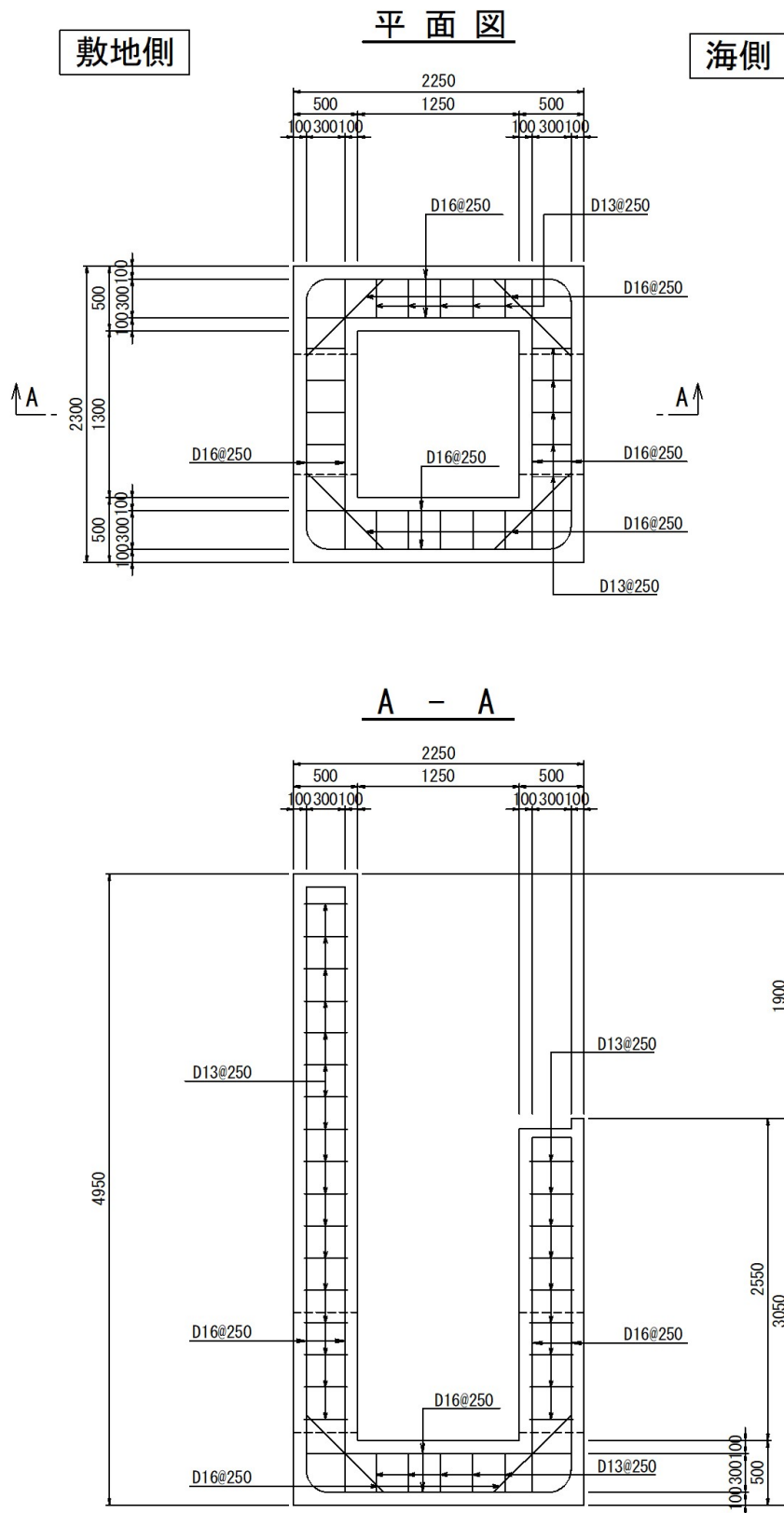
図 8-1(8) 概略配筋図 (集水枿 (屋外排水路逆止弁①))
