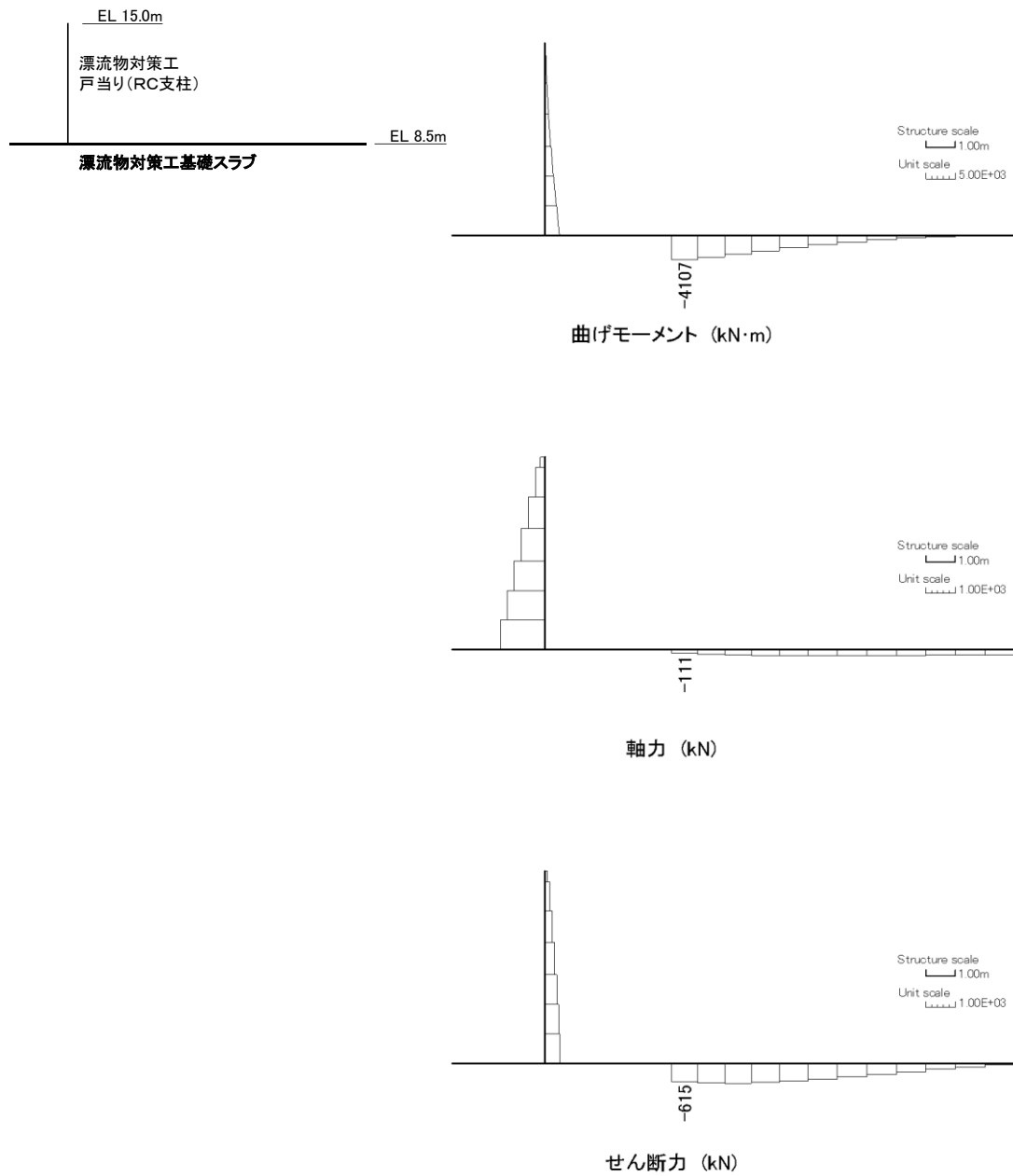
図 6.3-3(2) 鉄筋の曲げ・軸力系の破壊に対する照査における 最大照査値の評価時刻での断面力 (S s -D (+-) , 解析ケース①, t=32.48s)
