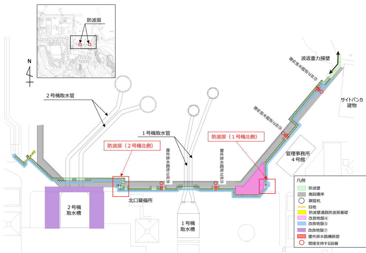
図 2.2-1 防波扉設置位置
