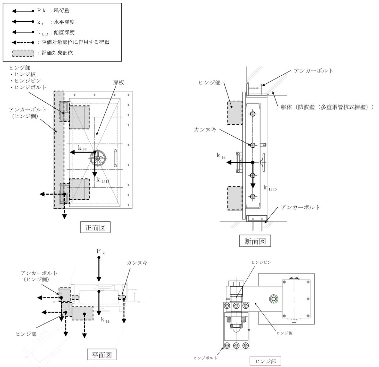
図 4.1-1 防波扉（1号機北側）及び防波扉（2号機北側）閉止時に作用する荷重の作用図
