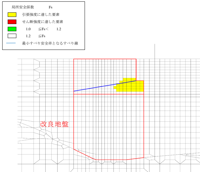
図 6.2-5 改良地盤の最小すべり安全率時刻における局所安全係数分布 ( S_s - N1 (-+) , 解析ケース①, t=7.56s )
