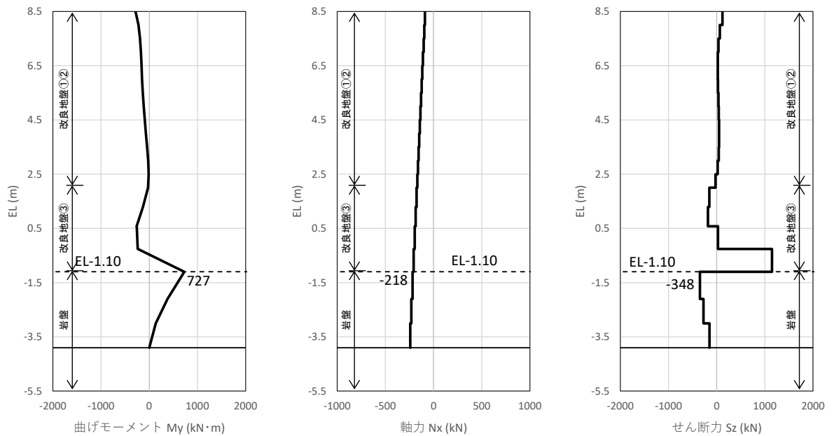
図 6.2-3 防波扉（鋼管杭）の曲げ・軸力系の破壊に対する照査における 最大照査値の評価時刻での断面力
