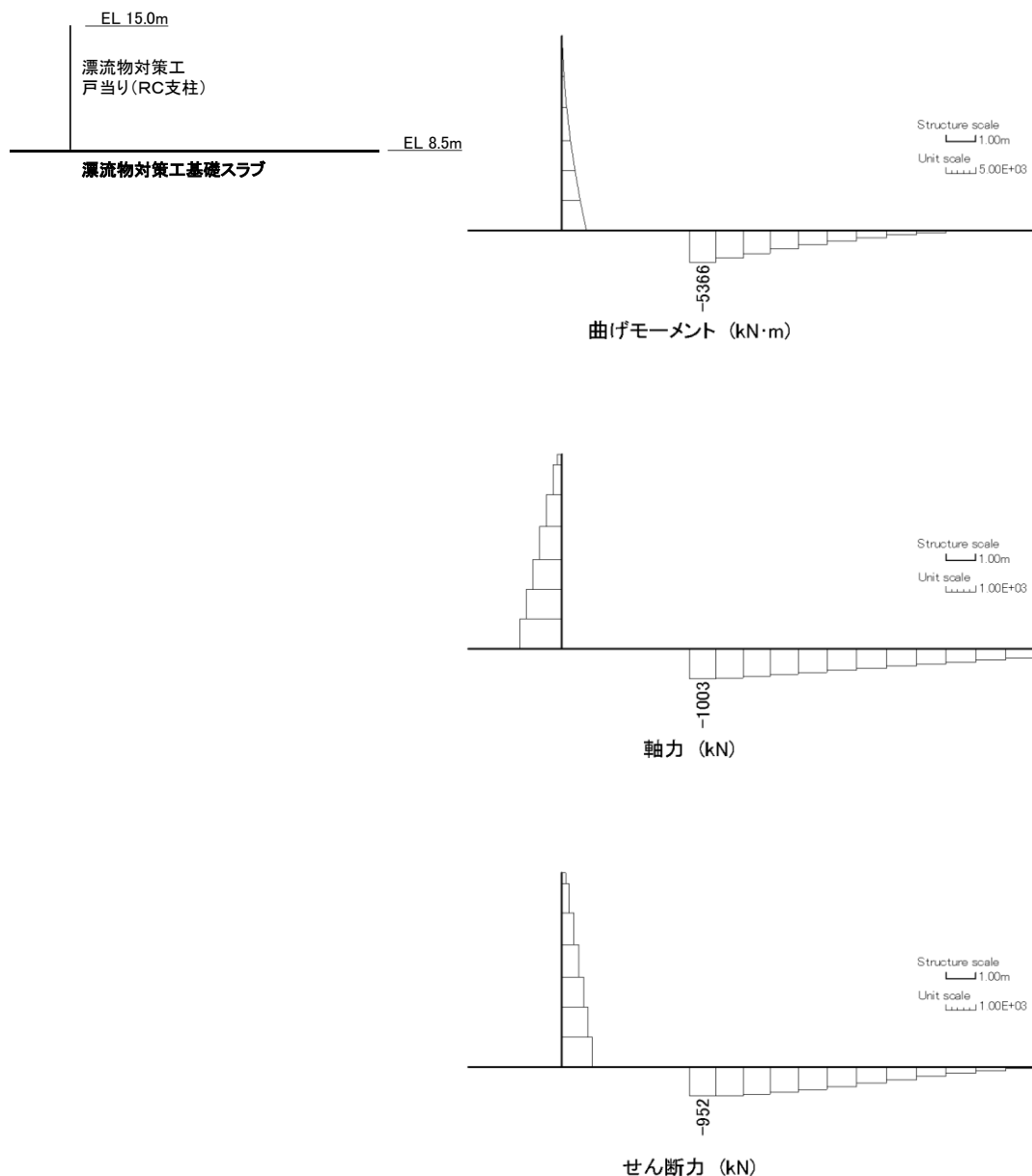
図 6.3-3(1) コンクリートの曲げ・軸力系の破壊に対する照査における最大照査値の評価時刻での断面力 (S s - D (+ -) , 解析ケース①, t=8.59s)
