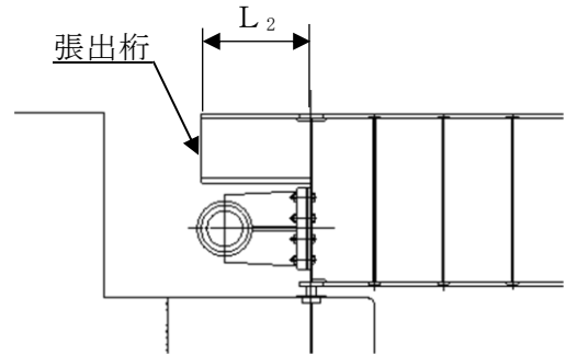
(扉体平面図)
