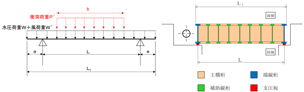
(扉体平面図)
