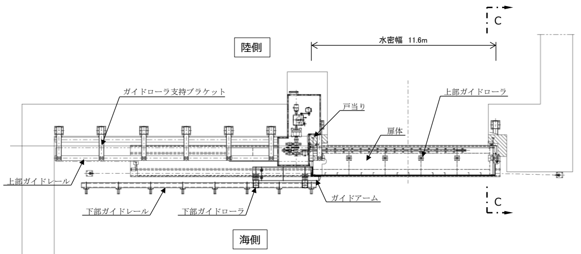
図 2.2-3(2) 防波扉の構造図 (鋼製扉体平面図, B-B 断面)
