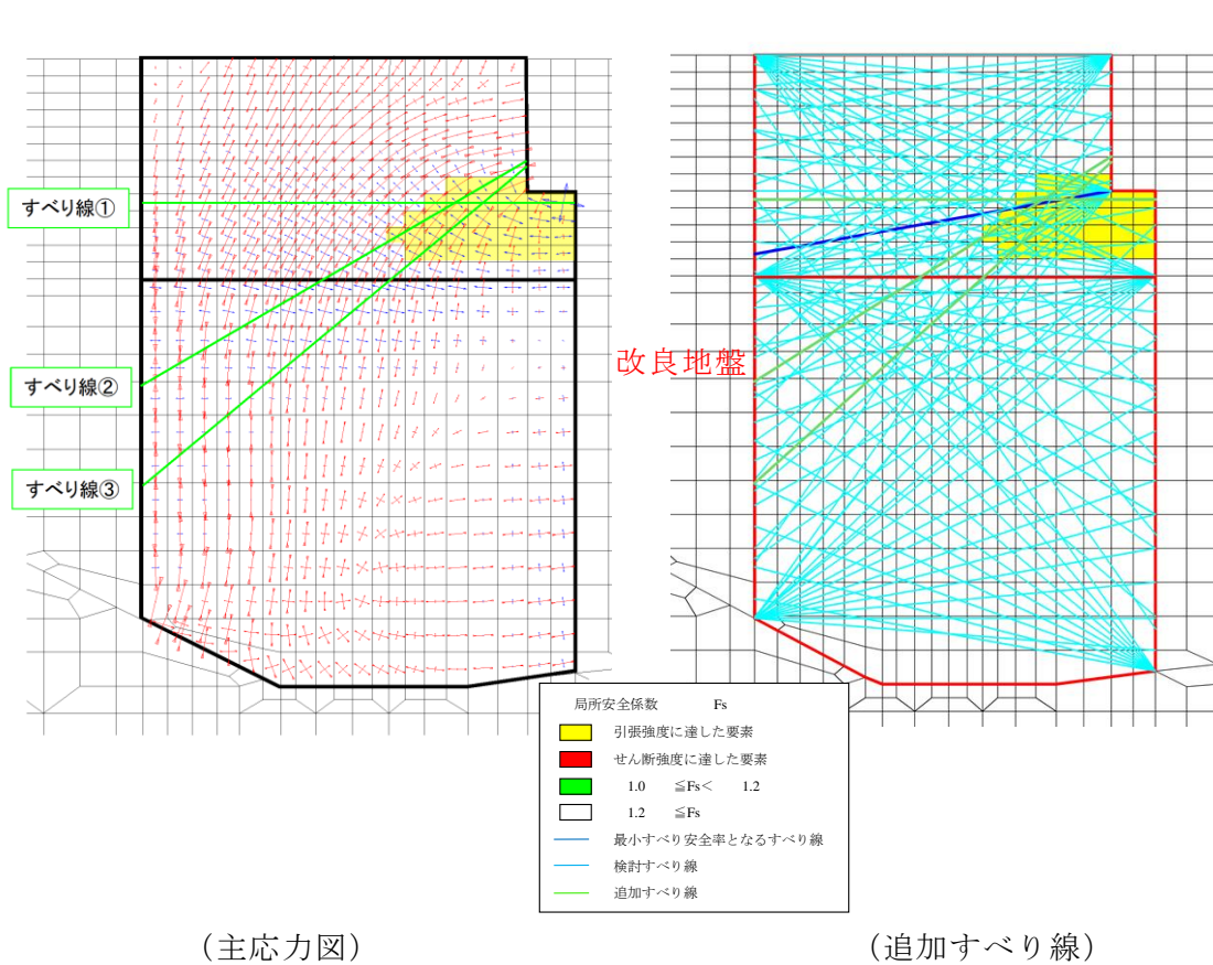
図 6.2-8 改良地盤の最小すべり安全率時刻における主応力図及び追加すべり線 ( S_s - N1 (-+) , 解析ケース①, t=7.56s )
