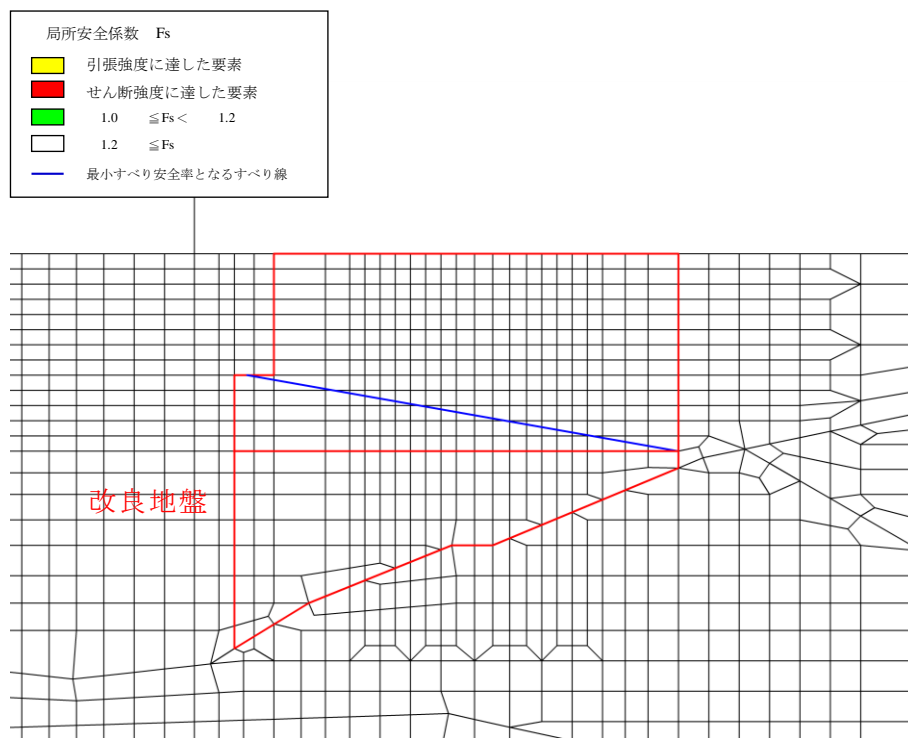
図 5.1-3 改良地盤の局所安全係数分布
