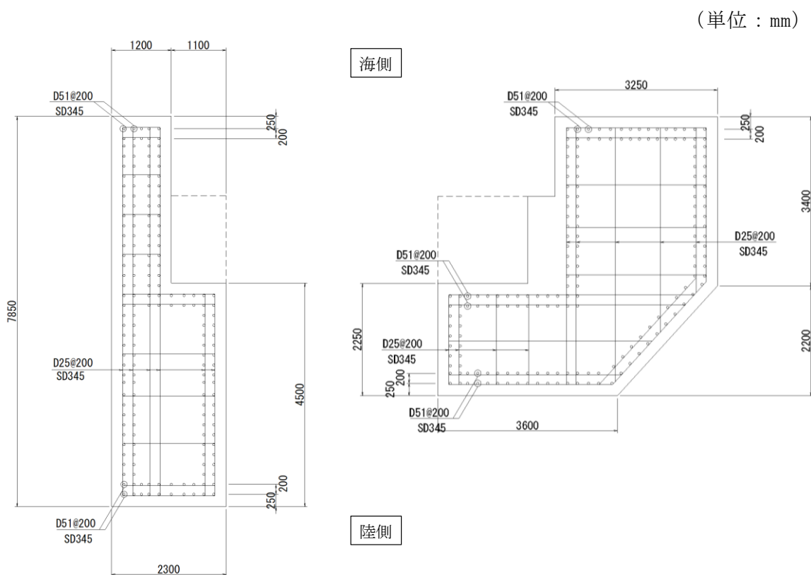
図 2.2-9(1) 漂流物対策工戸当り (RC支柱) の概略配筋図 (A-A断面)
