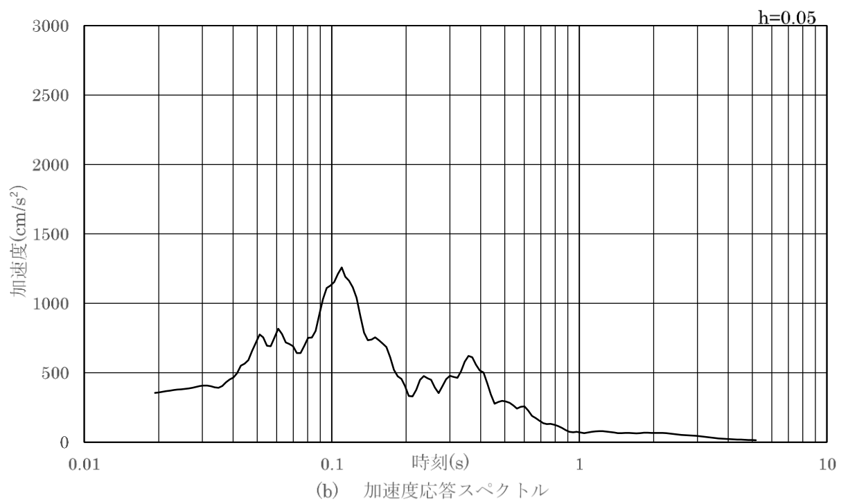
図 4.5-9 入力地震動の加速度時刻歴波形及び加速度応答スペクトル (鉛直成分：S s - N 1)
