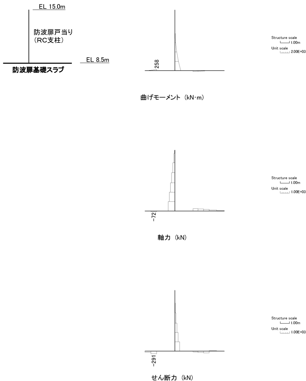
図 5.1-2(1) コンクリートの曲げ・軸力系の破壊に対する照査及びせん断照査における断面力
