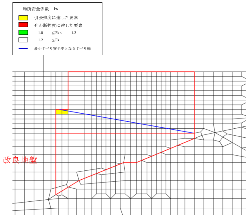
図 6.2-5 改良地盤の最小すべり安全率時刻における局所安全係数分布 ( S_s - D(-+) , 解析ケース①, t = 8.58s )
