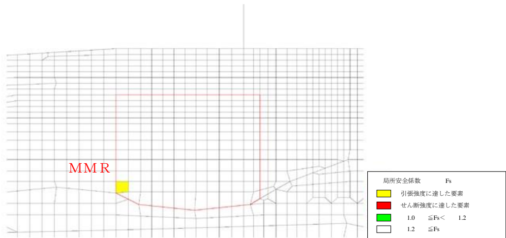
図 6.3-6(5) MMRの引張応力最大時刻の局所安全係数
