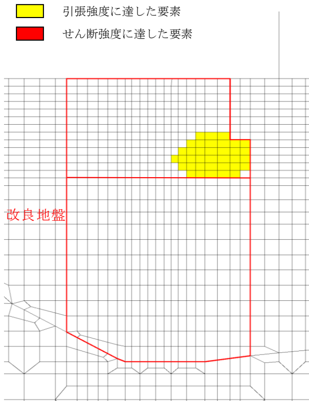
図 6.2-7 全時刻における破壊履歴図 ( S_s - N_1 (一十), 解析ケース①)
