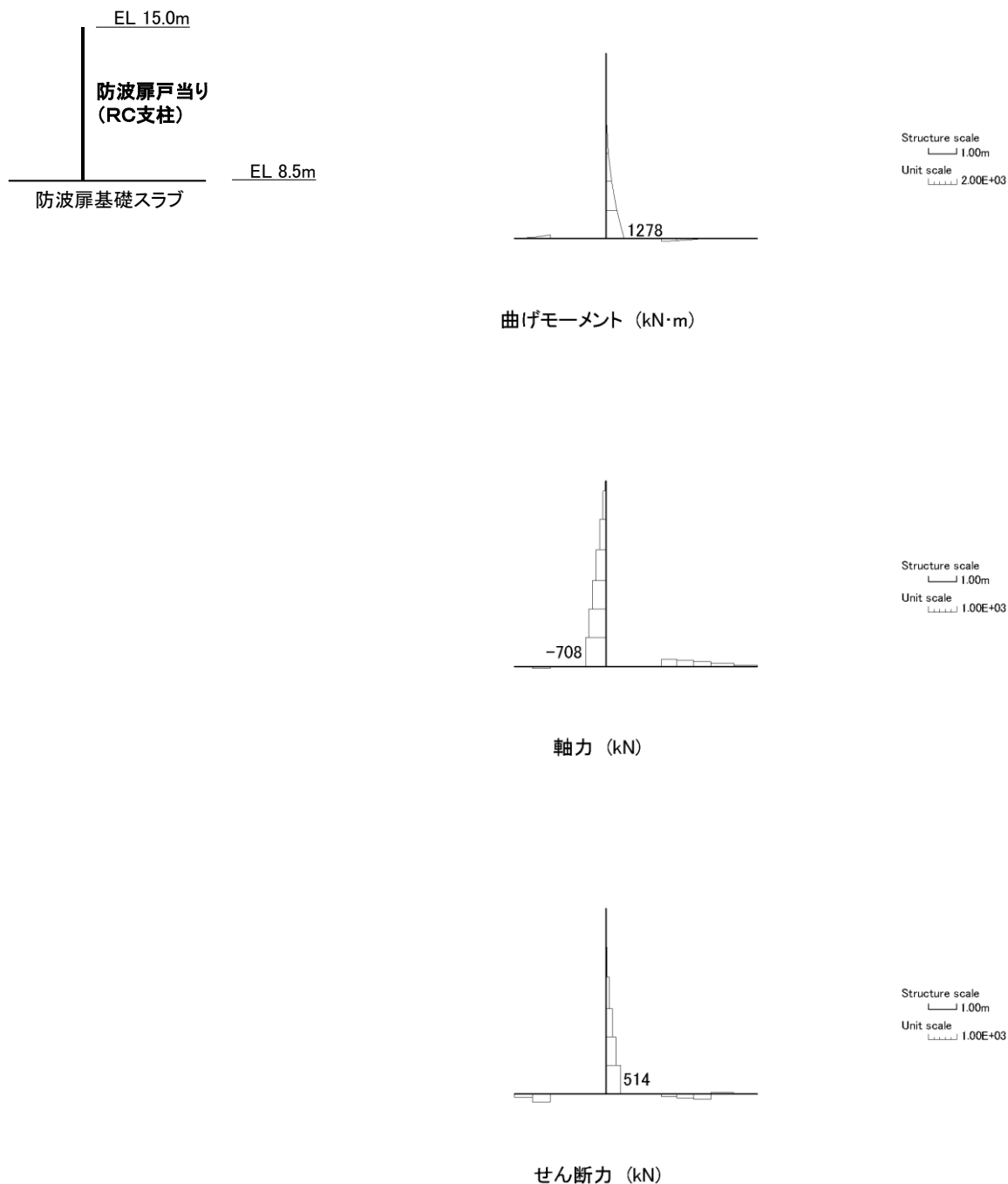
図 5.1-1 コンクリート及び鉄筋の曲げ・軸力系の破壊に対する照査及びせん断照査における断面力 2.2.6-91
