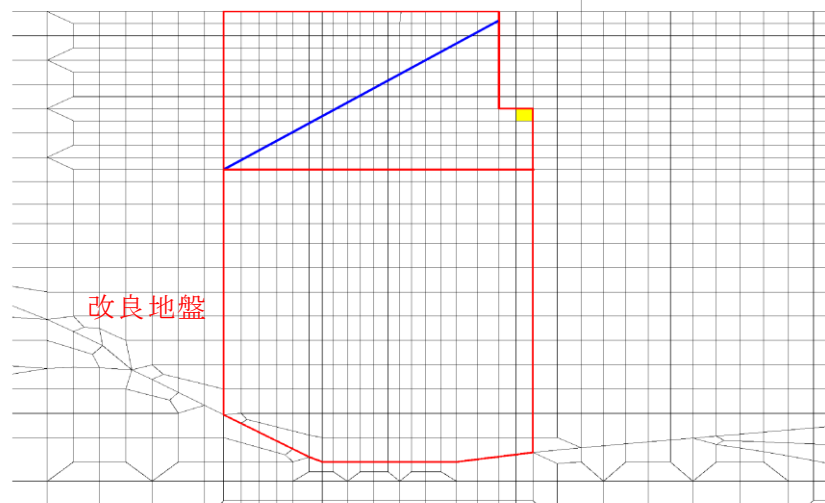
図 5.1-3 改良地盤の局所安全係数分布
