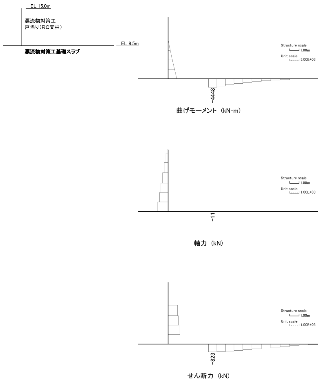
図 5.2-2 コンクリート及び鉄筋の曲げ・軸力系の破壊に対する照査及びせん断照査における断面力
