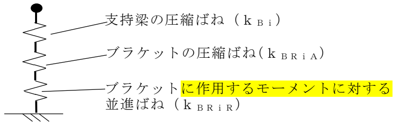
図 4-2 水平方向 (EW方向) のばねモデル
