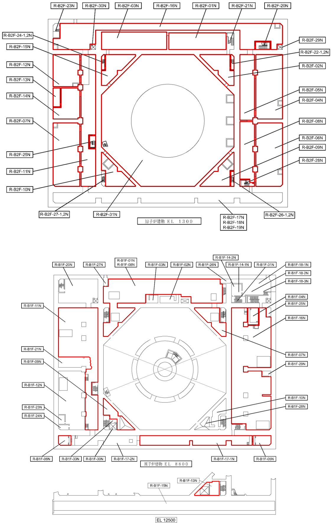
図 2-1 溢水防護区画 (1/14)
