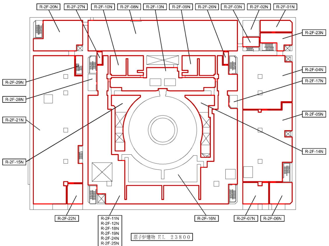
図 2-1 溢水防護区画 (2/14)
