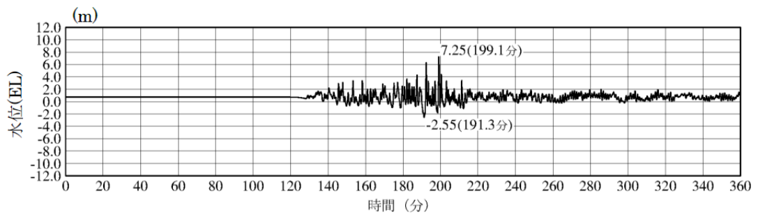
3号機放水槽（入力津波5，防波堤無し）
