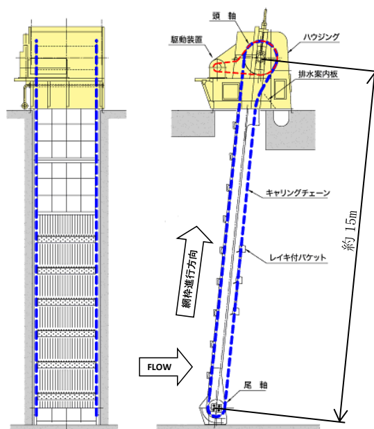
図 3-39 除じん機の概要
