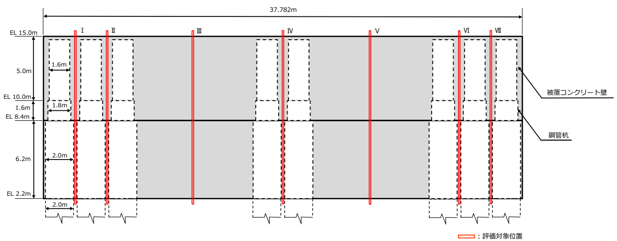
図 5.2.1-1(6) 評価対象位置図 (④-④断面 正面図)
