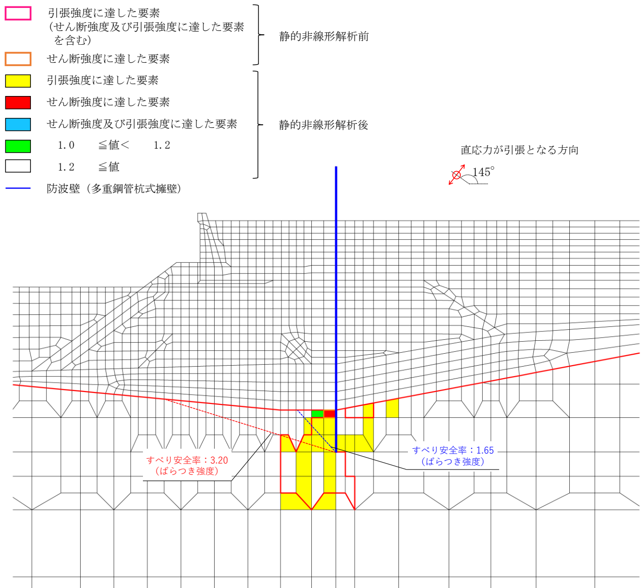
図 4.2.9-11 静的非線形解析による鋼管杭周辺岩盤の局所安全係数分布図 (②-②断面) (S s - D (-+), 解析ケース②, t=15.04s, 鋼管杭の曲げ・軸力系の破壊に対する照査 における最大照査値発生時刻)
