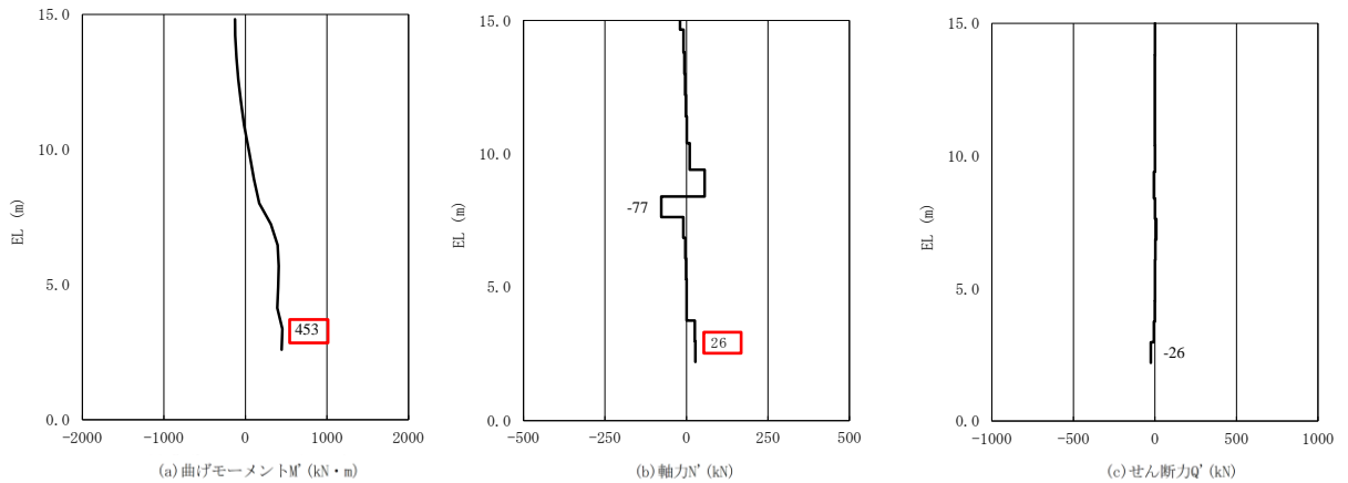
図 5.2.2-2(2) 鉄筋の曲げ・軸力系の破壊に対する照査に用いる断面力 (③-③断面, S_s - D(-+) , 評価対象位置Ⅳ)
