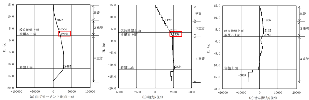
図 2.1-2(2) 3重管部の鋼管杭の曲げ・軸力系の破壊に対する照査 における最大照査値の評価時刻での断面力 (③-③断面, S s - D (-+), t=9.55s , 3重管部)
