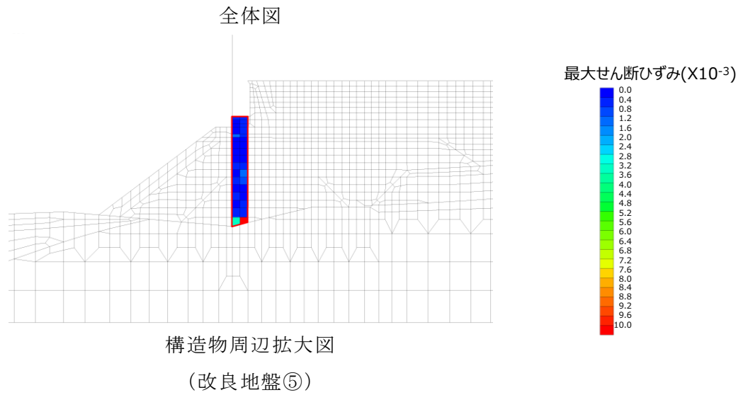
図 4.2.6-1(2) ③-③断面の最大せん断ひずみ分布 (解析ケース②, S_s - D (-+))
