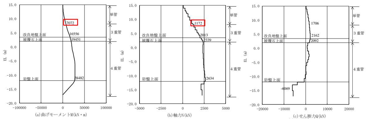
図 2.1-2(1) 単管部の鋼管杭の曲げ・軸力系の破壊に対する照査 における最大照査値の評価時刻での断面力 (③-③断面, S s - D (-+), t=9.55s , 単管部)
