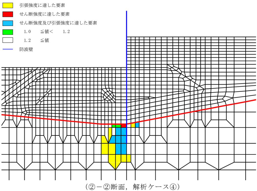
図 4.2.12-13 解析ケース②及び解析ケース④における 鋼管杭根入れ部周辺の岩盤の破壊領域の比較 (2-2)断面)
