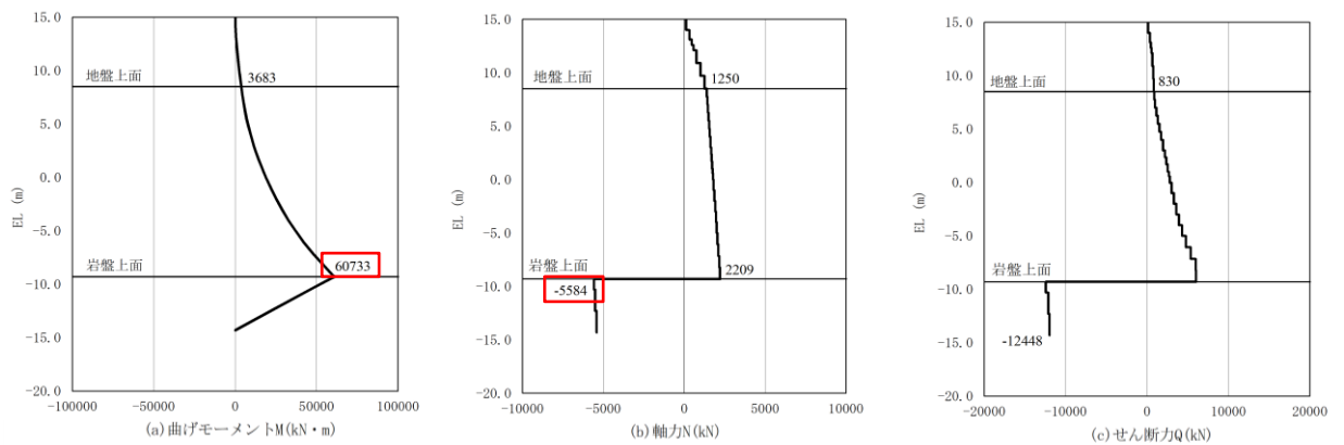
(一般部 (①-①断面), S s - D (-+), t=13.19s)
