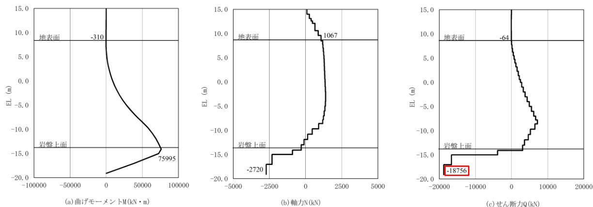
図 4.2.3-1(1) 鋼管杭のせん断破壊に対する照査における 最大照査値の評価時刻での断面力 (②-②断面, S_s - D(-+) , t=15.04s )
