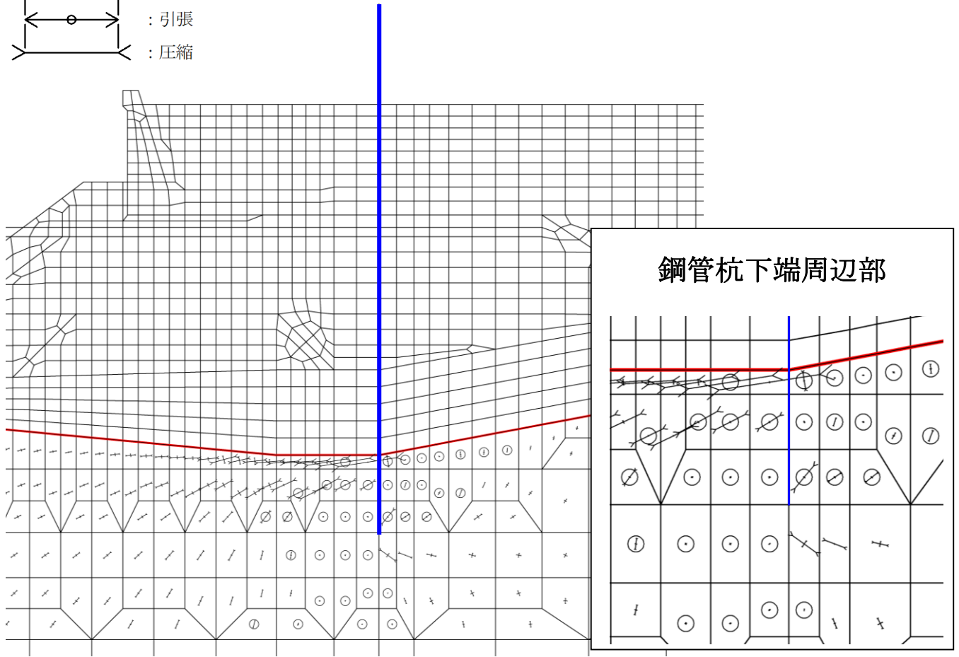
図 4.2.9-12 静的非線形解析による鋼管杭周辺岩盤の主応力図 (②-②断面)
