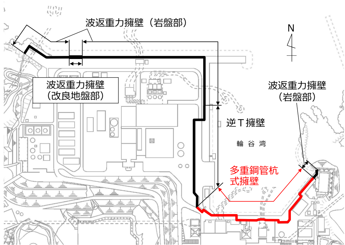
図 2.1-1 防波壁（多重鋼管杭式擁壁）の位置図
