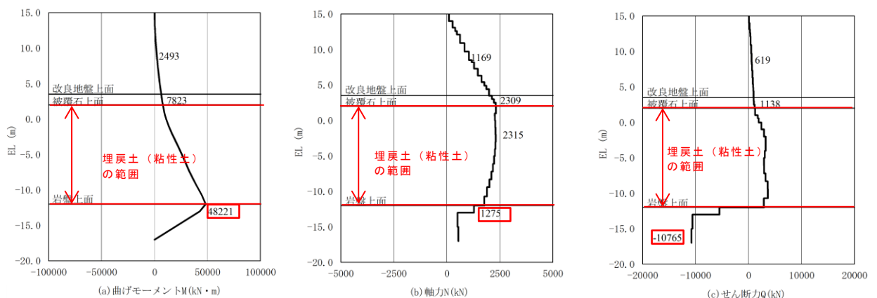
図 6.2.3-2 鋼管杭の曲げ・軸力系の破壊に対する照査における最大照査値の評価時刻での断面力
