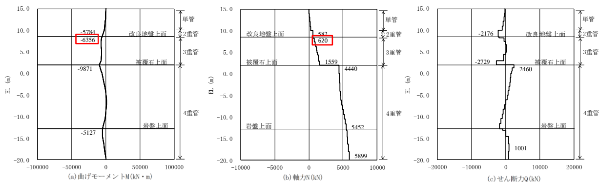
図 2.1-3(2) 2重管部の鋼管杭の曲げ・軸力系の破壊に対する照査 における最大照査値の評価時刻での断面力
