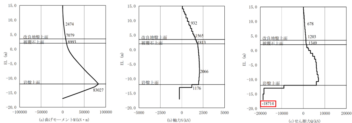
図 4.2.3-1(2) 鋼管杭のせん断破壊に対する照査における 最大照査値の評価時刻での断面力 (③-③断面, S_s - D(-+) , t=13.21s )
