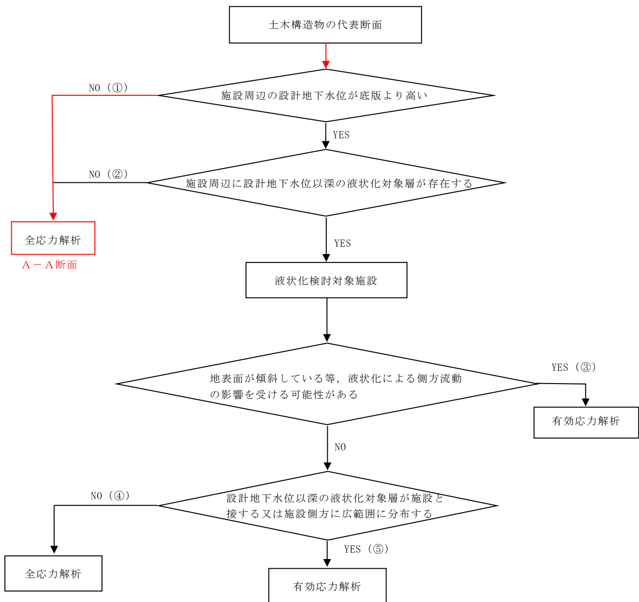
図 2-10 解析手法の選定フロー
