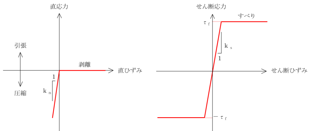
図 2-18 ジョイント要素の力学特性
