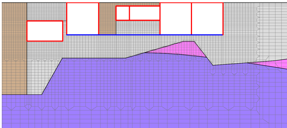
図 2-17 地震応答解析モデル図 (A-A 断面)
