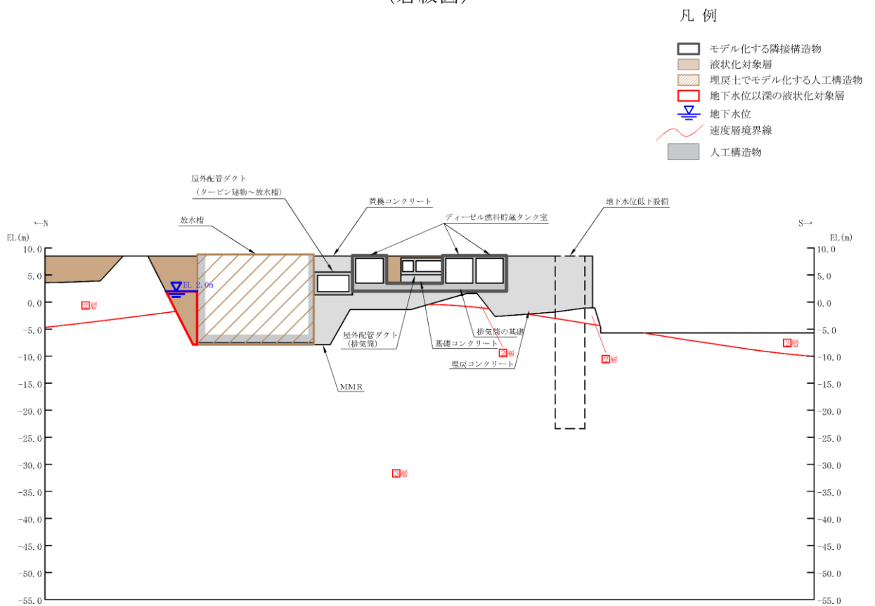
図 2-7 屋外配管ダクト (排気筒) 評価対象断面図 (A-A断面位置)
