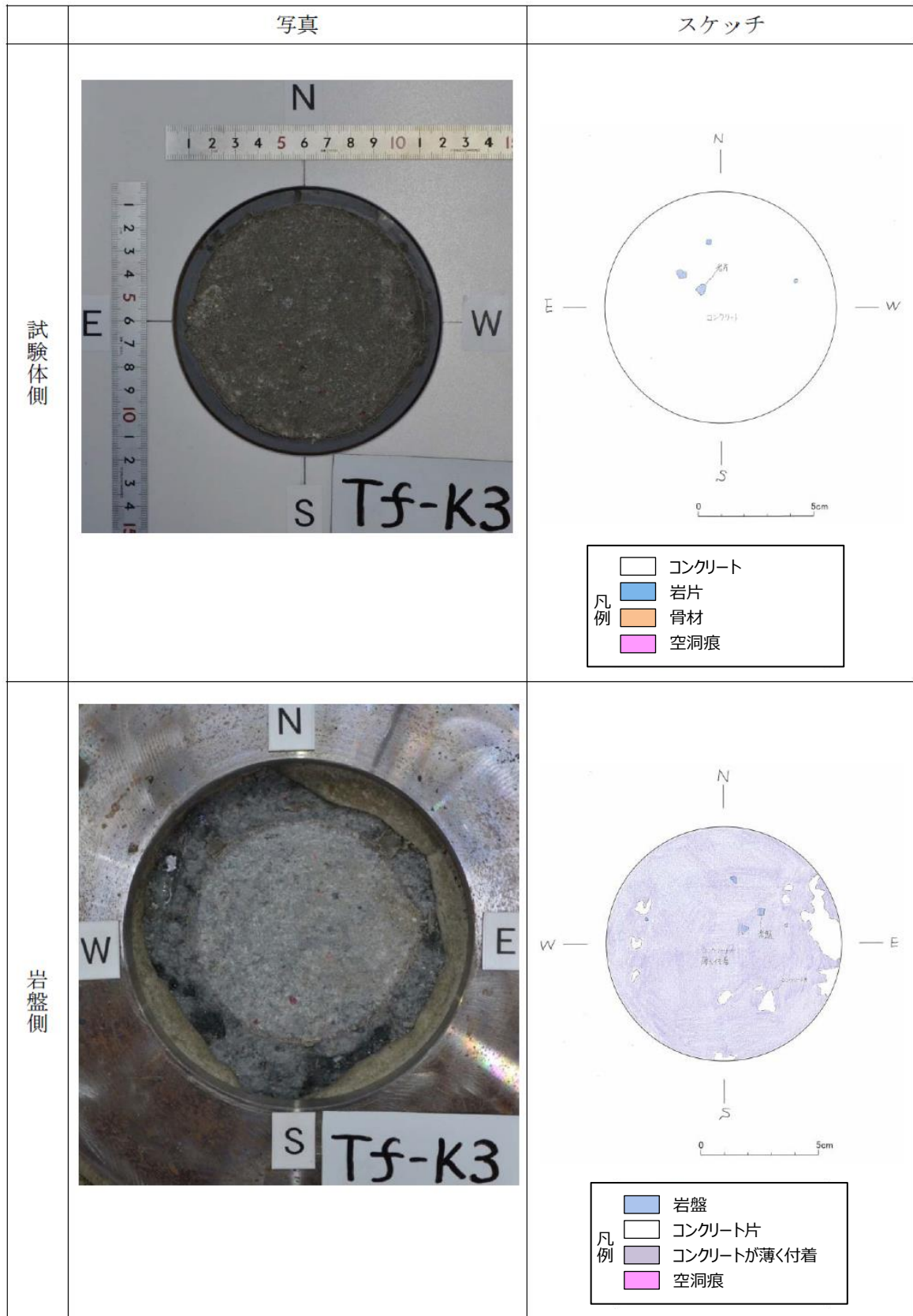
図 2-2 (10) 付着力試験後の破断面の状況 (凝灰岩-レベルコンクリート)
