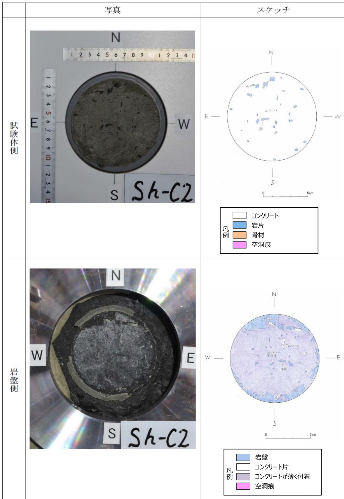
図 2-1 (8) 付着力試験後の破断面の状況 (黒色頁岩-レベルコンクリート)
