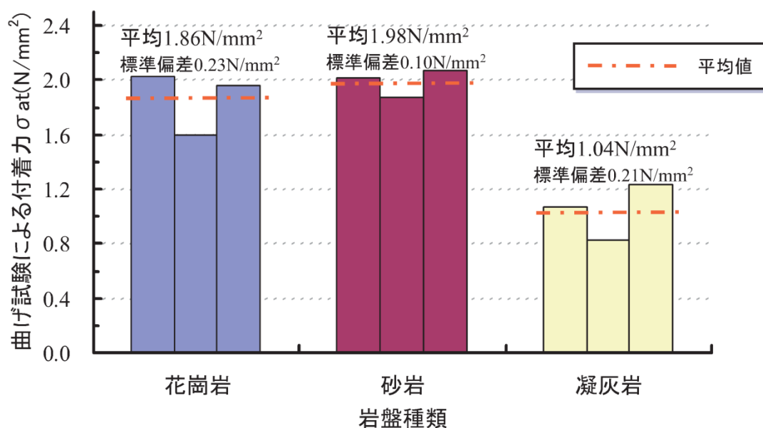
図 3-6 曲げ試験による付着力
