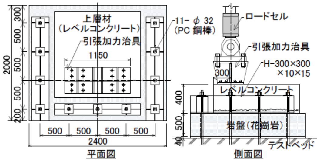
図 3-8 加力方法
