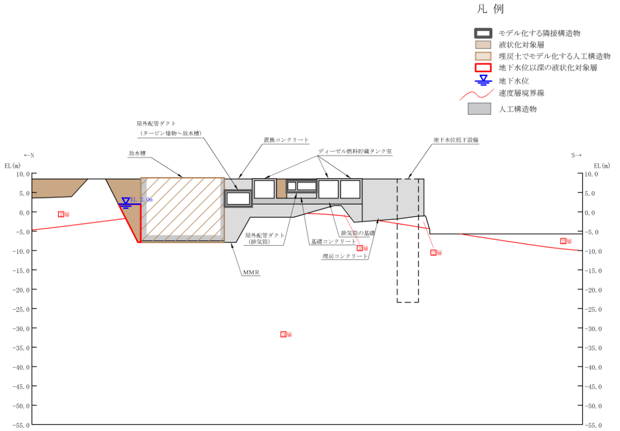
図 3-2 デーゼル燃料貯蔵タンク室 評価対象地質断面図 (A-A 断面位置)
