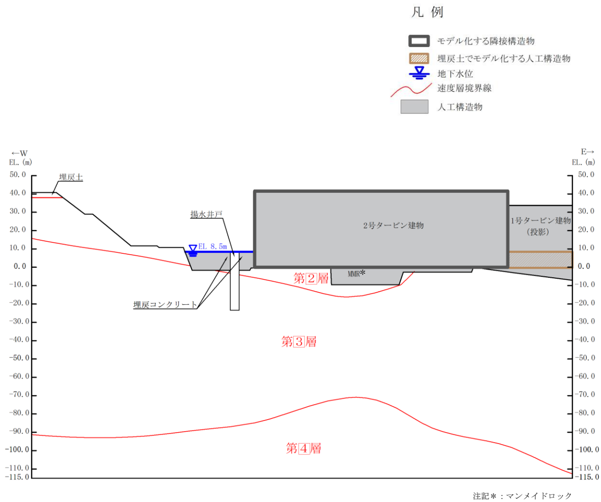
図 3-2 評価対象断面図 (A-A 断面 (東西方向))
