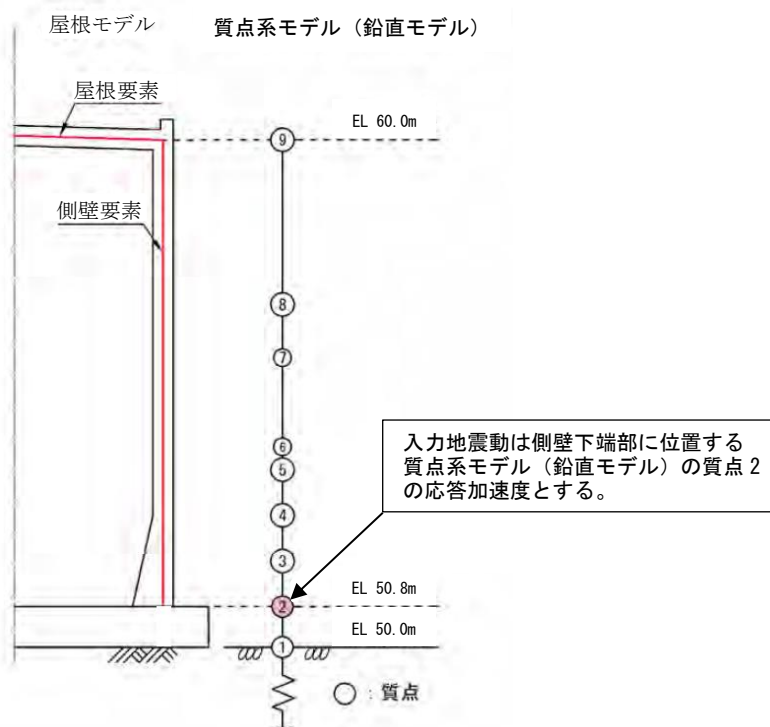
図 3.1-14 屋根モデルの入力地震動の概念図
