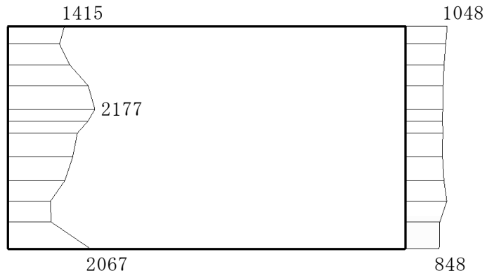
(a) S_s - D(++) 水平
