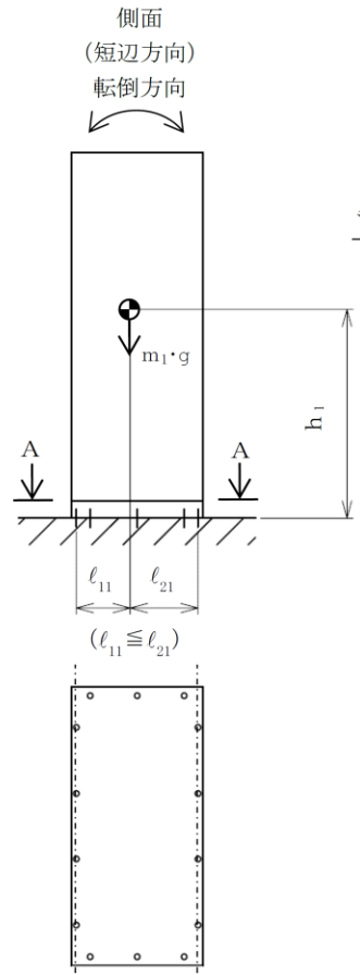
A~A 矢視図
