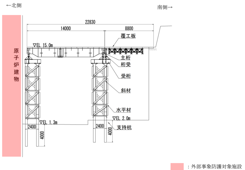
図 2-2 断面図 (A-A 断面)
