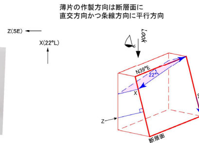
0 10cm 走向・傾斜 N39°E 80° SE X: 条線方向(下向きを正とする) Z: 断層面の法線方向(上壁側を正とする)
