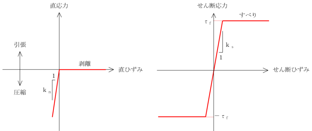
図 3.5.1-13 ジョイント要素の力学特性
