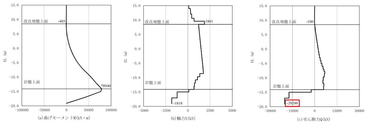
(改良地盤部 (②-②断面), S_s - D(-+) , t=14.97s )
