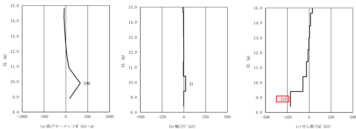
図 5.2.3-1(1) コンクリートのせん断破壊に対する照査に用いる断面力
