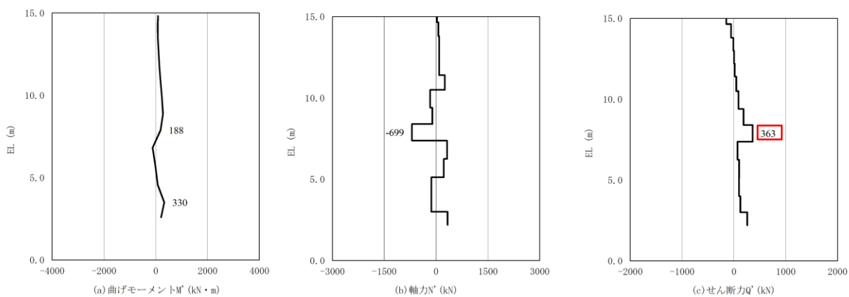
図 5.2.3-1(3) コンクリートのせん断破壊に対する照査に用いる断面力
