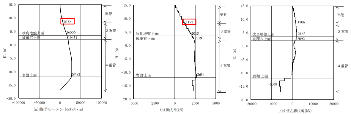
図 2.1-2(1) 単管部の鋼管杭の曲げ・軸力系の破壊に対する照査 における最大照査値の評価時刻での断面力 (③-③断面, S s - D (-+), t=9.55s , 単管部)
