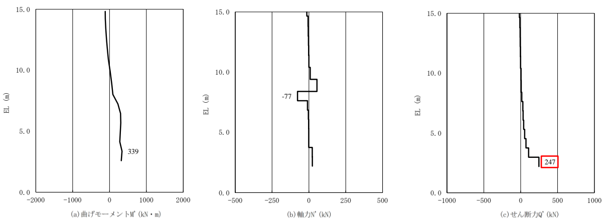
図 5.2.3-1(2) コンクリートのせん断破壊に対する照査に用いる断面力
