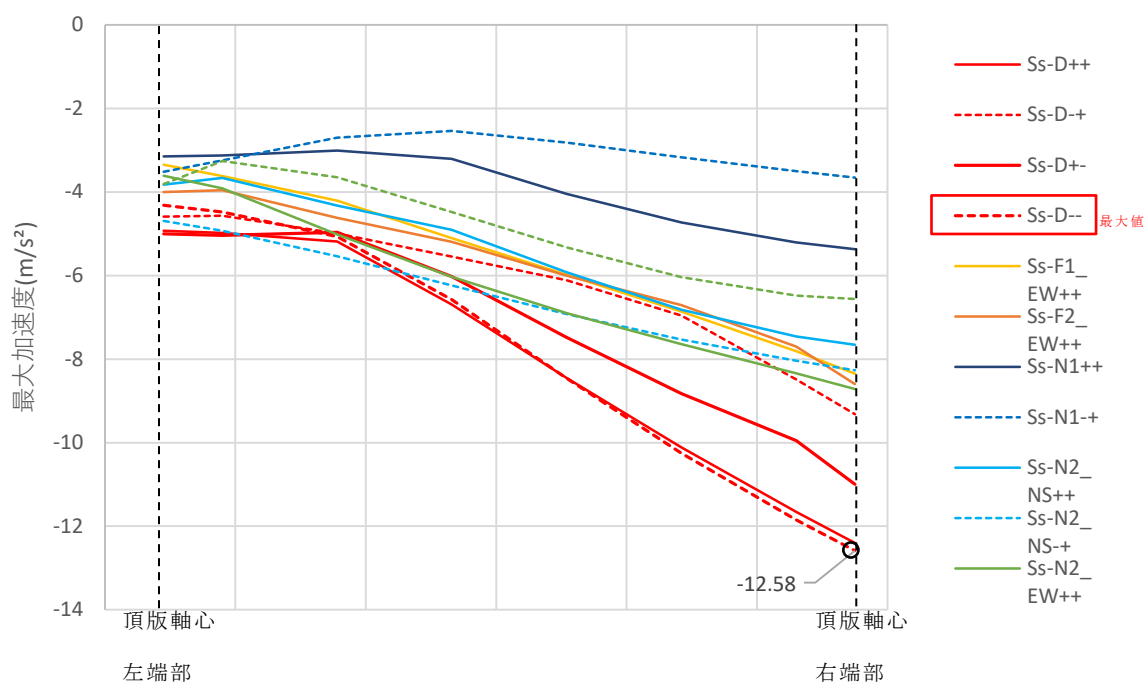
図 5-4 頂版に作用する加速度分布図（解析ケース①）
