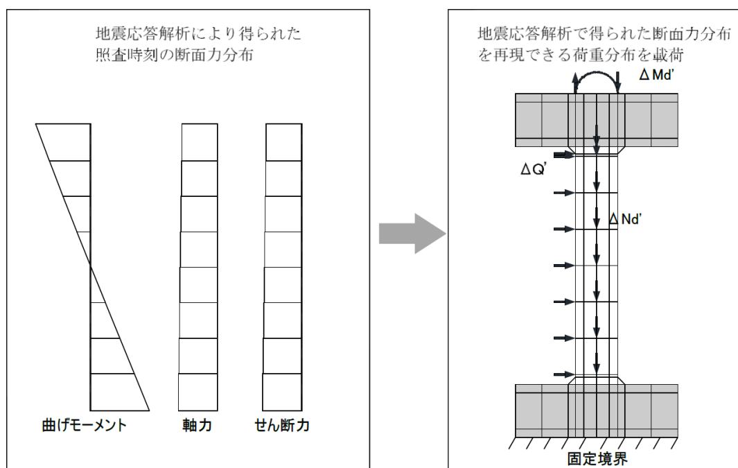
図 4-34 材料非線形解析における荷重状況
