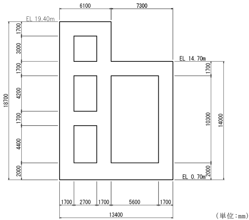
図 2-5 第 1 ベントフィルタ格納槽 断面図 (A-A断面)
