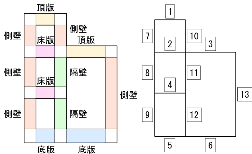
図2-21 評価部位位置図
