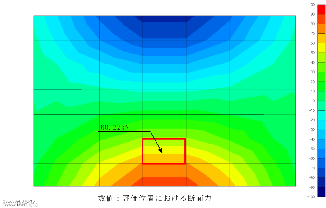
図 5-33 4 辺固定版における断面力図 (頂版, X 方向)
