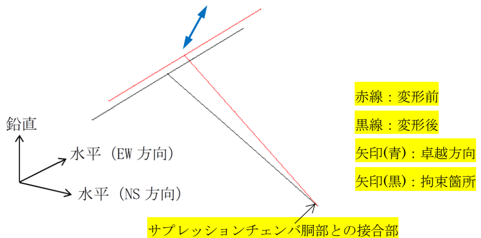
図 4-1 振動モード (1 次モード □ s)
