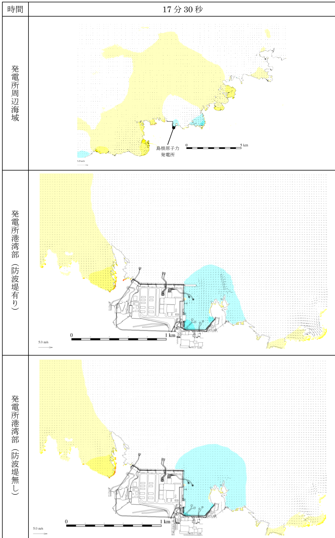
図 4-36 基準津波 4 の水位変動・流向ベクトル
