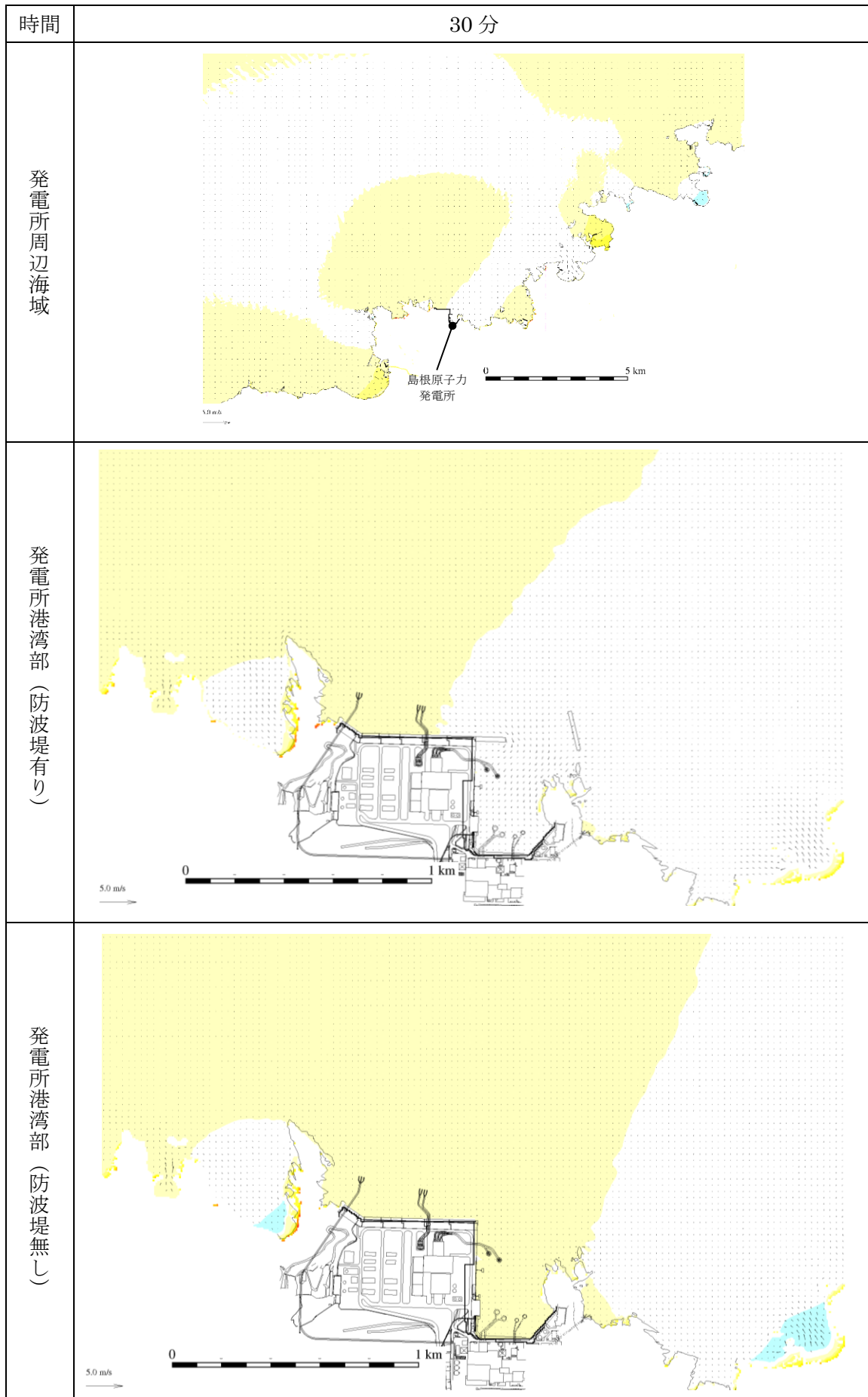
図 4-61 基準津波 4 の水位変動・流向ベクトル
