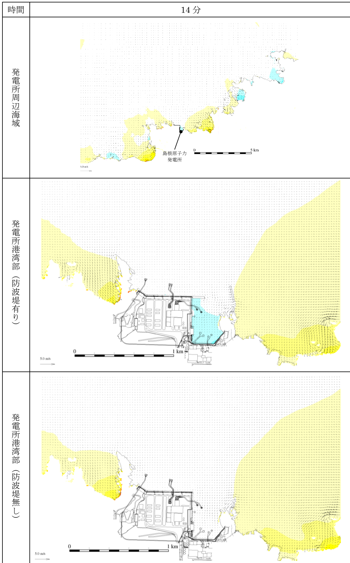
図 4-29 基準津波 4 の水位変動・流向ベクトル
