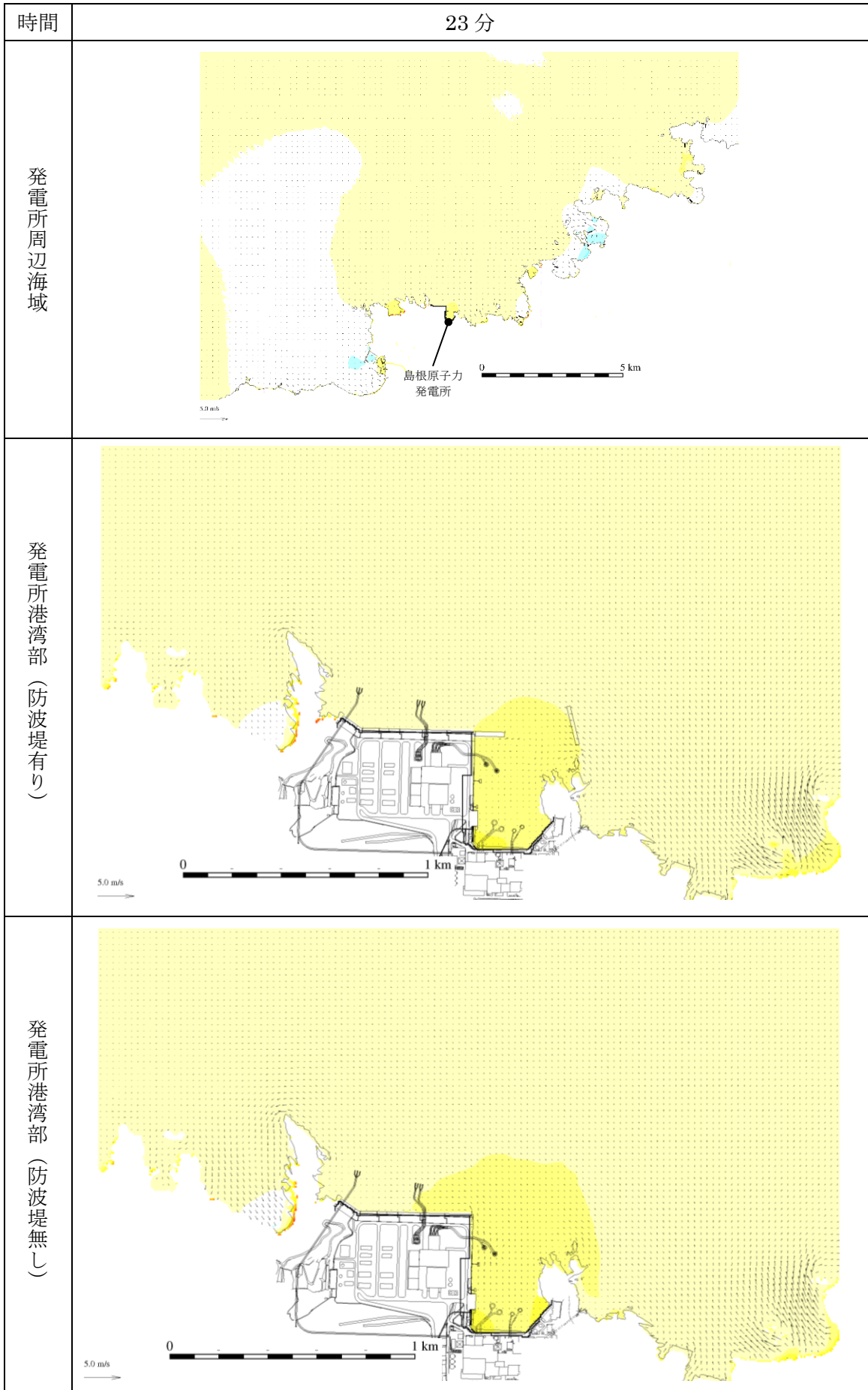
図 4-47 基準津波 4 の水位変動・流向ベクトル
