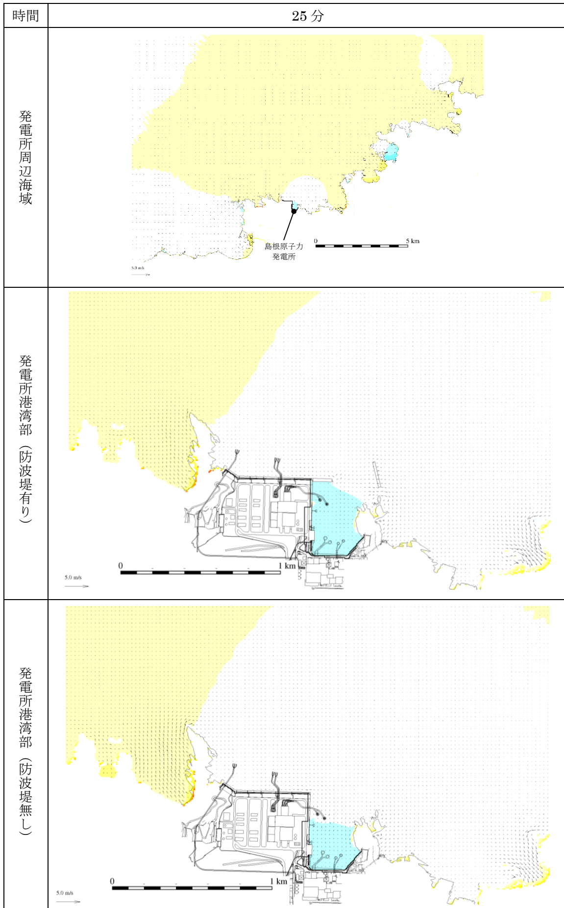
図 4-51 基準津波 4 の水位変動・流向ベクトル
