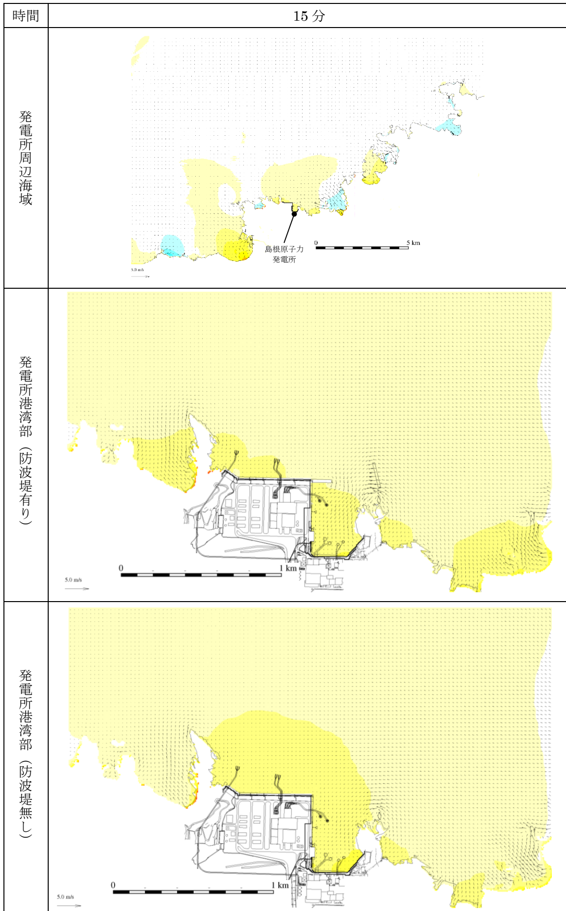
図 4-31 基準津波 4 の水位変動・流向ベクトル
