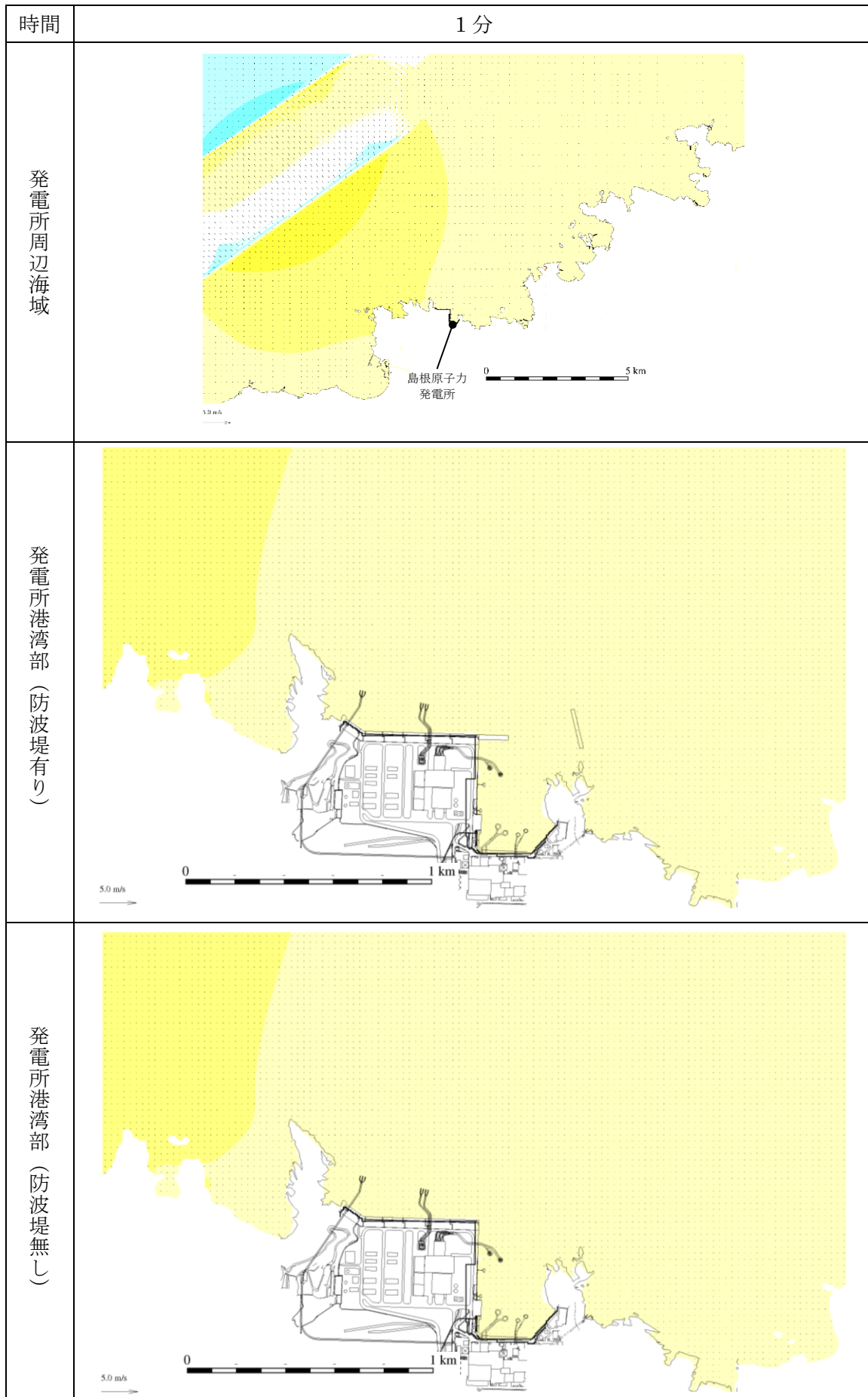
図 4-3 基準津波 4 の水位変動・流向ベクトル
