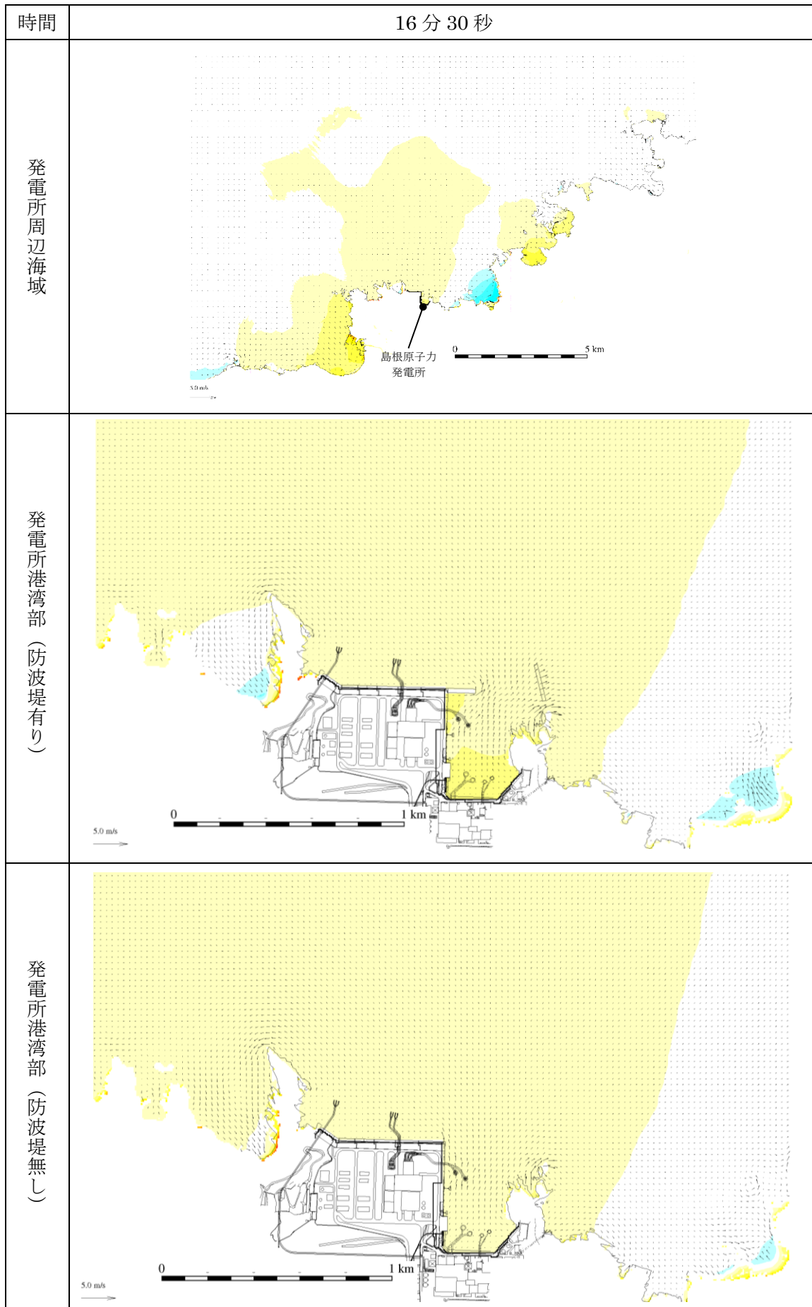
図 4-34 基準津波 4 の水位変動・流向ベクトル
