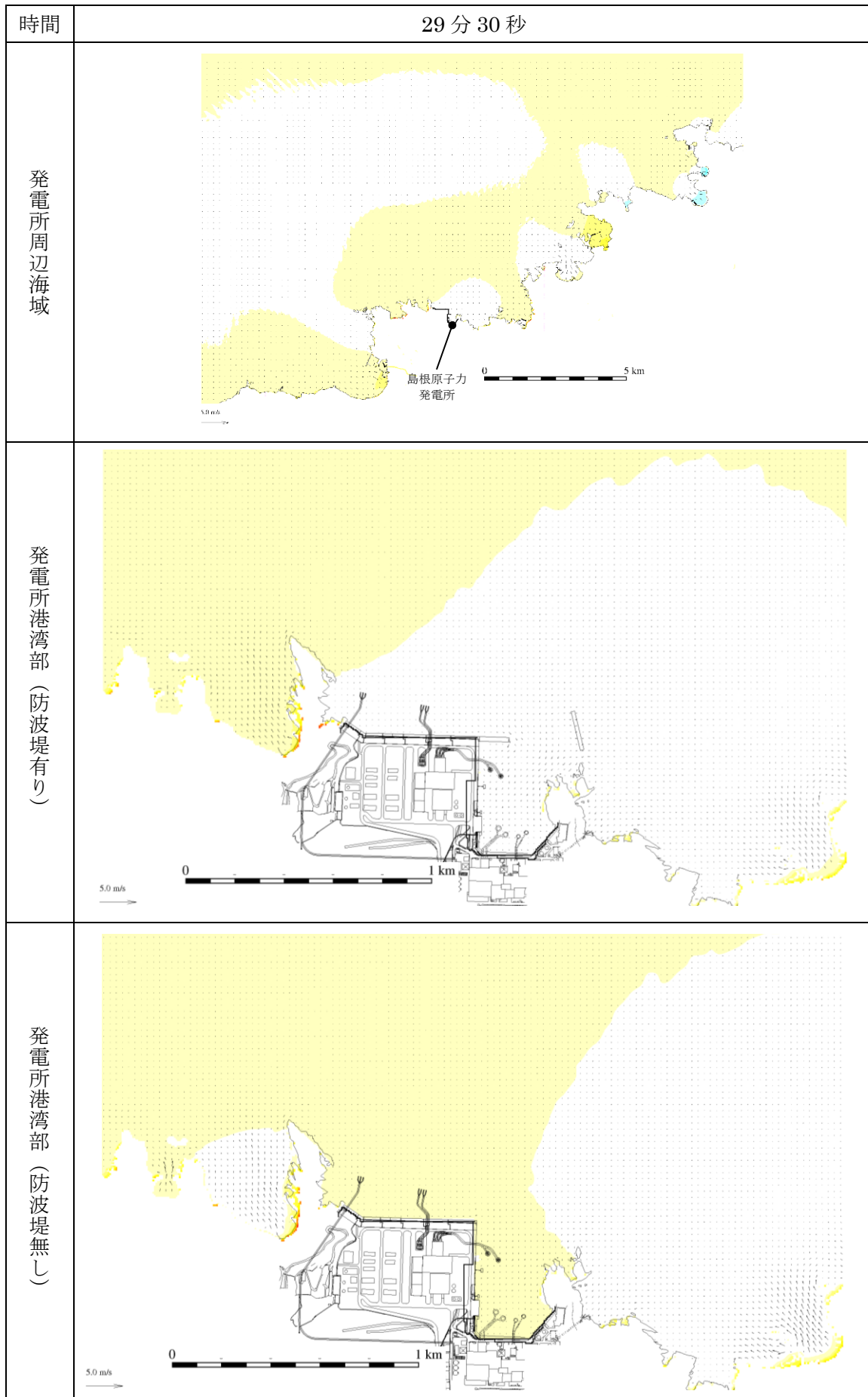
図 4-60 基準津波 4 の水位変動・流向ベクトル
