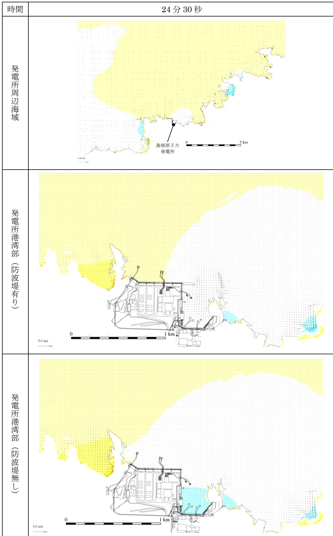
図 4-50 基準津波 4 の水位変動・流向ベクトル
