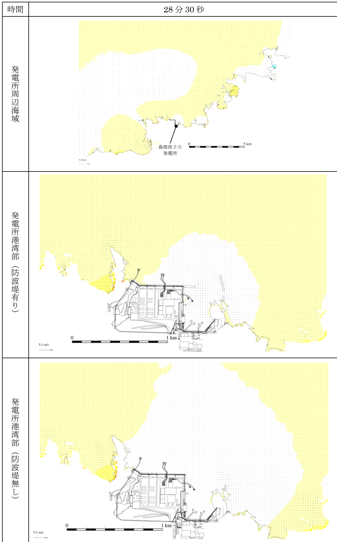
図 4-58 基準津波 4 の水位変動・流向ベクトル
