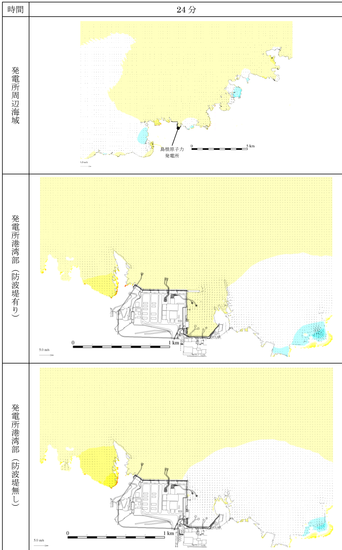
図 4-49 基準津波 4 の水位変動・流向ベクトル
