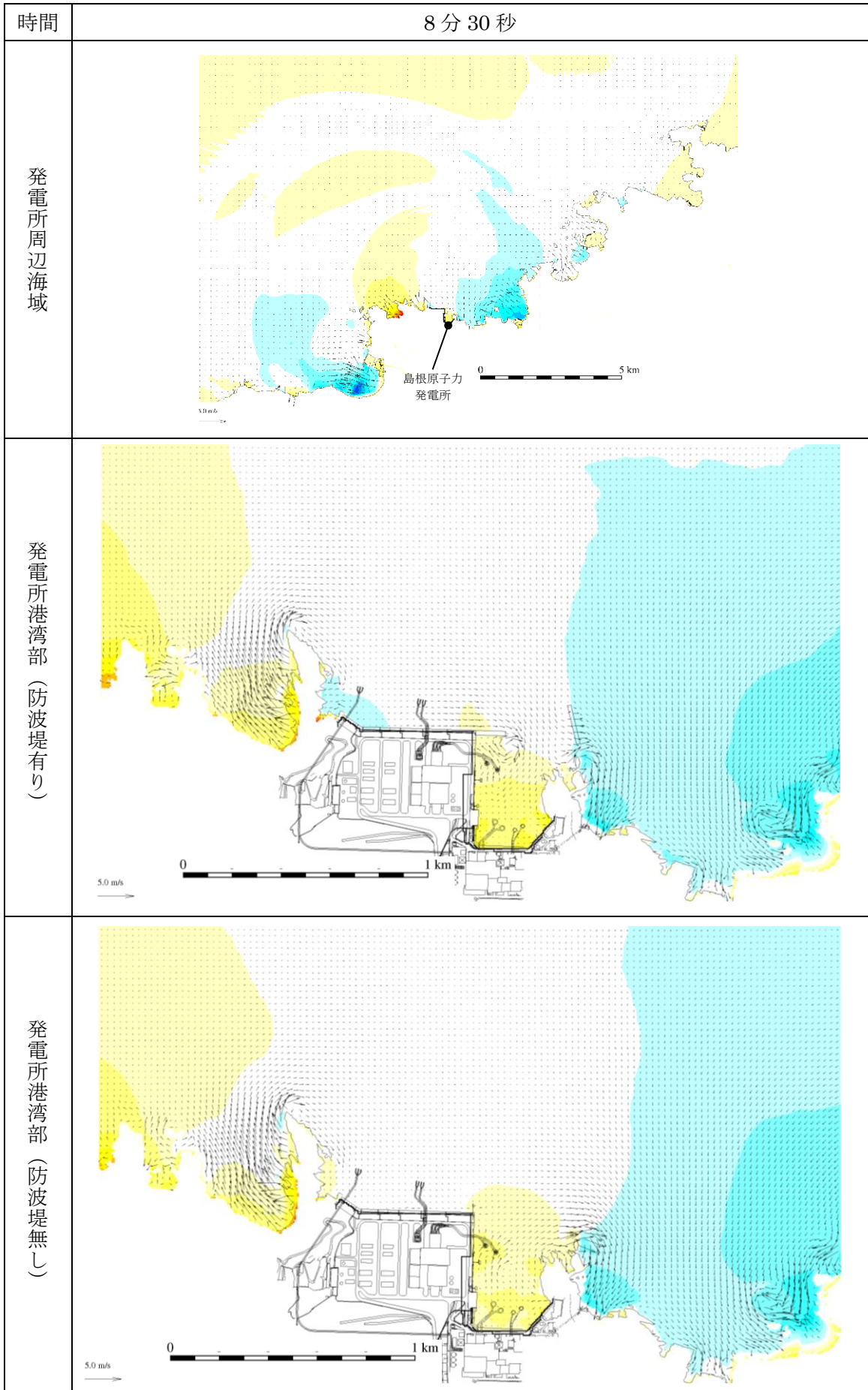
図 4-18 基準津波 4 の水位変動・流向ベクトル
