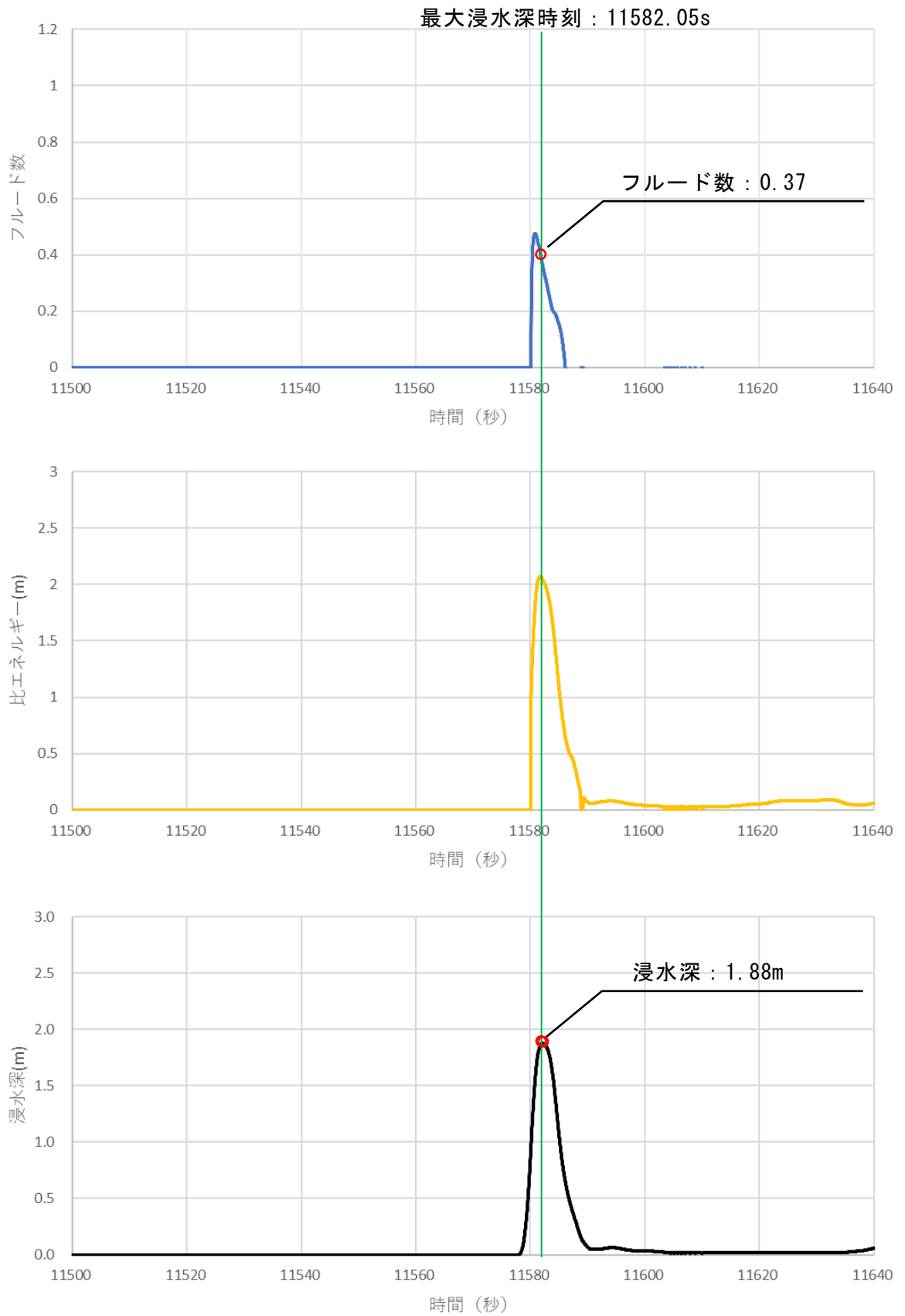
図 1.6.2-53 基準津波 1 を用いた防波壁無しの検討結果における フールド数、比エネルギー及び浸水深の時系列分布
