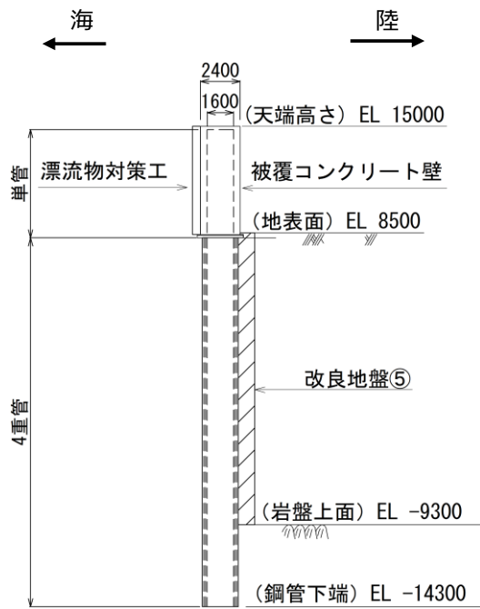
(断面図)
