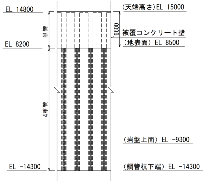
(正面図)
