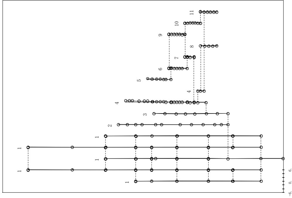
図 2.2.2-13 (16/40) 刺激関数 (第 8 次モード, N S 方向) : 今回工認モデル
