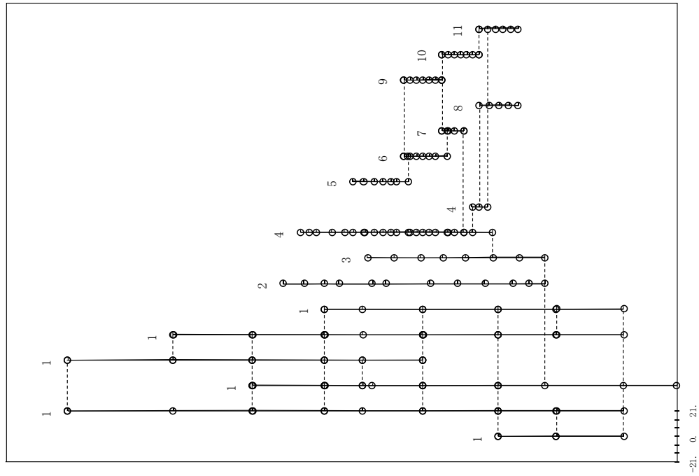
図 2.2.2-13 (40/40) 刺激関数 (第 10 次モード, EW方向) : 今回工認モデル
