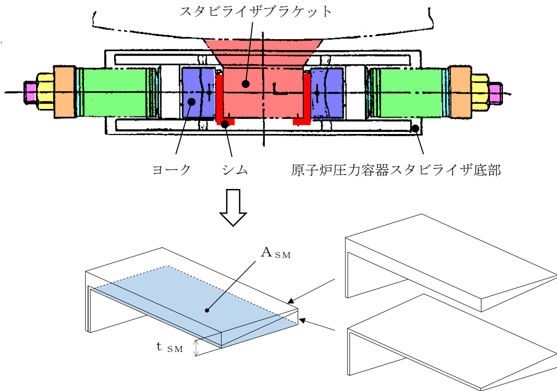
図 2.2.1.2.2-16 シム概略図
