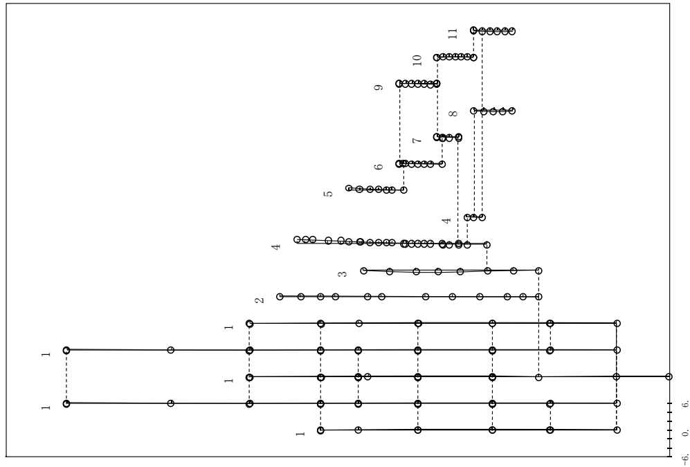
図 2.2.2-13 (15/40) 刺激関数 (第 8 次モード, N S 方向) : 影響検討モデル 3
