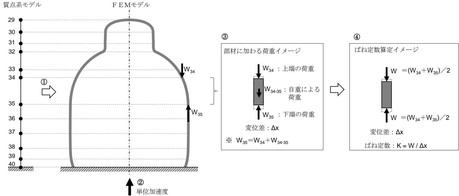
図 3. 3. 1-1 FEMモデルを用いた球殻部のばね定数算定方法
