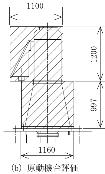
図 3-6 風荷重の受圧面積 (HPSWポンプ)
