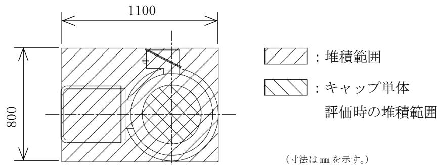
図 3-4 鉛直荷重の受圧面積 (HP SWポンプ)
