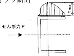
ギャラリ断面
