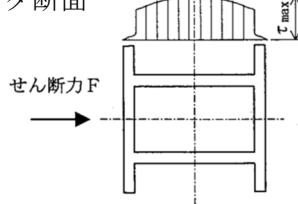
ガーダ断面
