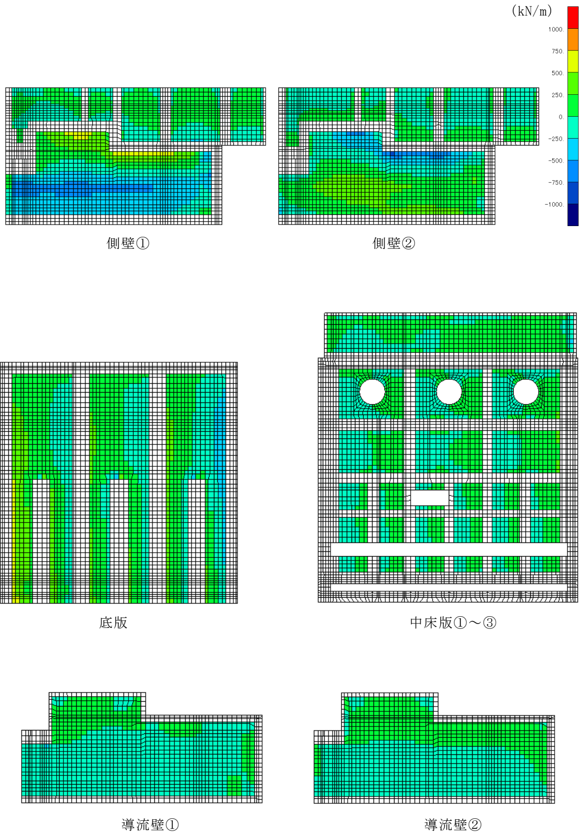
図 10-5(1) 静的地震力 ( K_h=0.16 (載荷方向: 東→西)) 載荷時の断面力分布図 (せん断力 (kN/m) : Q_x ) (参考) 6-26
