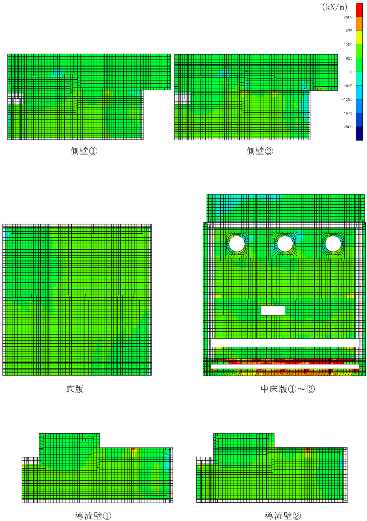
図 10-3(1) 静的地震力 ( K_h=0.16 (載荷方向: 東→西)) 載荷時の断面力分布図 (軸力 (kN/m) : N_x , 圧縮 : +) (参考) 6-20
