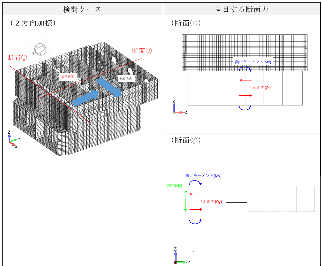
図3-11 着目する断面力
