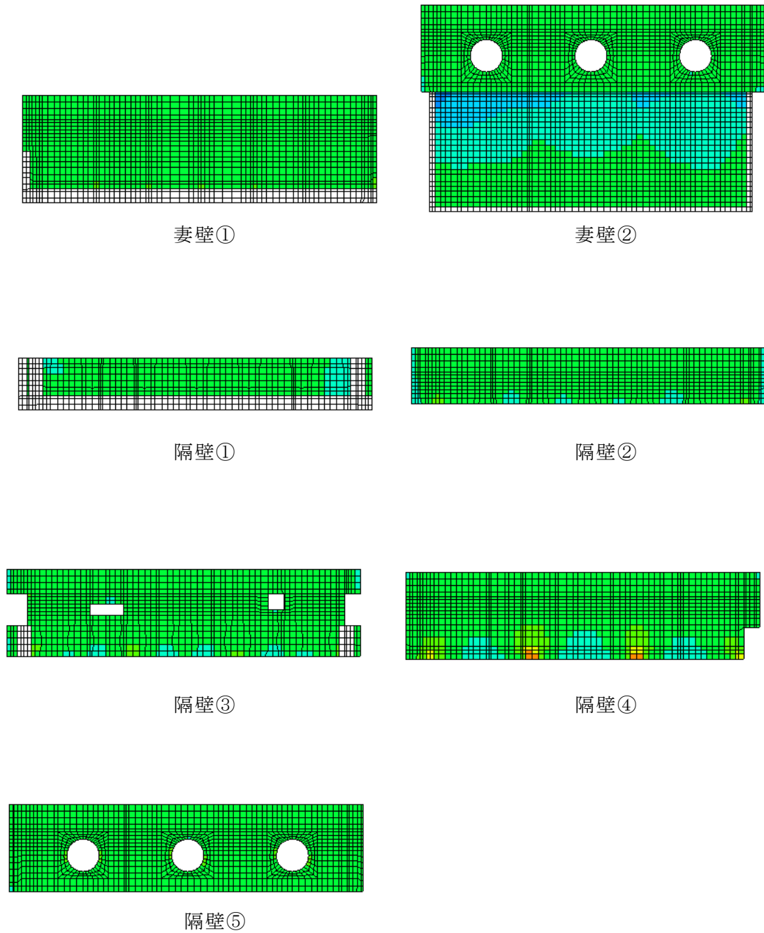
図 10-10(3) 静的地震力 ( K_h = -0.16 (載荷方向: 西→東)) 載荷時の断面力分布図 (軸力 (kN/m) : N_y , 圧縮 : +)
