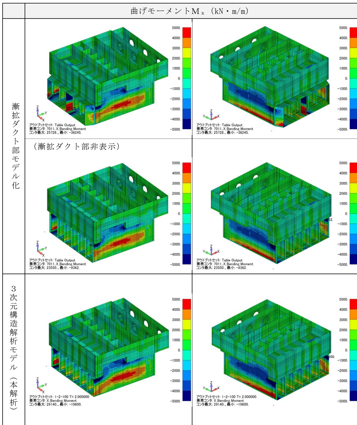
図 3-3 断面力図 (曲げモーメント M_x (kN・m/m), No. 1)
