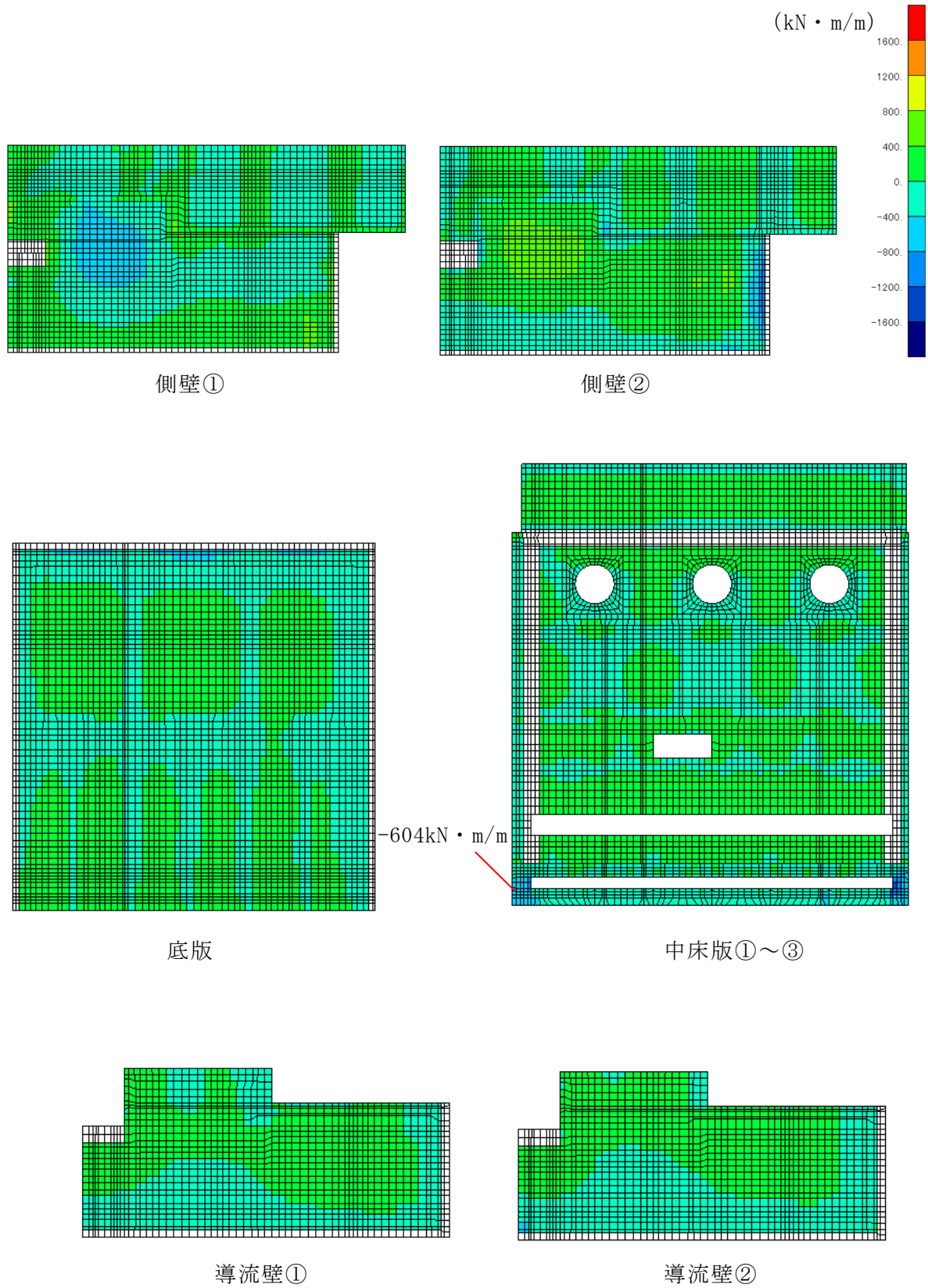
図 10-8(1) 静的地震力 ( K_h = -0.16 (荷重方向: 西→東)) 荷重時の断面力分布図 (曲げモーメント (kN · m/m) : M_y )
