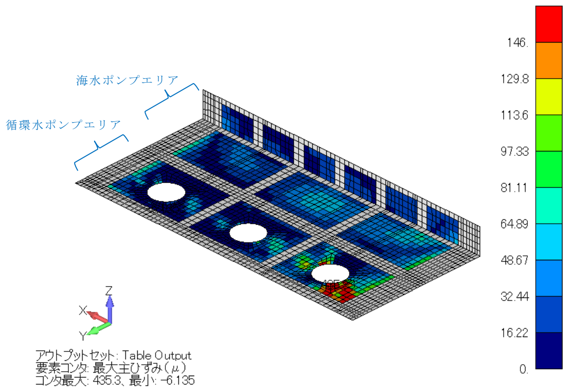
図 6-2 ひび割れ法線方向ひずみ分布
