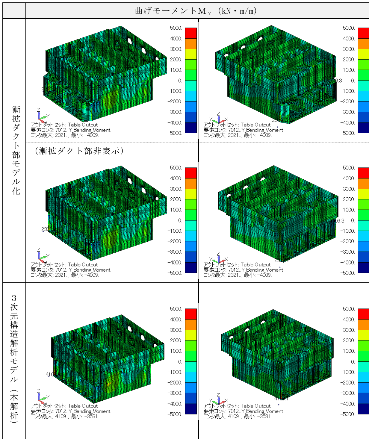
図 3-14 断面力図 (曲げモーメント M_y (kN・m/m), No. 2)
