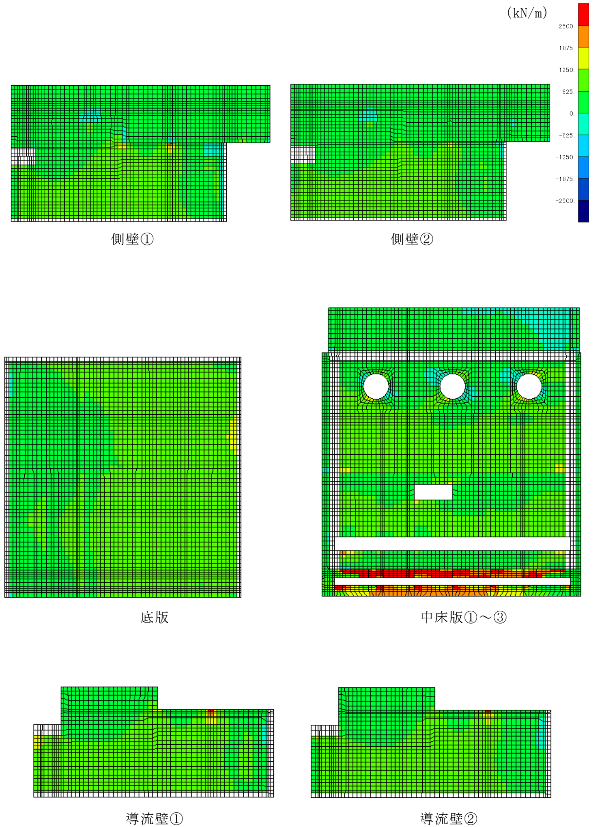
図 10-9(1) 静的地震力 ( K_h = -0.16 (載荷方向: 西→東)) 載荷時の断面力分布図 (軸力 (kN/m) : N_x , 圧縮: +) (参考) 6-38
