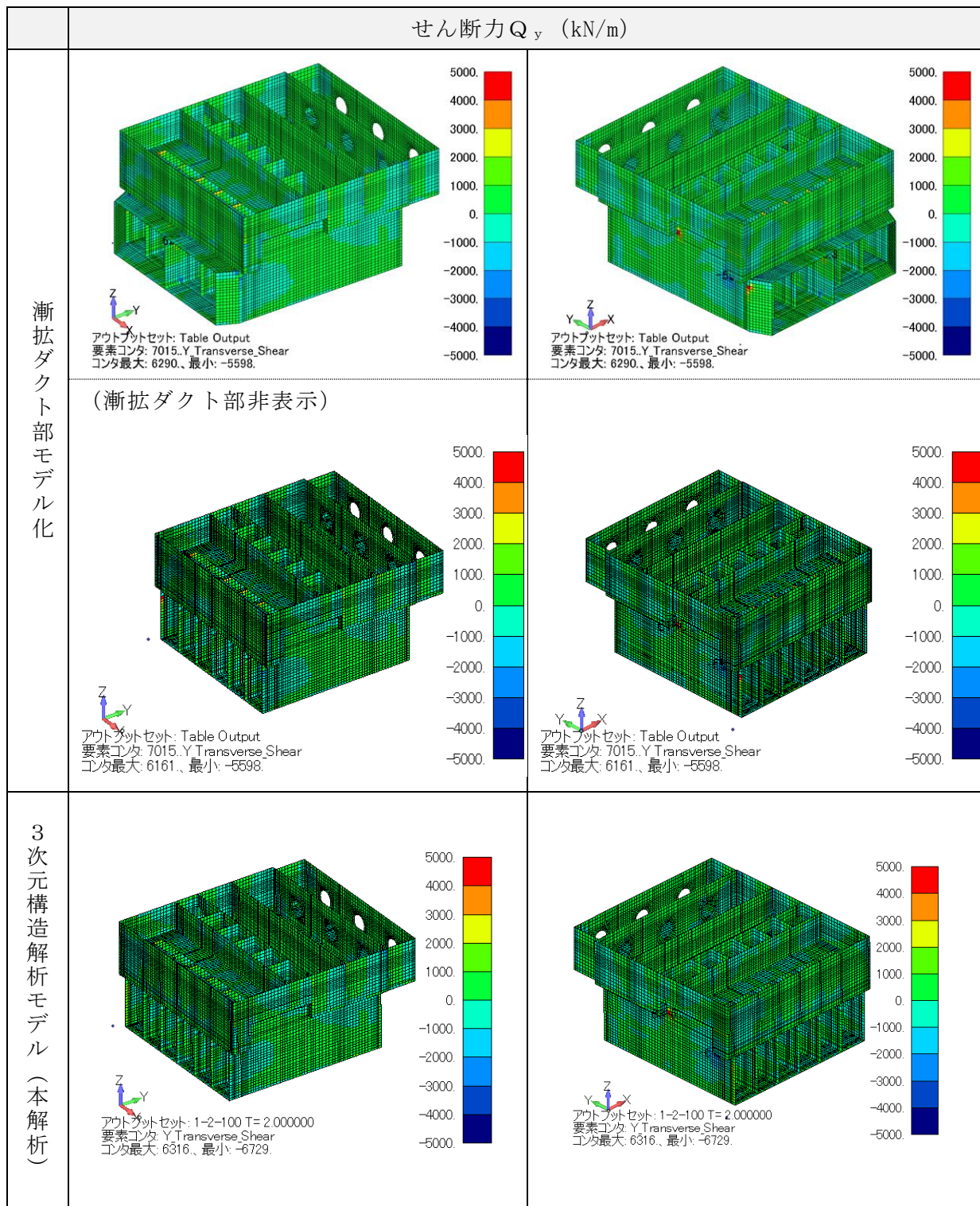
図 3-36 断面力図 (せん断力 Q_y (kN/m), No. 3)
