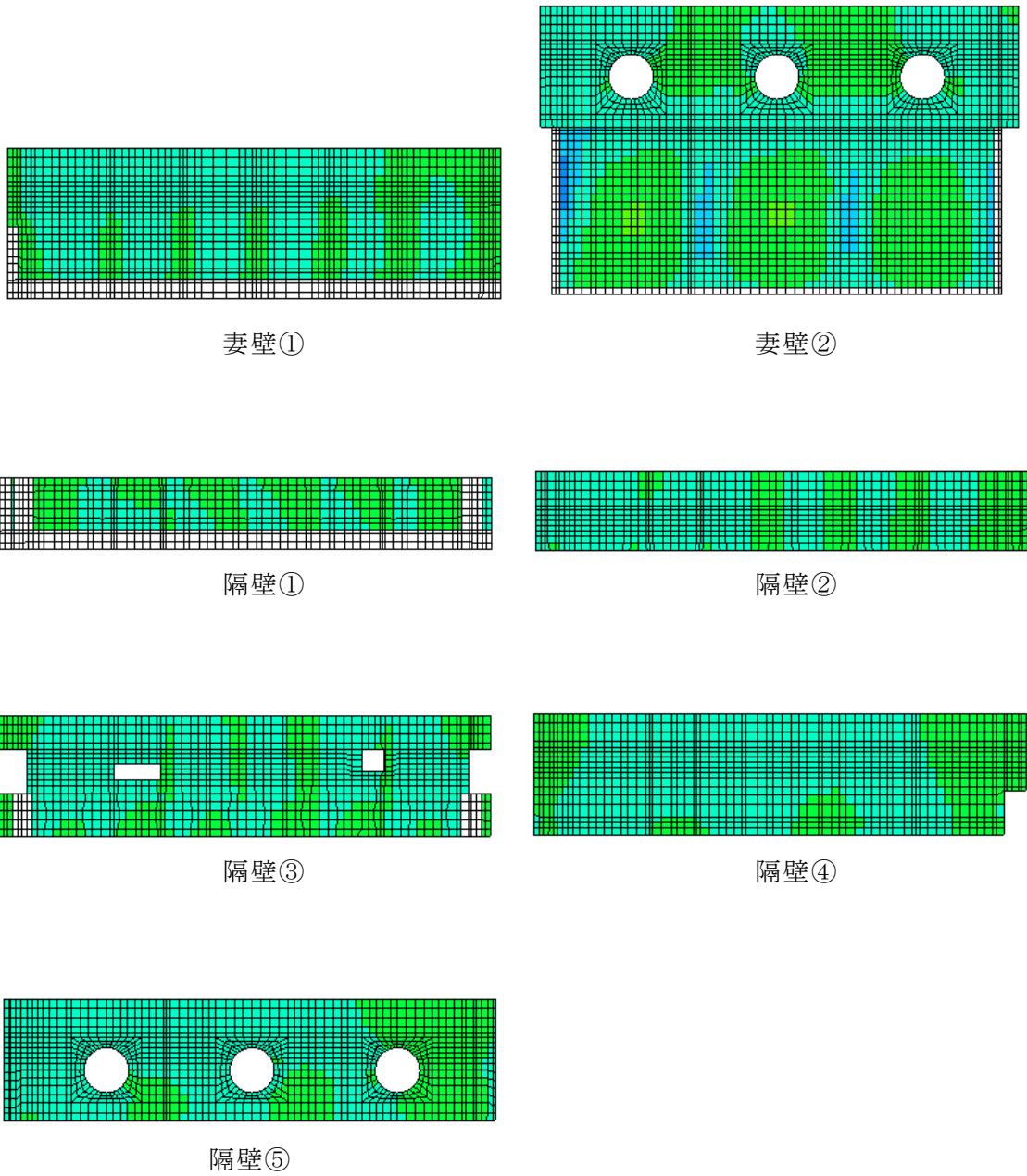
図 10-1(3) 静的地震力 ( K_h=0.16 (載荷方向：東→西)) 載荷時の断面力分布図 (曲げモーメント ( \text{kN}\cdot\text{m}/\text{m} ) : M_x )
