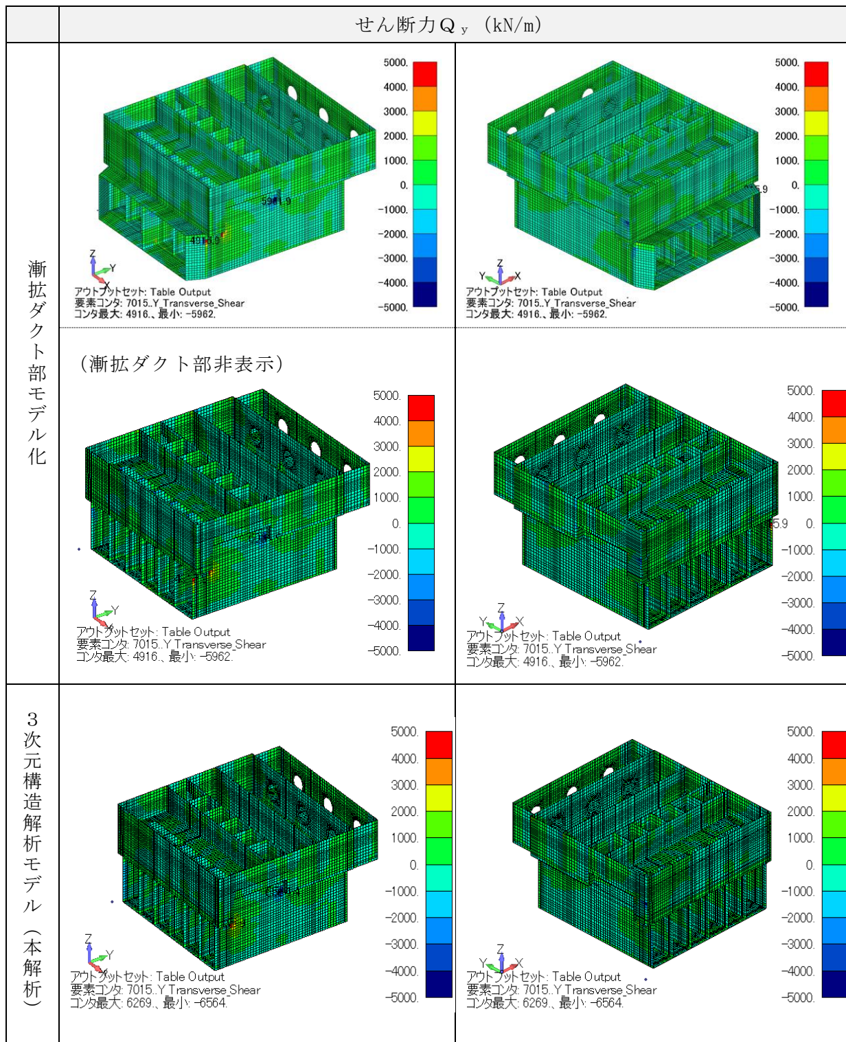
図 3-16 断面力図 (せん断力 Q_y (kN/m), No. 2)
