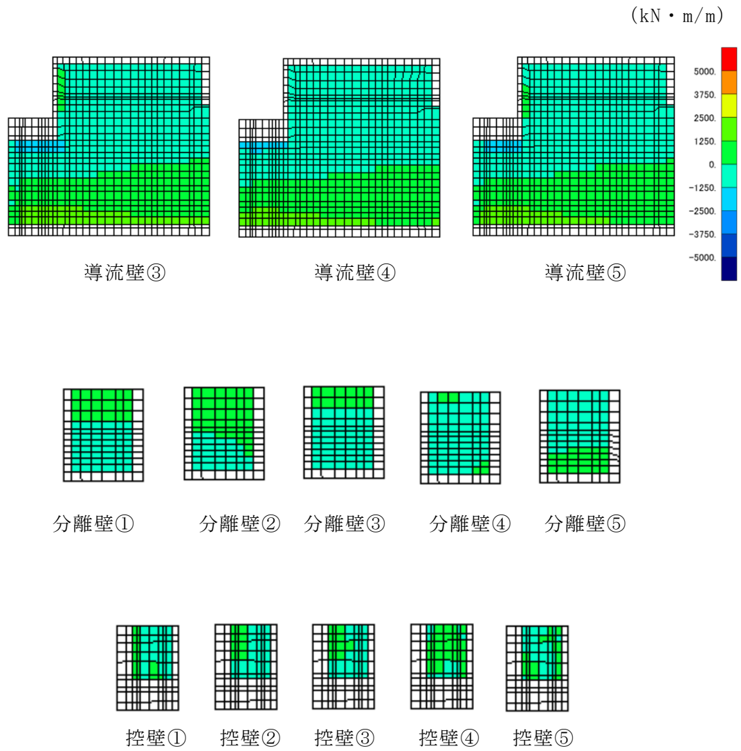
図 6-39 せん断破壊に対する照査値最大時の断面力分布図 (曲げモーメント (kN · m) : M_x ) (側壁, 解析ケース②, S_s - D (-+) )
