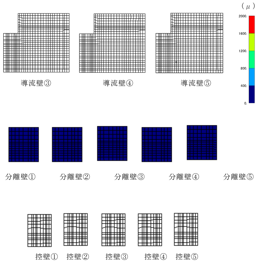
図 6-33 曲げ・軸力系の破壊に対する照査値最大時のひずみ分布図 (主筋ひずみ) (中床版, 解析ケース②, S_s - D (-+) )
