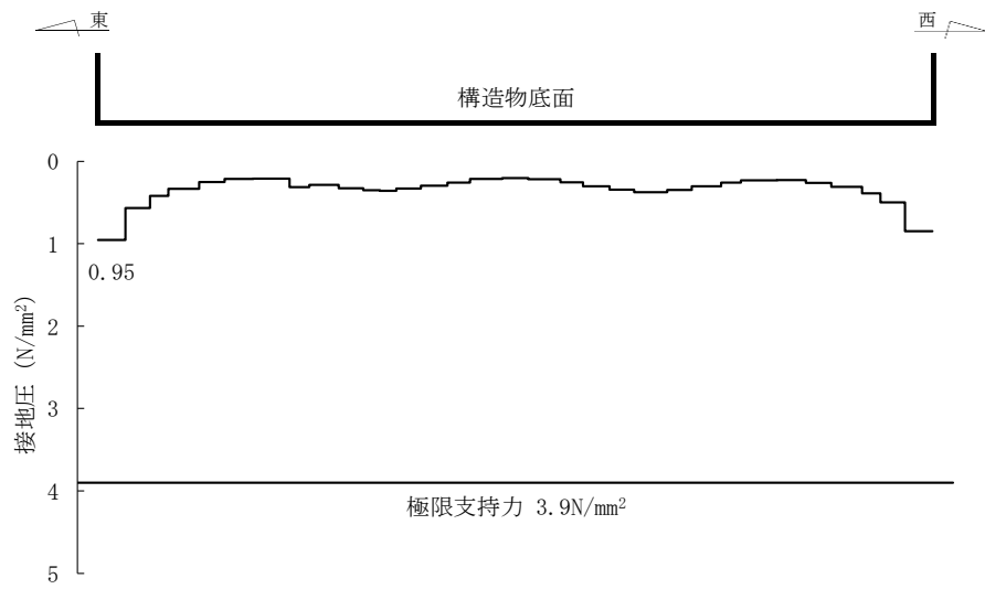
図 6-61 基礎地盤の最大接地圧分布図
