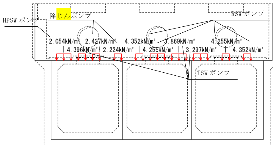
図 3-40 機器・配管の荷重図 (海水ポンプエリア)
