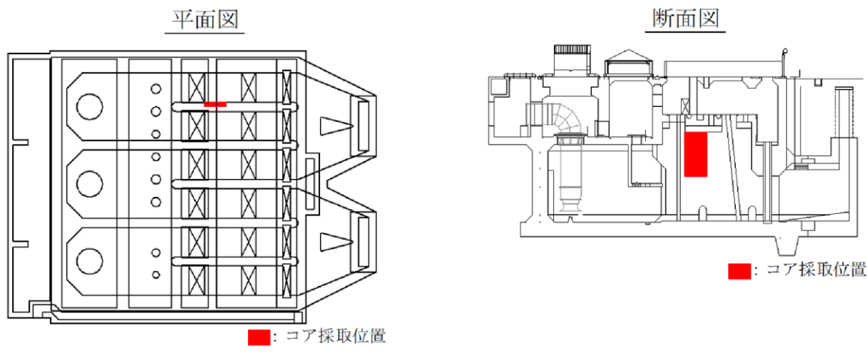
図 3-66 コア採取位置図
