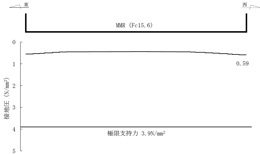
図 6-62 基礎地盤の最大接地圧分布図
