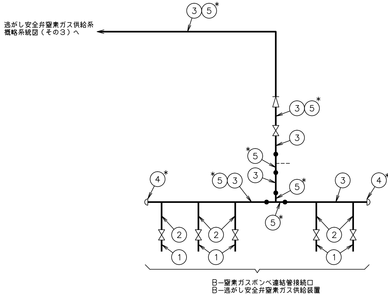
逃がし安全弁窒素ガス供給系概略系統図(その4)
