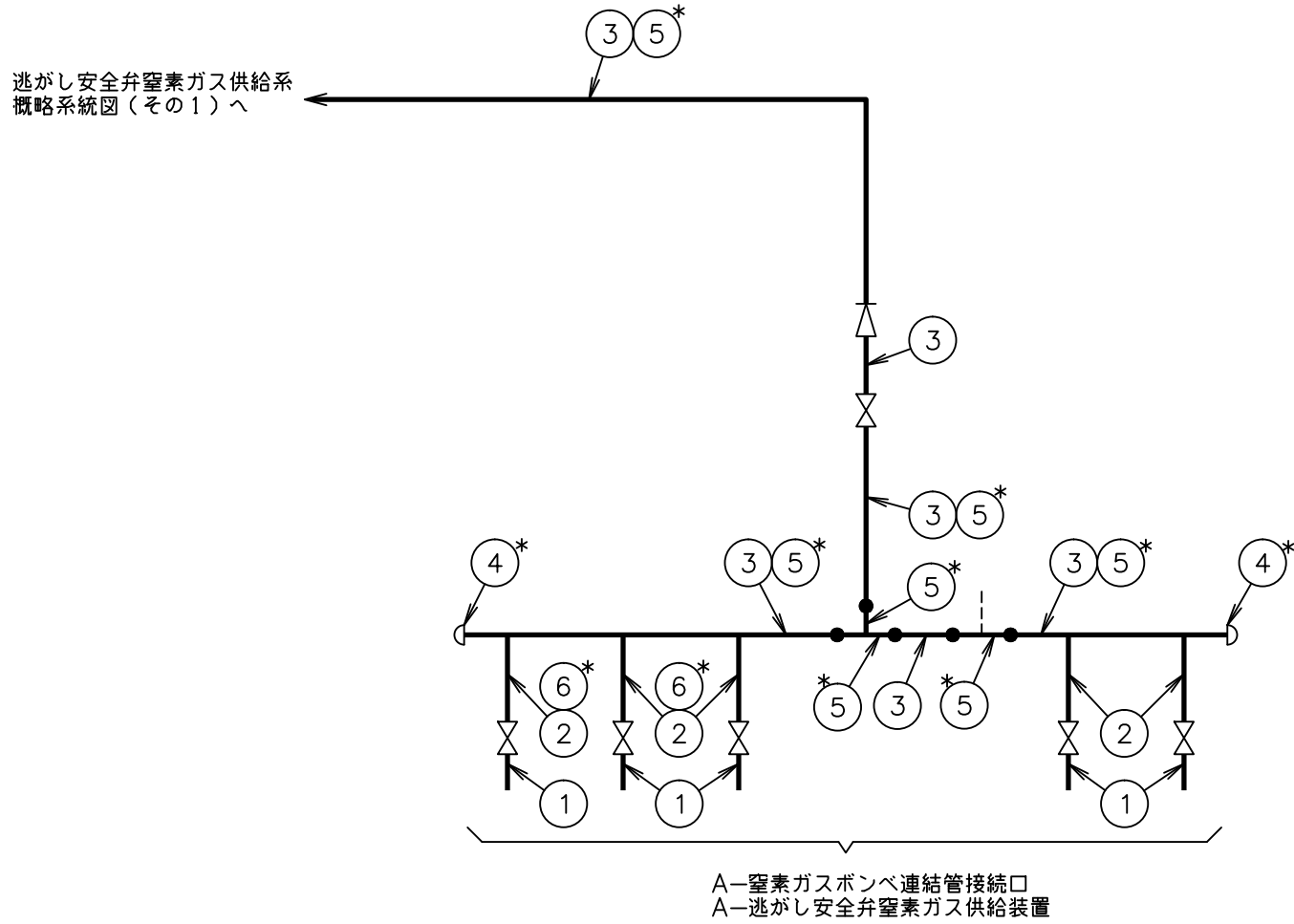
注記*：管継手 逃がし安全弁窒素ガス供給系概略系統図(その2)
