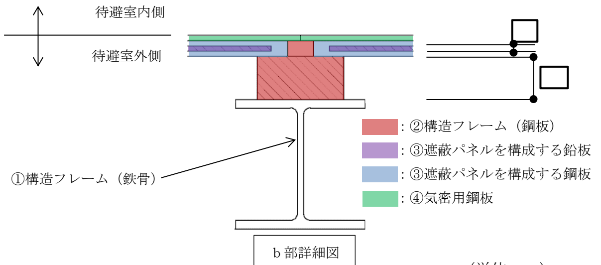
図 2-3 中央制御室待避室の概略断面図 (A-A)
